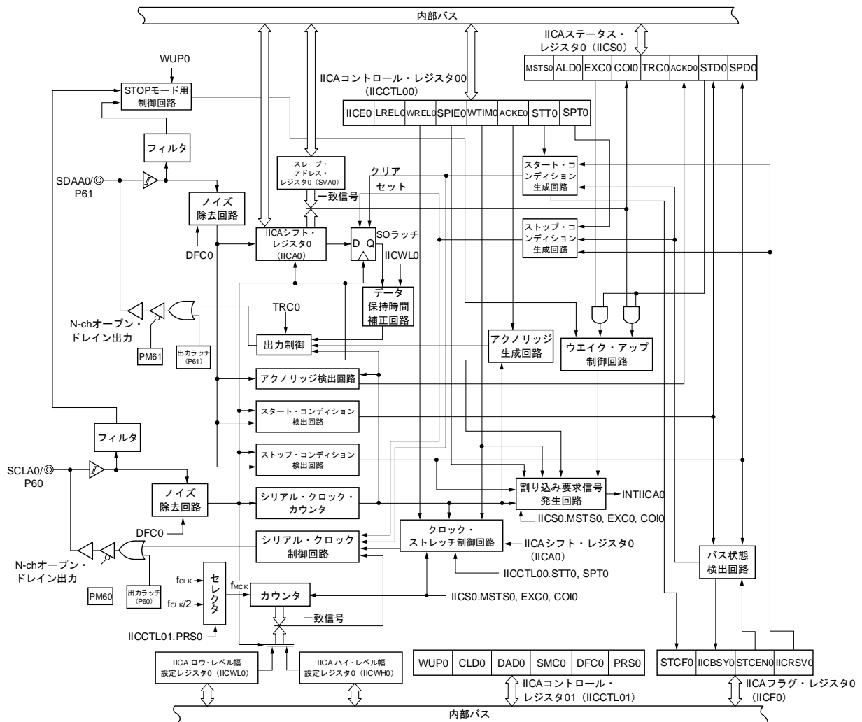
図13-1 シリアル・インタフェースIICA0のブロック図
