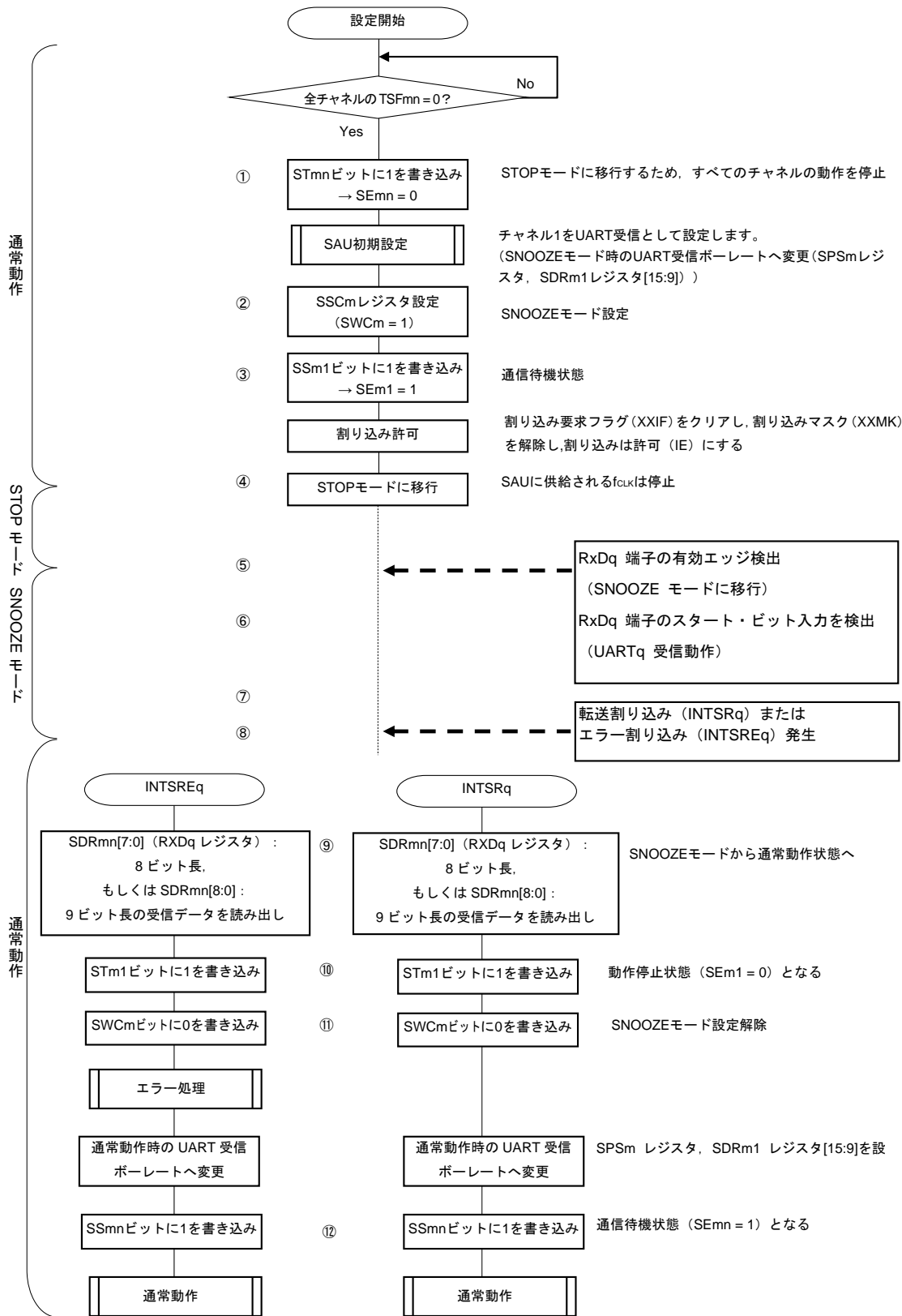
図12-92 SNOOZEモード動作 (EOCm1 = 0, SSECm = 0/1 もしくは EOCm1 = 1, SSECm = 0) 時の フロー・チャート
