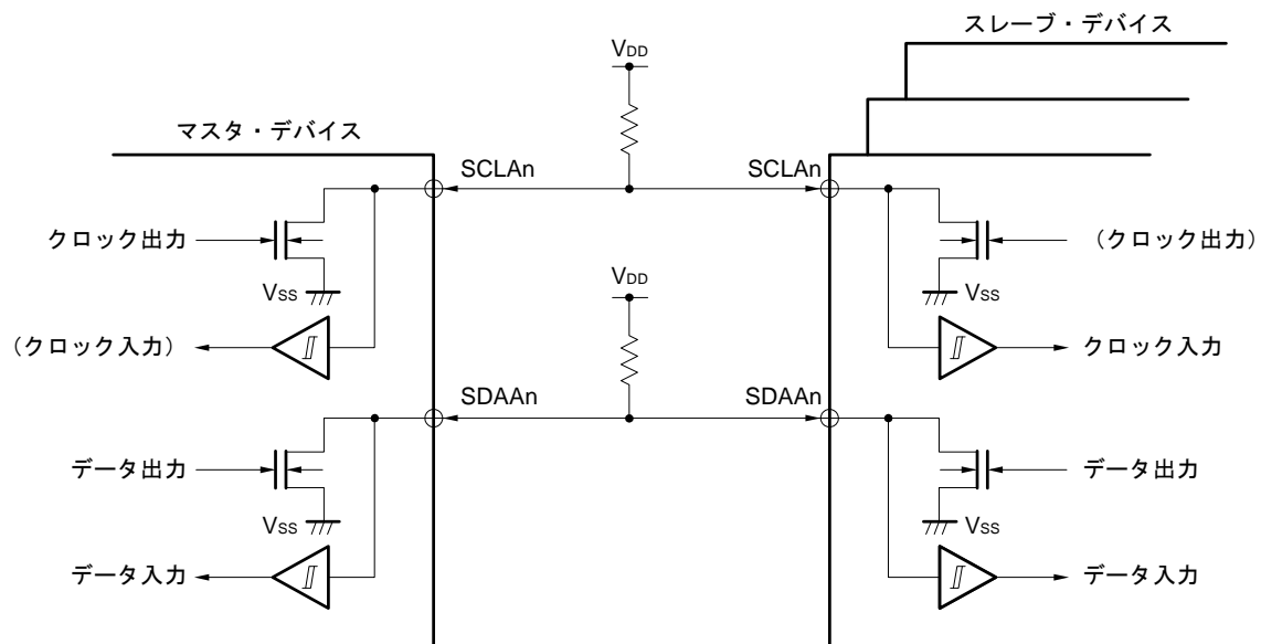
図13-13 端子構成図
