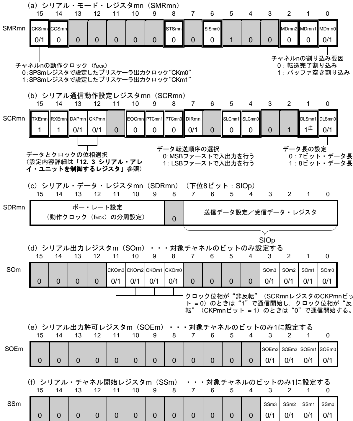
図12-41 簡易SPI (CSI00, CSI01, CSI10, CSI11, CSI20, CSI21, CSI30, CSI31) のマスタ送受信時の
