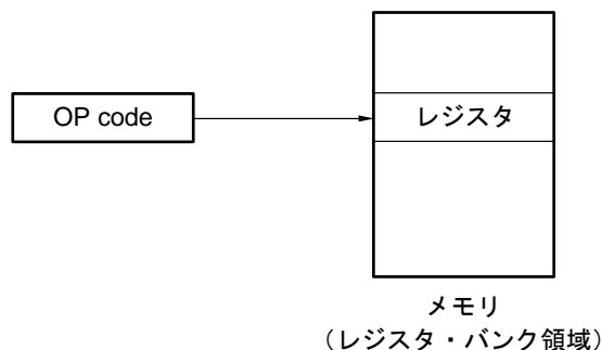
図3-25 レジスタ・アドレッシングの概略
