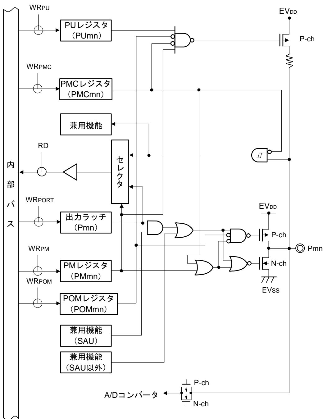
図2-9 端子タイプ 7-3-2 の端子ブロック図
