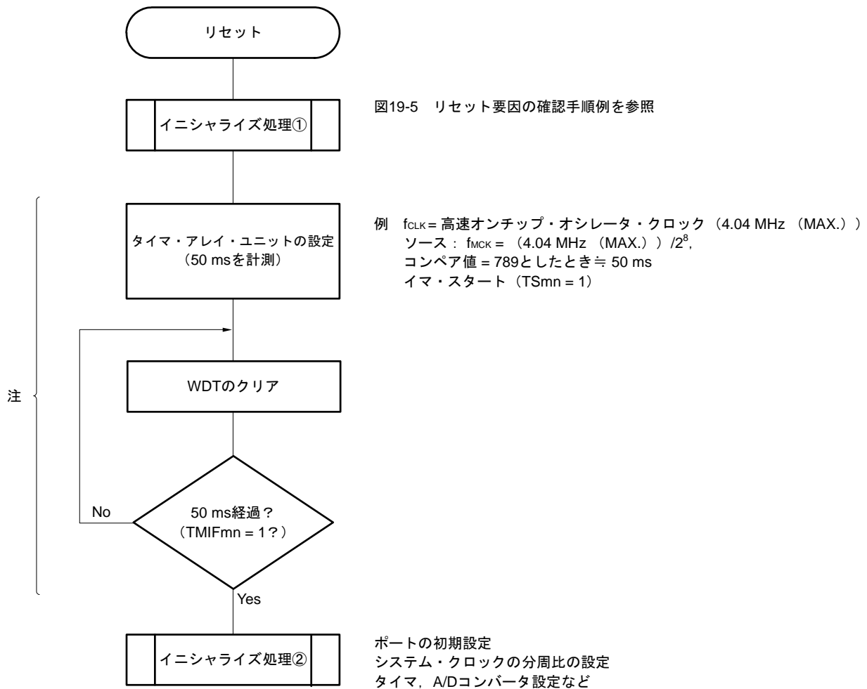
図21-10 LVD検出電圧付近での電源電圧変動が50 ms以下の場合のソフト処理例
