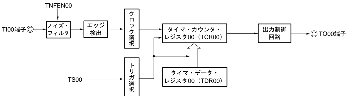
図6-49 分周器としての動作のブロック図
