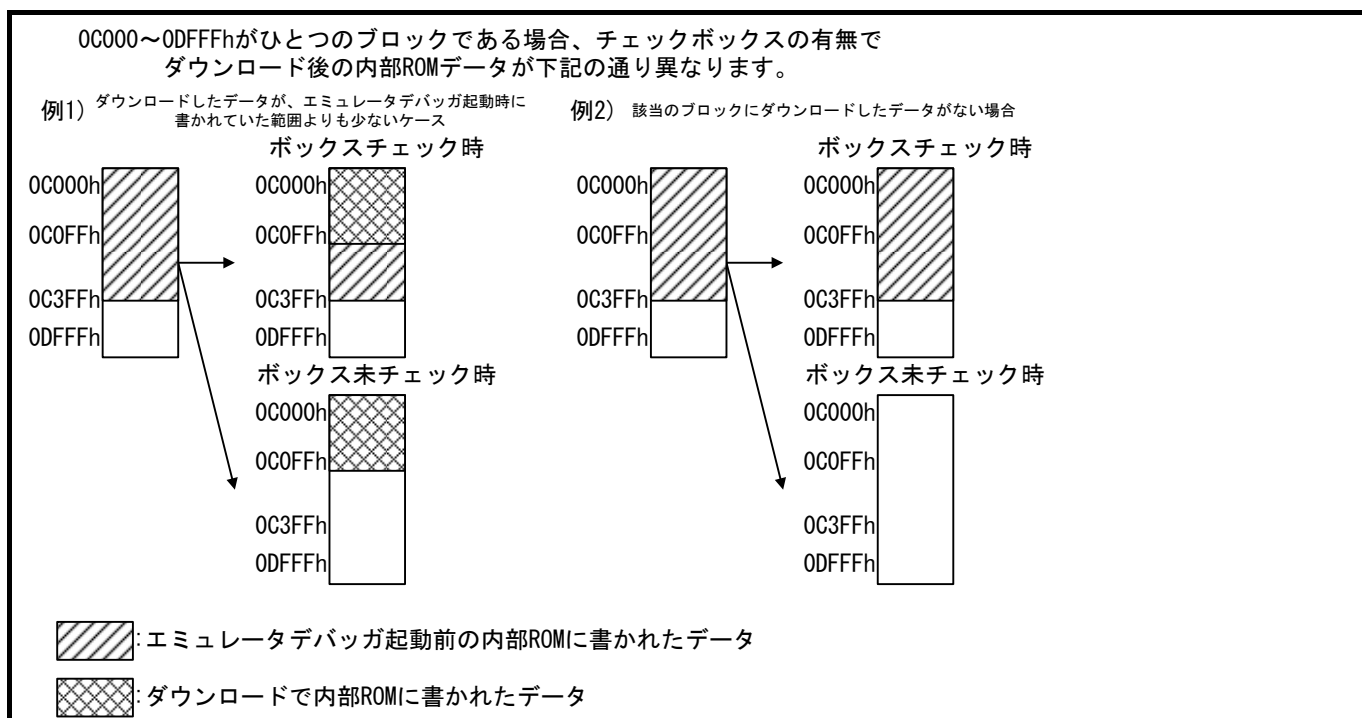
図 4.34 チェックボックスのチェック有無による、ダウンロード後の内部ROMデータの差異
