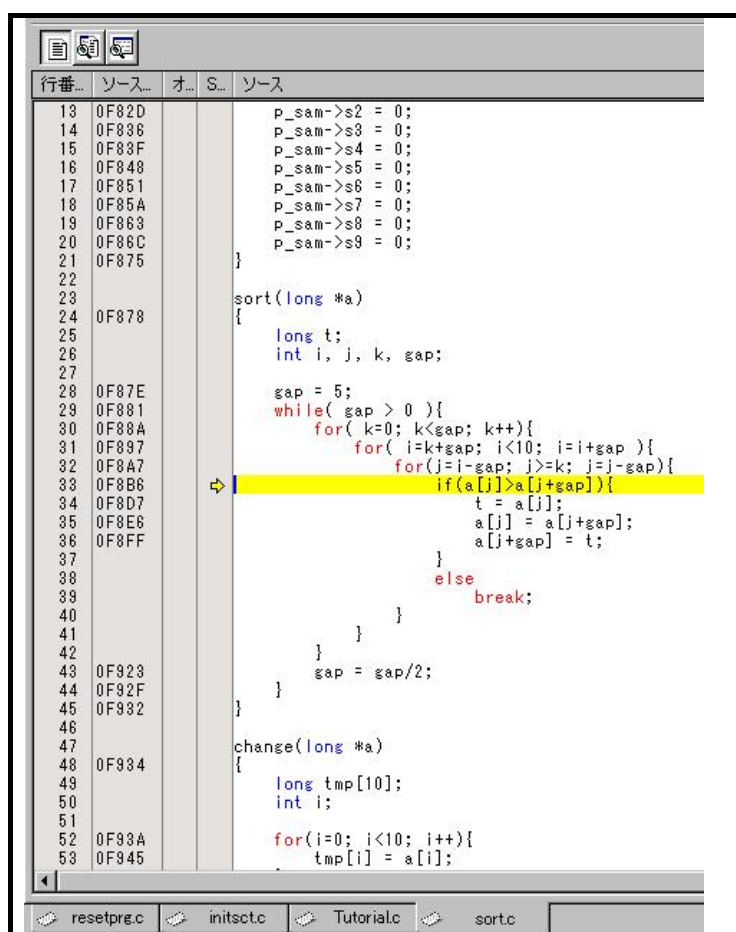
図 6.19 [エディタ]ウィンドウ (ステップイン)
