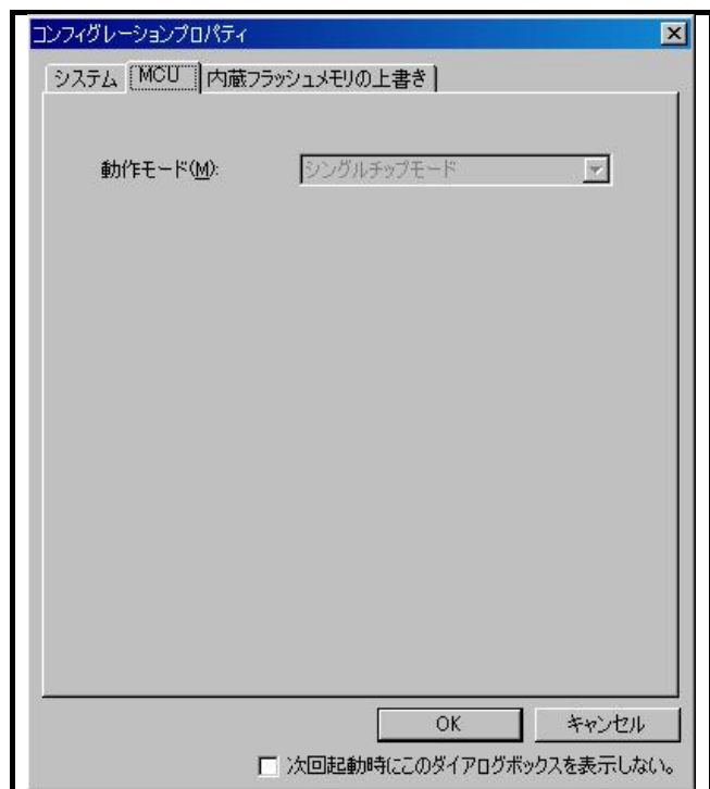
図 4.32 [コンフィグレーションプロパティ]ダイアログボックス (MCUタブ)
