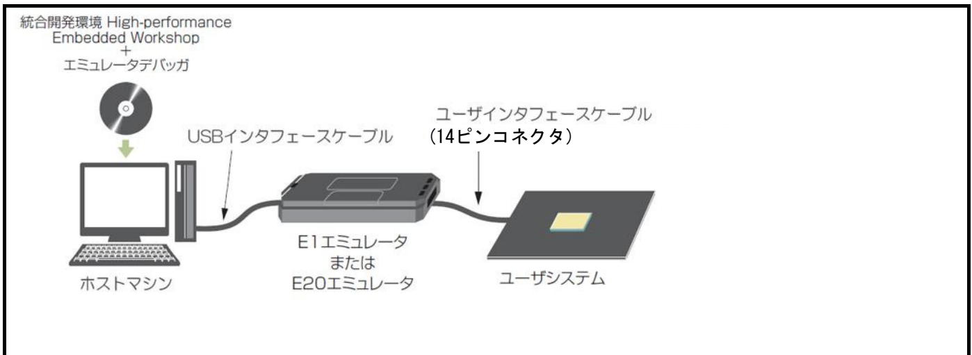
図 4.14 システムチェックの構成
