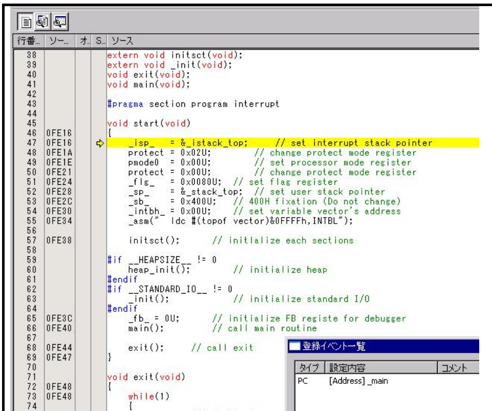
図 5.17 ドラッグ&amp;ドロップによるイベント追加
