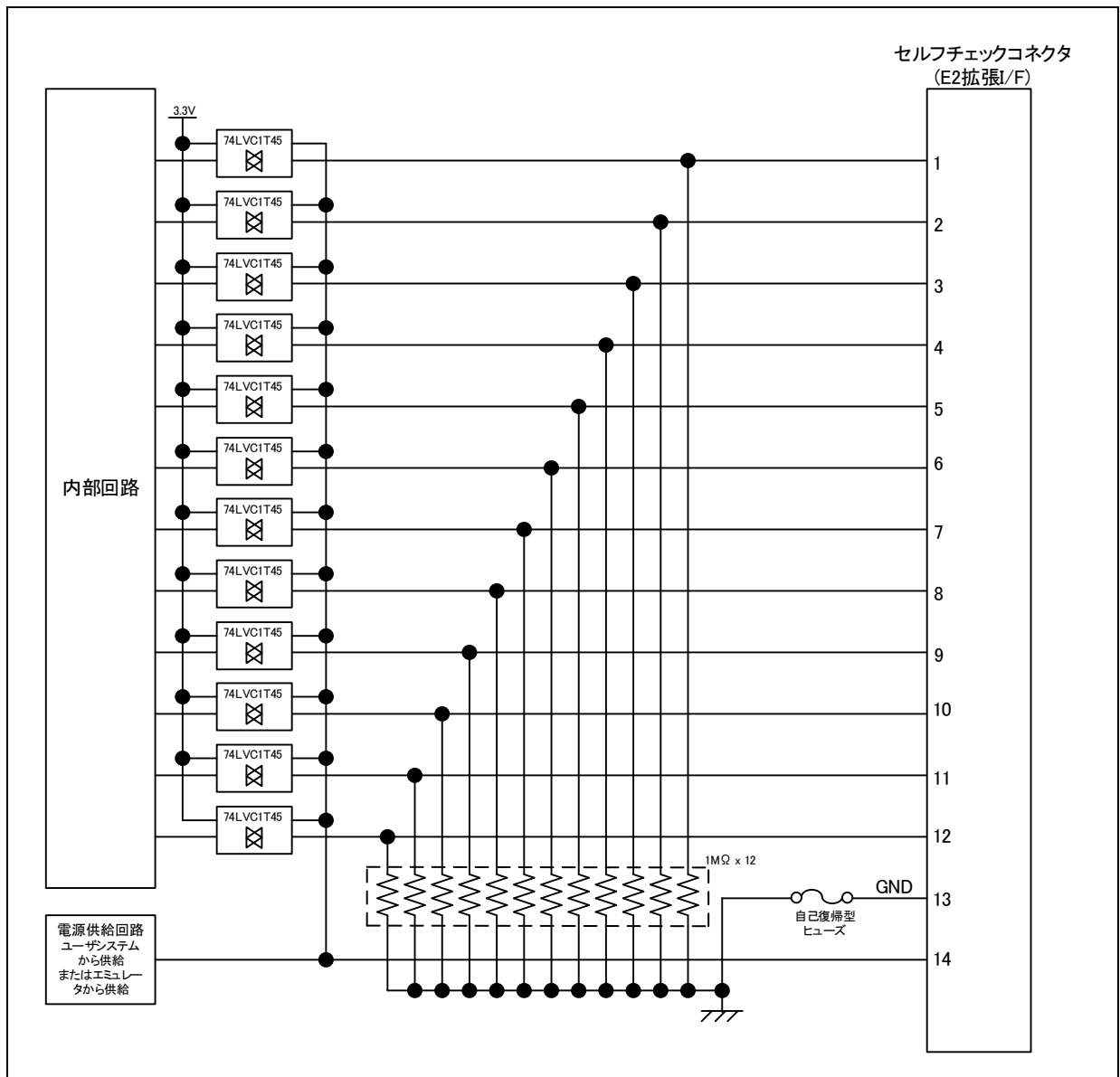
図B.2 E2拡張I/Fの内部回路
