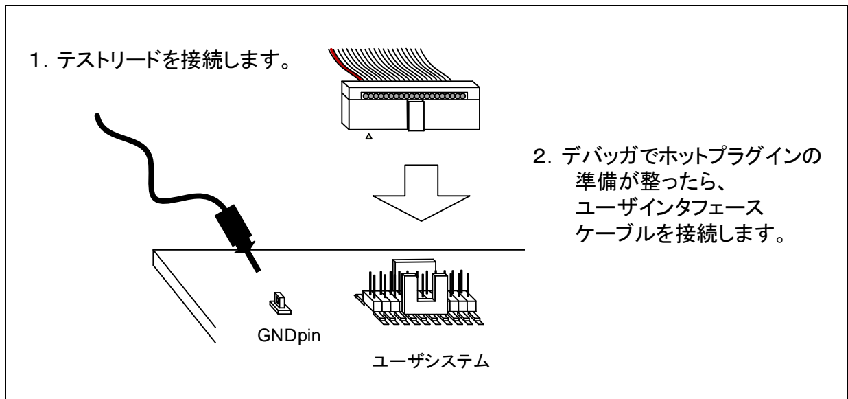
図2-7 ホットプラグイン接続方法(変換アダプタを使用しない場合)
