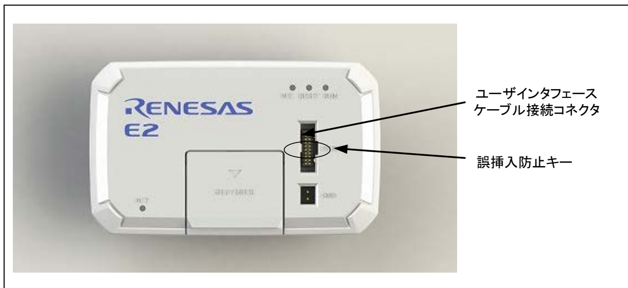
図2-2 E2のユーザインタフェースケーブル接続コネクタの配置
