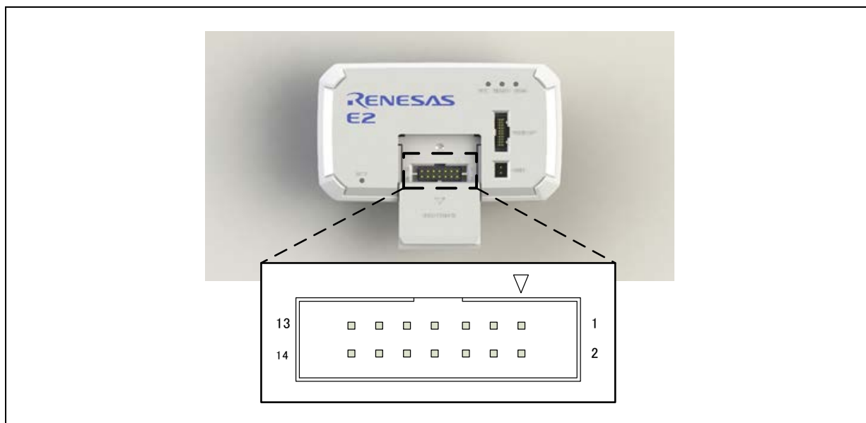
図B.1 セルフチェックコネクタ(E2拡張I/F)のピン配置
