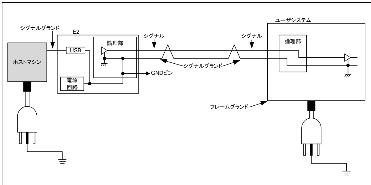
図2-8 システムグランド系の接続
