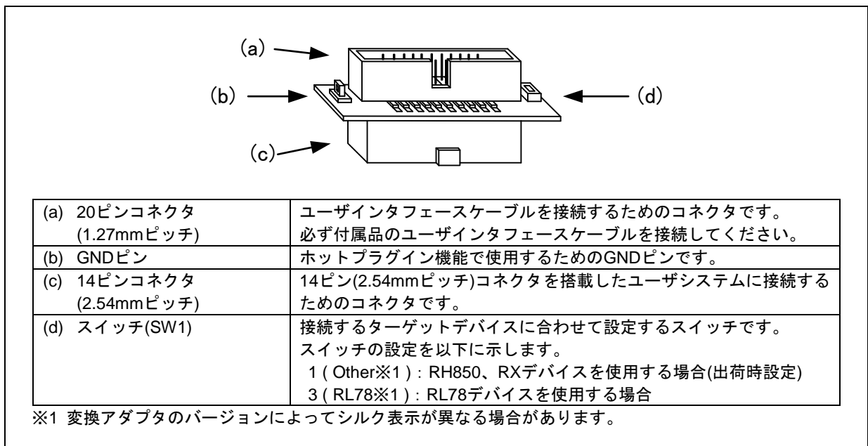
図 1-5 20ピン(1.27mmピッチ)/14ピン(2.54mmピッチ)コネクタ変換アダプタ
