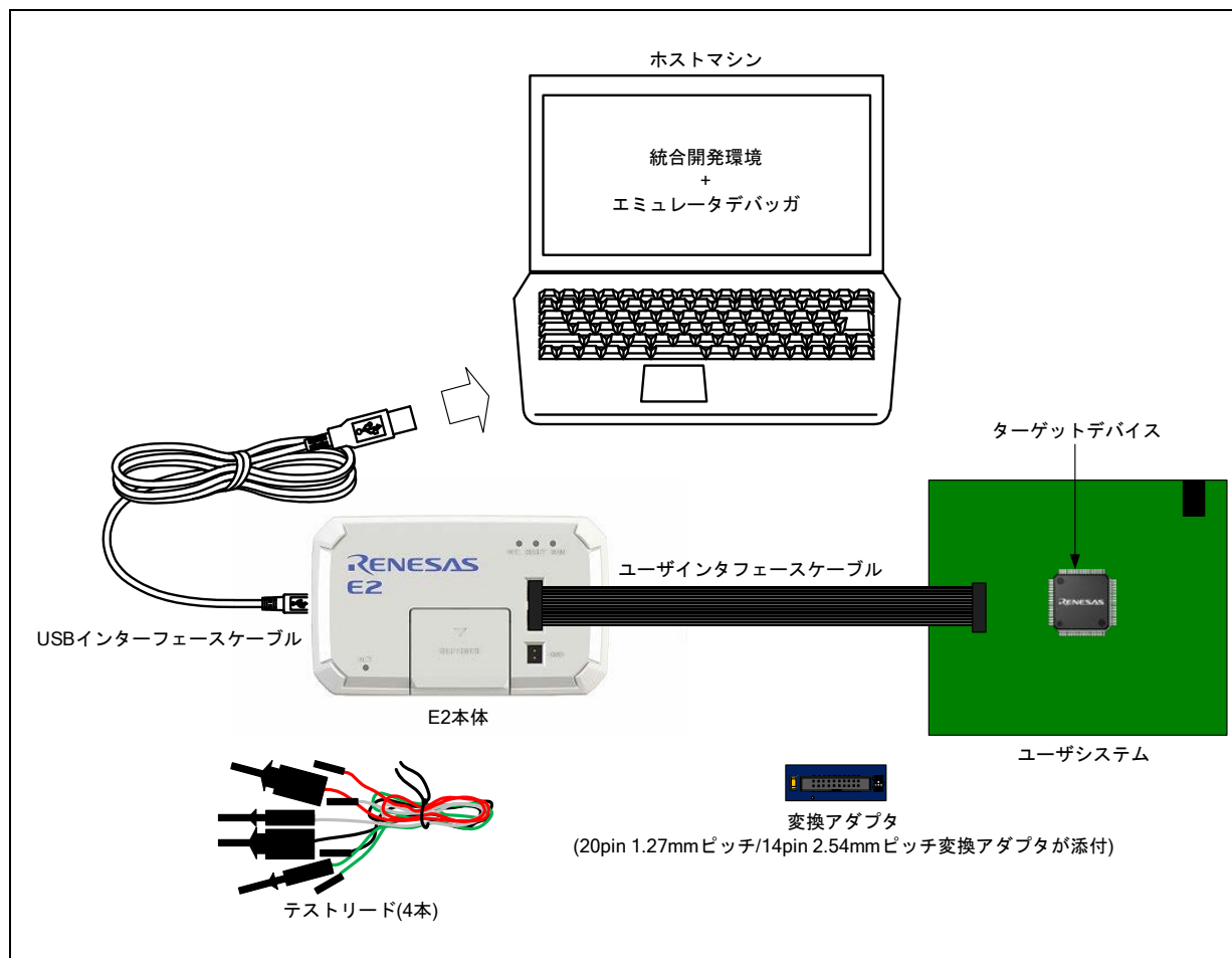
図 1-1 E2のシステム構成例
