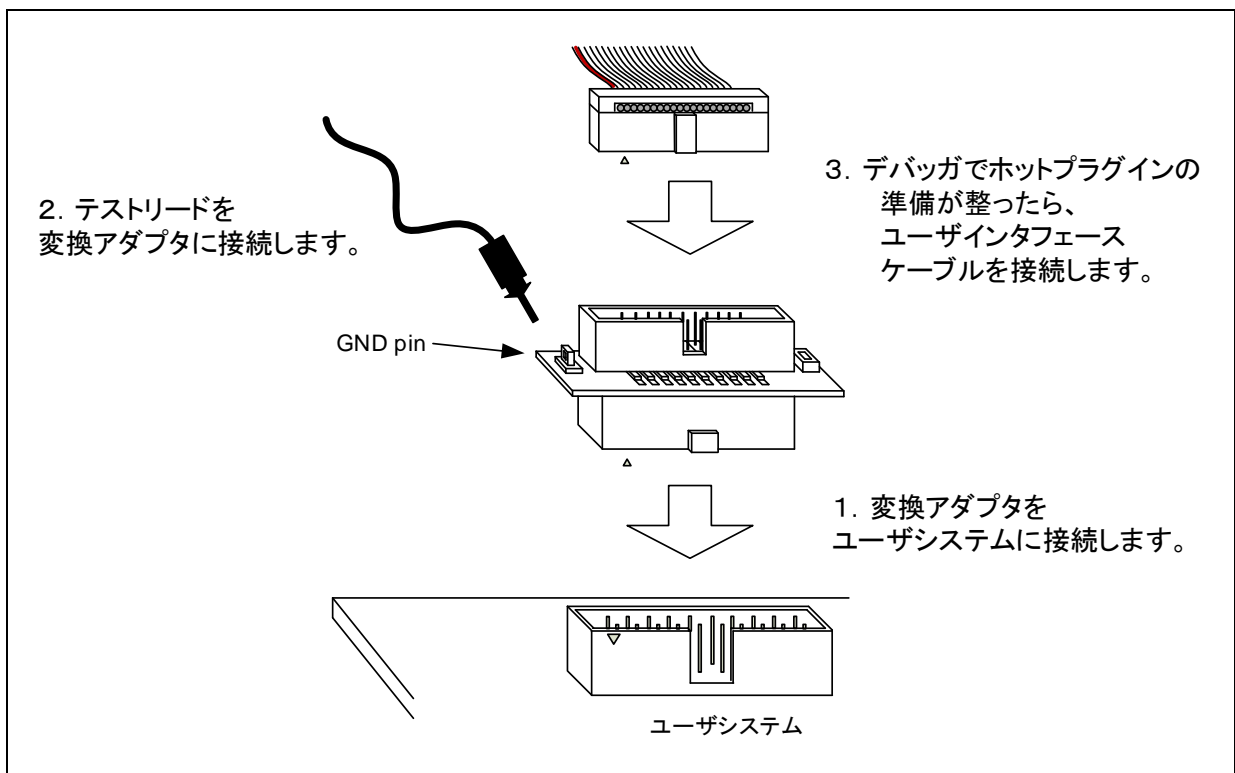
図2-6 ホットプラグイン接続方法
