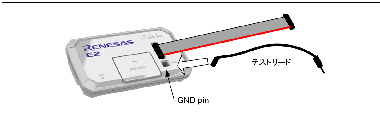
図2-5 E2のユーザインタフェースケーブルとテストリードの接続
