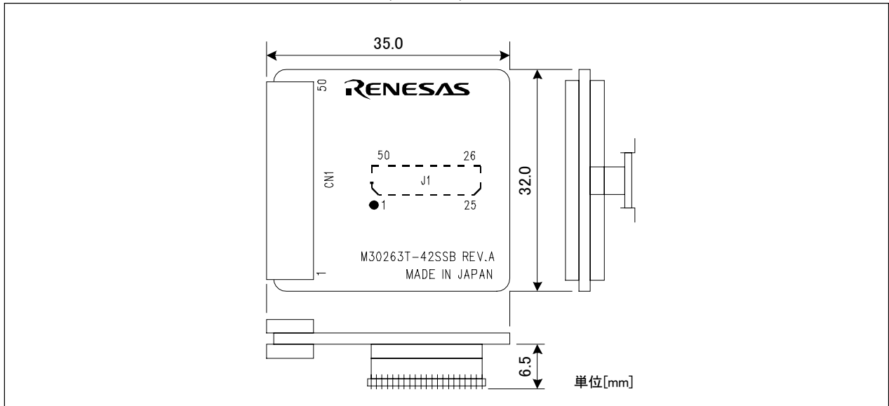
図3 M30263T-42SSBターゲット接続部の寸法
