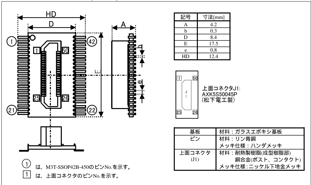
図4 M3T-SSOP42B-450の寸法
