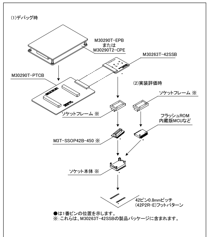
図2 M30263T-42SSBの使用方法
