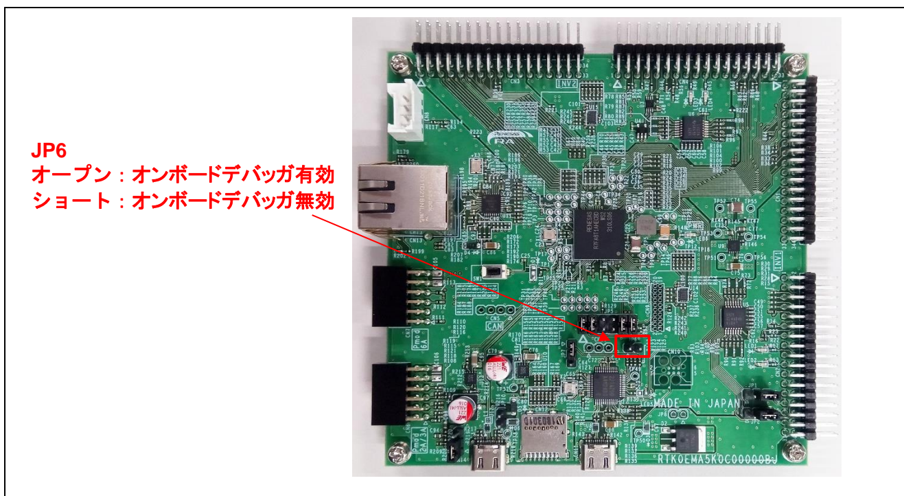
図 5-1 ジャンパーJP6 の設定
