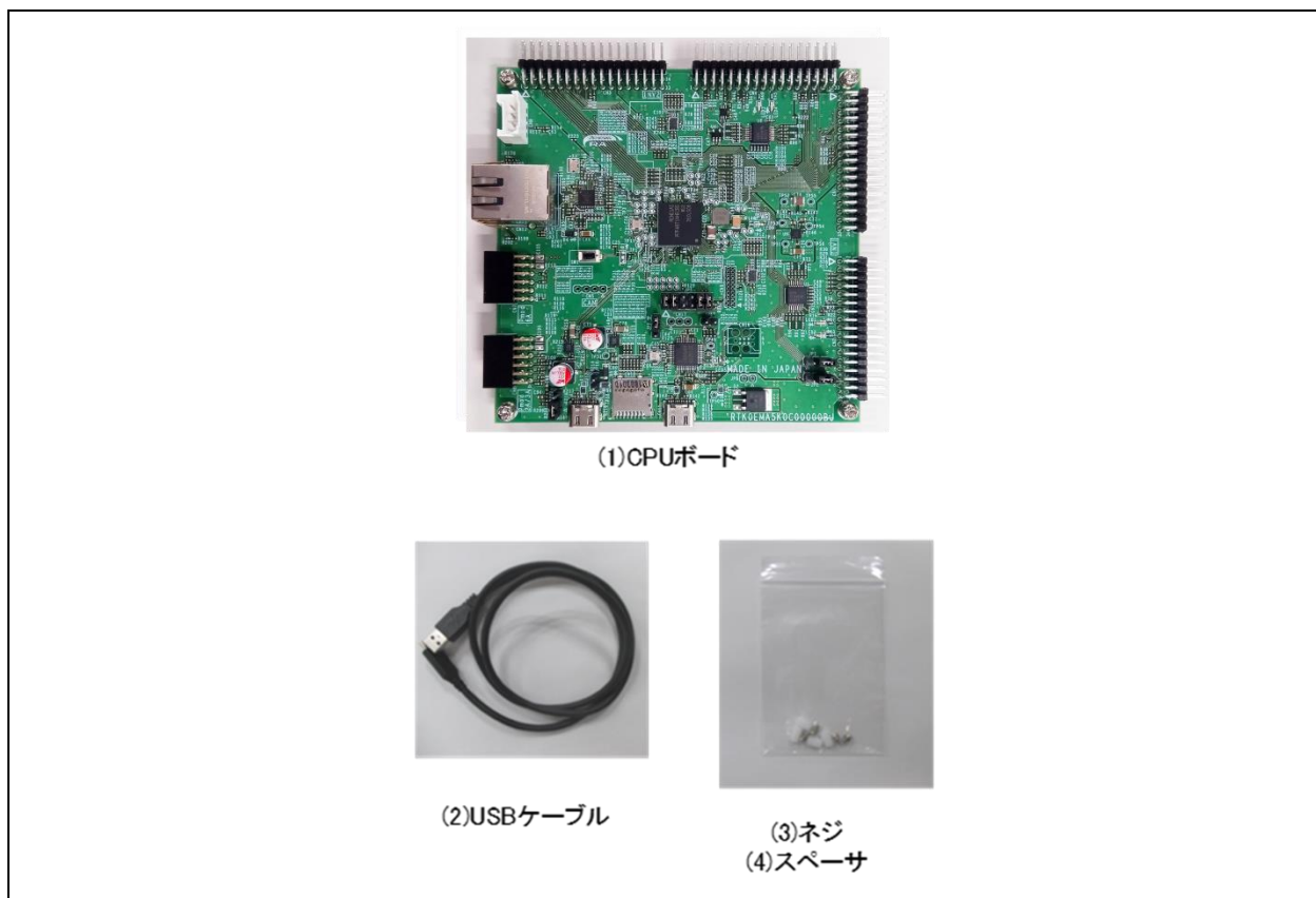
図 2-1 製品構成
