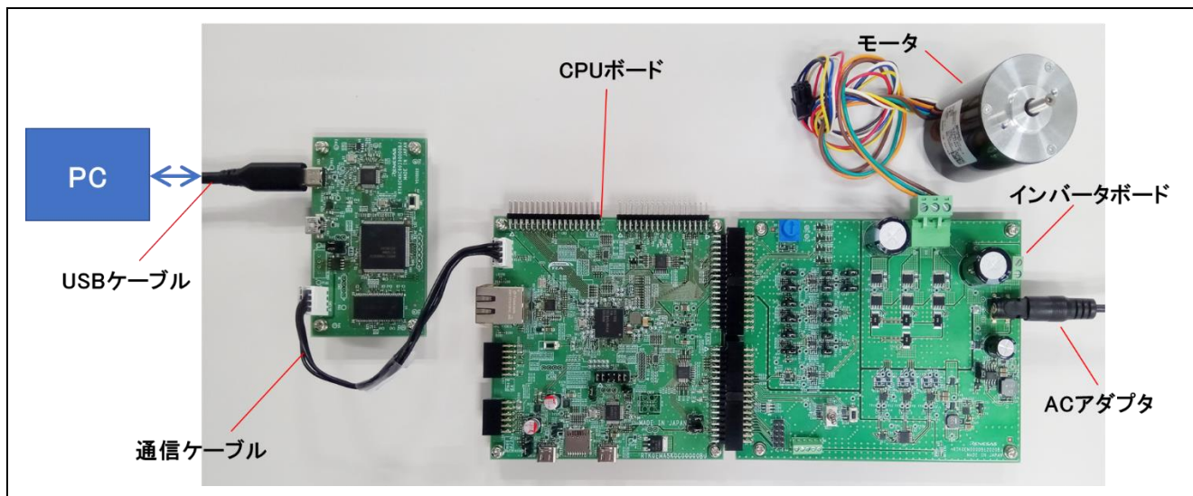
図 4-5 ボード接続例
