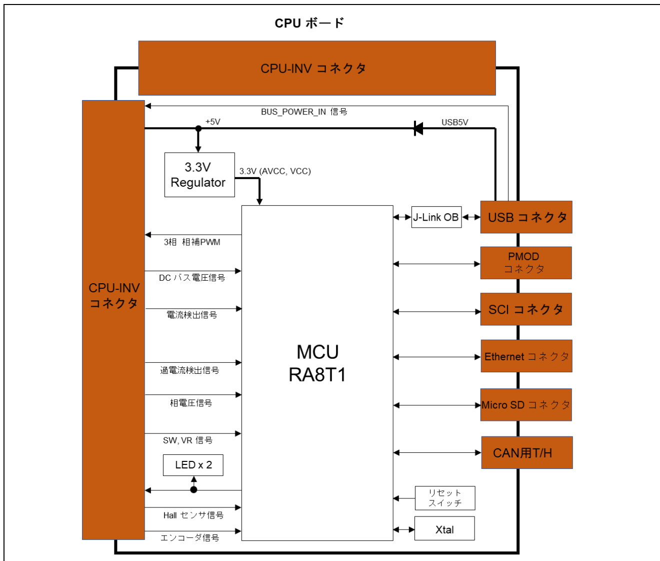
図 4-1 CPU ボードのブロック図
