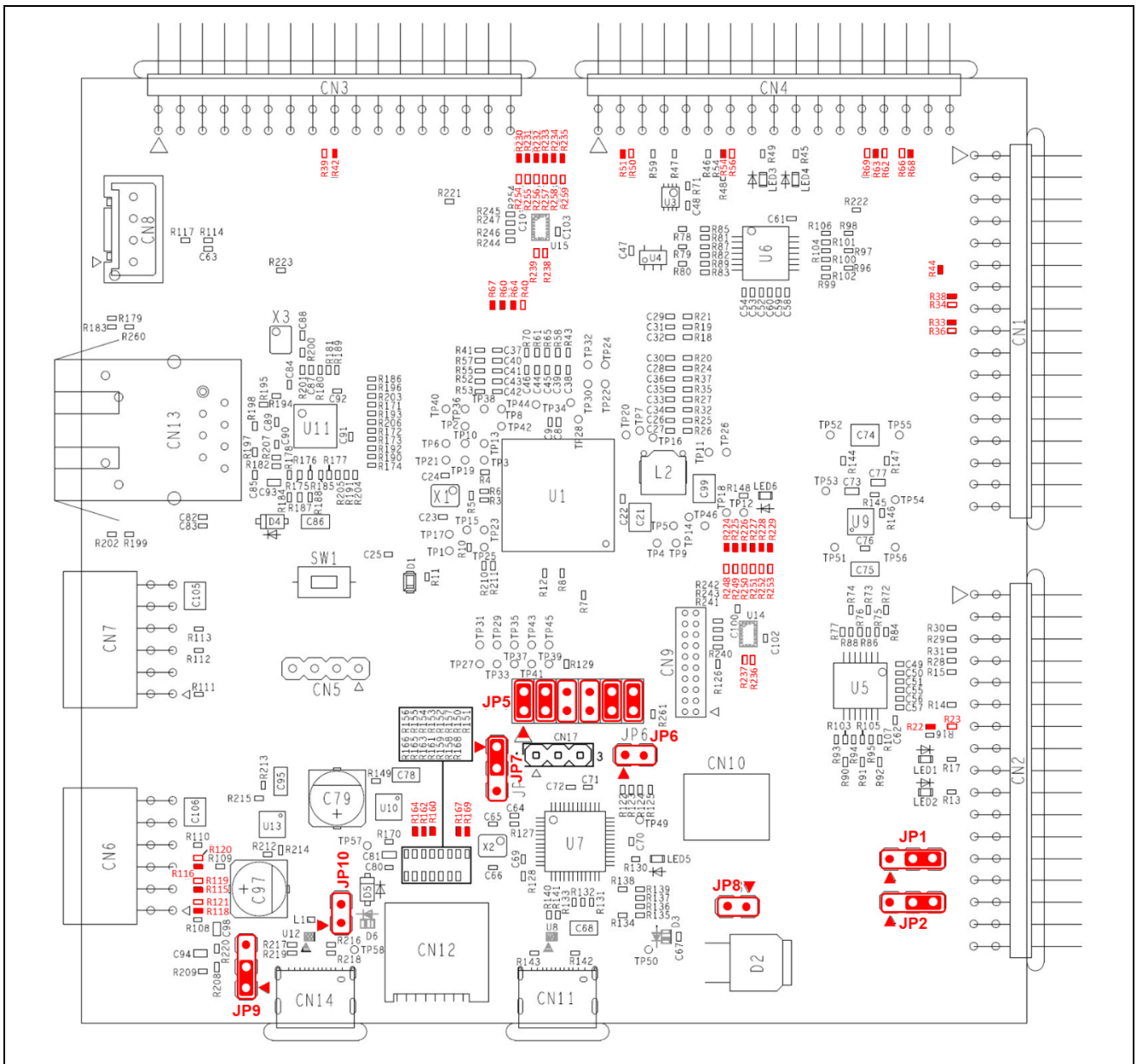
図 4-4 ジャンパーピン、ジャンパー抵抗の初期設定
