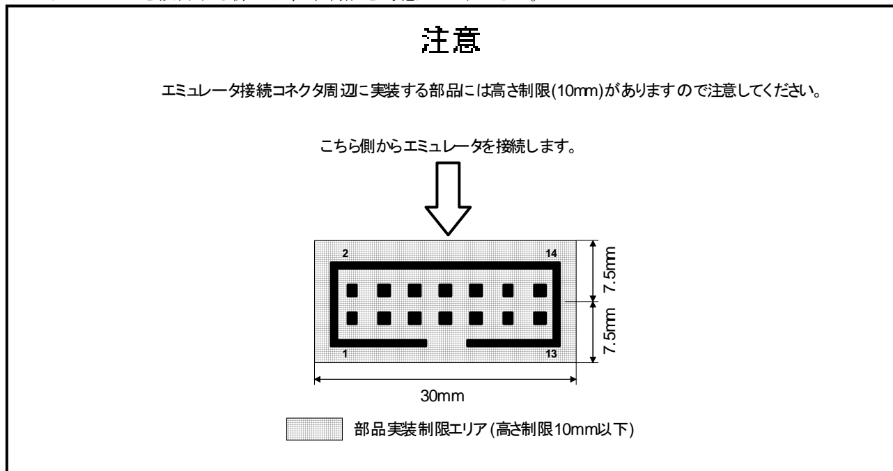
図 3 ユーザシステム上の本アダプタ接続コネクタ周辺に対する部品実装制限
