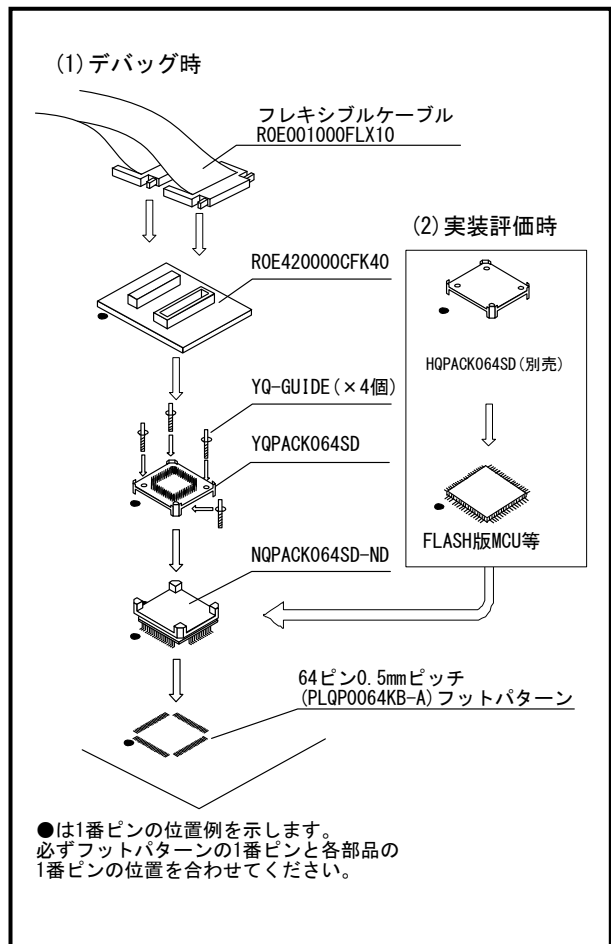
図2 ROE420000CFK40の用途
