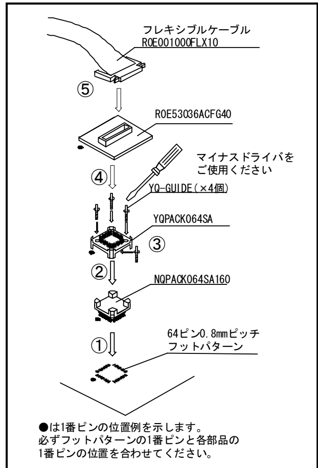
図3 ROE53036ACFG40装着手順
