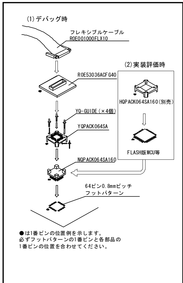
図2 ROE53036ACFG40の用途
