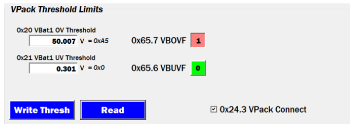
Figure 48. VBOVF
