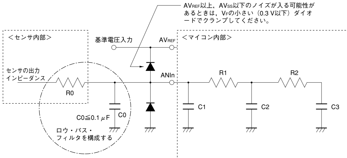
図11-20 信号源インピーダンスが高い場合の回路例
