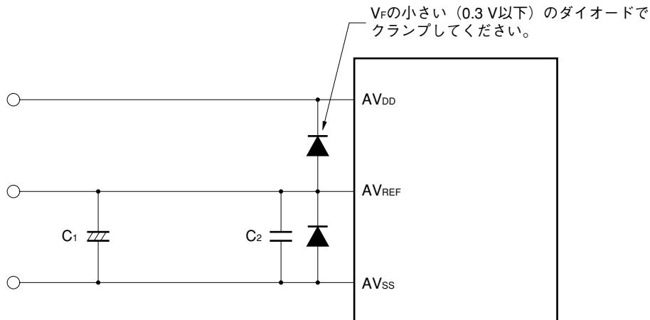
図11-18 AVREF端子とコンデンサの接続例
