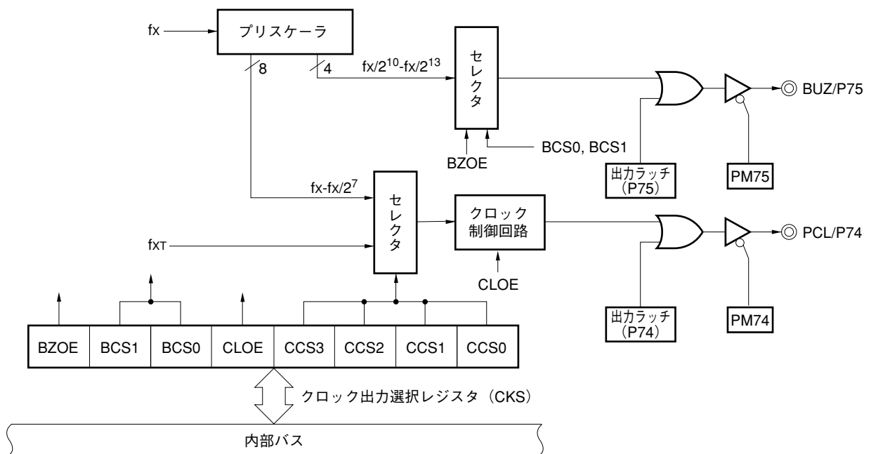
図10-1 クロック出力／ブザー出力制御回路のブロック図
