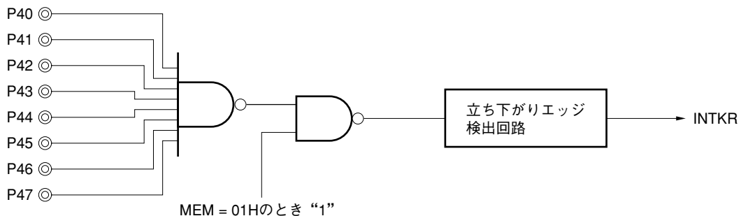
図4-11 立ち下がりエッジ検出回路のブロック図
