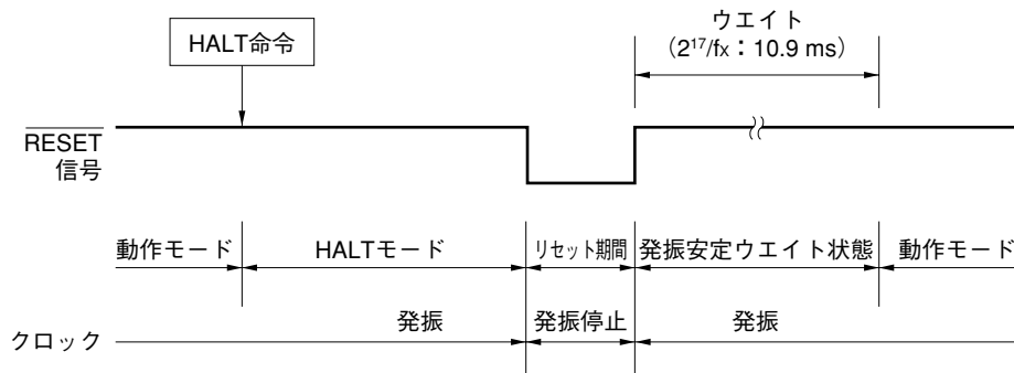
図16-3 HALTモードの RESET 入力による解除
