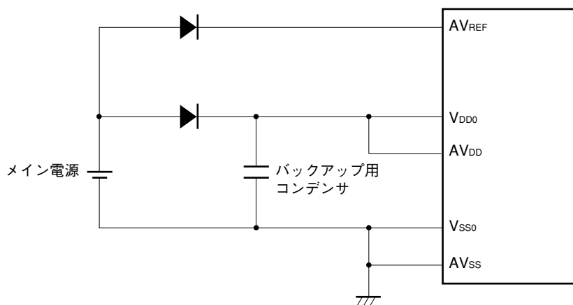
図11-17 AVDD端子の処理
