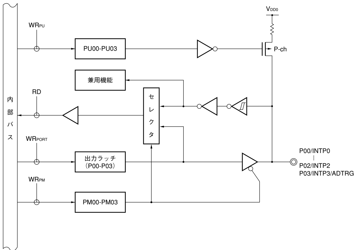
図4-2 P00-P03のブロック図
