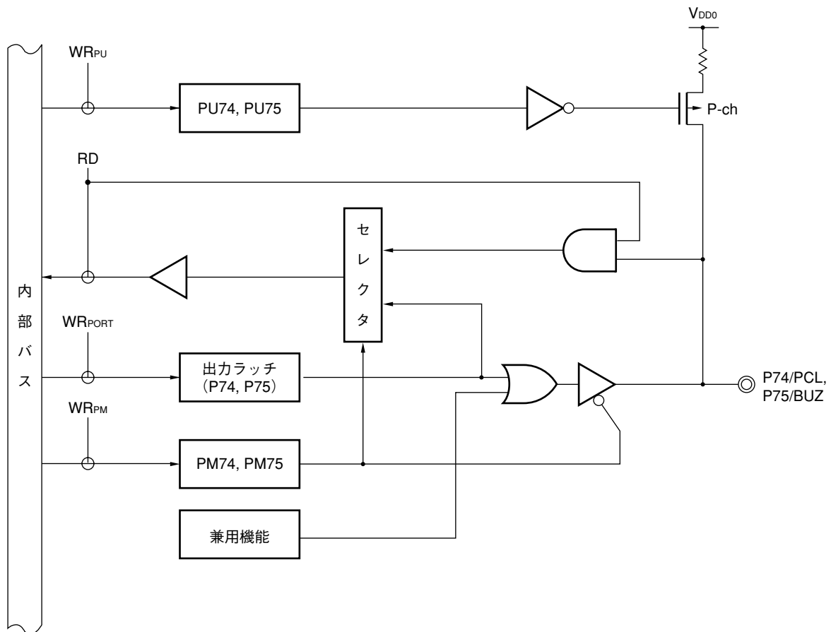
図4-15 P74, P75のブロック図
