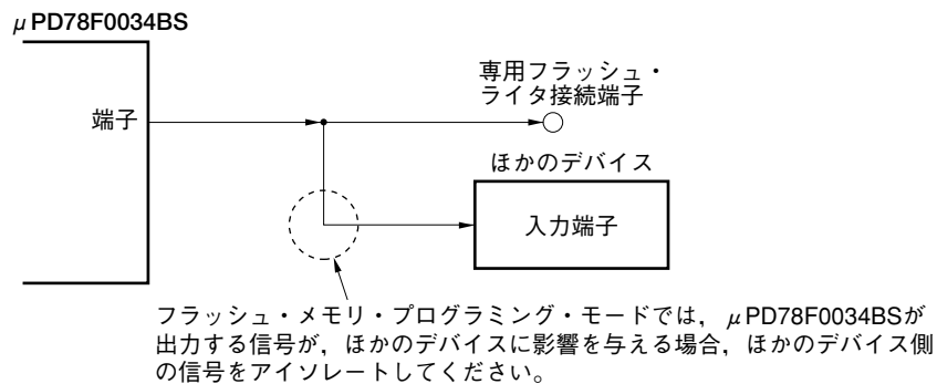
図18-7 ほかのデバイスの異常動作
