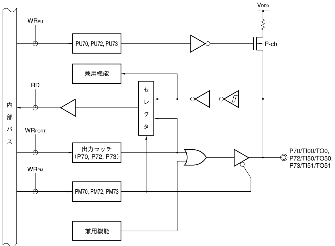
図4-13 P70, P72, P73のブロック図
