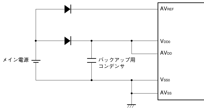
図12-18 AVDD端子の処理
