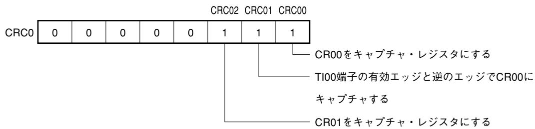
(b) キャプチャ/コンペア・コントロール・レジスタ0 (CRC0)
