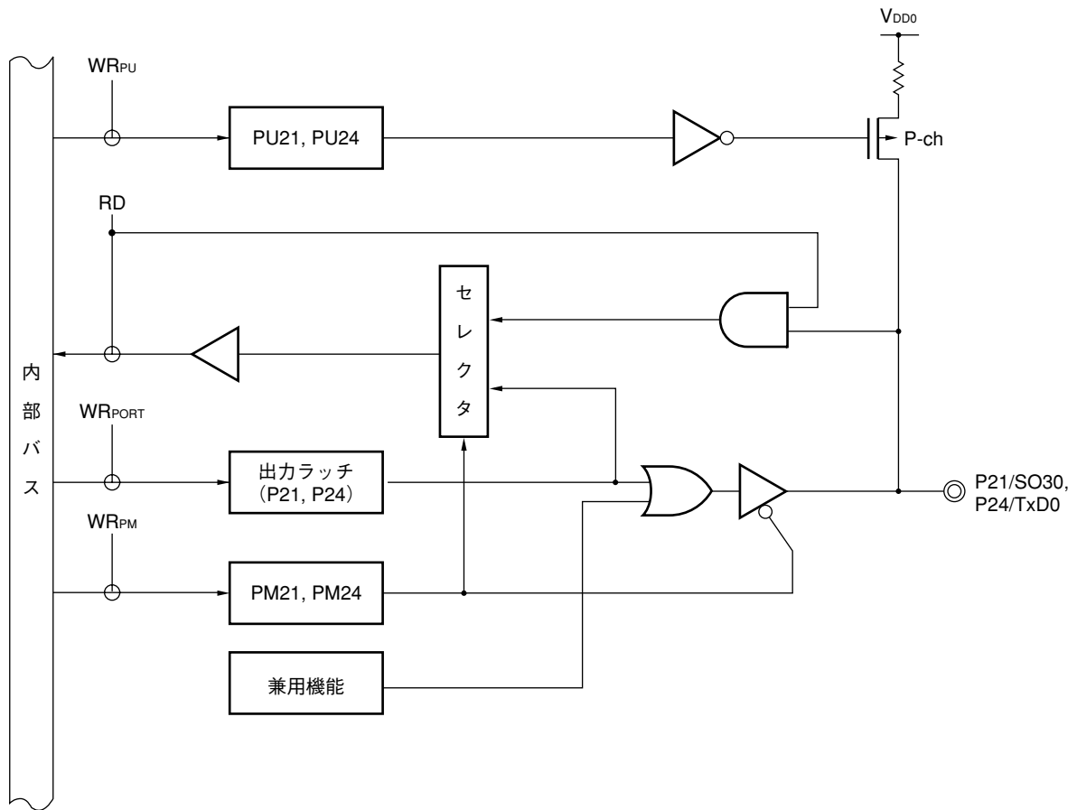
図4-5 P21, P24のブロック図
