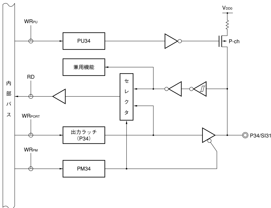
図4-7 P34のブロック図
