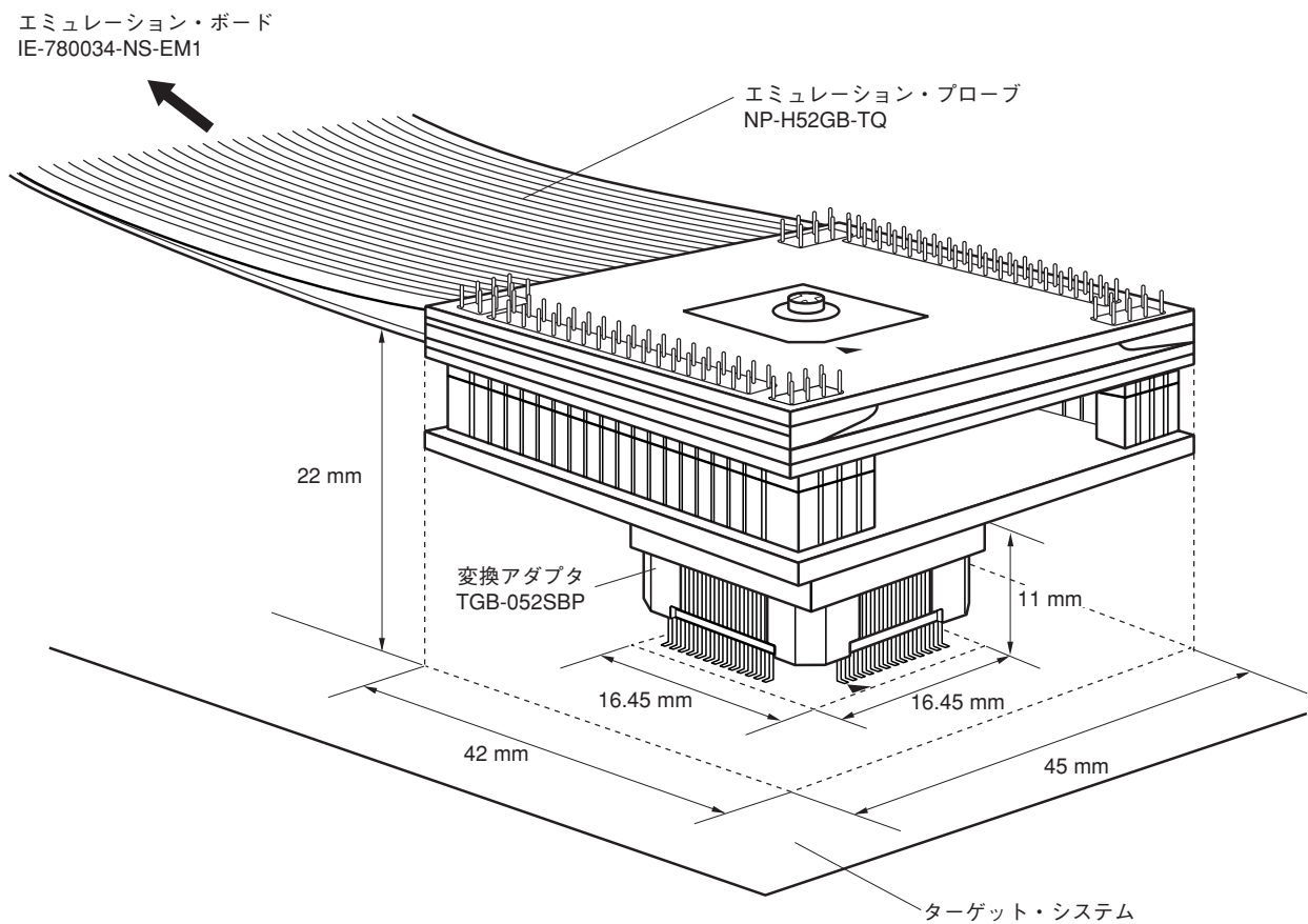
図C-2 ターゲット・システムの接続条件 (NP-H52GB-TQの場合)
