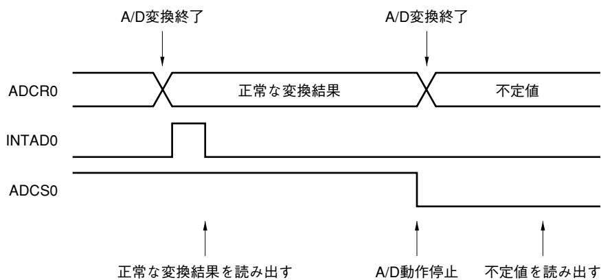
図12-17 変換結果を読み出すタイミング (変換結果が不定値の場合)
