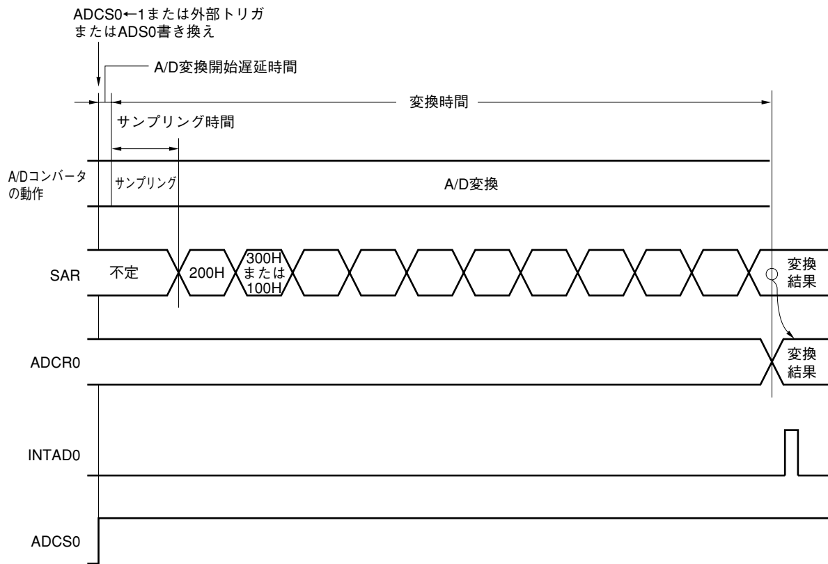
図12-5 10ビットA/Dコンバータの基本動作
