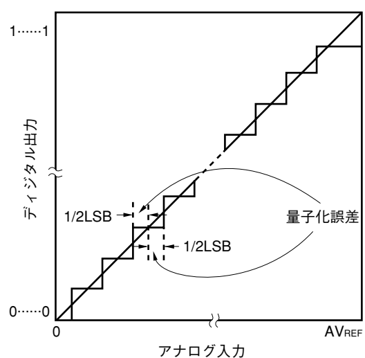
図12-10 量子化誤差
