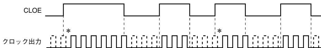
図10-4 リモコン出力応用例
