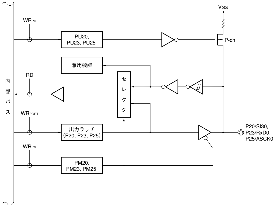
図4-4 P20, P23, P25のブロック図
