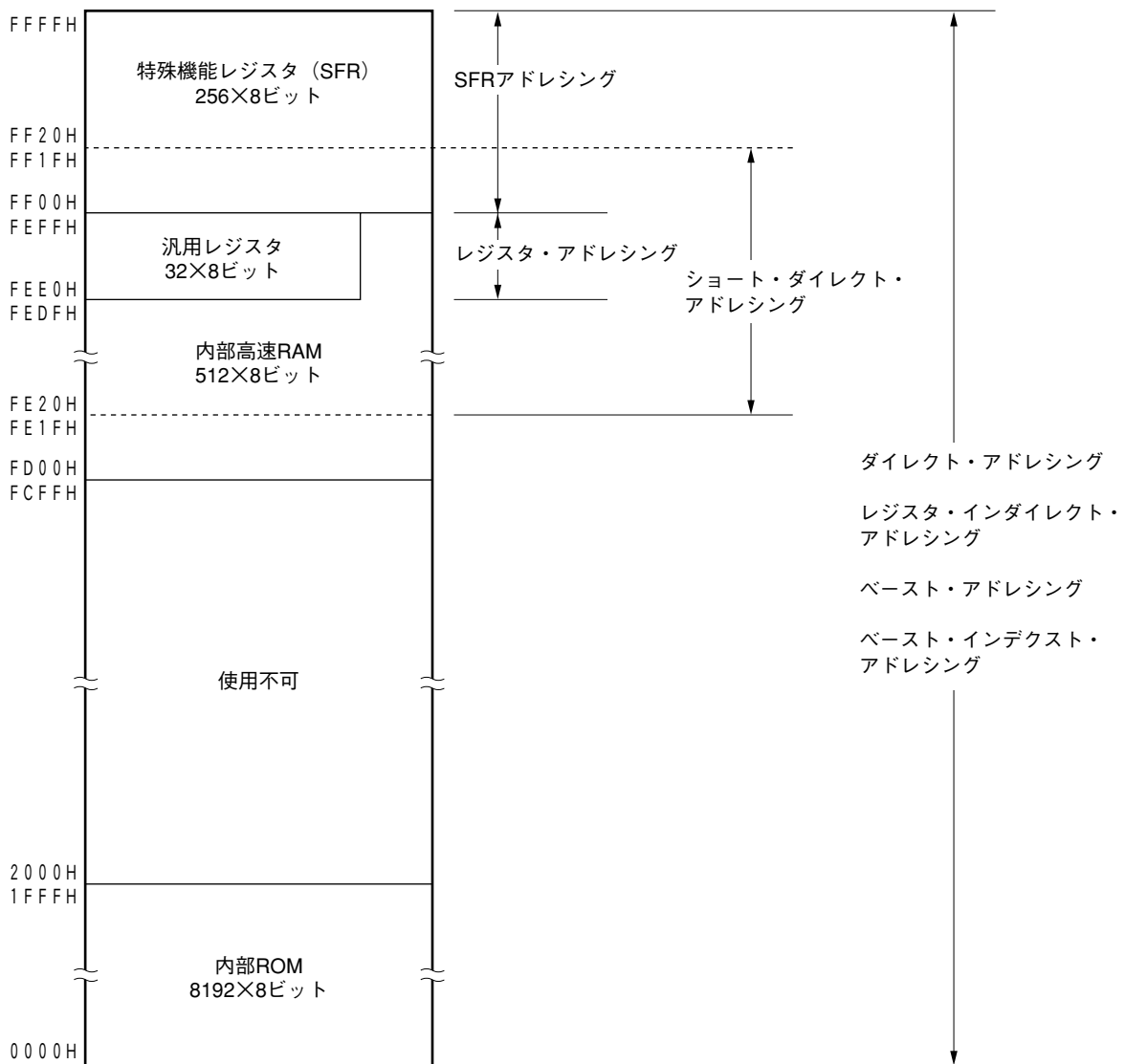
図3-6 データ・メモリとアドレッシングの対応 ( \mu PD780021AS, 780031AS)
