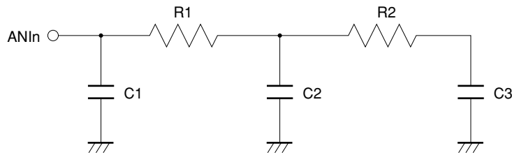
図11-19 ANI0-ANI3端子内部等価回路
