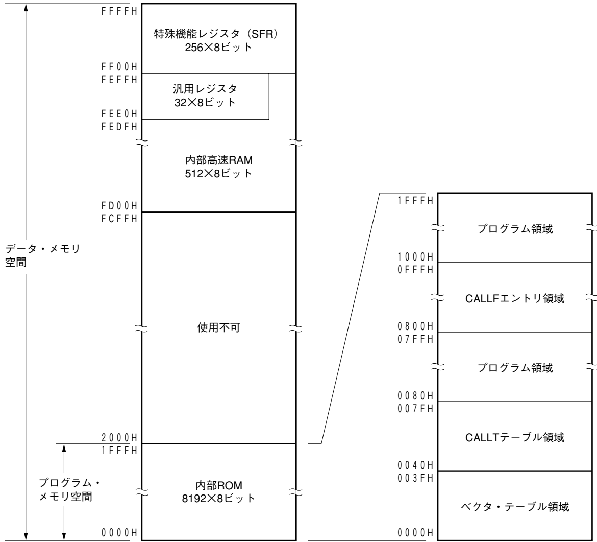
図3-1 メモリ・マップ (μPD780021AS, 780031AS)
