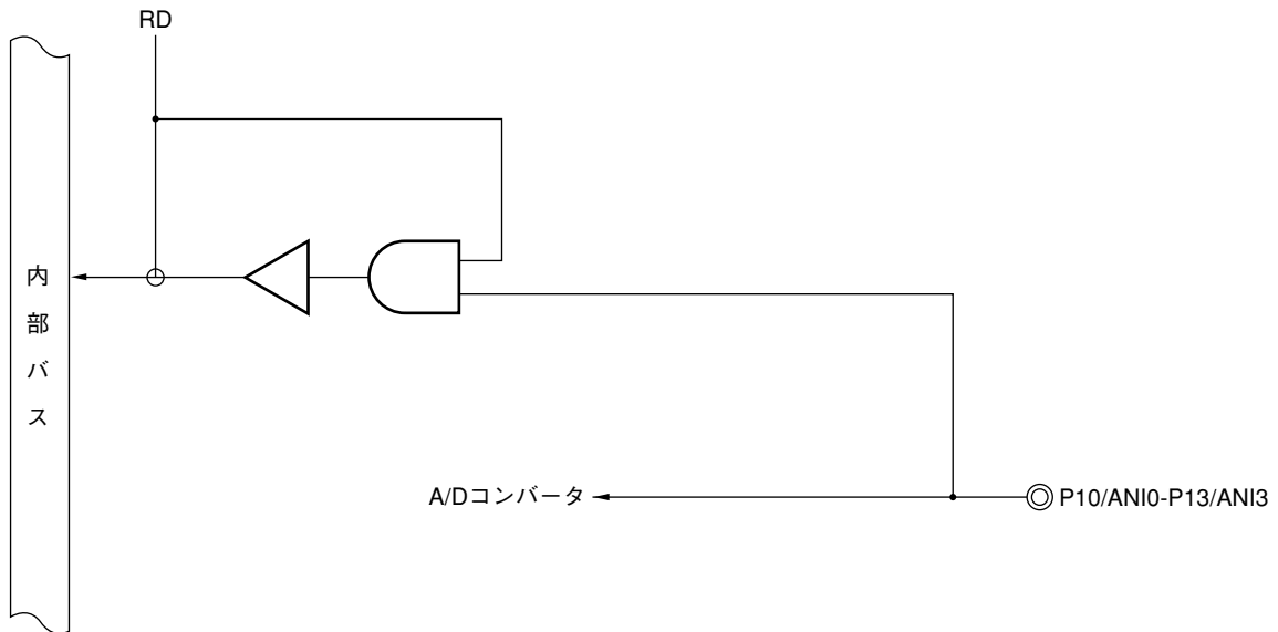
図4-3 P10-P13のブロック図
