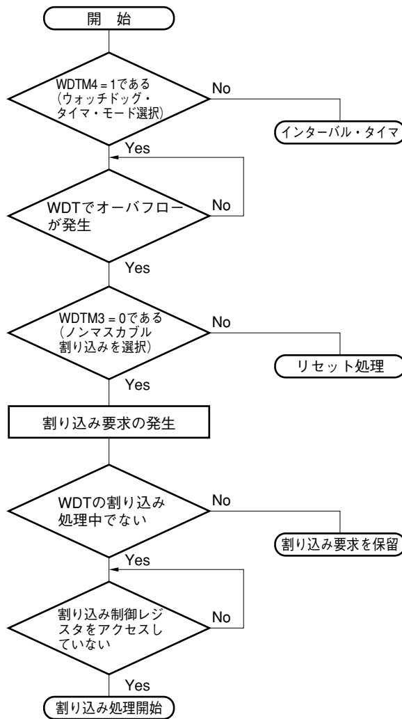
図15-8 ノンマスカブル割り込み要求発生から受け付けまでのフロー・チャート
