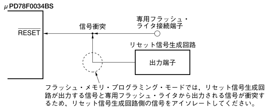
図18-8 信号の衝突 (RESET端子)
