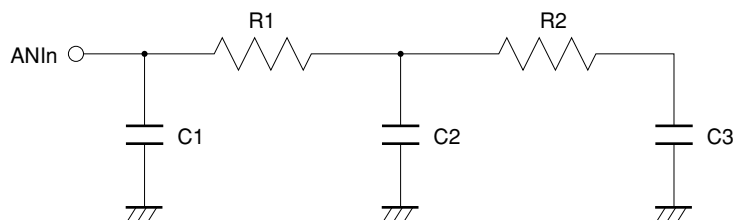
図12-20 ANI0-ANI3端子内部等価回路
