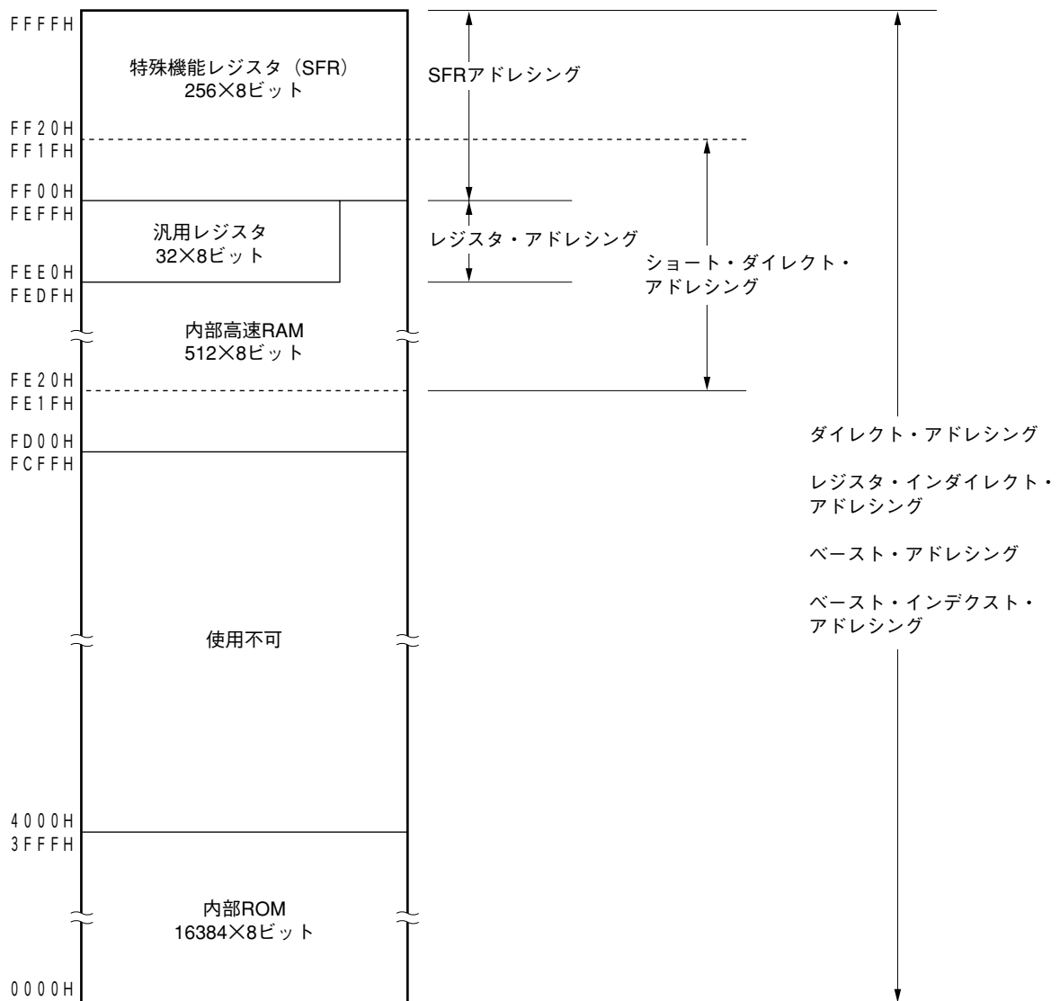
図3-7 データ・メモリとアドレッシングの対応 (μPD780022AS, 780032AS)
