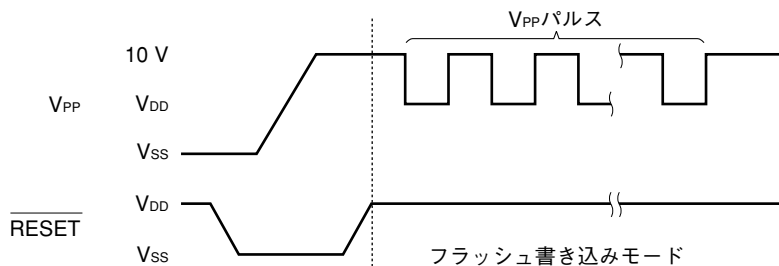
図18-3 通信方式選択フォーマット
