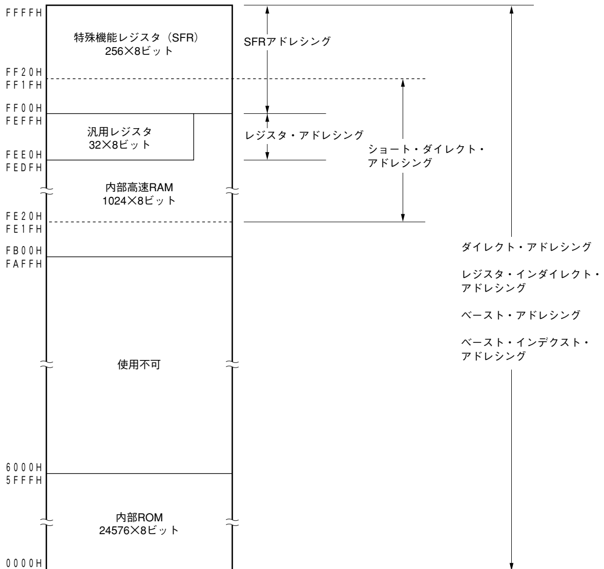
図3-8 データ・メモリとアドレッシングの対応 (μPD780023AS, 780033AS)
