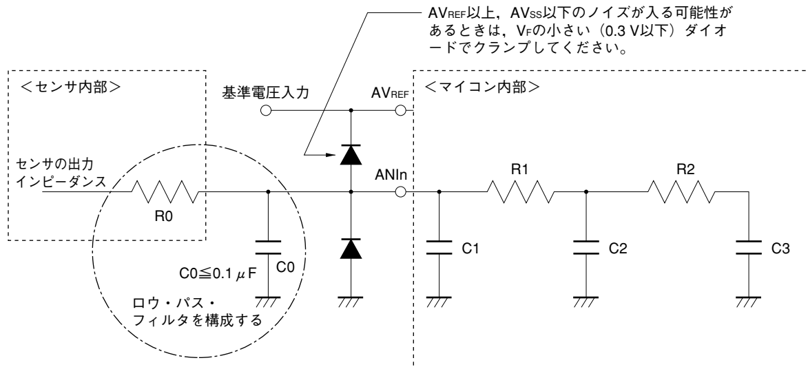
図12-21 信号源インピーダンスが高い場合の回路例
