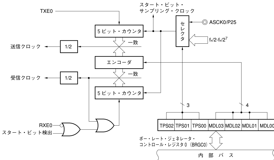
図13-2 ボー・レート・ジェネレータのブロック図
