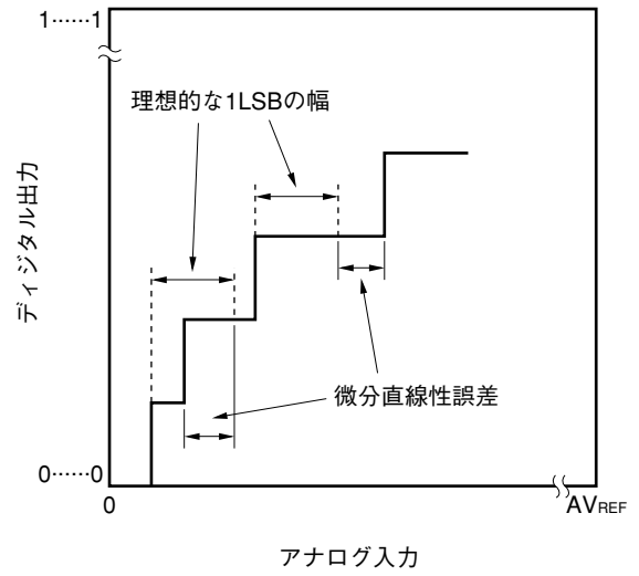
図11-13 微分直線性誤差
