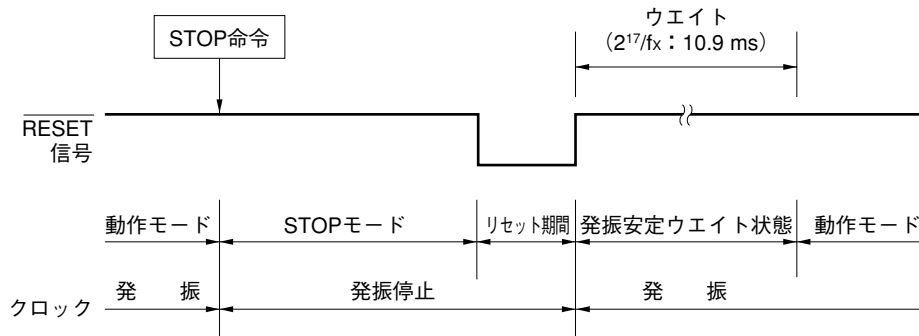
図16-5 STOPモードの \overline{\text{RESET}} 入力による解除
