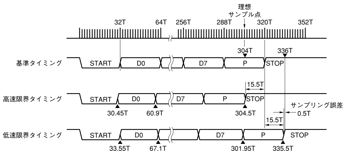
図13-7 サンプルング誤差を考慮したボー・レートの許容誤差 (k = 0の場合)
