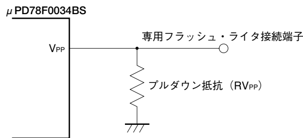
図18-5 V PP 端子の接続例
