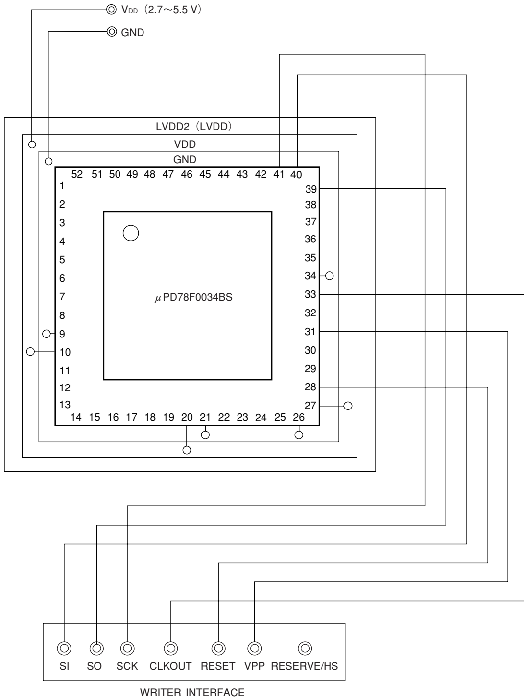
図18-12 疑似3線式シリアルI/O方式でのフラッシュ書き込み用アダプタ配線例
