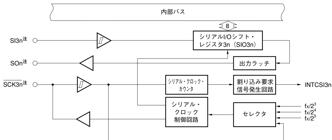
図14-1 シリアル・インタフェースSIO3nのブロック図
