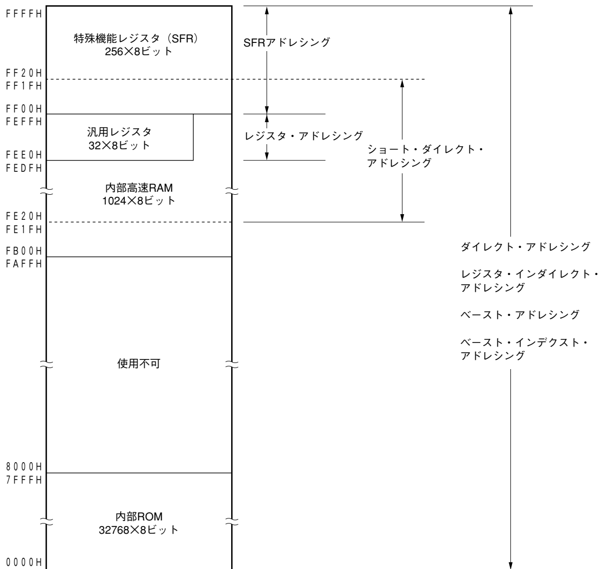
図3-9 データ・メモリとアドレッシングの対応 (μPD780024AS, 780034AS)
