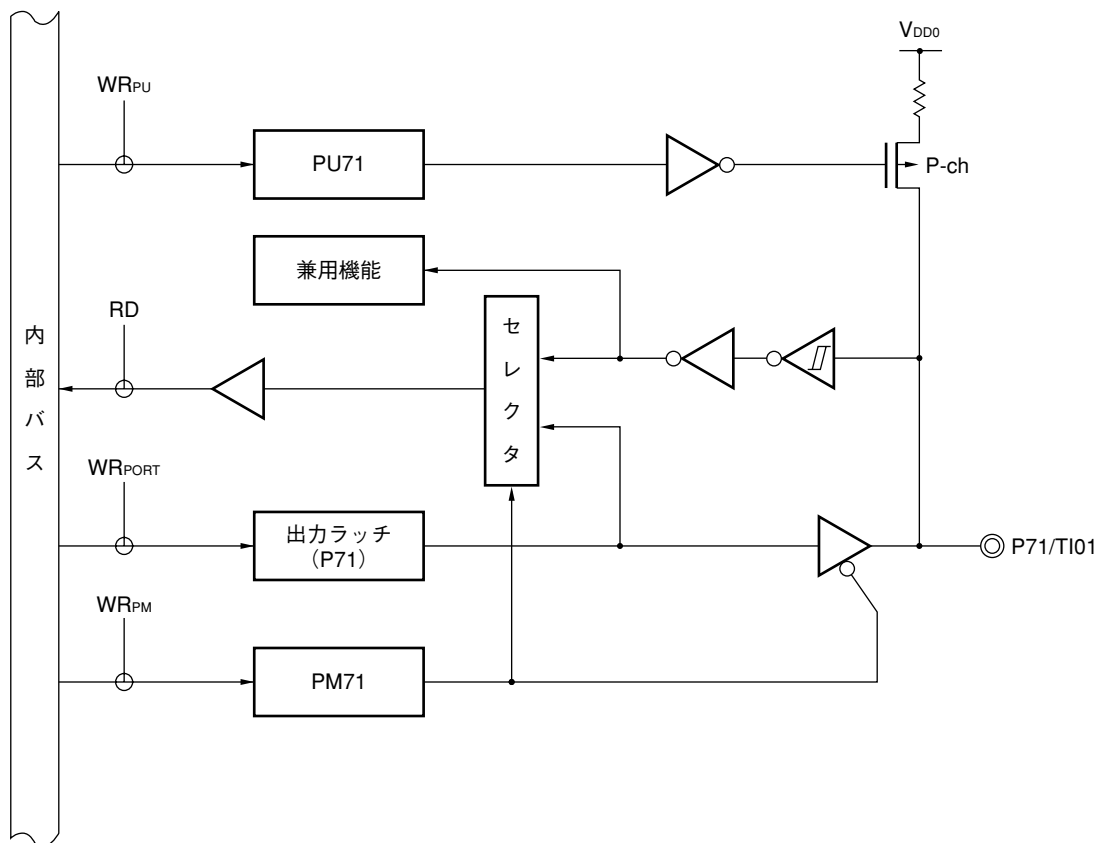
図4-14 P71のブロック図
