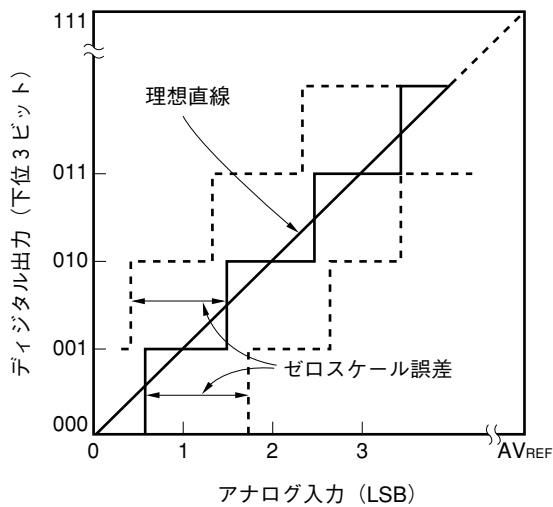
図12-11 ゼロスケール誤差
