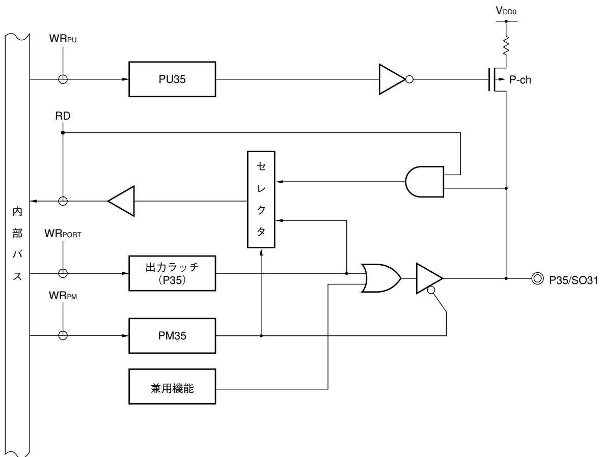
図4-8 P35のブロック図
