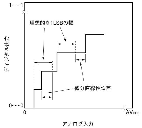
図12-14 微分直線性誤差
