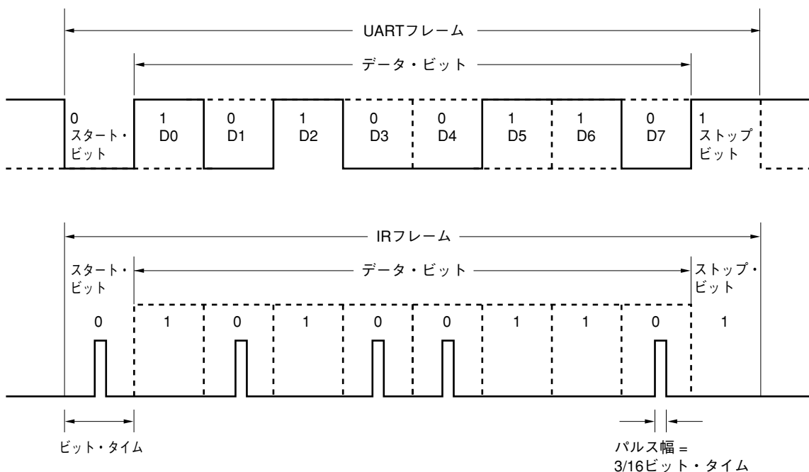
図13-12 赤外線データ転送モードとUARTモードのデータ・フォーマットの比較
