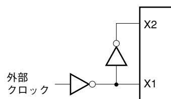
(b) 外部クロック
