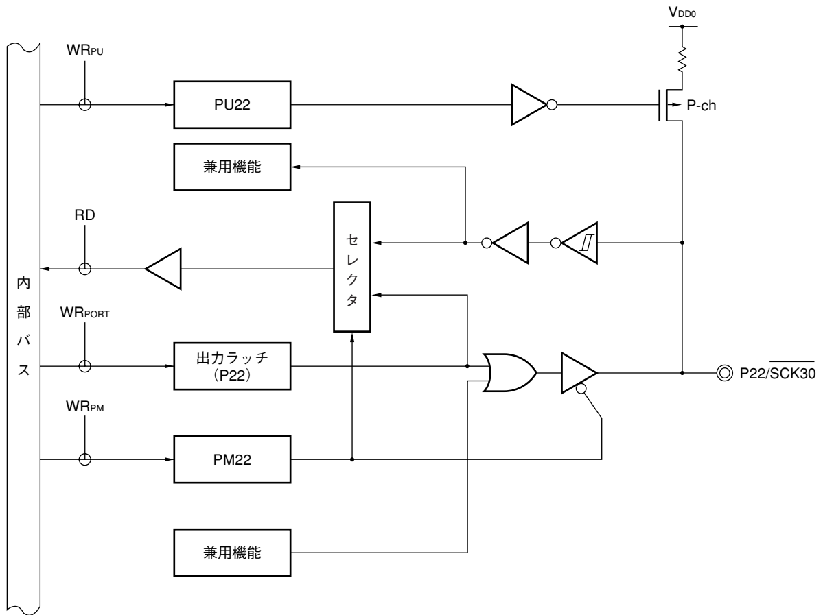
図4-6 P22のブロック図
