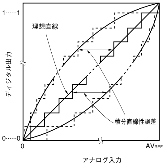
図11-12 積分直線性誤差
