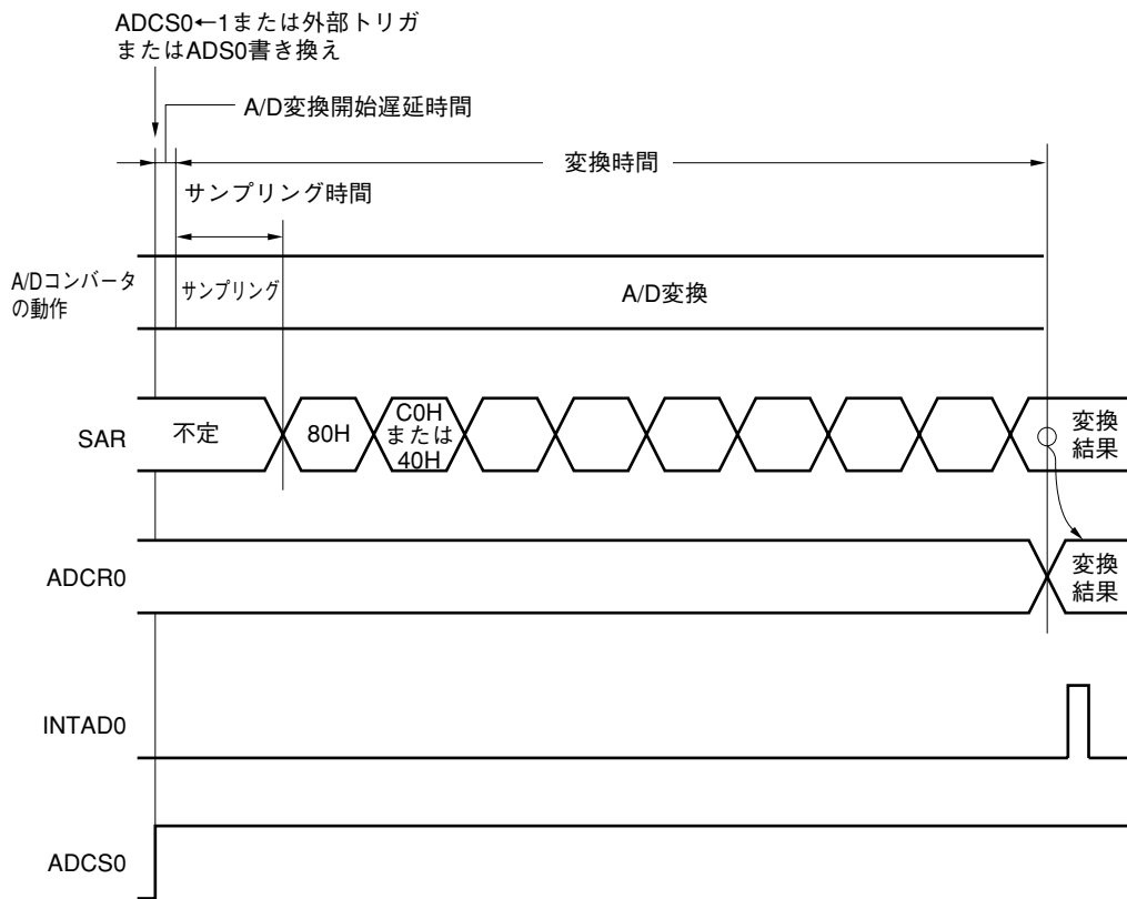
図11-4 8ビットA/Dコンバータの基本動作
