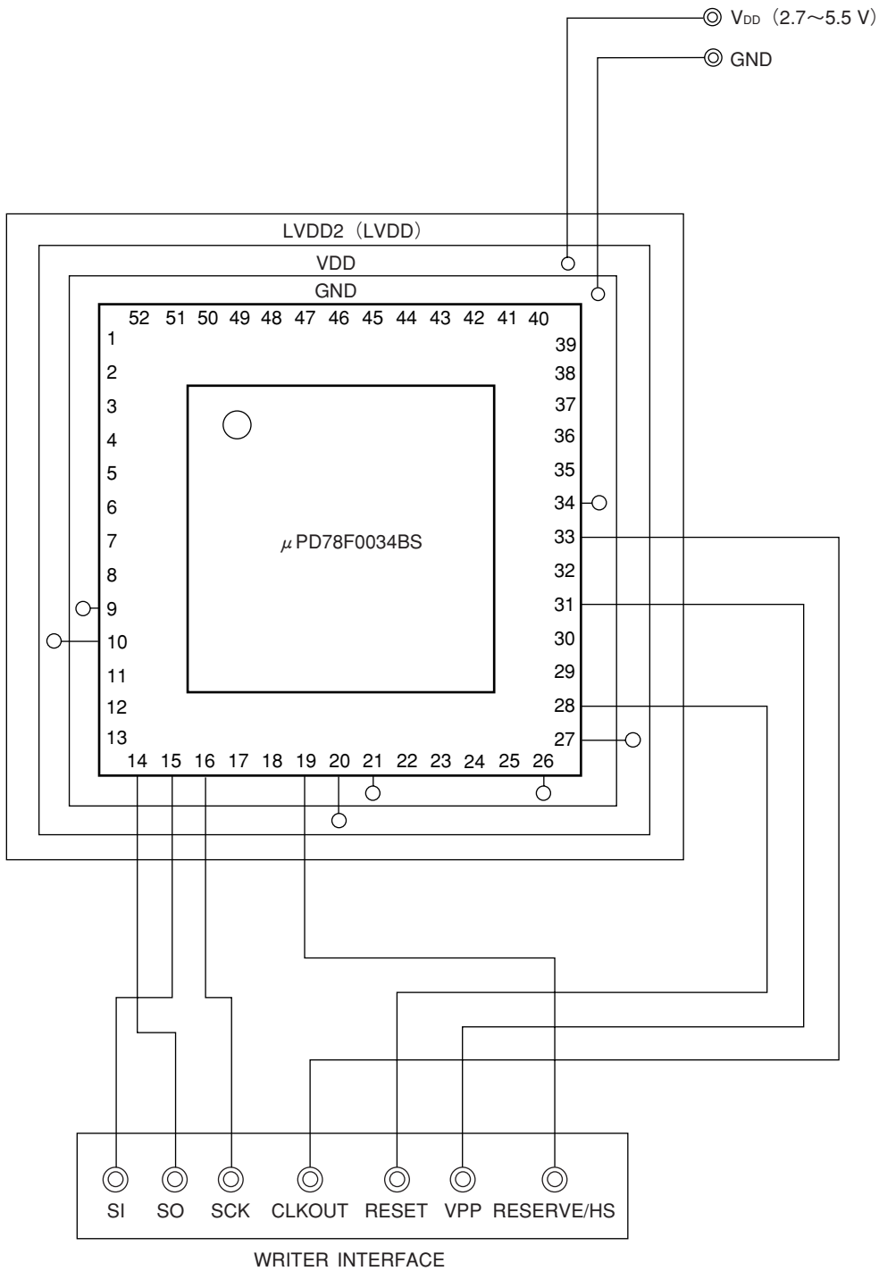
図18-10 3線式シリアルI/O方式でのフラッシュ書き込み用アダプタ配線例（ハンドシェイク使用時）
