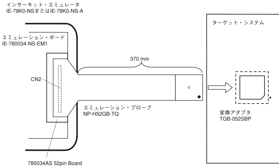
図C-2 ターゲット・システムの接続条件 (NP-H52GB-TQの場合)
