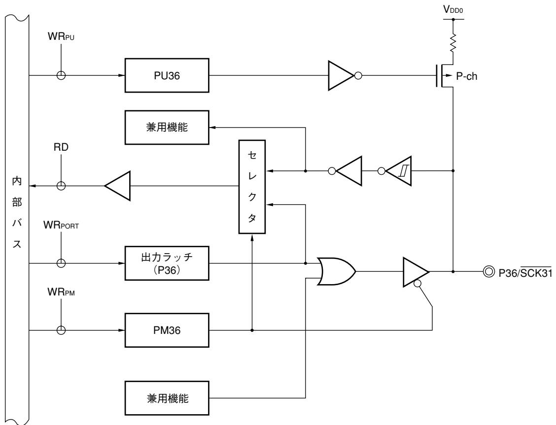
図4-9 P36のブロック図
