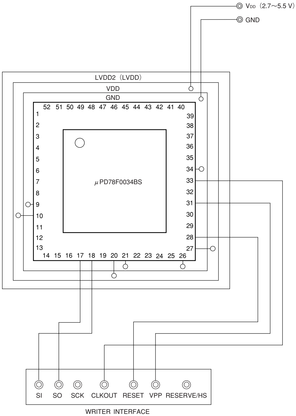
図18-11 UART方式でのフラッシュ書き込み用アダプタ配線例
