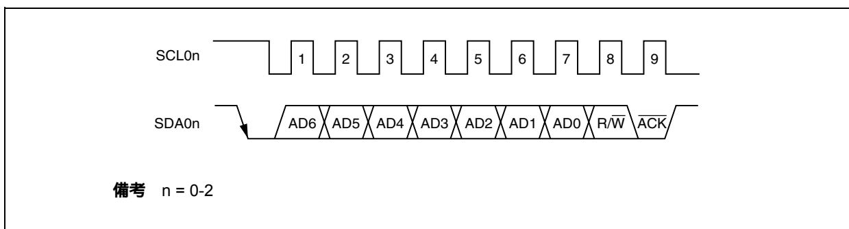
図17 - 11 アクノリッジ (ACK)
