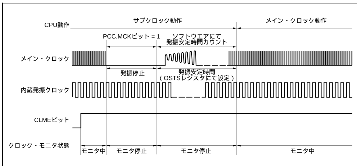
図26 - 5 メイン・クロック停止時 (任意) の動作
