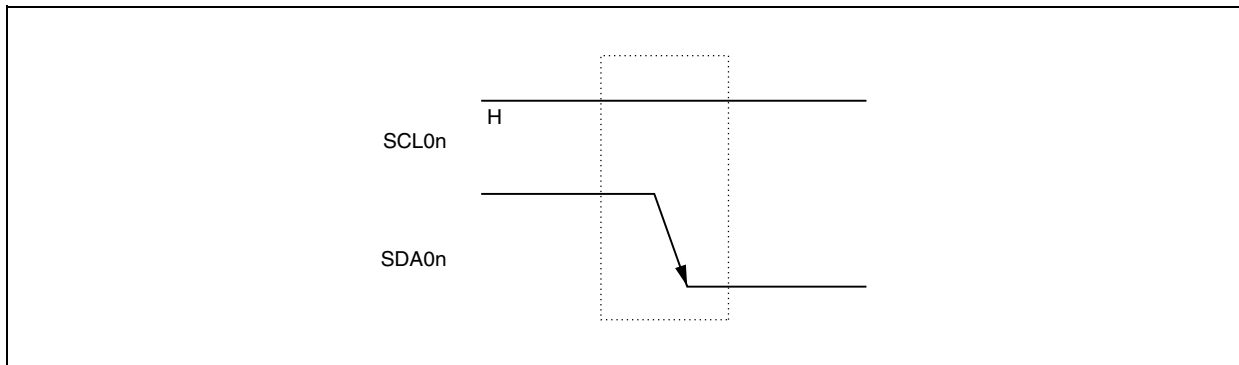
図17-8 スタート・コンディション
