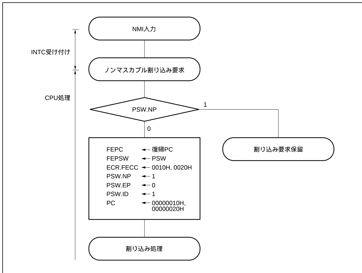
図22 - 2 ノンマスクابل割り込みの処理形態
