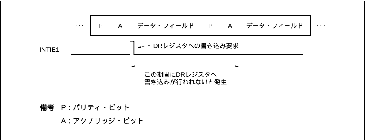
図18 - 14 オーバラン・エラーの発生タイミング
