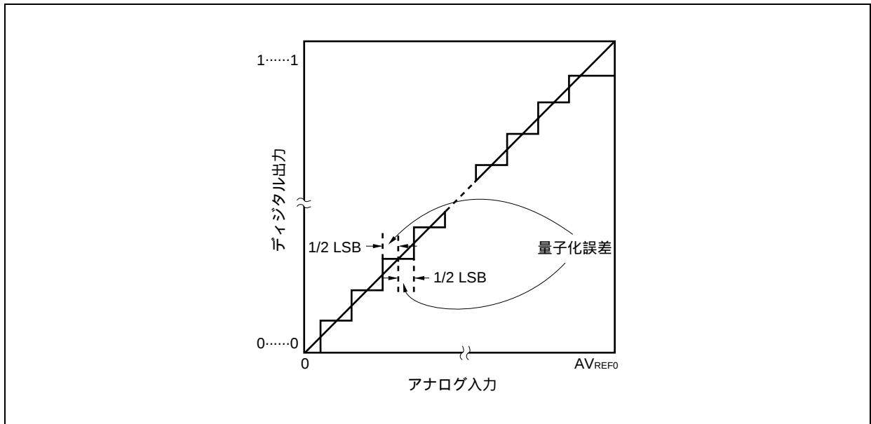
図13 - 17 量子化誤差
