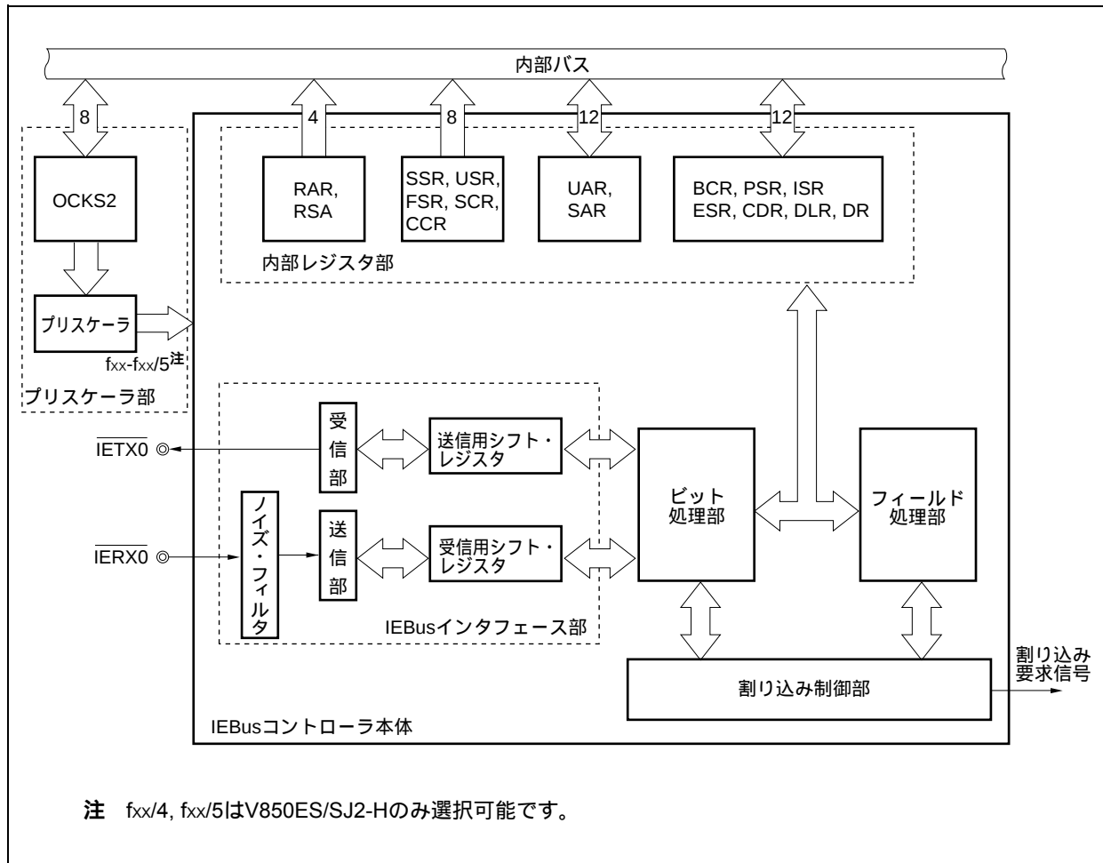
図18 - 10 IEBusコントローラのブロック図
