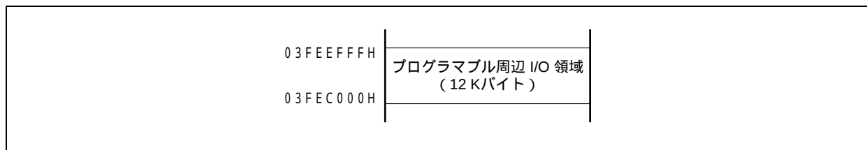
図3 - 11 プログラマブル周辺I/O領域
