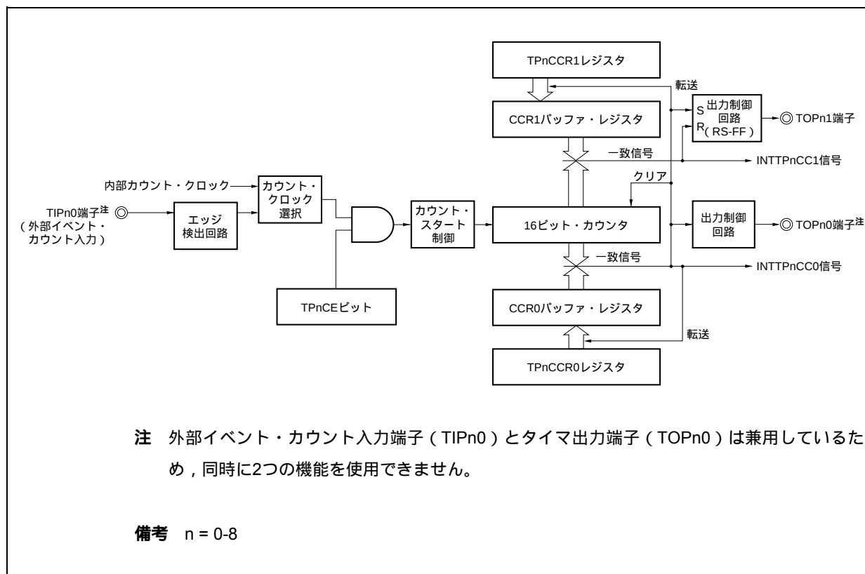
図7 - 28 PWM出力モードの構成図
