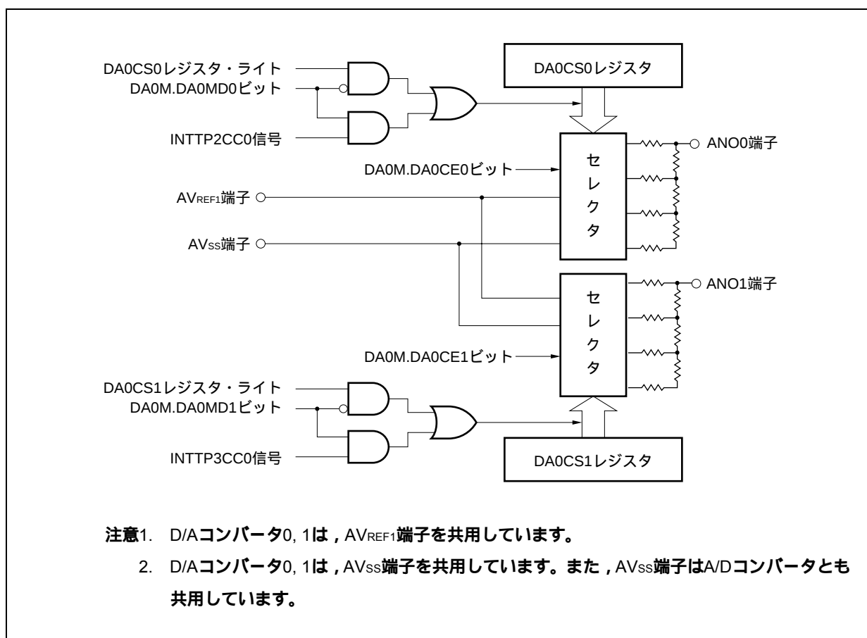
図14 - 1 D/Aコンバータのブロック図
