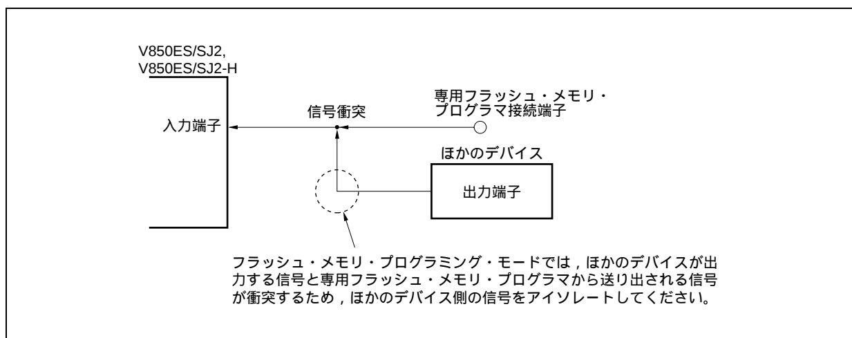
図30 - 12 信号の衝突（シリアル・インタフェースの入力端子）
