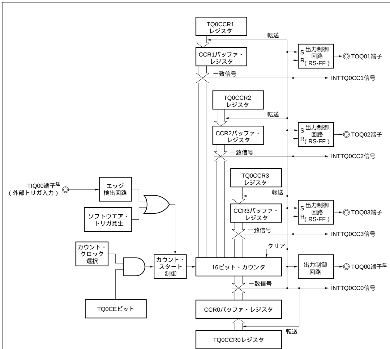
図8 - 20 外部トリガ・パルス出力モードの構成図
