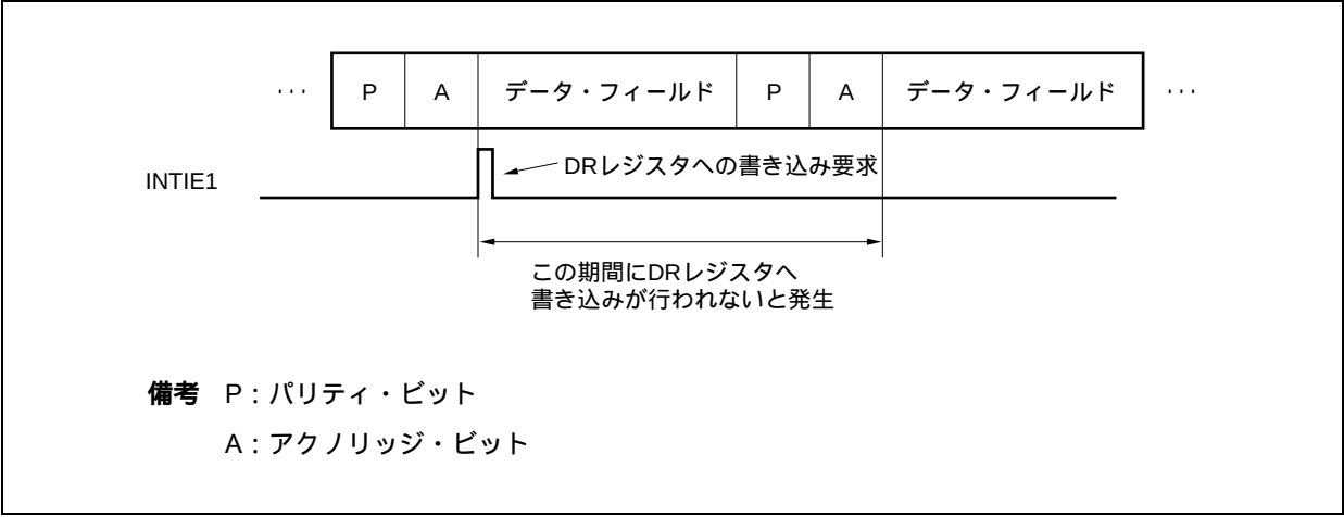
図18 - 13 アンダラン・エラーの発生タイミング
