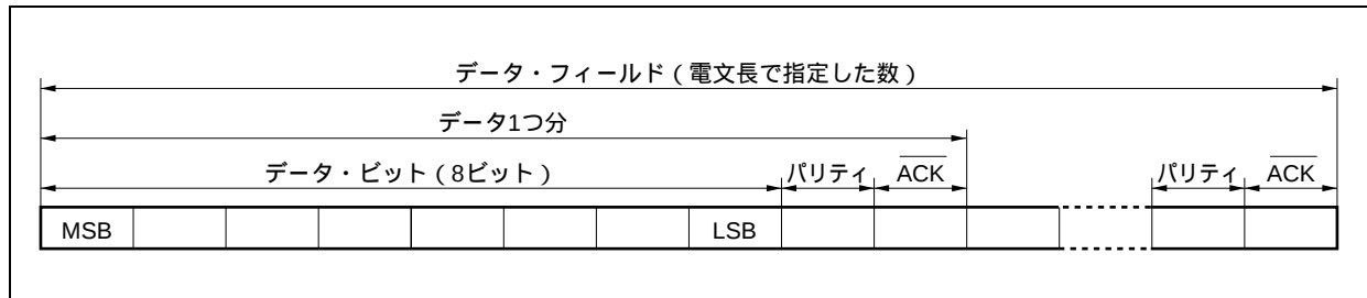
図18 - 6 データ・フィールド
