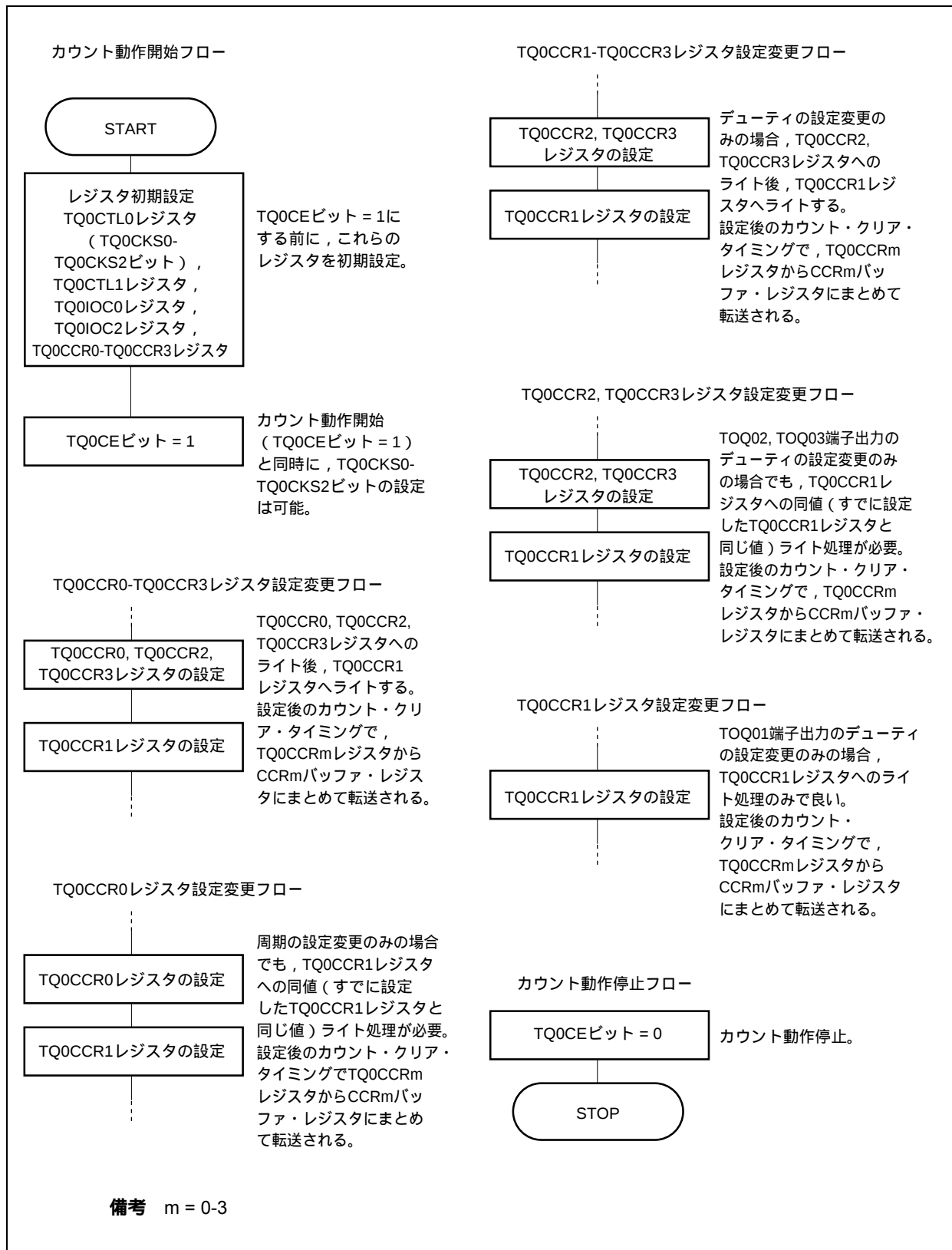
図8 - 31 PWM出力モード使用時のソフトウェア処理フロー (2/2)
