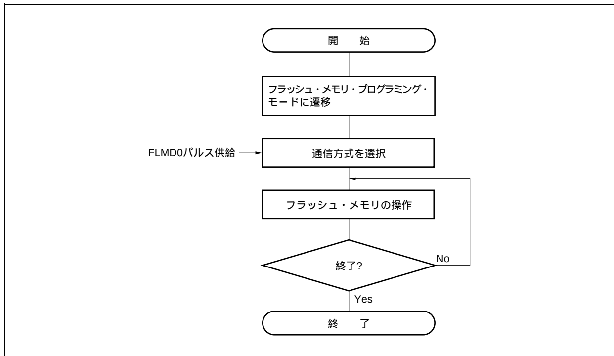
図30 - 7 フラッシュ・メモリの操作手順
