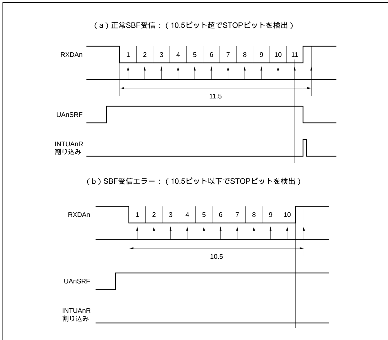
図15 - 9 SBF受信
