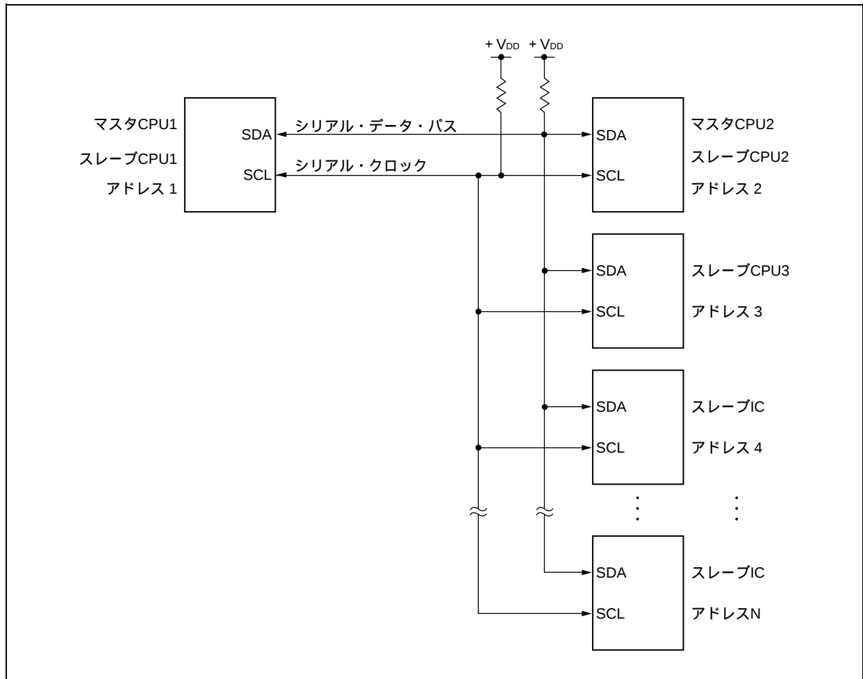
図17 - 5 I 2 Cバスによるシリアル・バス構成例
