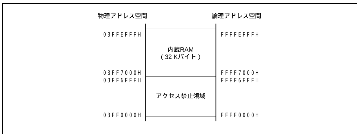
図3 - 7 内蔵RAM領域 (32 Kバイト)
