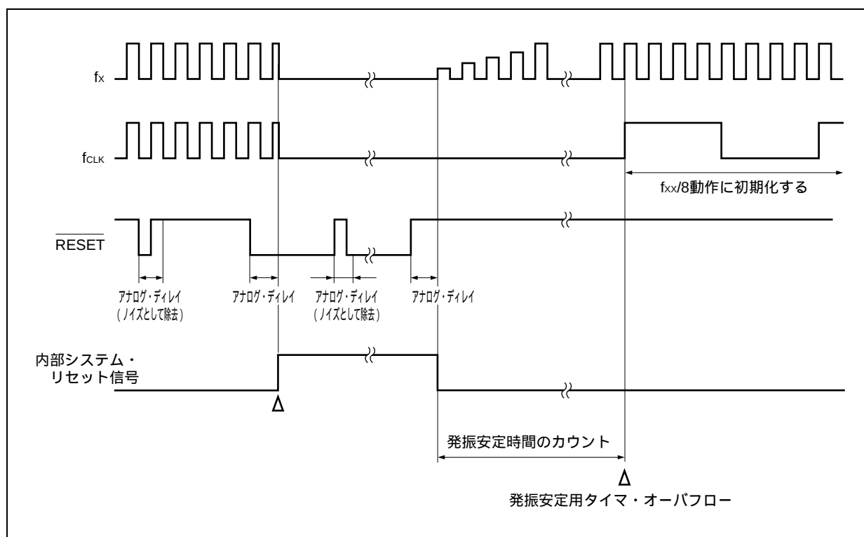
図25 - 3 パワーオン時のリセット動作のタイミング
