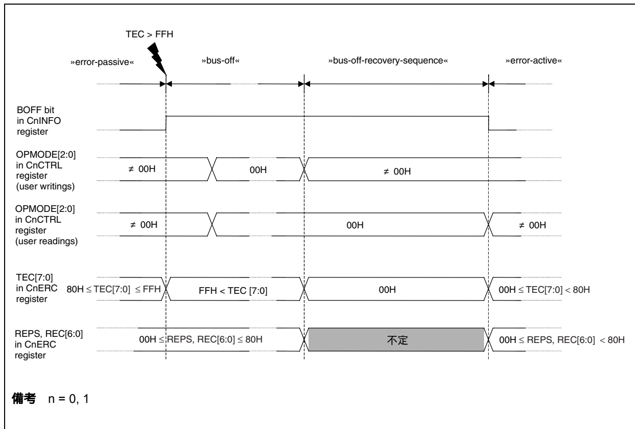
図19 - 17 通常リカバリ・シーケンスによるバス・オフからの復帰動作
