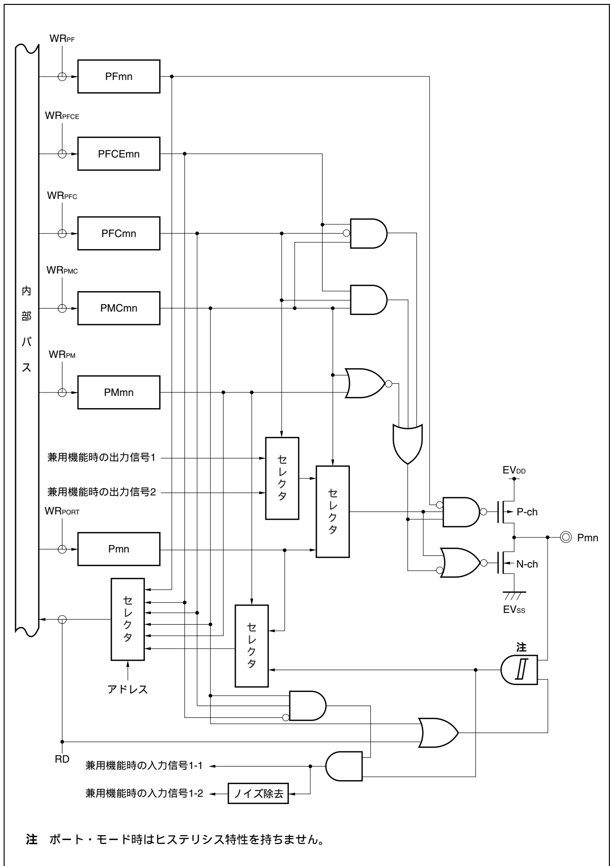
図4 - 29 タイプU - 5のブロック図
