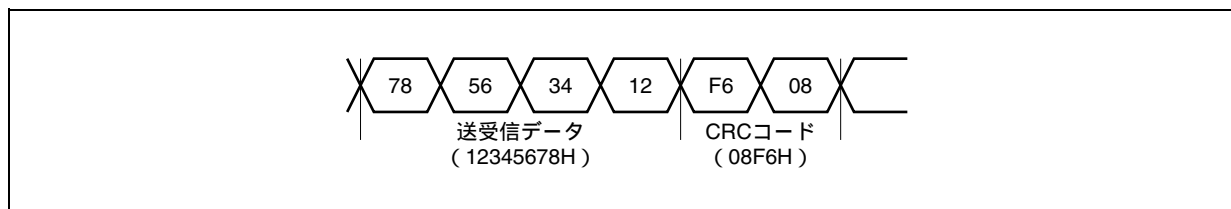
図21 - 4 CRC送信例
