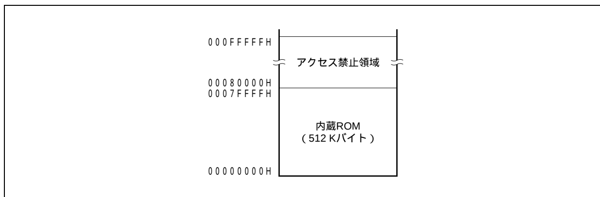
図3 - 5 内蔵ROM領域 (512 Kバイト)
