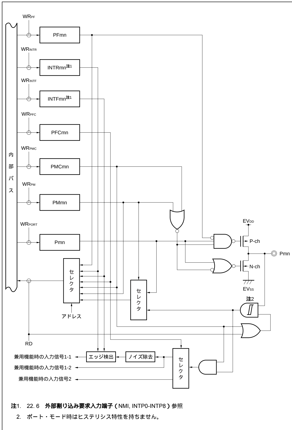
図4 - 24 タイプN - 3のブロック図
