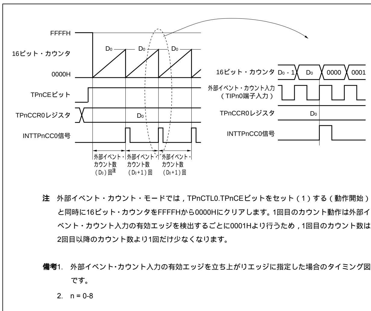
図7-14 外部イベント・カウント・モードの基本タイミング
