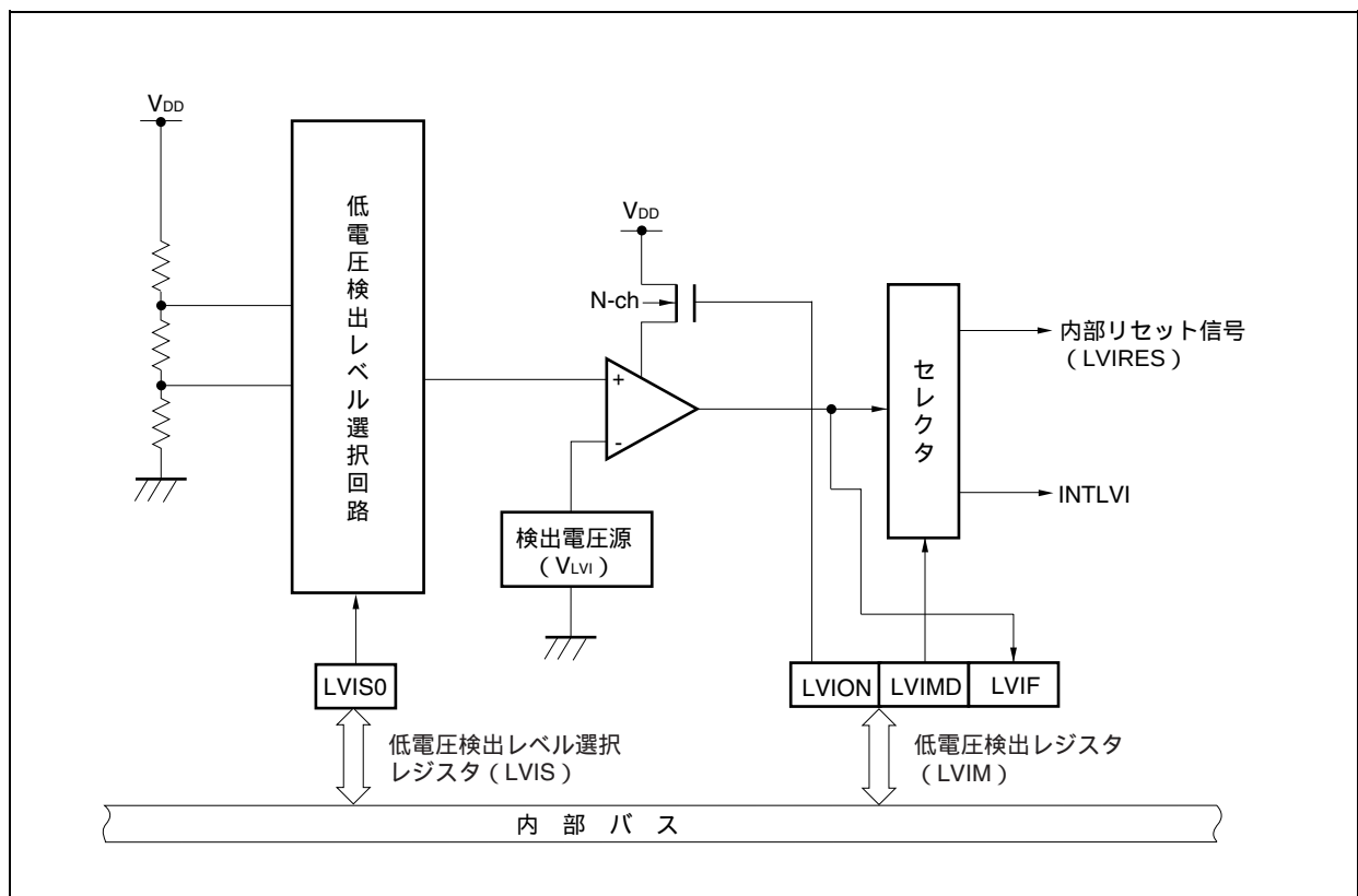
図27 - 1 低電圧検出回路のブロック図
