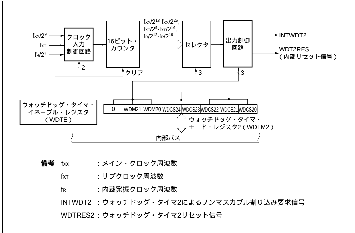
図11 - 1 ウォッチドッグ・タイマ2のブロック図
