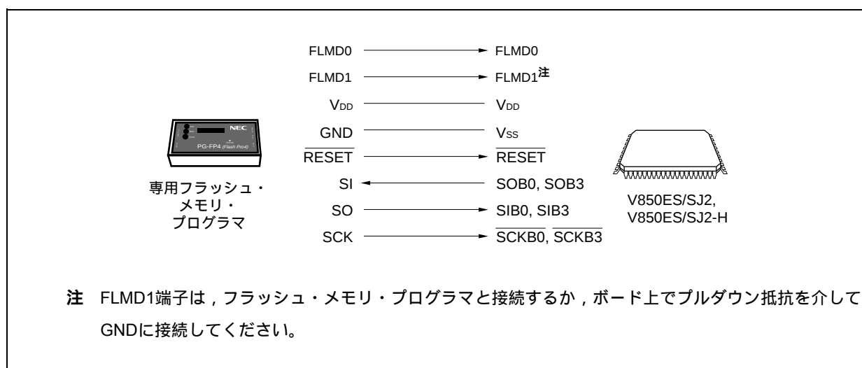
図30 - 4 専用フラッシュ・メモリ・プログラマとの通信 (CSIB0, CSIB3)
