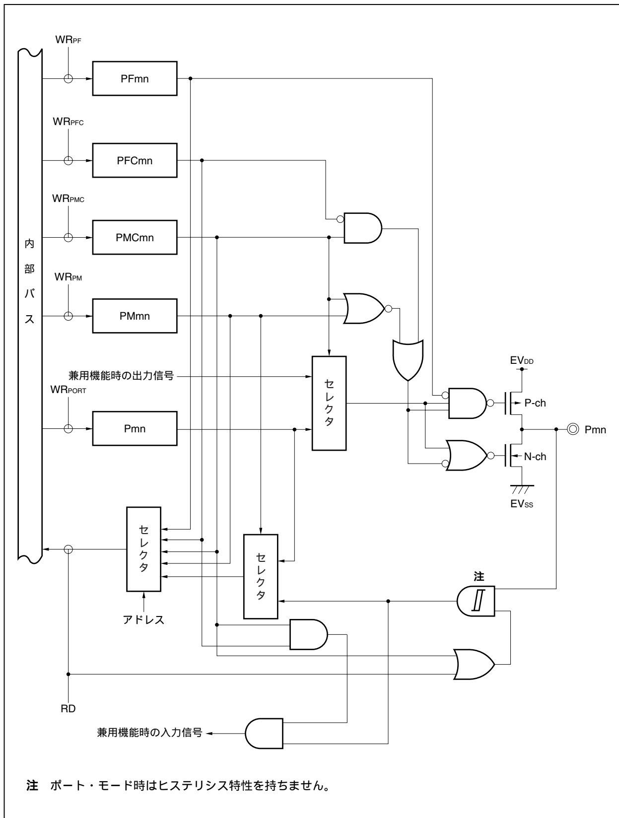
図4 - 14 タイプG - 2のブロック図
