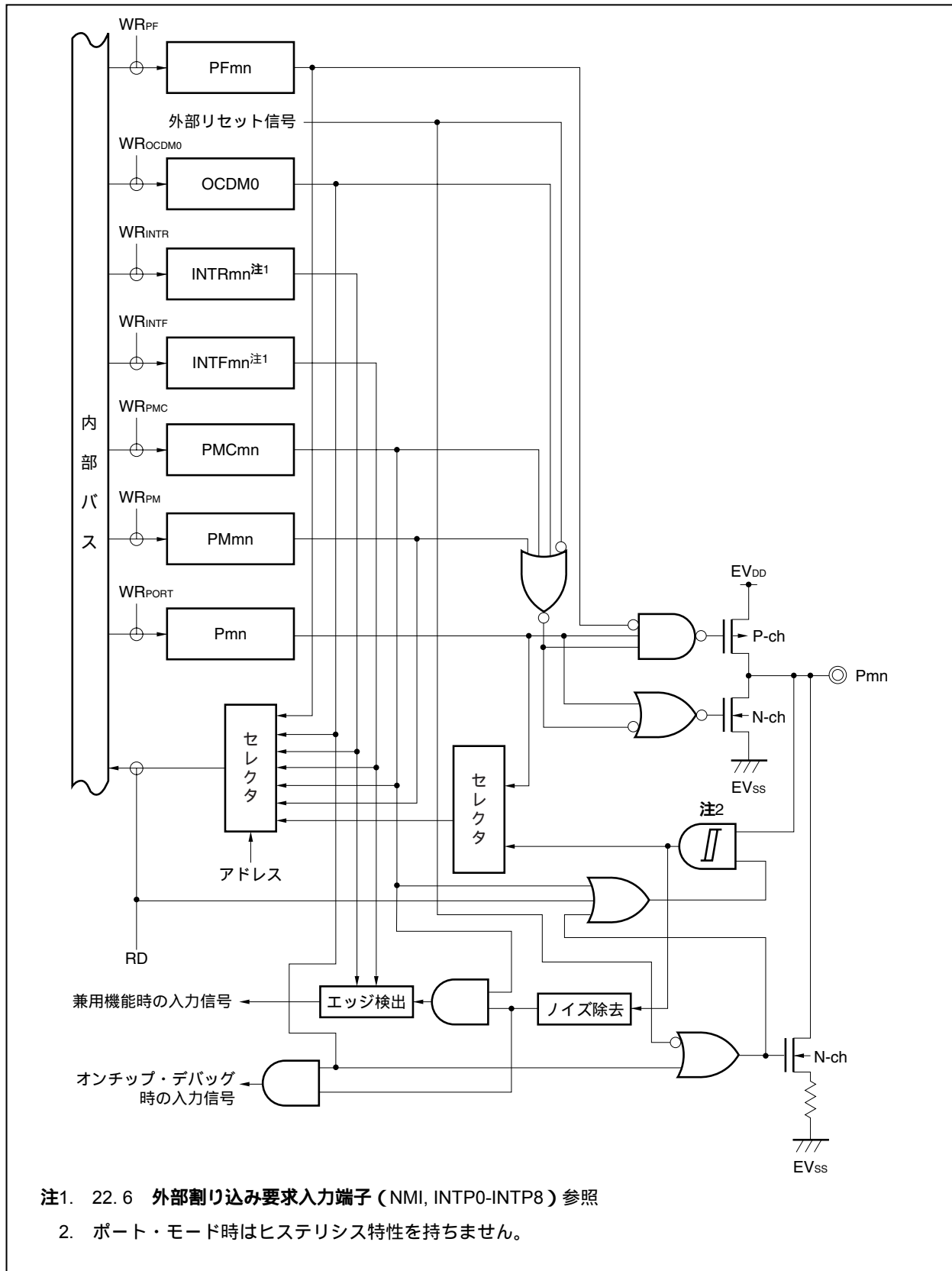
図4 - 40 タイプAA - 1のブロック図
