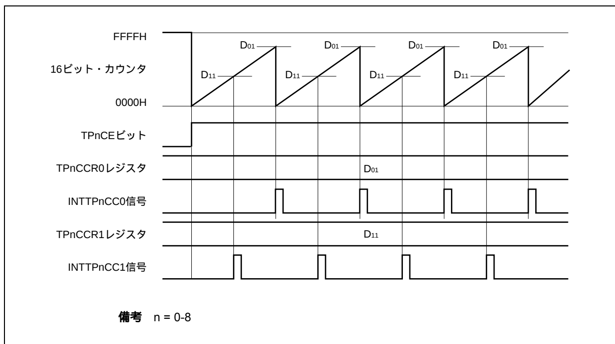
図7 - 18 D01 D11の場合のタイミング図
