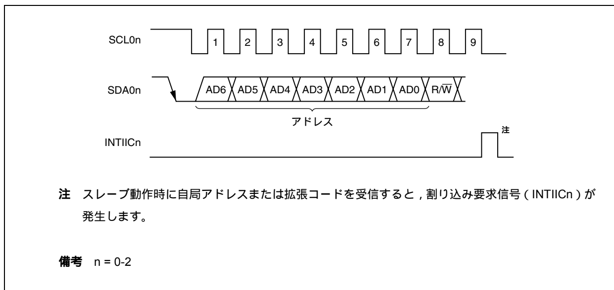
図17-9 アドレス
