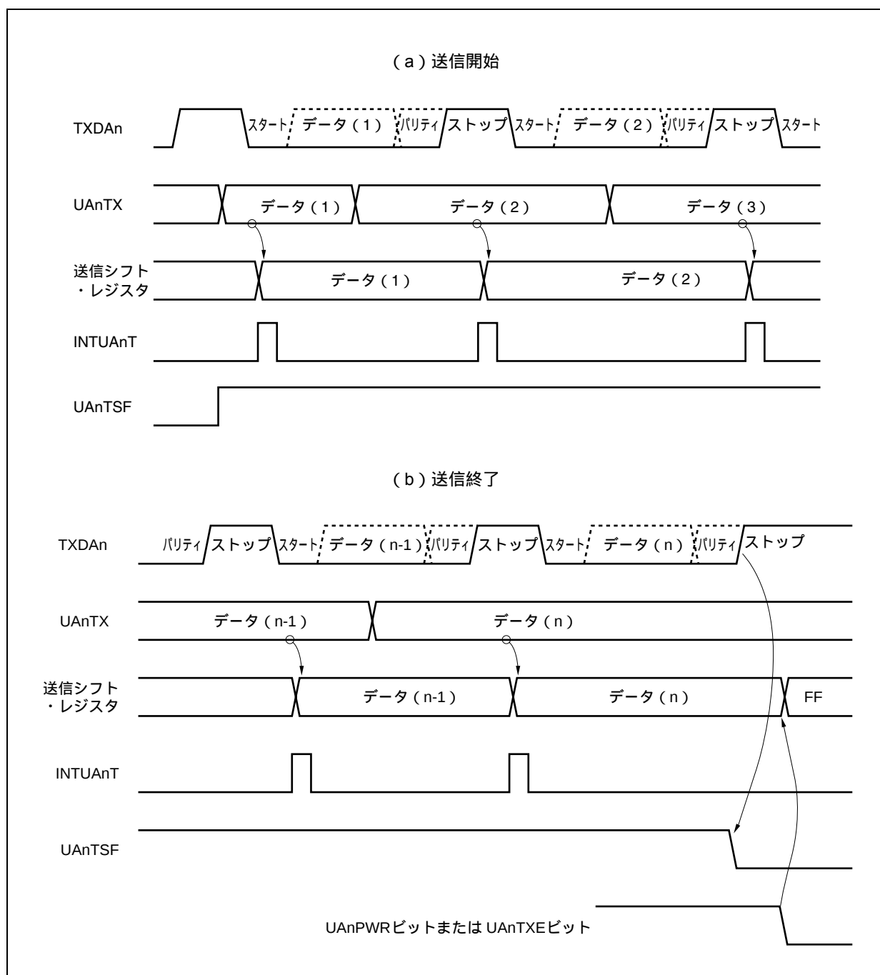
図15 - 12 連続送信動作のタイミング
