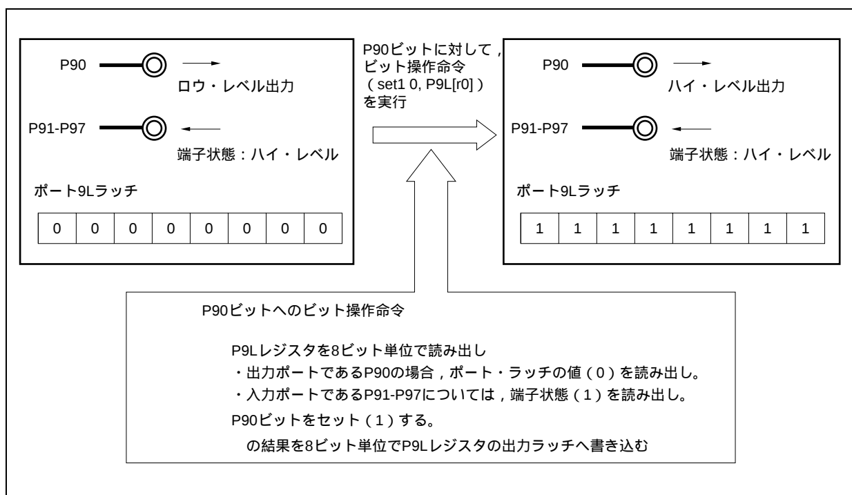
図4 - 43 ビット操作命令（P90端子の場合）
