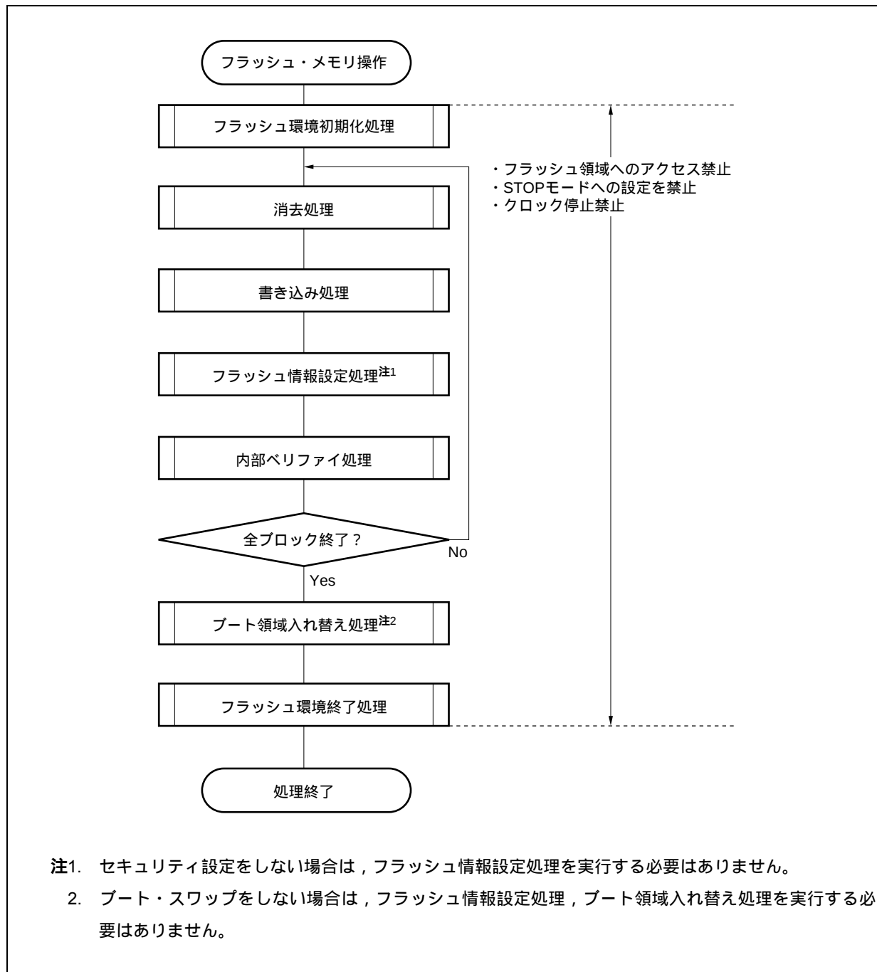
図30 - 17 標準セルフ・プログラミング・フロー
