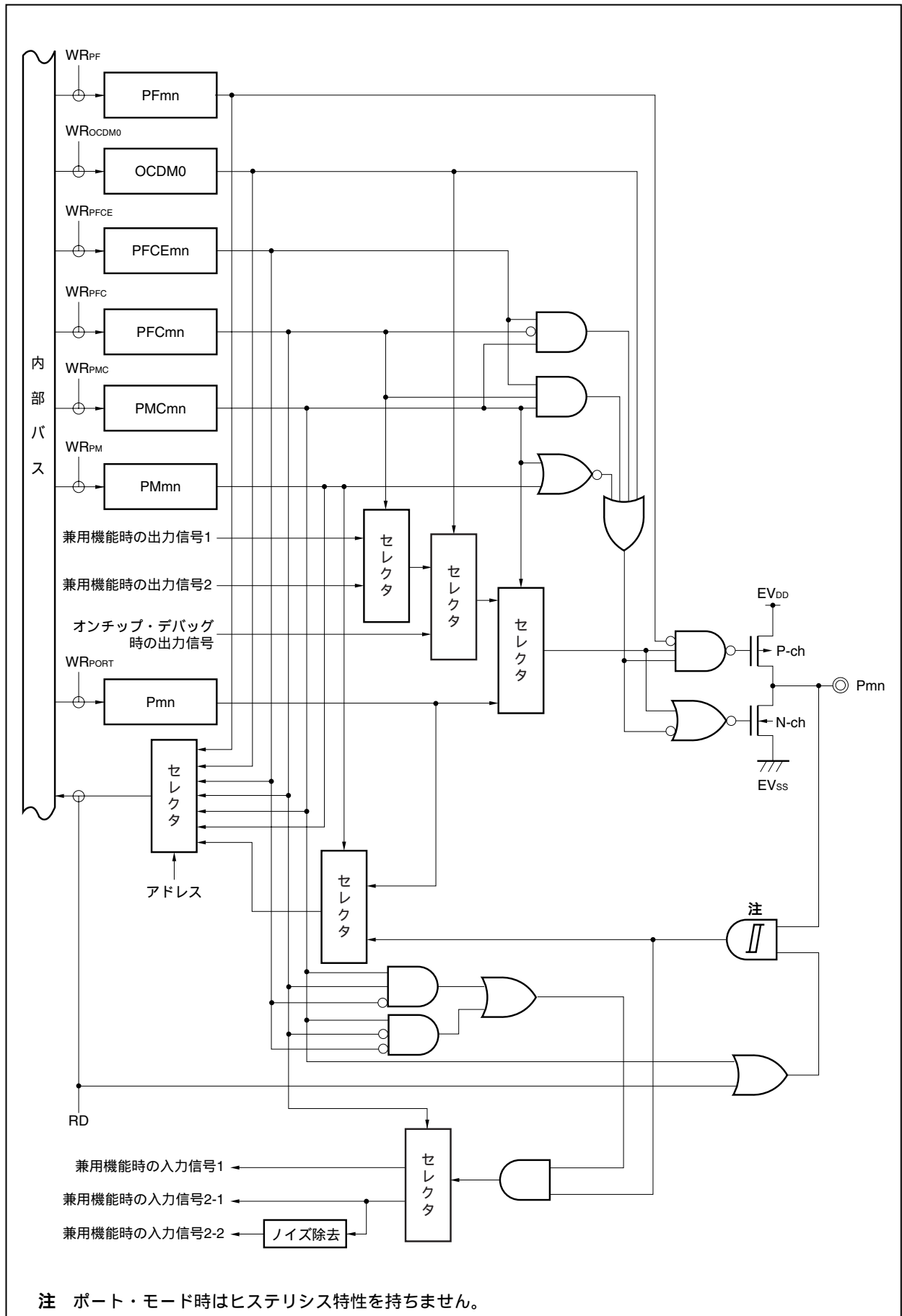
図4 - 31 タイプU - 7のブロック図
