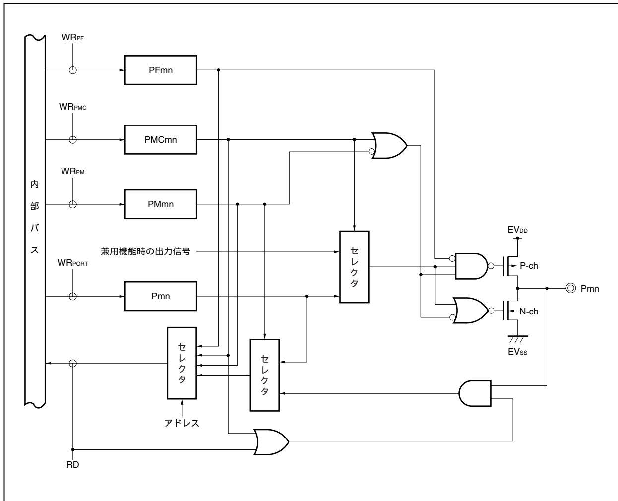
図4 - 11 タイプE - 2のブロック図
