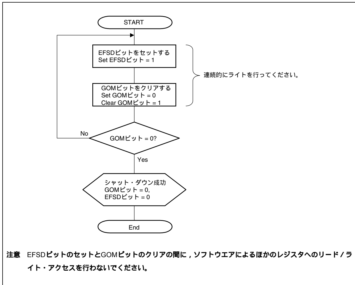
図19 - 57 強制シャット・ダウン処理
