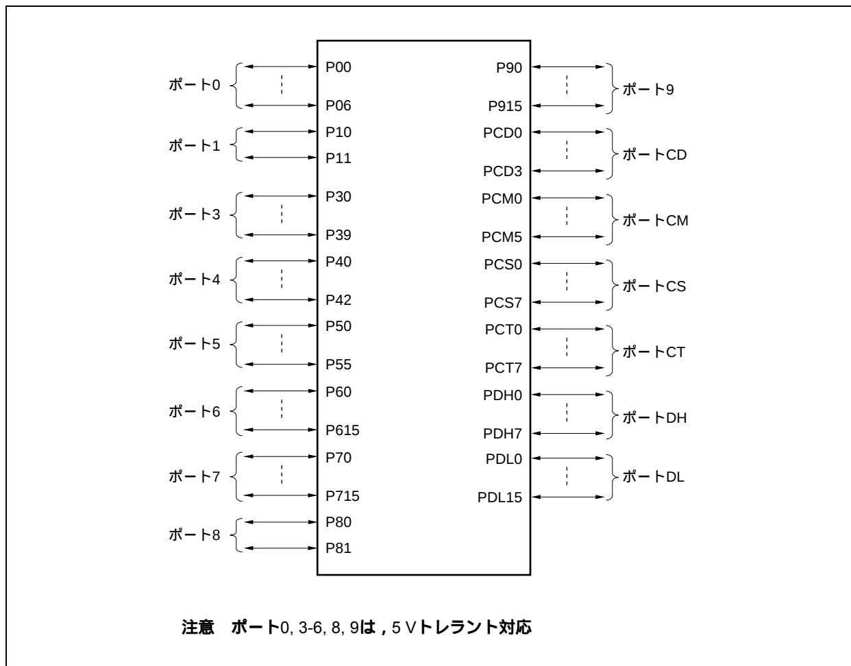
図4 - 1 ポートの構成図
