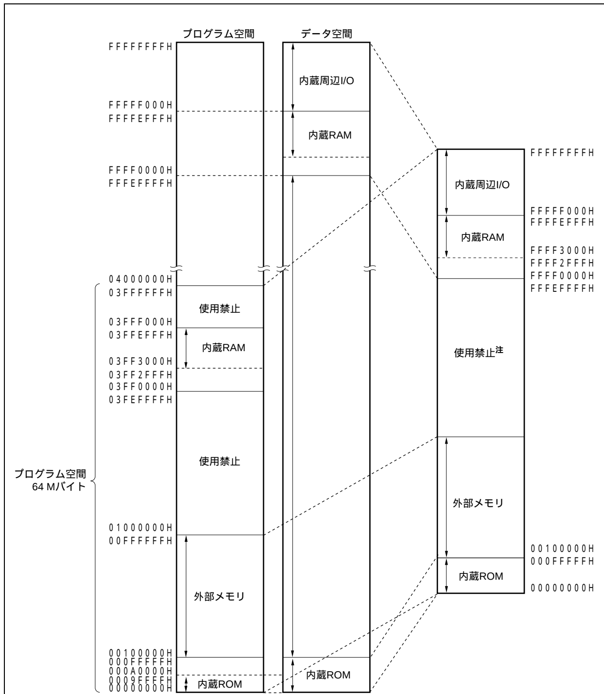
図3 - 12 推奨メモリ・マップ
