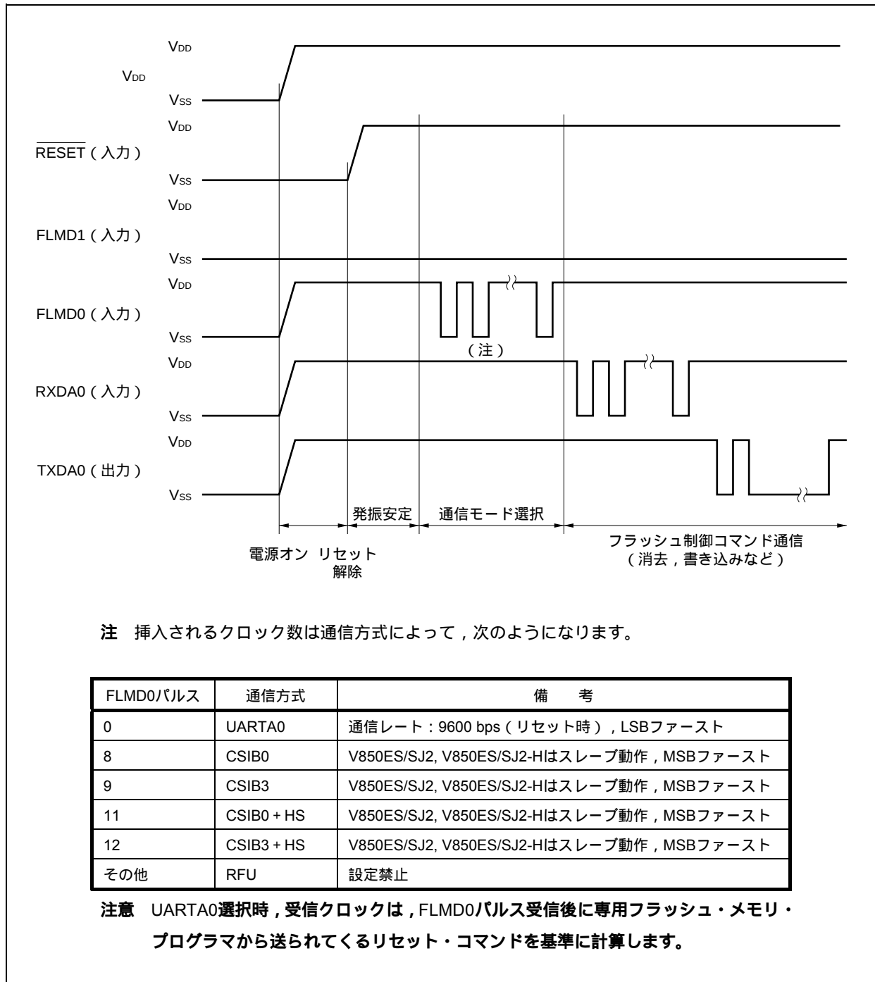
図30 - 8 通信方式の選択
