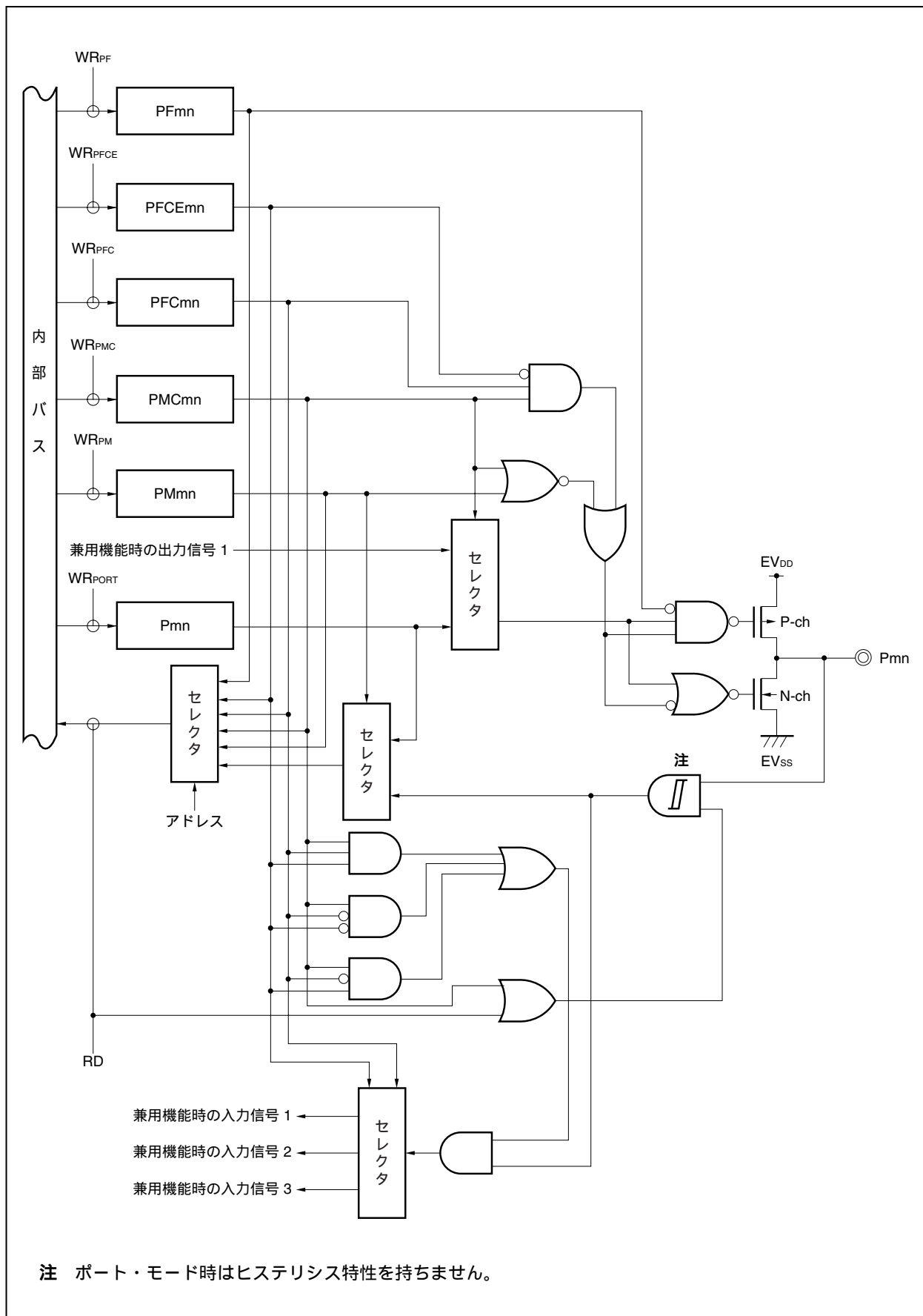
図4 - 27 タイプU - 3のブロック図
