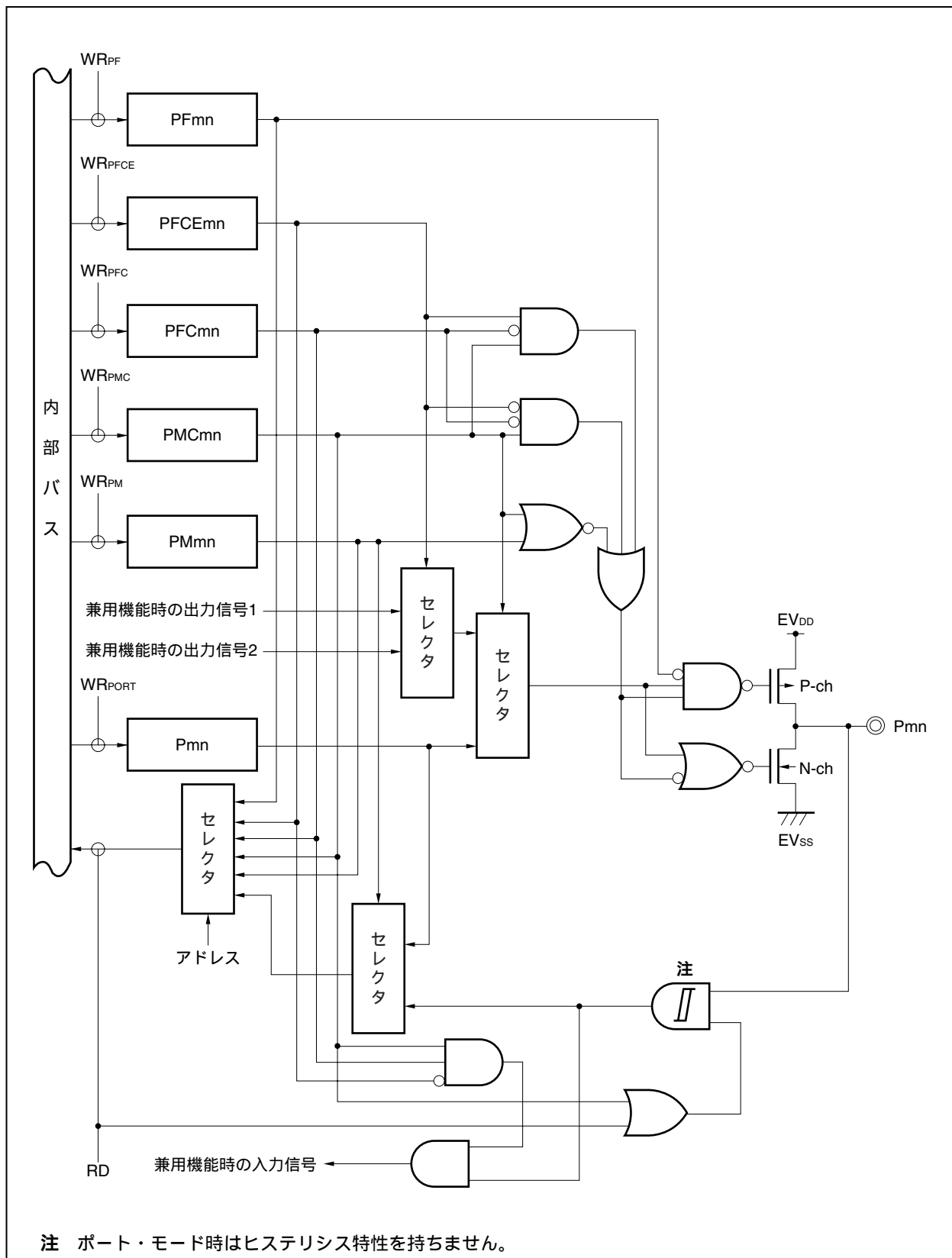
図4 - 36 タイプU - 12のブロック図
