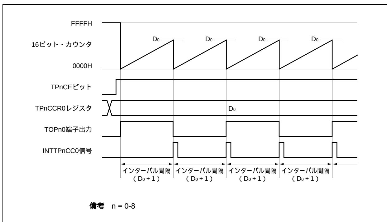
図7-7 インターバル・タイマ・モード動作の基本タイミング
