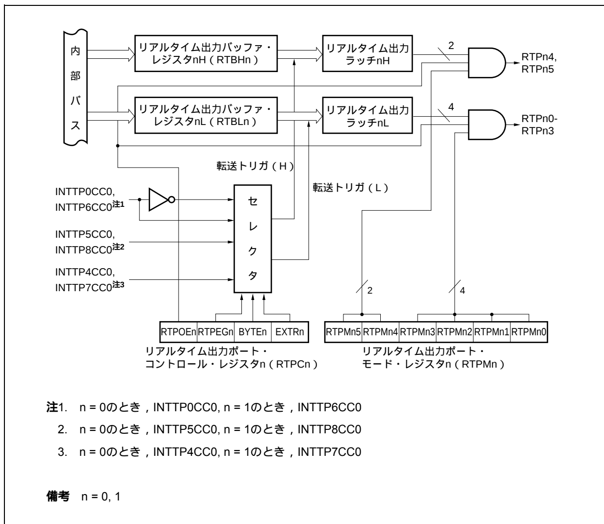
図12 - 1 RTOのブロック図
