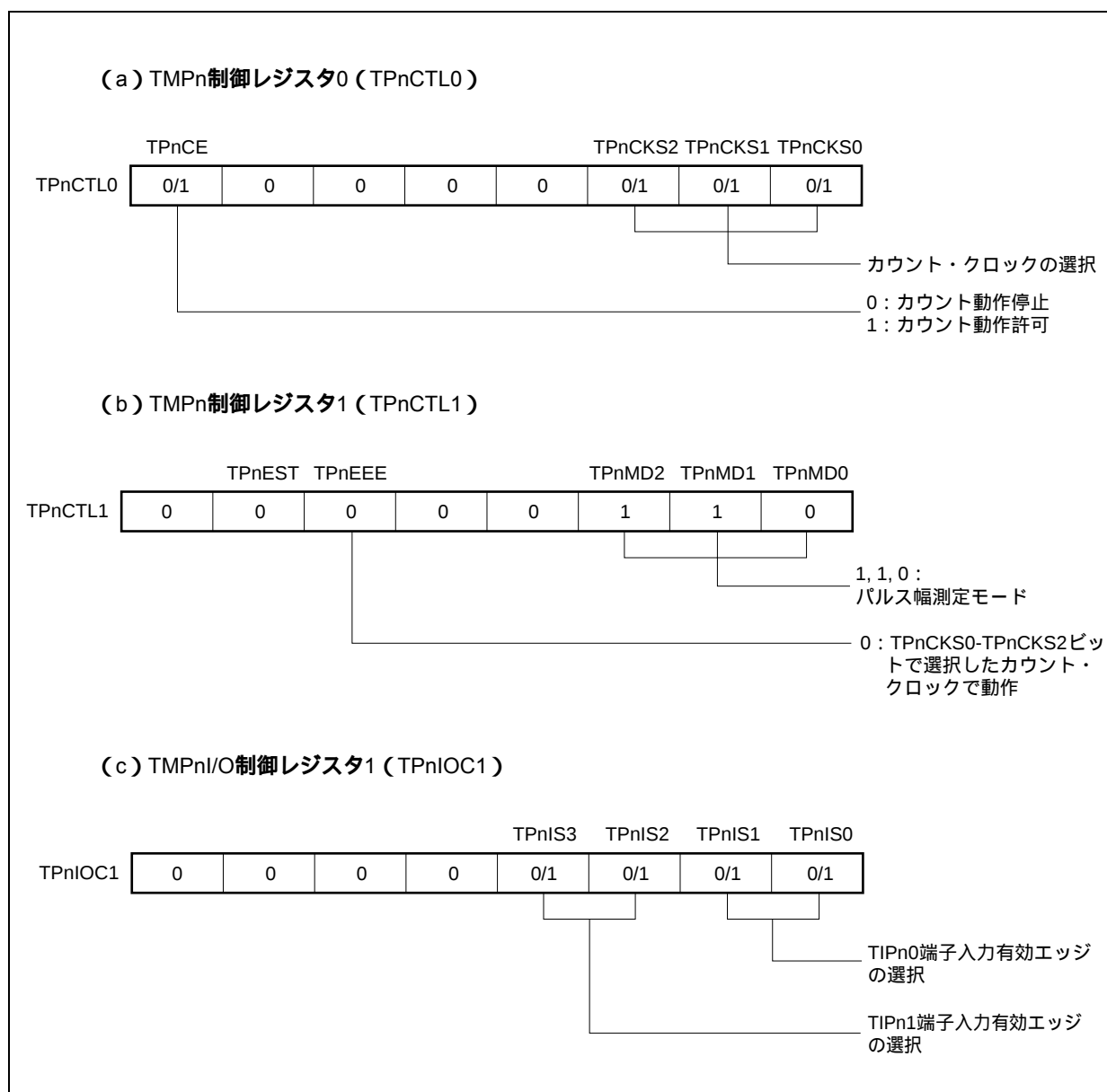
図7 - 40 パルス幅測定モード動作時のレジスタ設定内容 (1/2)
