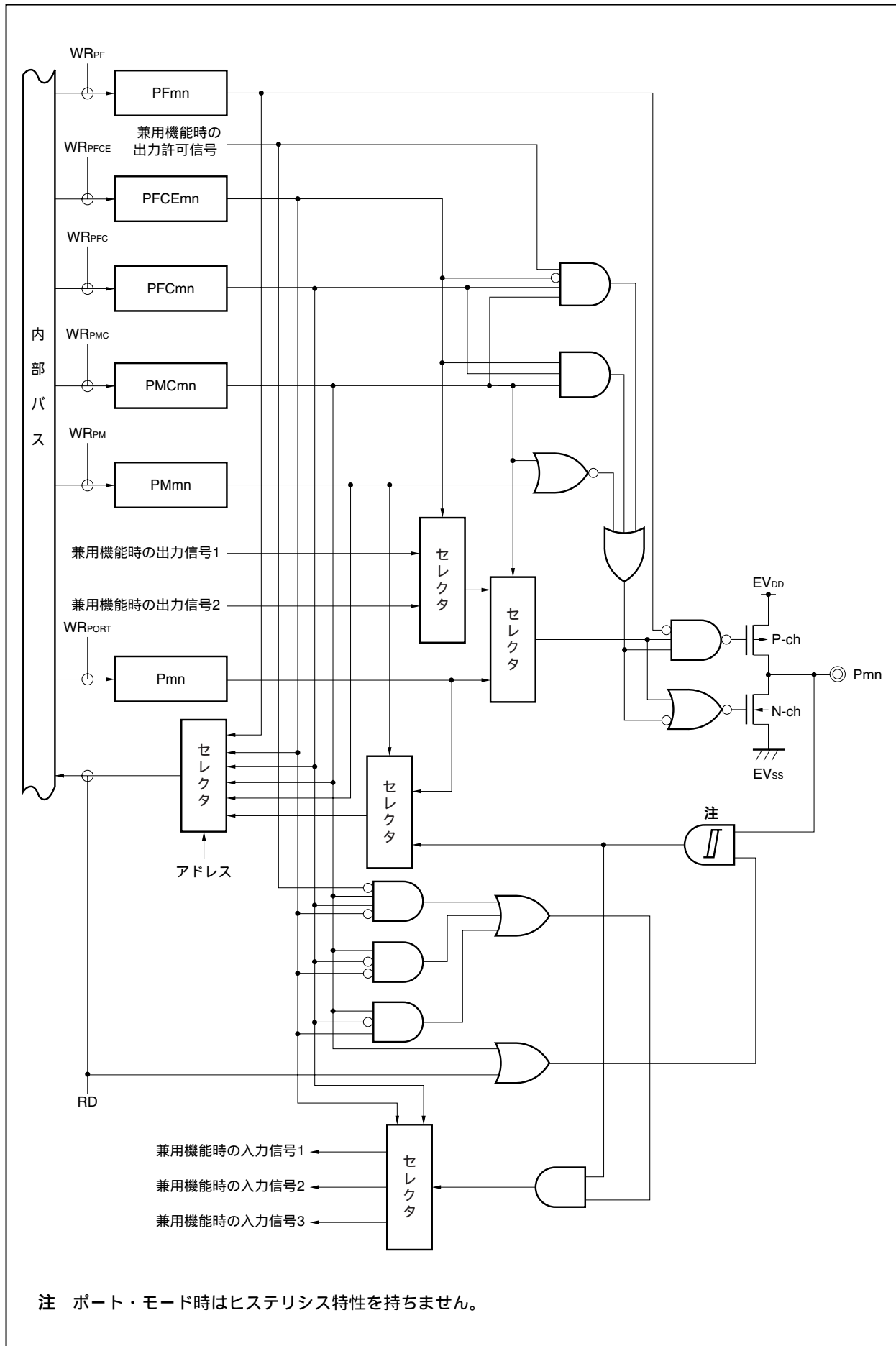
図4 - 25 タイプU - 1のブロック図
