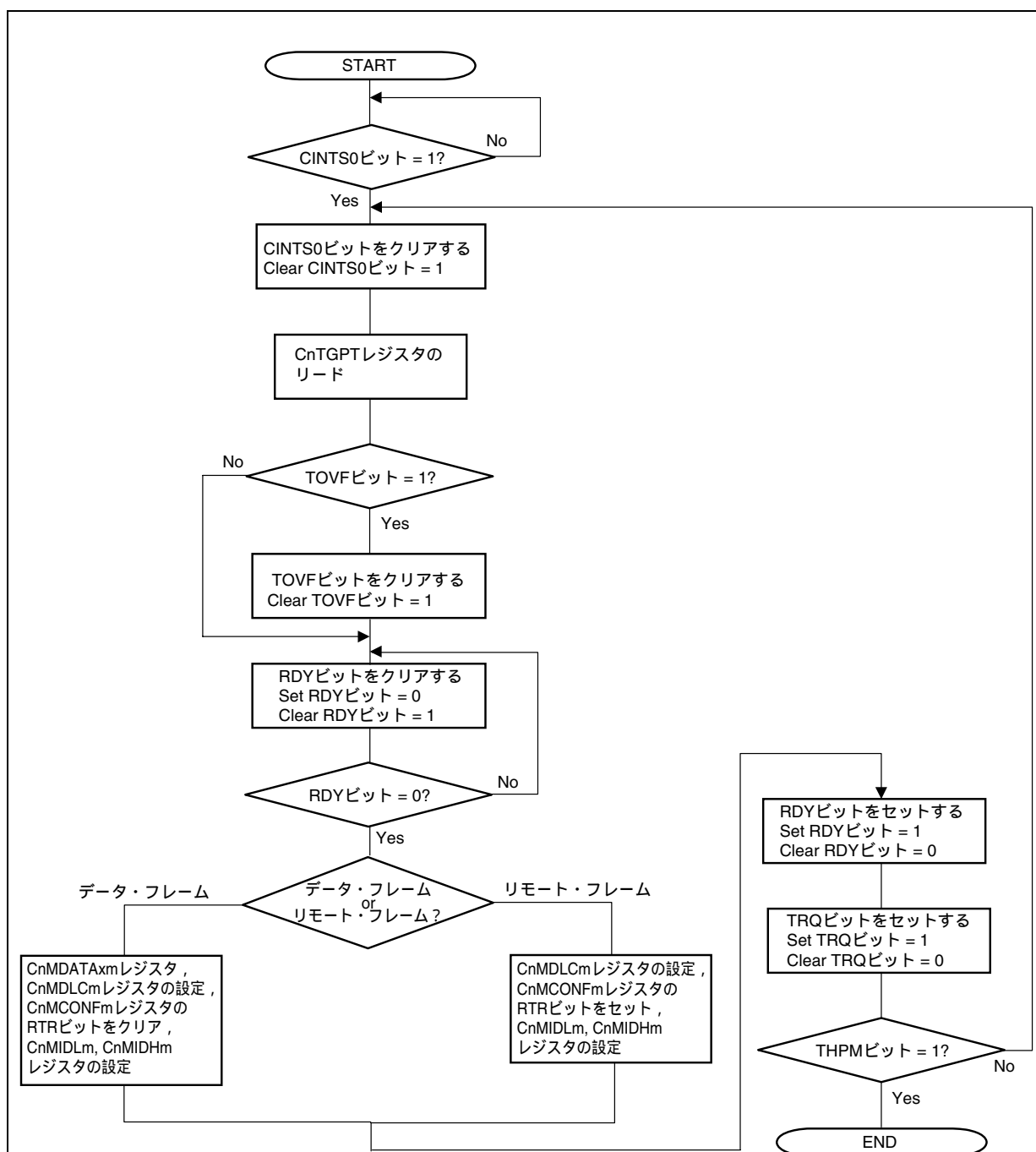
図19 - 45 ソフトウェア・ポーリングによる送信処理
