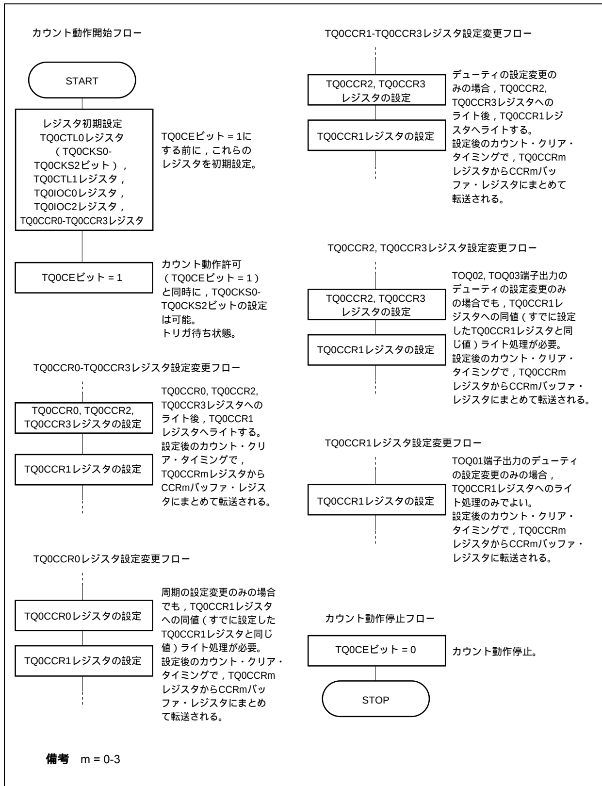
図8 - 23 外部トリガ・パルス出力モード使用時のソフトウェア処理フロー (2/2)
