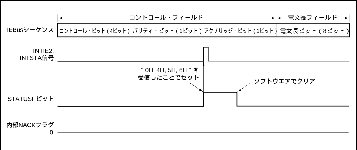
図18 - 16 割り込み要求信号発生タイミング（ , , の場合）
