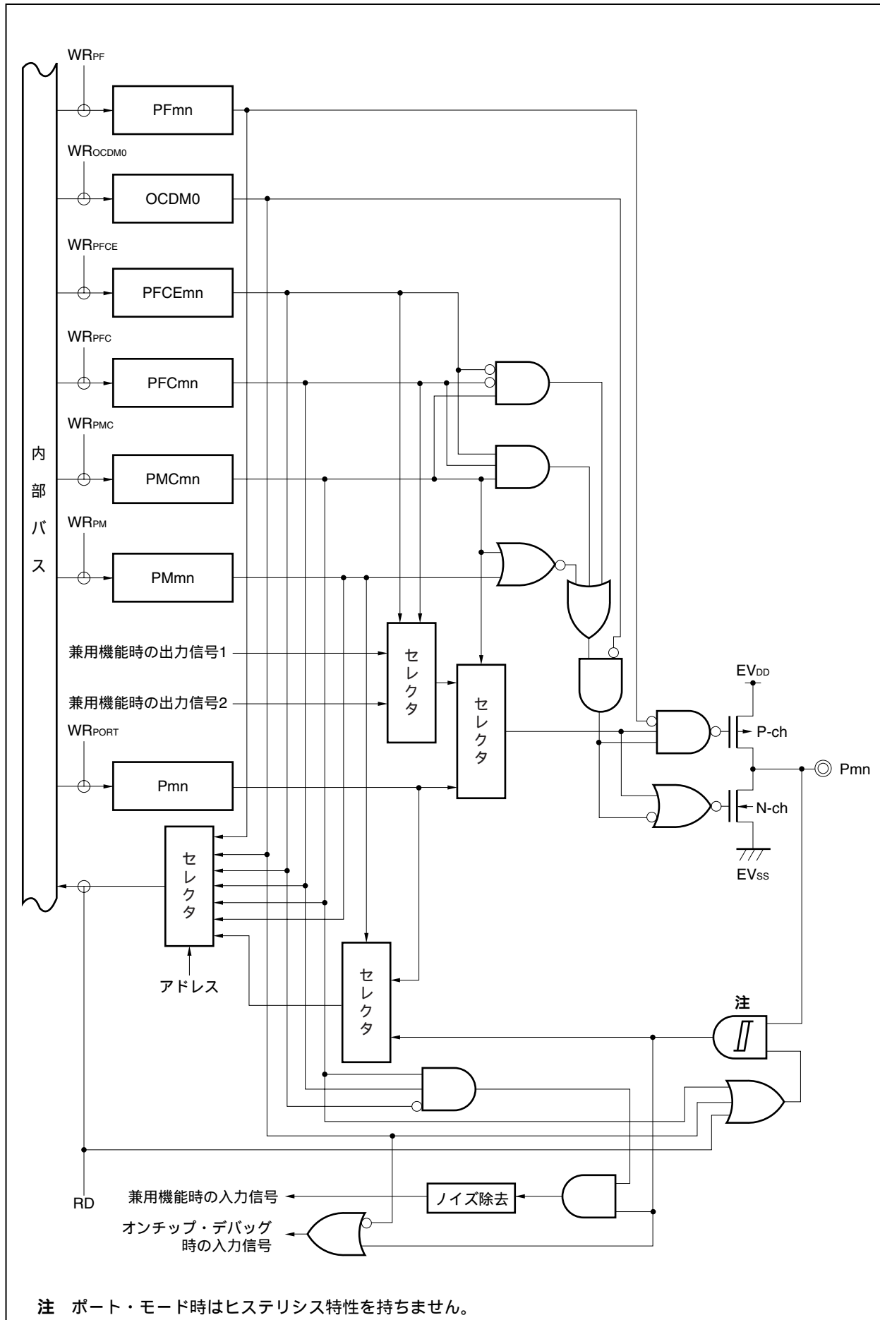
図4 - 32 タイプU - 8のブロック図
