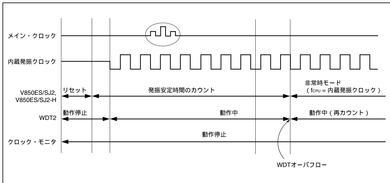
図25 - 7 リセット解除後の動作
