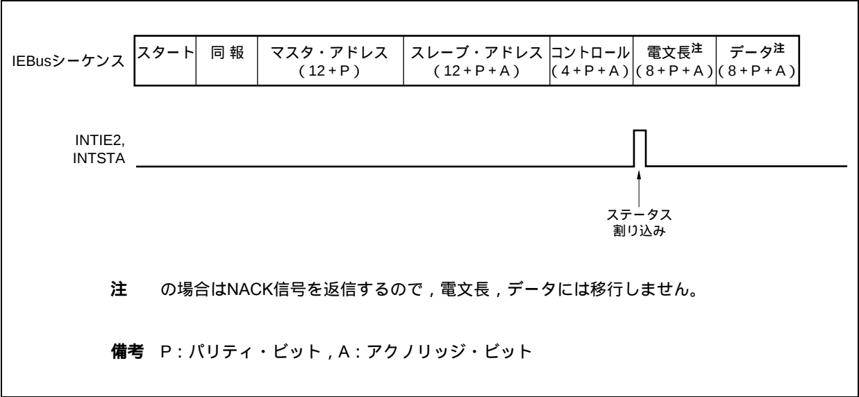
図18 - 18 ロック状態中のINTIE2, INTSTA割り込み要求信号発生タイミング（ , の場合）
