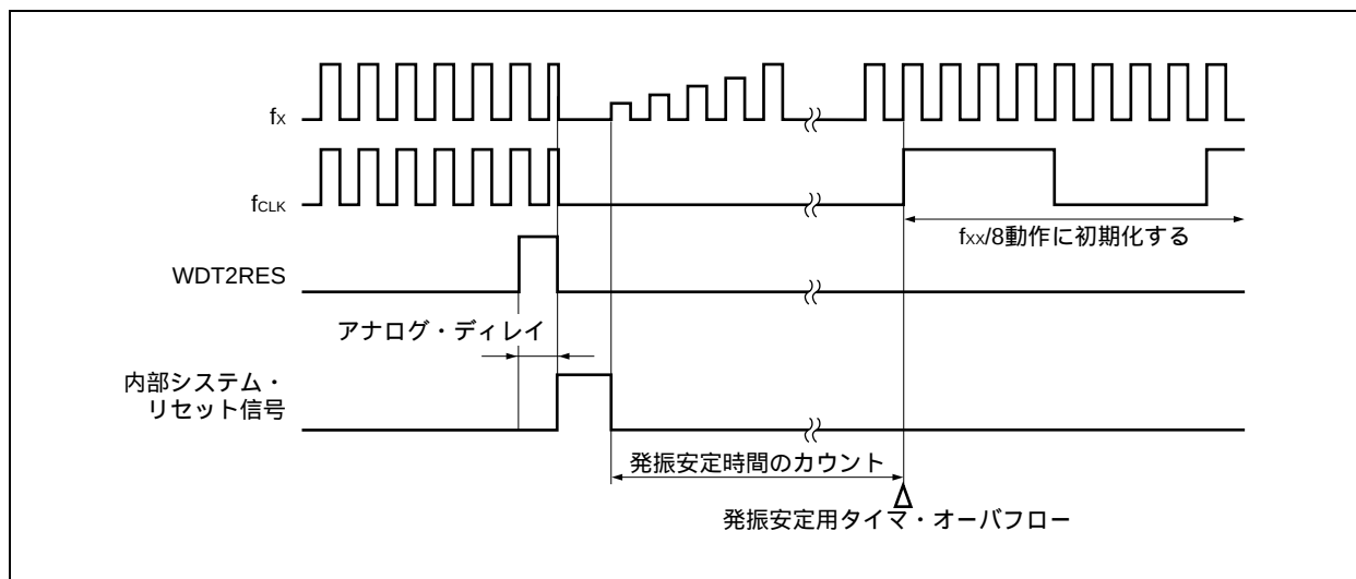
図25 - 4 WDT2RES信号発生によるリセット動作のタイミング
