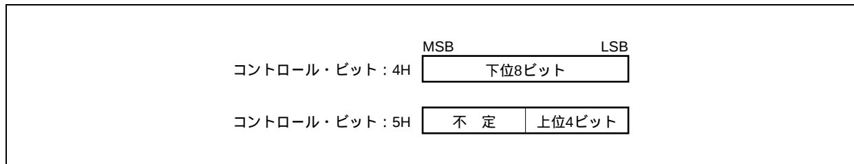
図18 - 8 ロック・アドレスの構成
