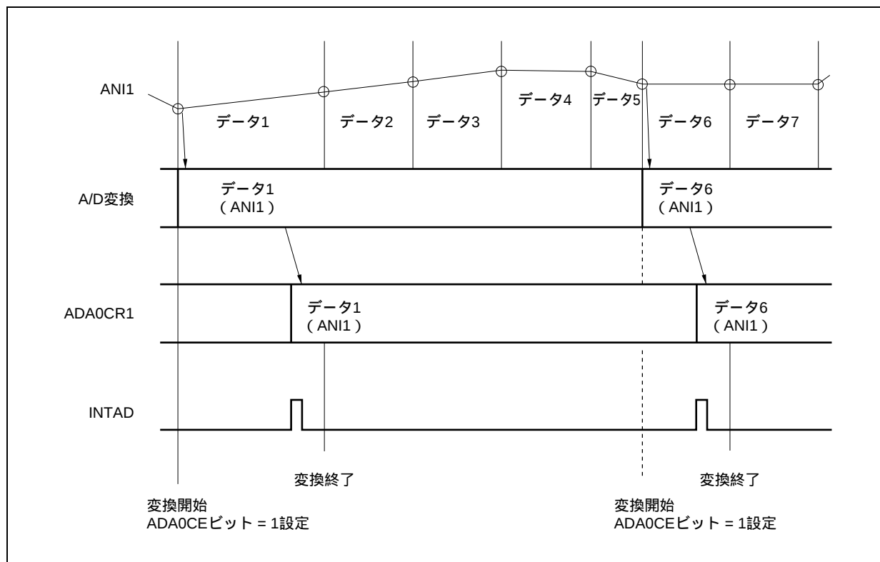
図13 - 6 ワンショット・セレクト・モード動作タイミング例 (ADA0Sレジスタ = 01H)
