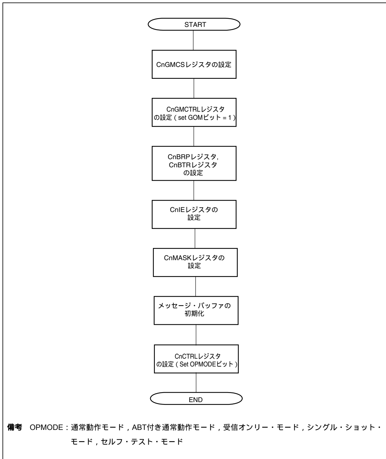
図19 - 36 初期化
