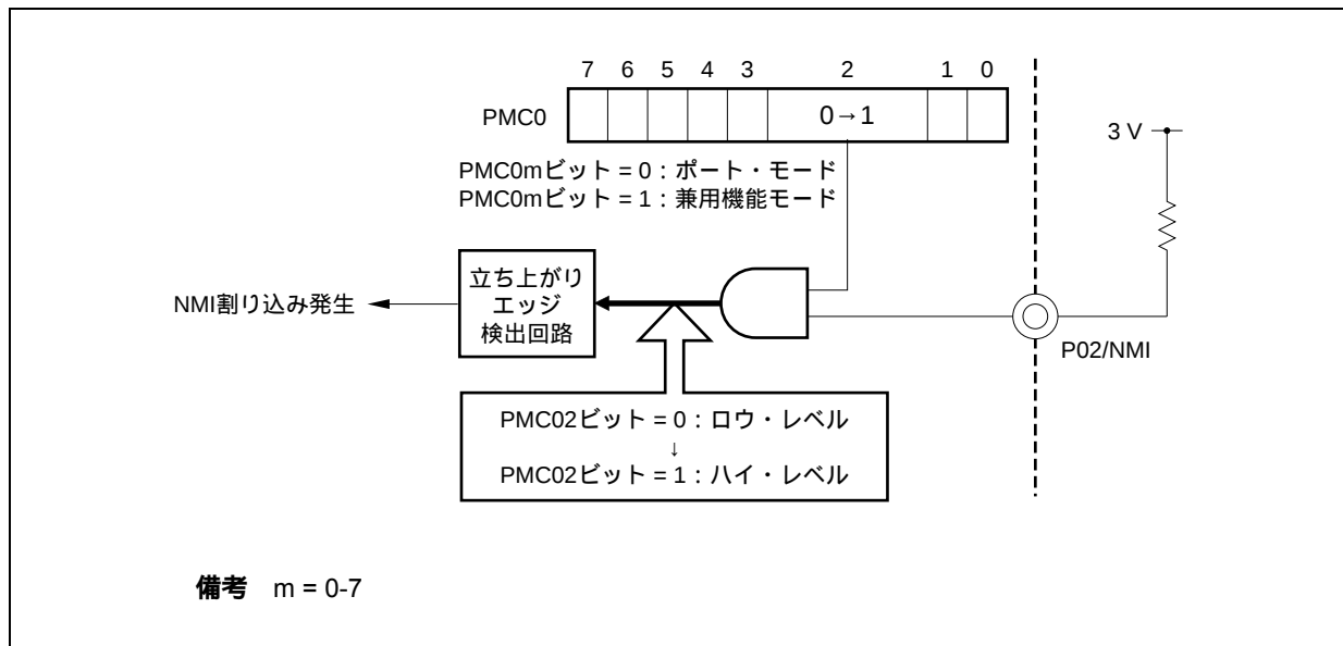
図4 - 41 P02端子からNMI端子への切り替え（悪い例）
