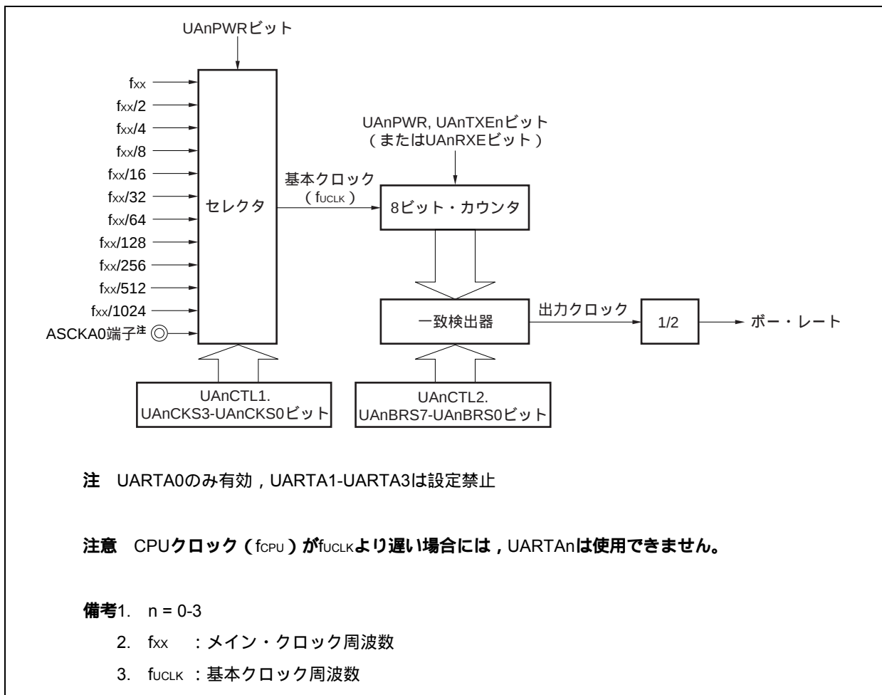
図15 - 16 ボー・レート・ジェネレータの構成
