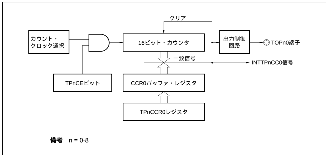
図7-6 インターバル・タイマの構成図
