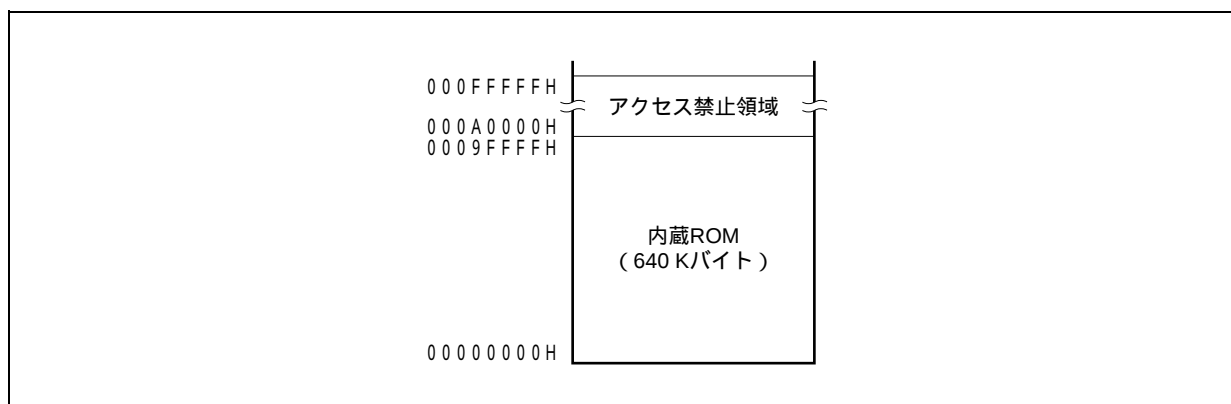
図3 - 6 内蔵ROM領域 (640 Kバイト)
