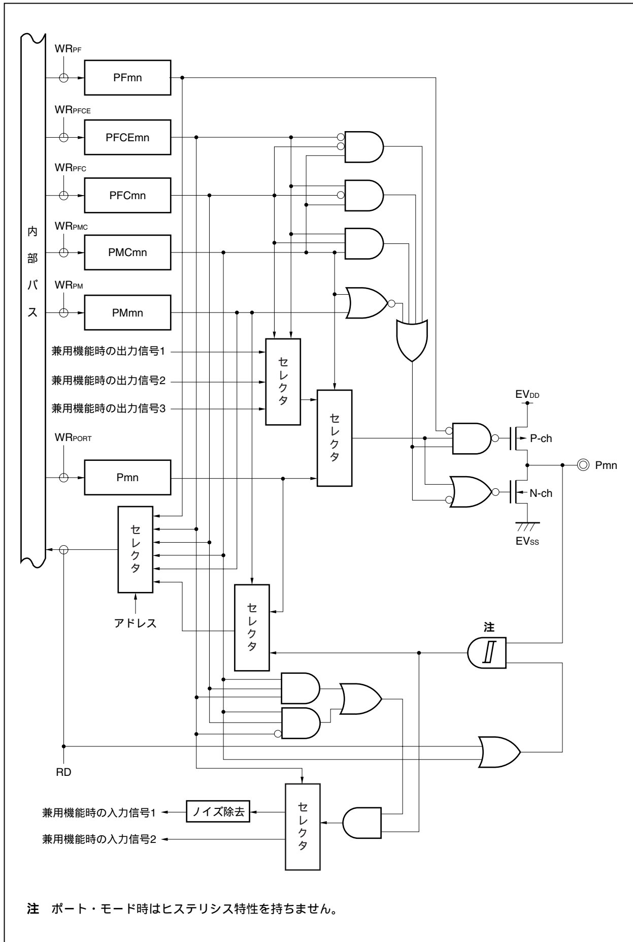
図4 - 34 タイプU - 10のブロック図
