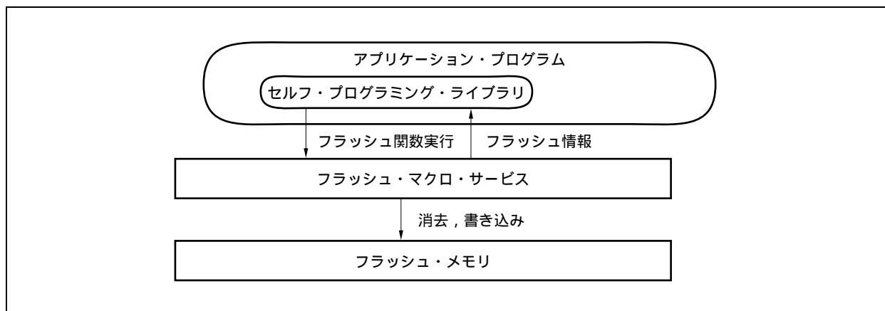
図30 - 15 セルフ・プログラミングの概念図
