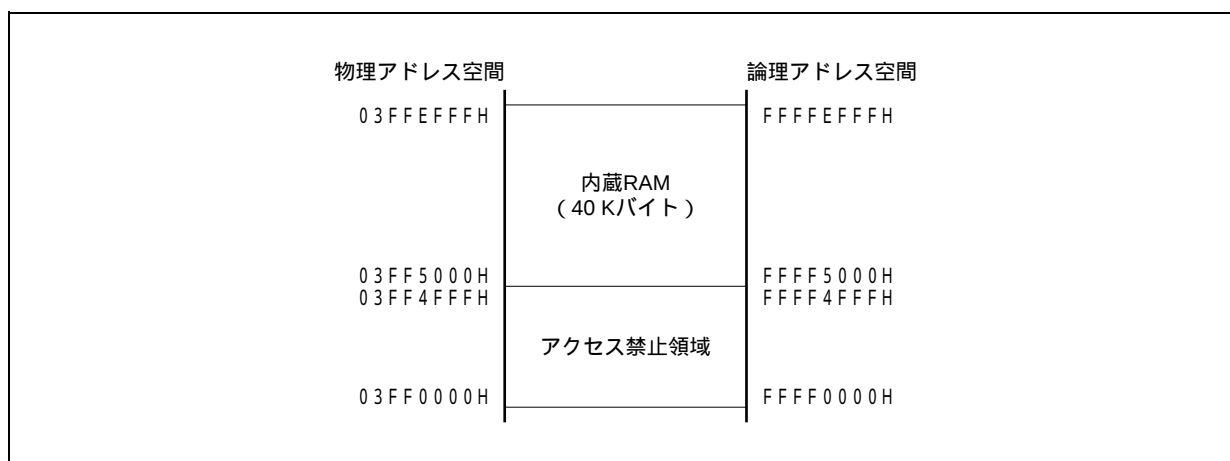
図3 - 8 内蔵RAM領域 (40 Kバイト)
