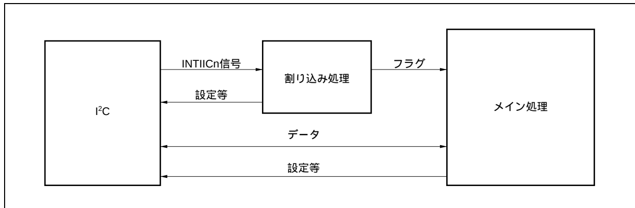
図17 - 20 スレーブ動作時のソフトウェア概要
