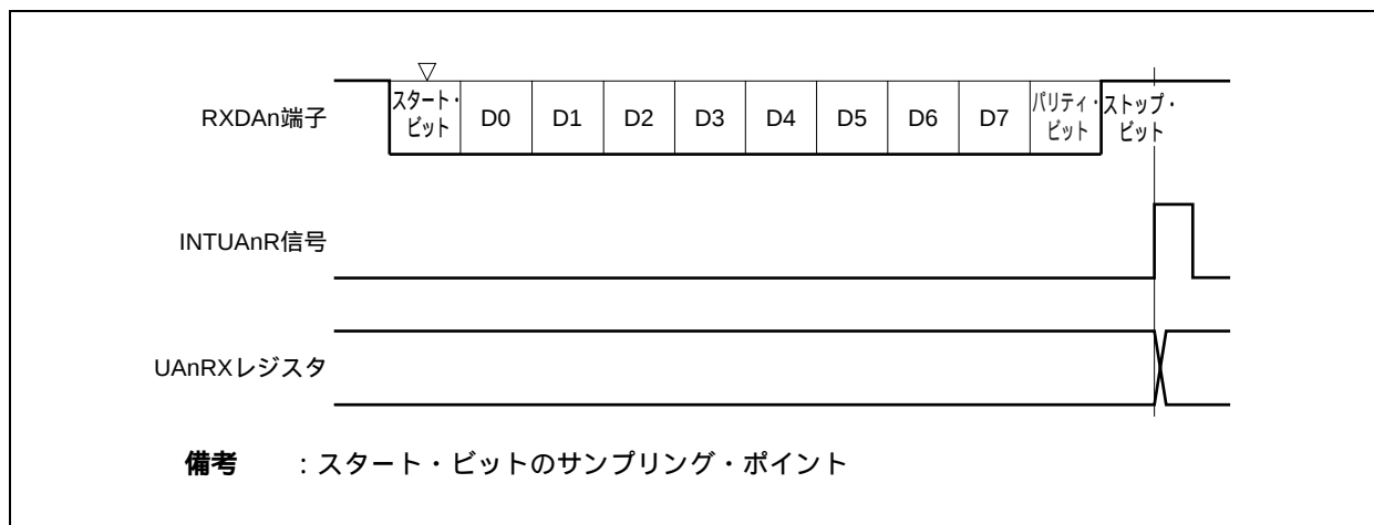
図15 - 13 UART受信
