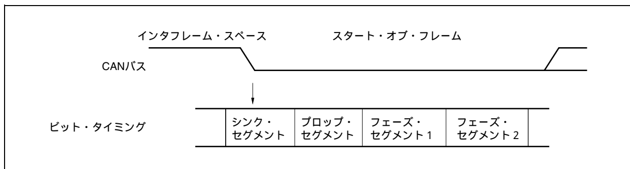
図19 - 20 バス・アイドル中のドミナント・レベル検出によるハードウェア同期
