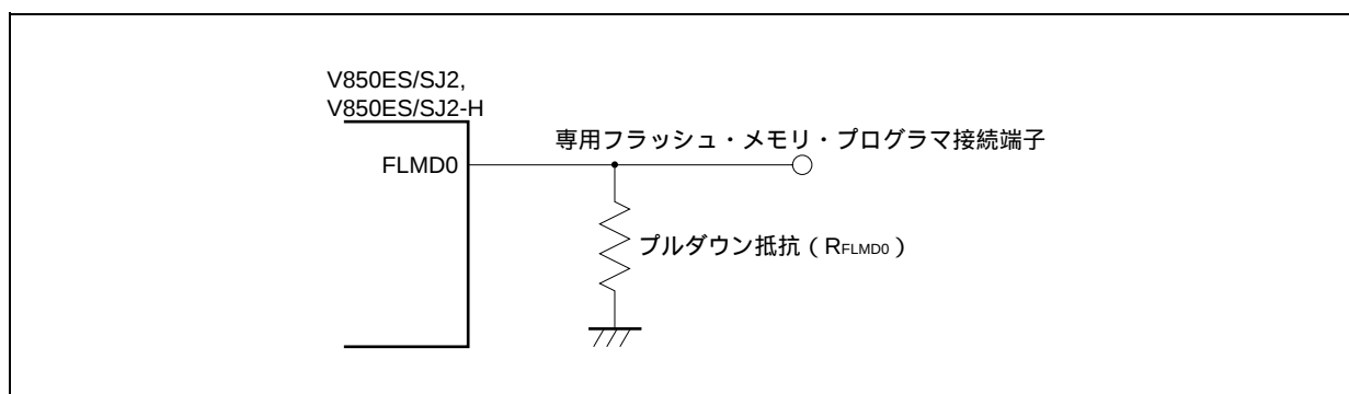
図30 - 10 FLMD0端子の接続例
