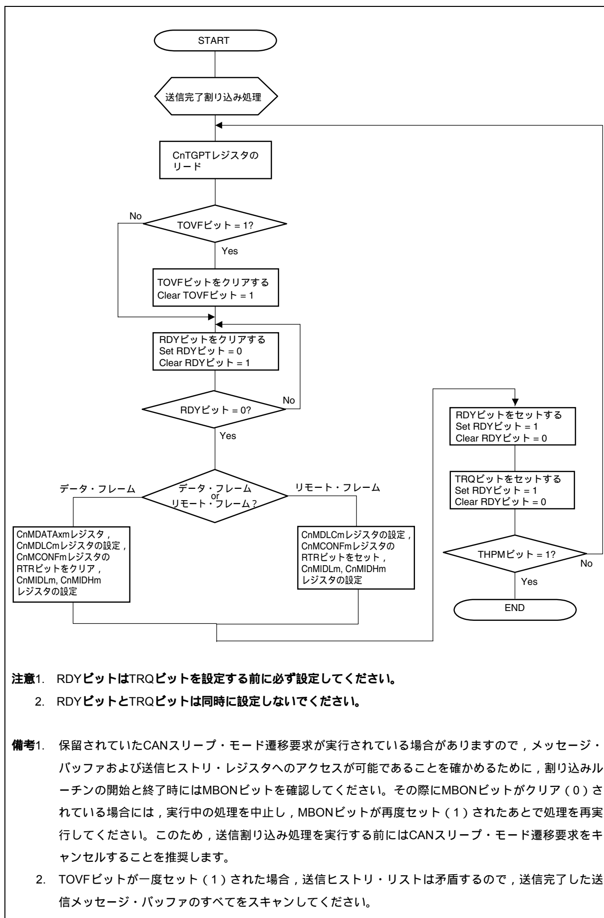
図19 - 44 割り込みによる送信処理 (CnTGPTレジスタを使用する場合)
