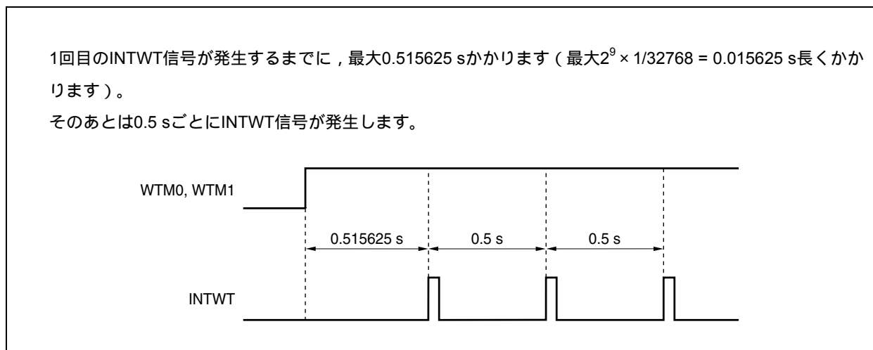
図10 - 3 時計タイマ割り込み要求信号 (INTWT) の発生例 (割り込み周期 = 0.5 sの場合)
