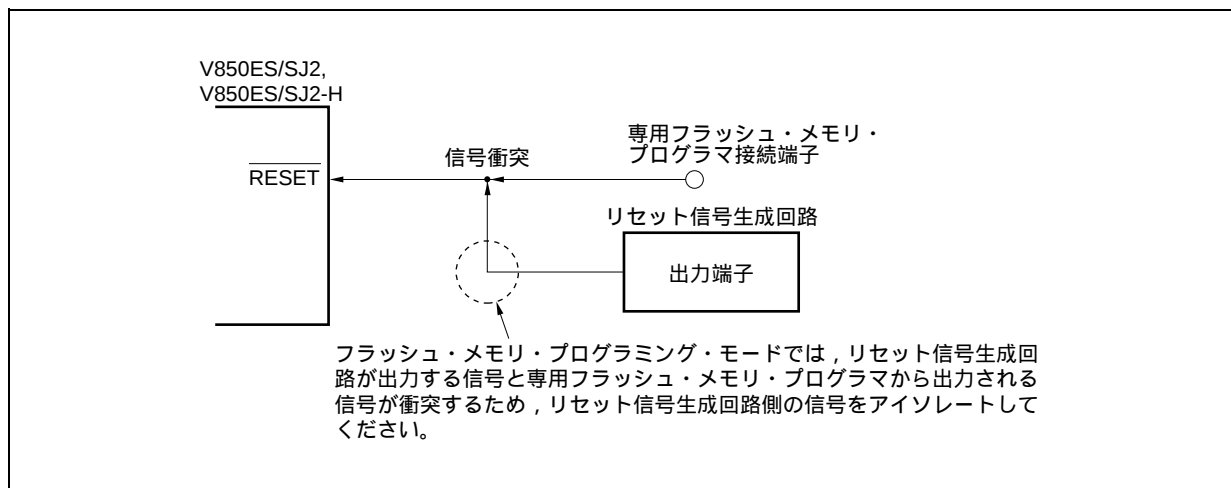
図30 - 14 信号の衝突 (RESET端子)
