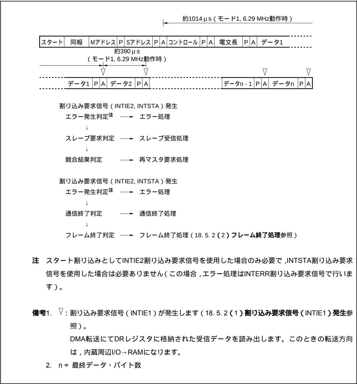
図18 - 27 マスタ受信
