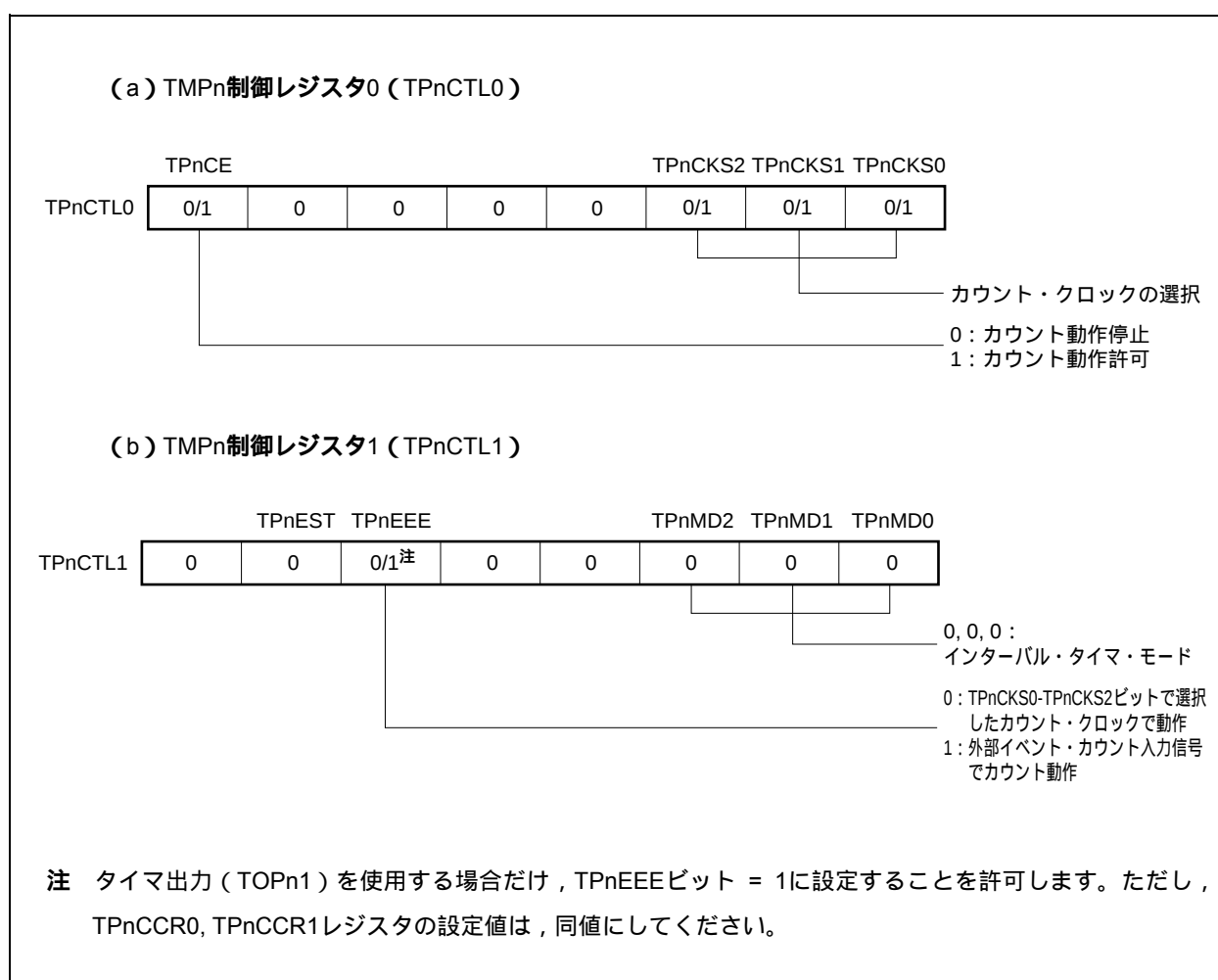
図7-8 インターバル・タイマ・モード動作時のレジスタ設定内容(1/3)
