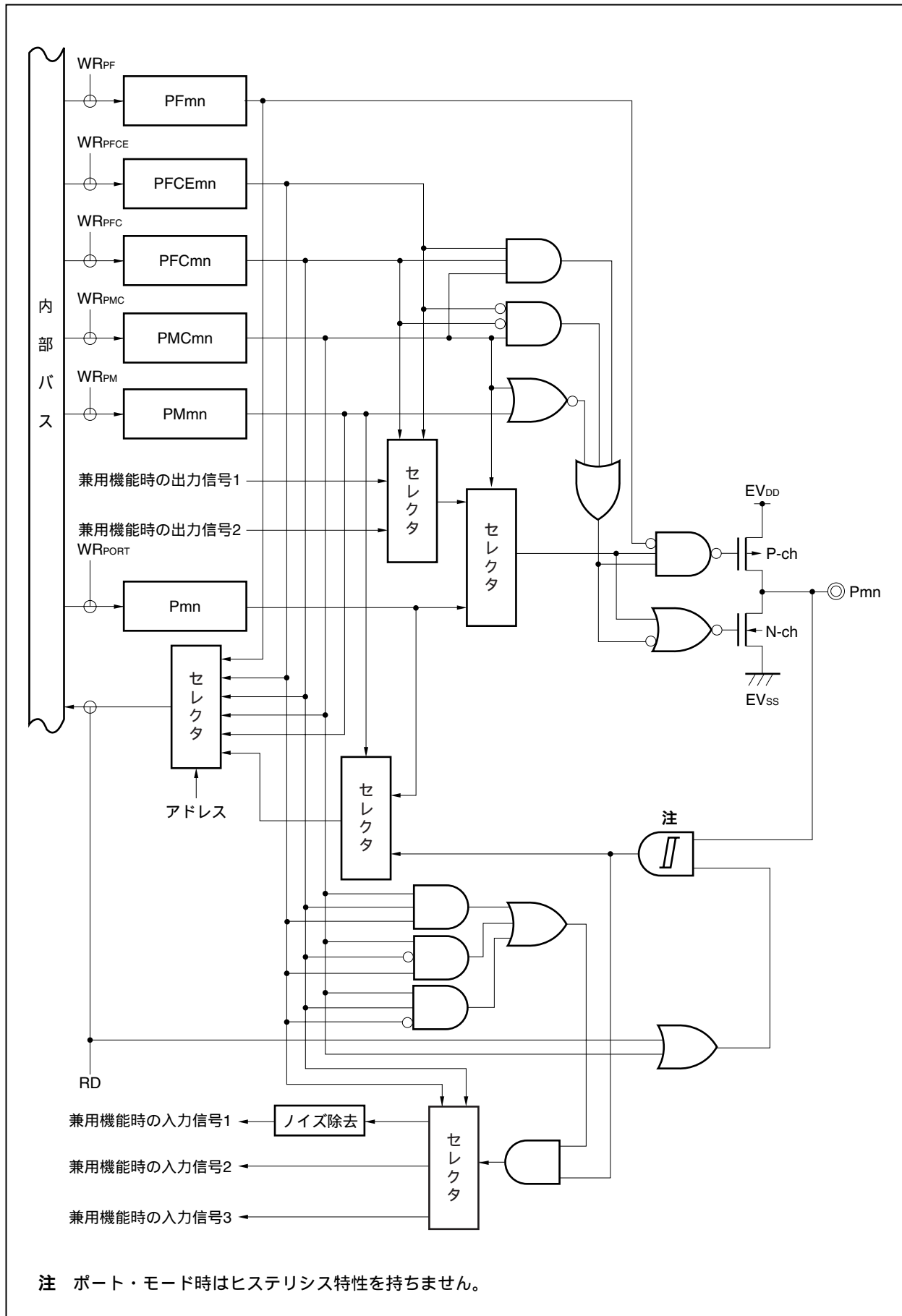
図4 - 35 タイプU - 11のブロック図
