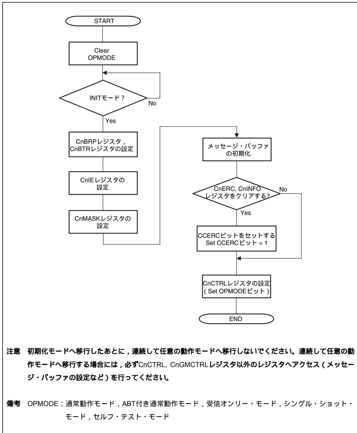
図19 - 37 再初期化
