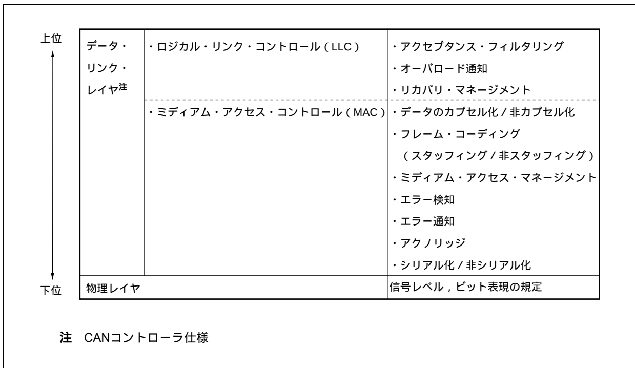
図19 - 2 各レイヤの構成
