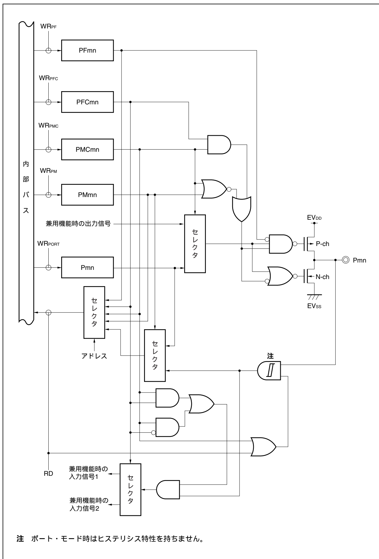
図4 - 18 タイプG - 6のブロック図
