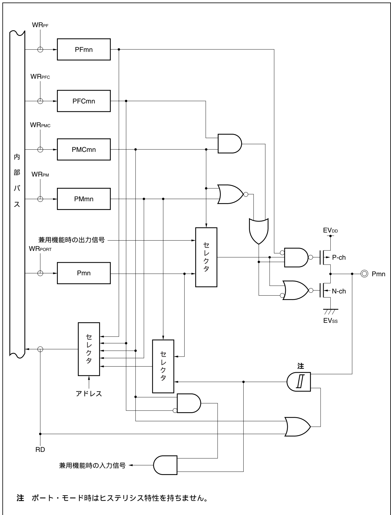
図4 - 13 タイプG - 1のブロック図
