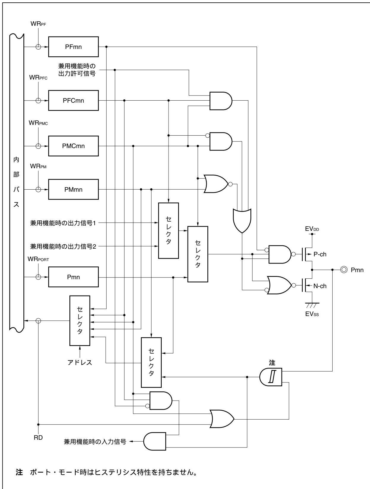
図4 - 17 タイプG - 5のブロック図
