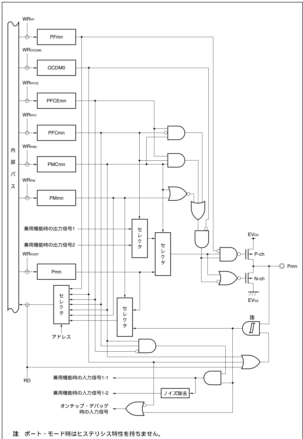
図4 - 30 タイプU - 6のブロック図
