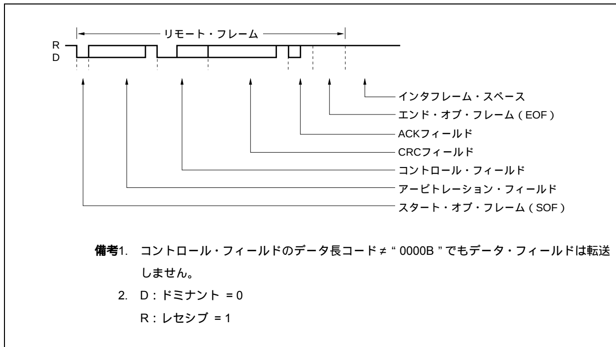
図19-4 リモート・フレーム
