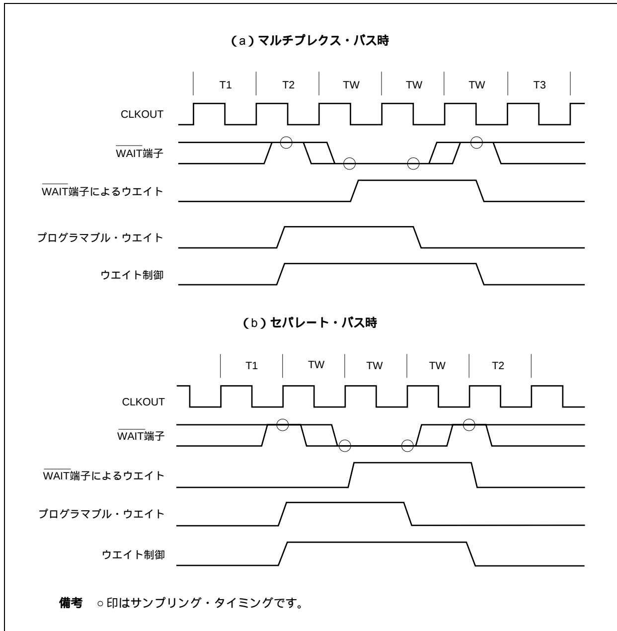
図5-3 ウェイト挿入例
