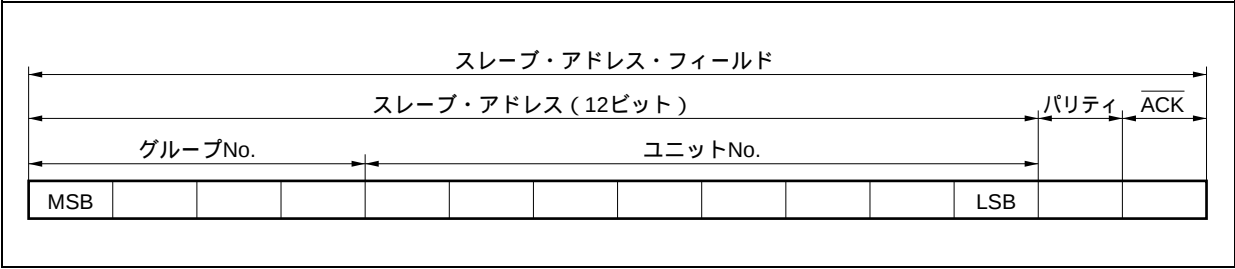
図18 - 3 スレーブ・アドレス・フィールド
