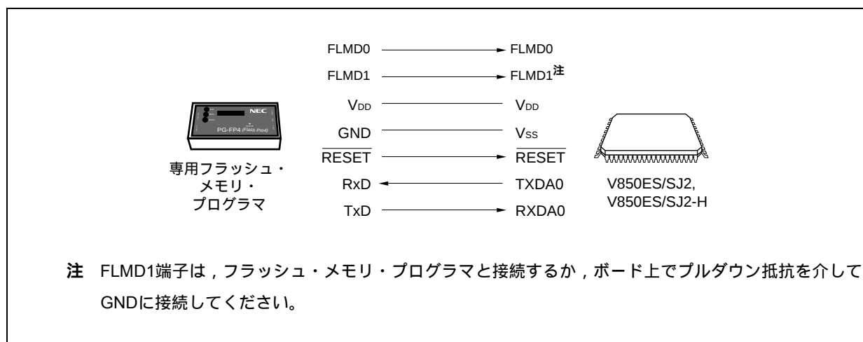
図30 - 3 専用フラッシュ・メモリ・プログラマとの通信 (UARTA0)
