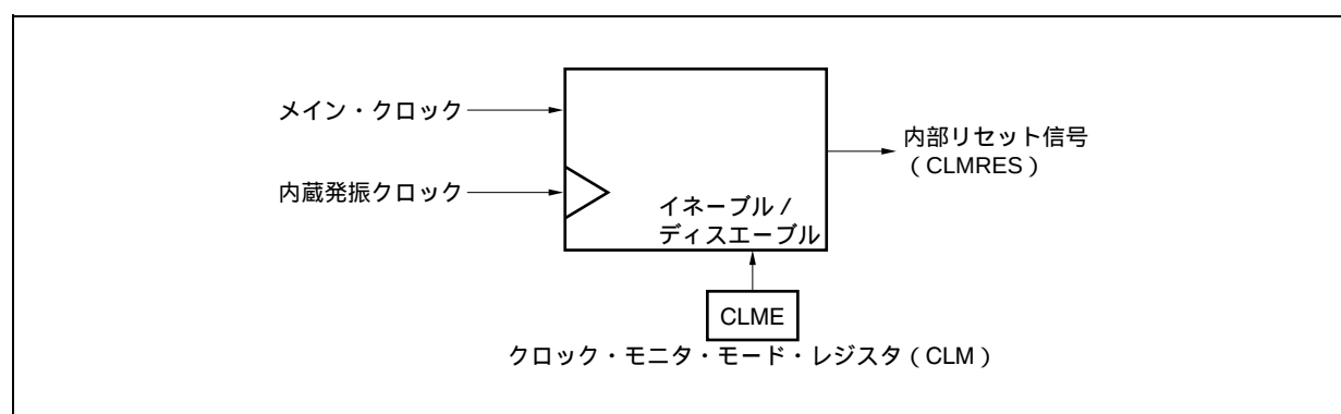
図26 - 1 クロック・モニタによるリセット動作のタイミング
