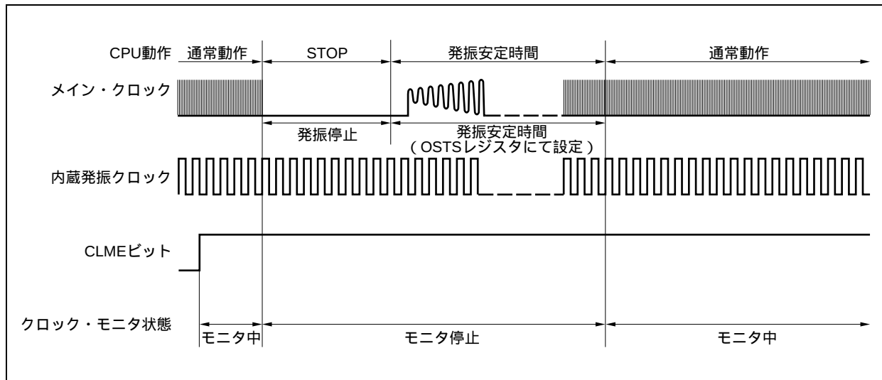
図26 - 4 STOPモード中およびSTOPモード解除後の動作
