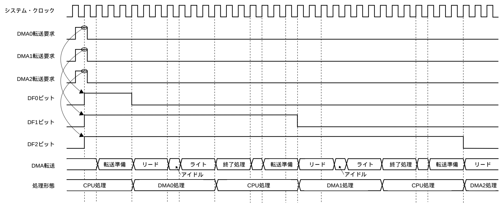
図20 - 1 DMAの優先順位（1）
