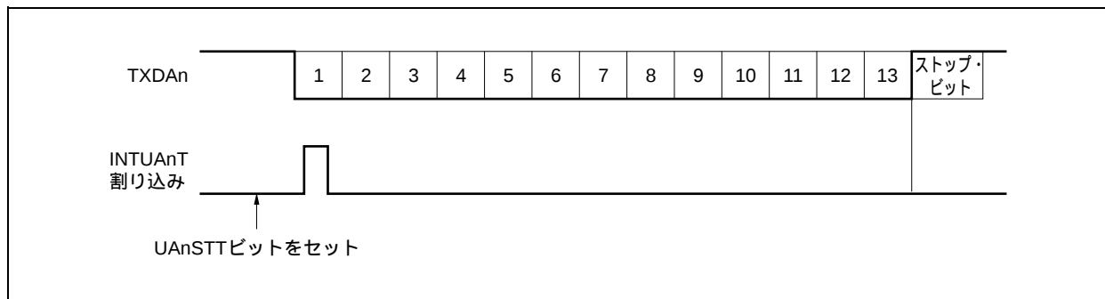
図15 - 8 SBF送信
