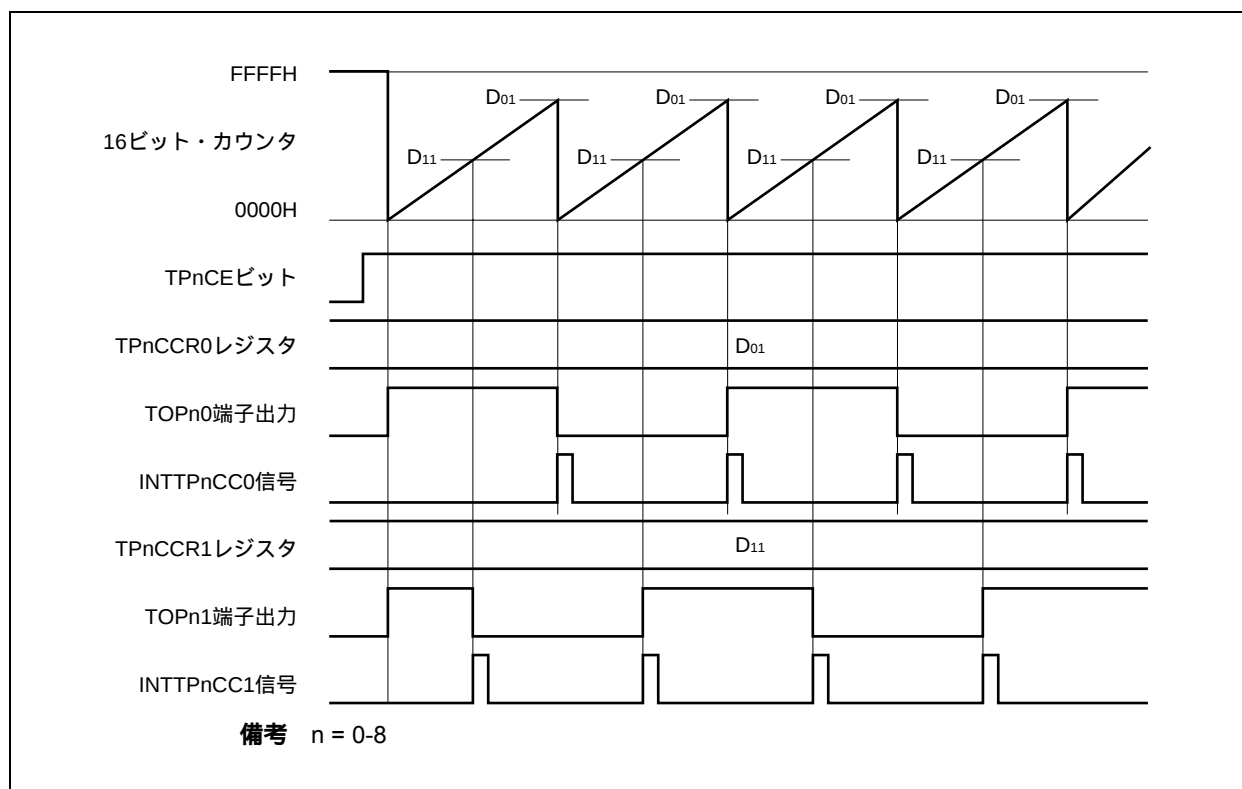
図7 - 11 D 01 D 11 の場合のタイミング図
