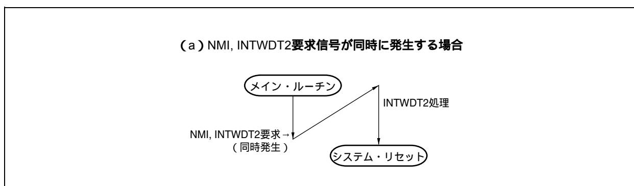
図22 - 1 ノンマスクابل割り込み要求信号の受け付け動作（1/2）
