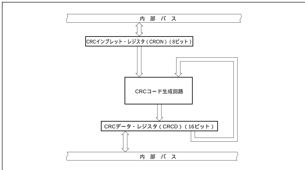
図21 - 1 CRCレジスタのブロック図
