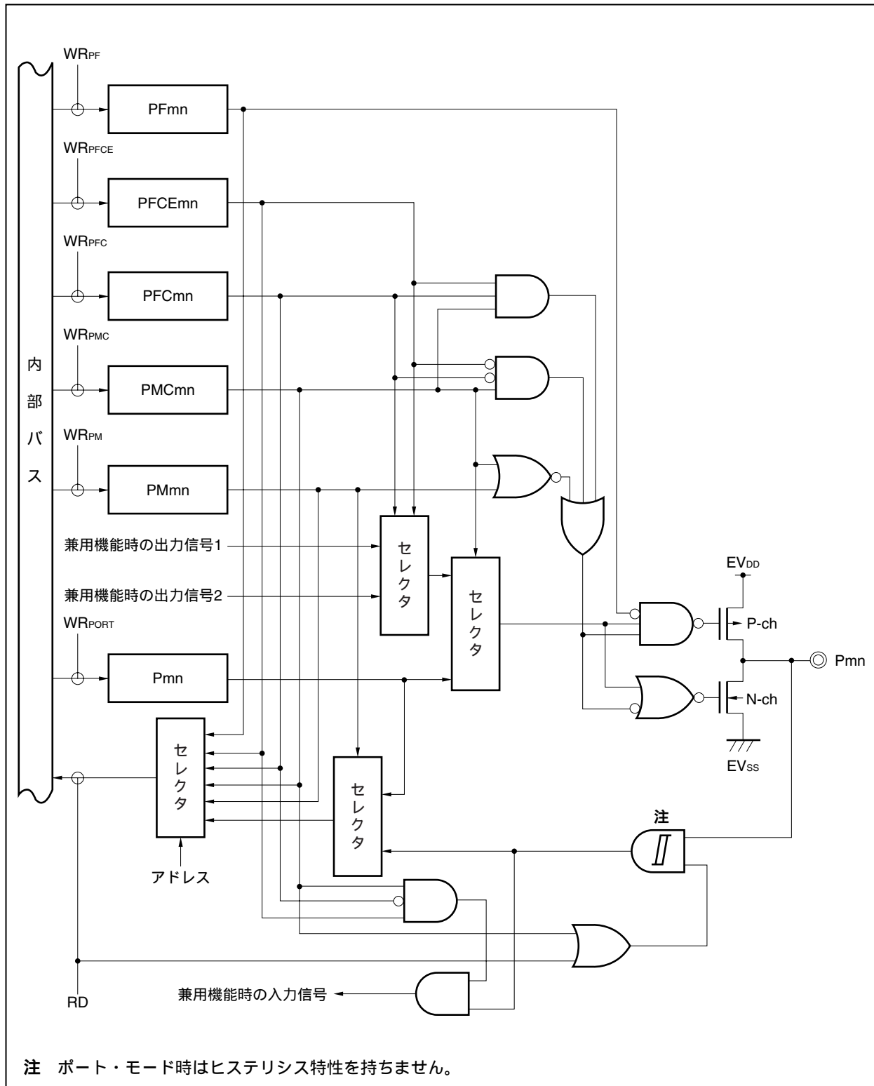
図4 - 37 タイプU - 13のブロック図
