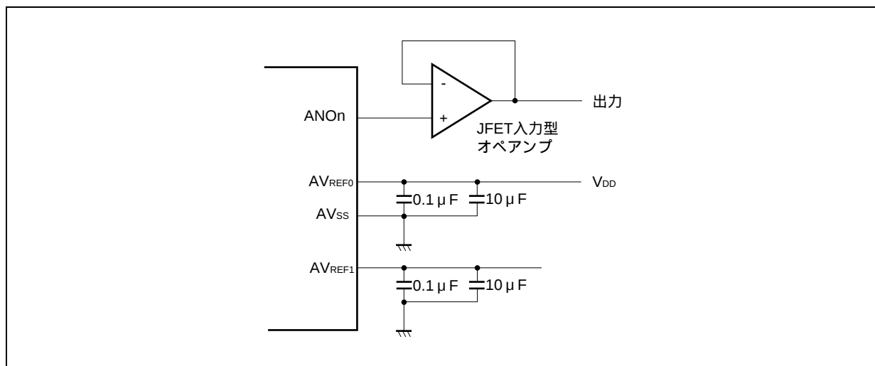
図14 - 2 外部端子の接続例
