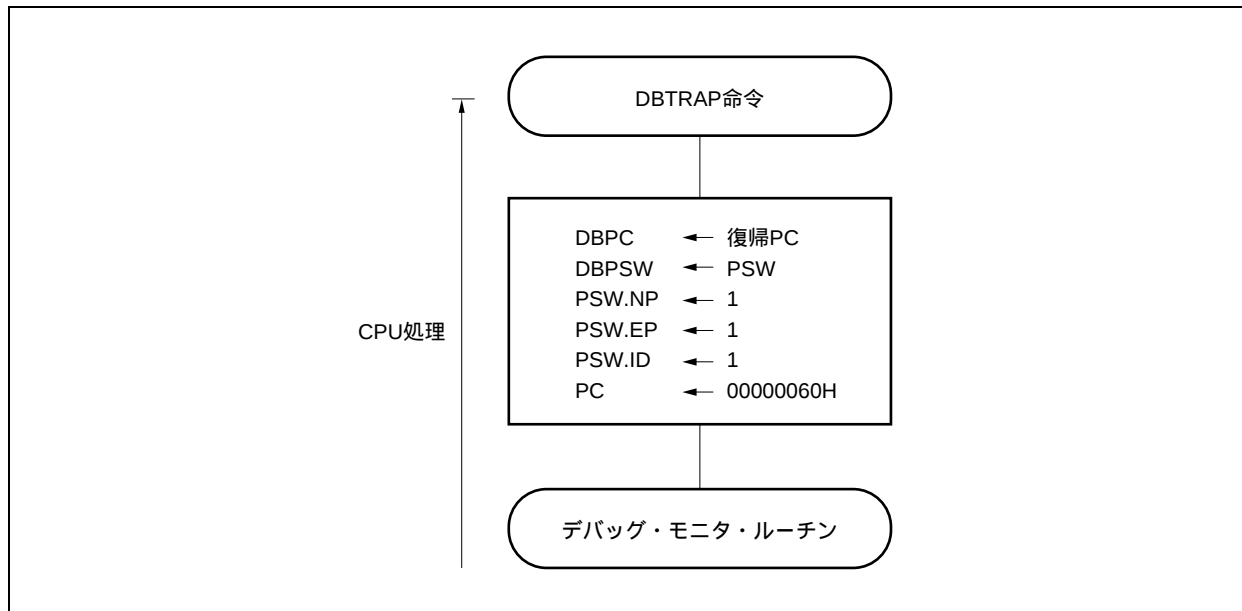
図22 - 13 デバッグ・トラップの処理形態
