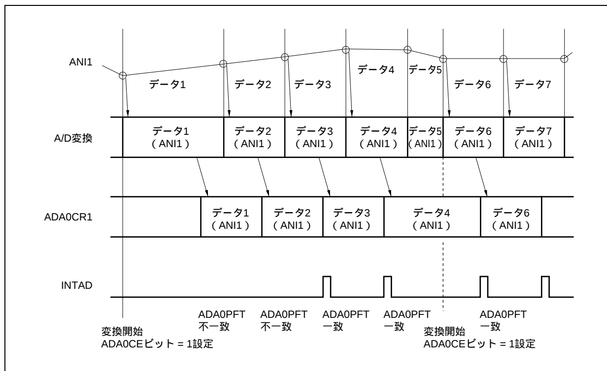
図13 - 8 連続セレクト・モード動作タイミング例 (パワー・フェイル比較時 : ADA0Sレジスタ = 01H)
