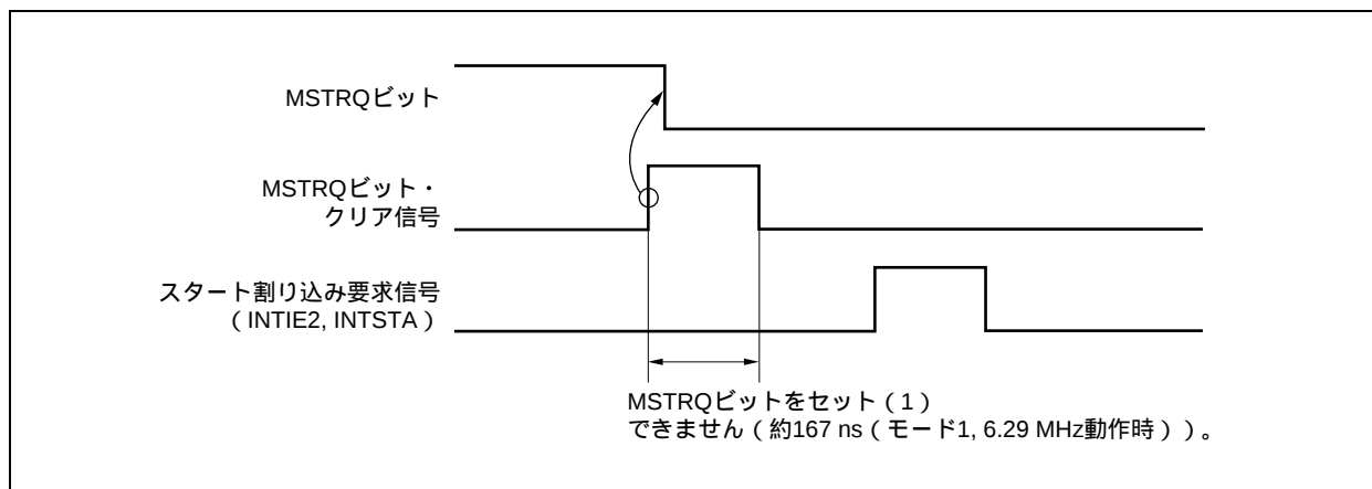
図18 - 11 MSTRQビットをセットできないタイミング
