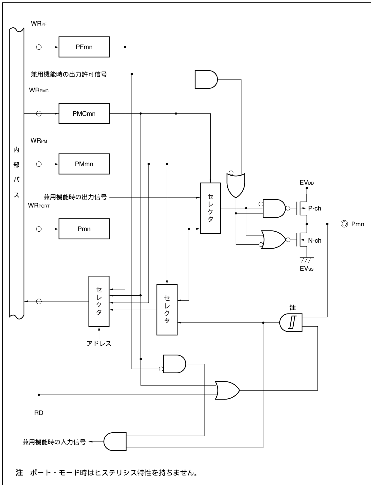
図4 - 12 タイプE - 3のブロック図
