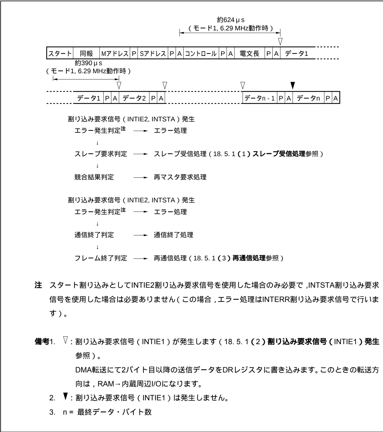
図18 - 26 マスタ送信
