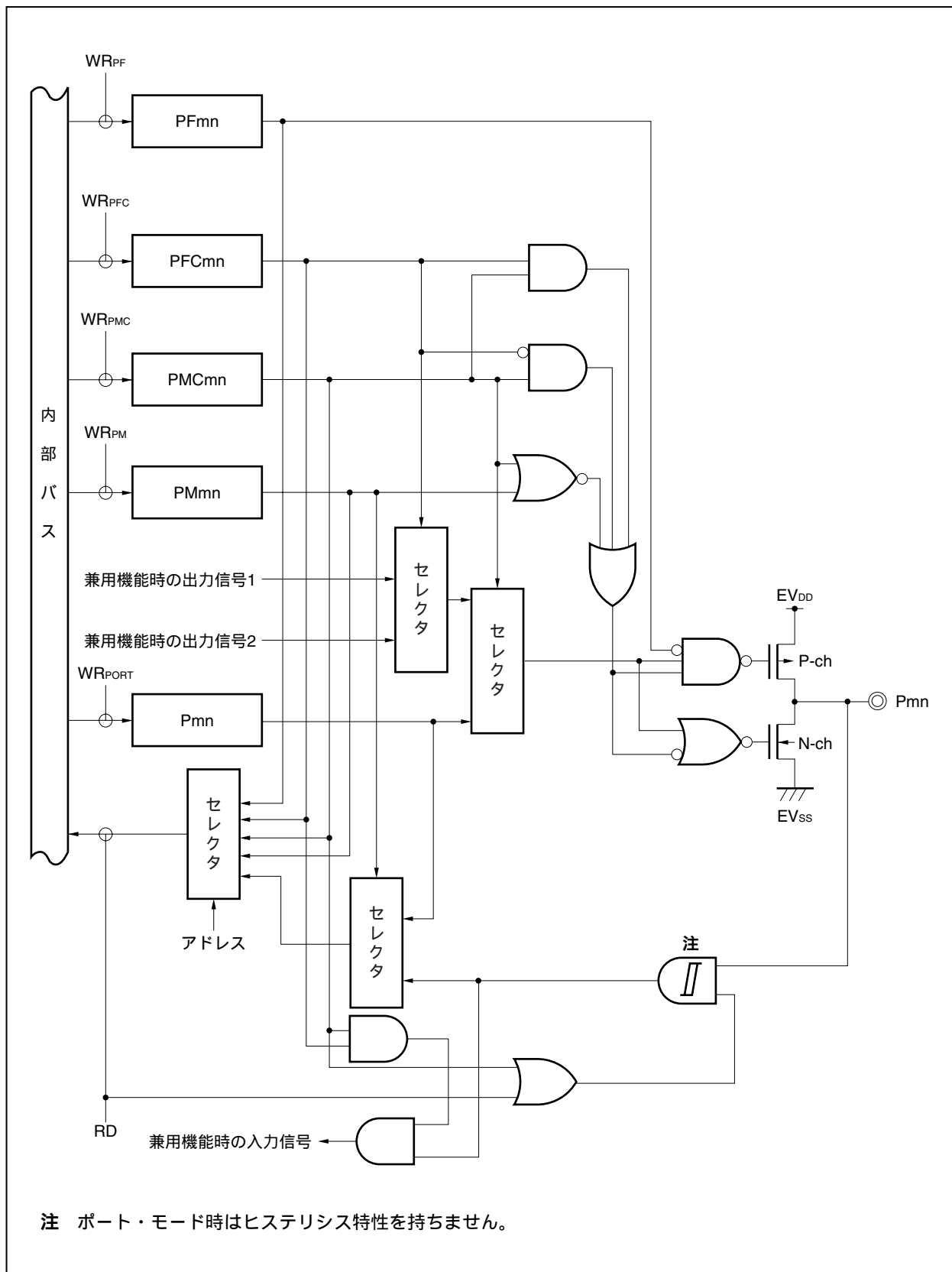
図4 - 19 タイプG - 12のブロック図
