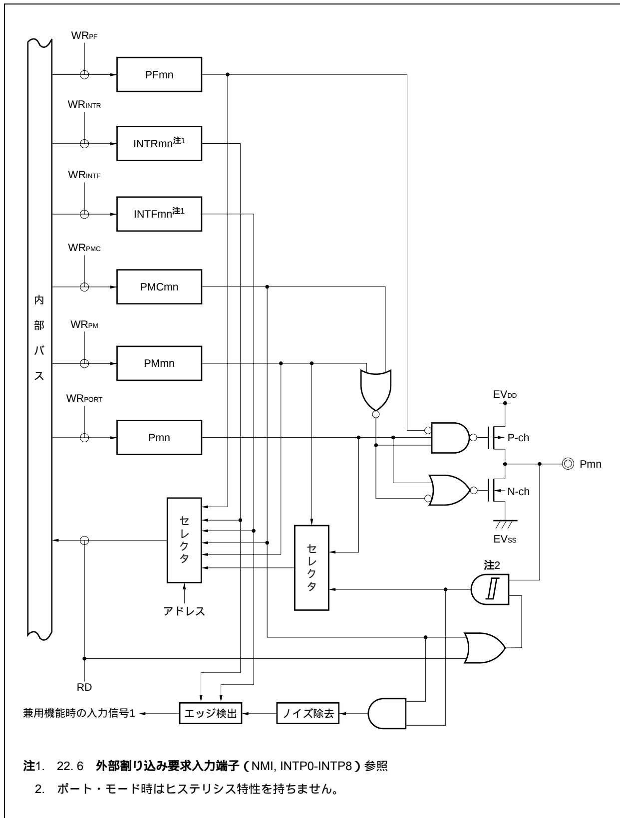
図4 - 20 タイプL - 1のブロック図
