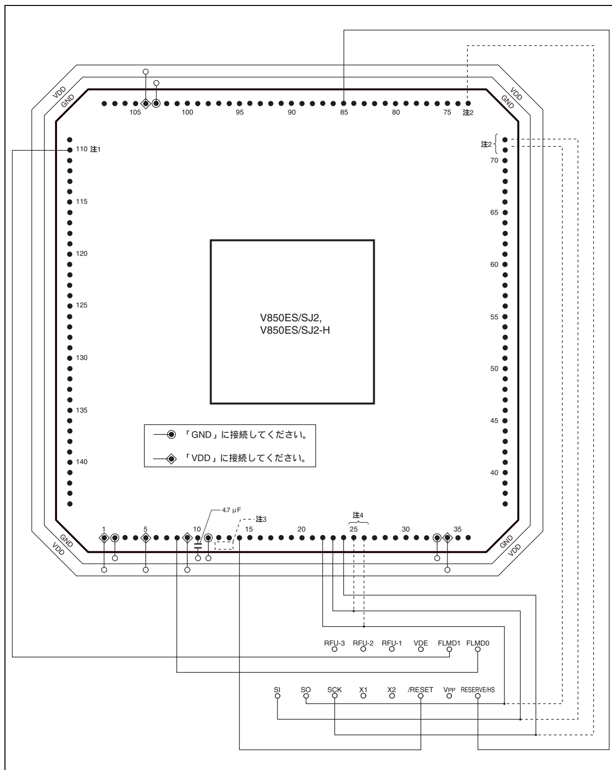
図30 - 6 V850ES/SJ2, V850ES/SJ2-Hフラッシュ書き込み用アダプタ (FA-144GJ-UEN-A) の配線例 (CSIB0 + HSモード時) (1/2)
