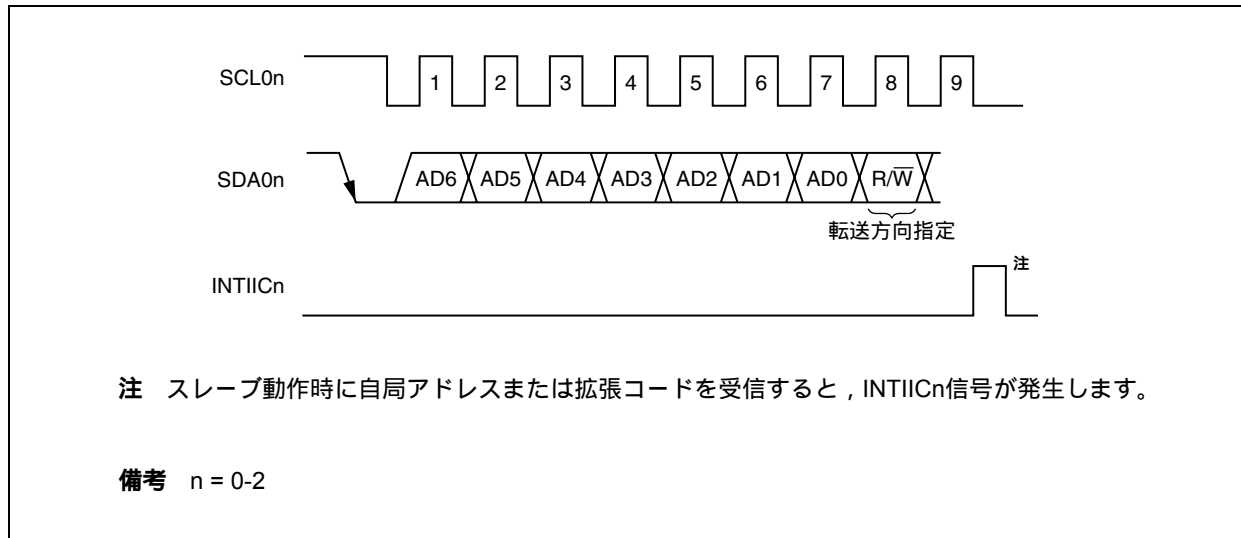
図17 - 10 転送方向指定
