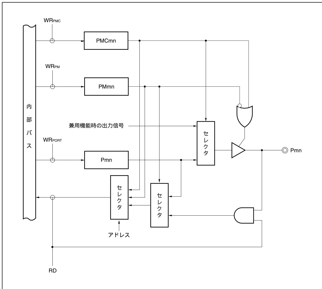
図4 - 8 タイプD - 2のブロック図
