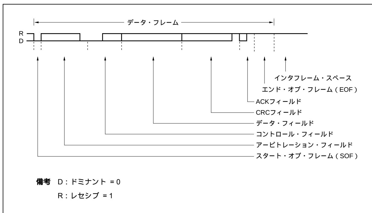
図19 - 3 データ・フレーム
