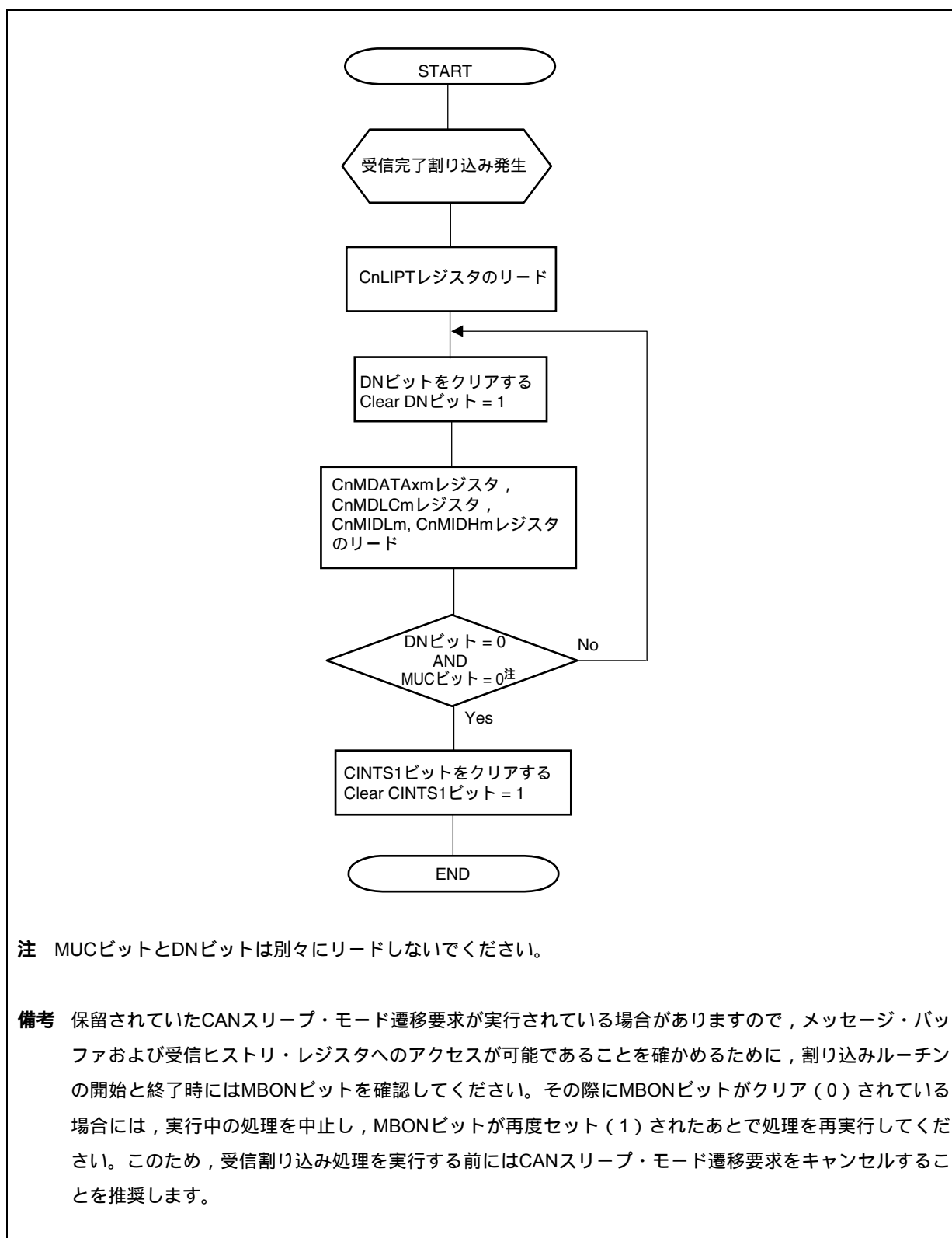
図19 - 49 割り込みによる受信処理 (CnLIPTレジスタを使用する場合)
