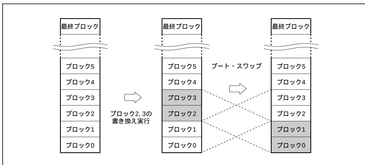
図30 - 16 全メモリ領域の書き換え (ブート・スワップ対応)
