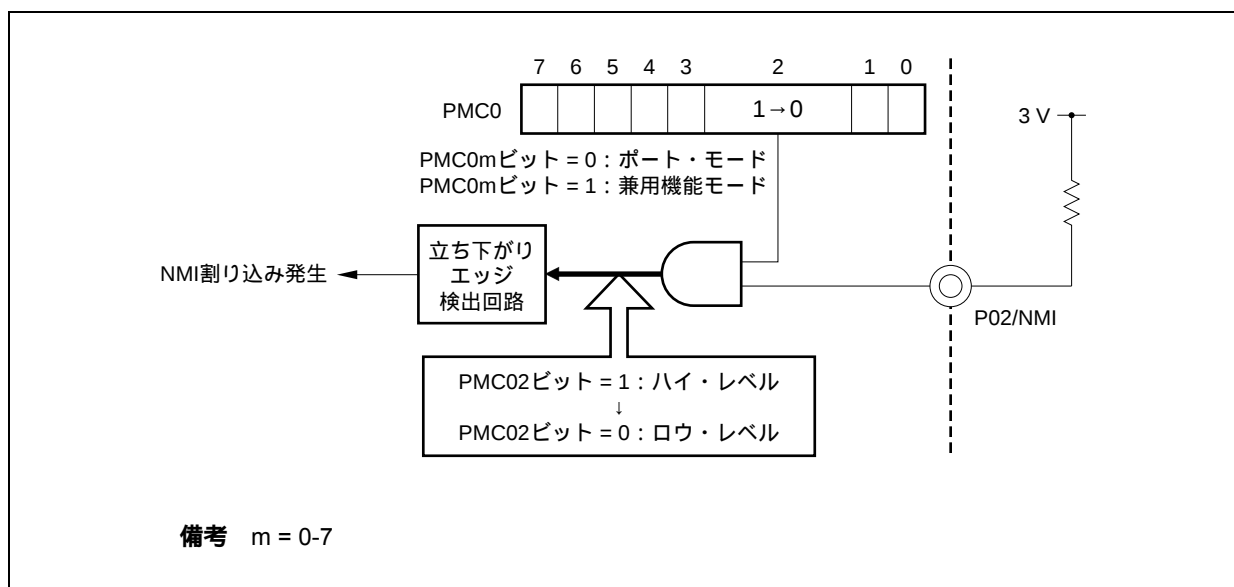
図4 - 42 NMI端子からP02端子への切り替え（悪い例）
