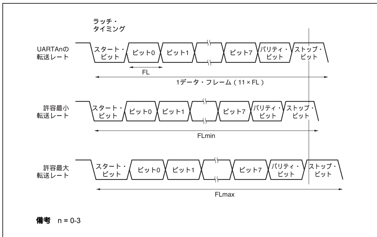
図15 - 17 受信時の許容ボー・レート範囲
