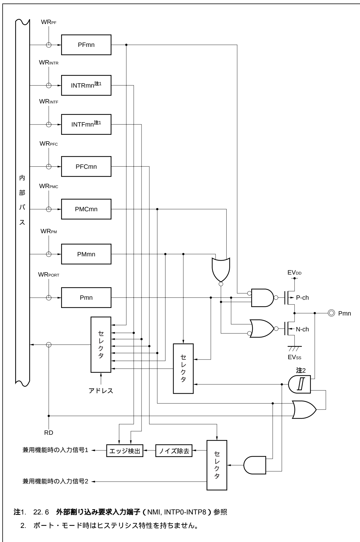
図4 - 22 タイプN - 1のブロック図
