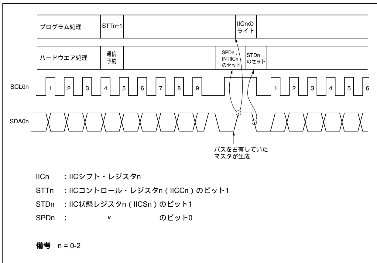
図17 - 15 通信予約のタイミング
