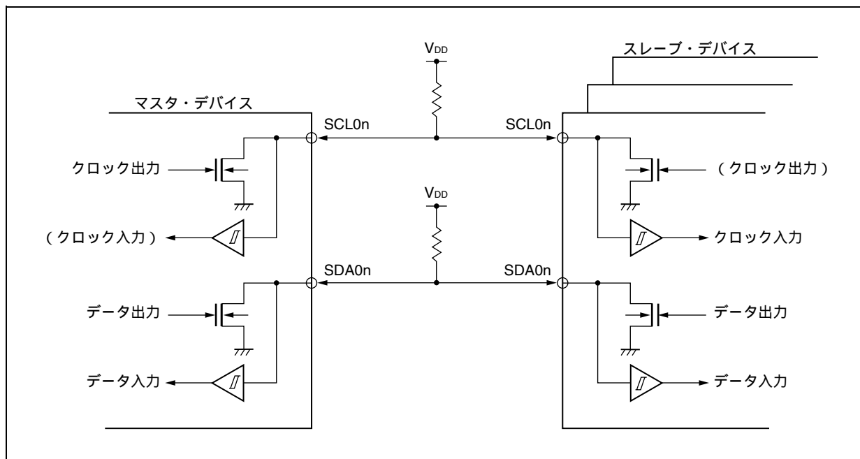
図17 - 6 端子構成図
