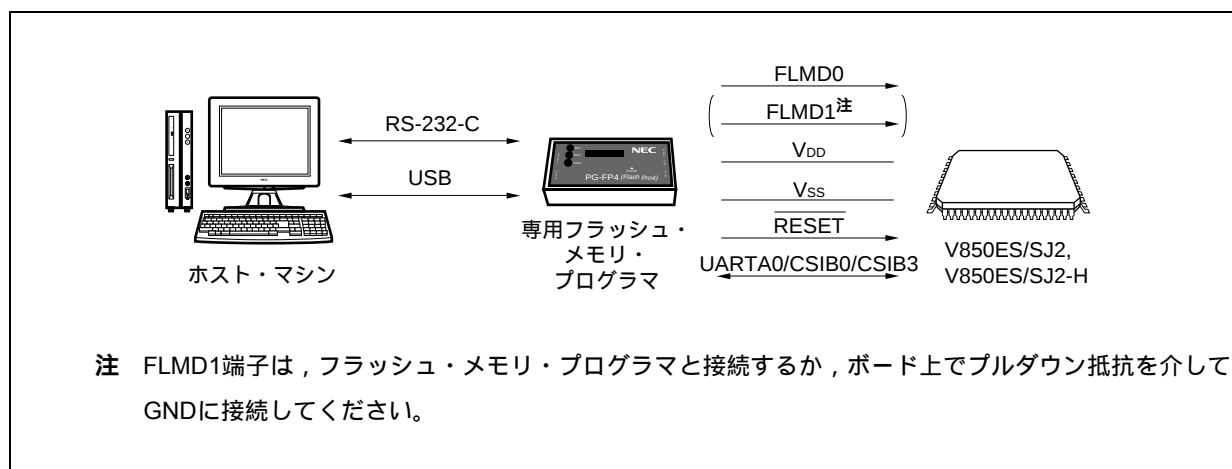
図30 - 2 フラッシュ・メモリにプログラムを書き込むための環境
