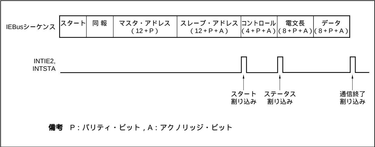
図18 - 19 ロック状態中のINTIE2, INTSTA割り込み要求信号発生タイミング（ の場合）
