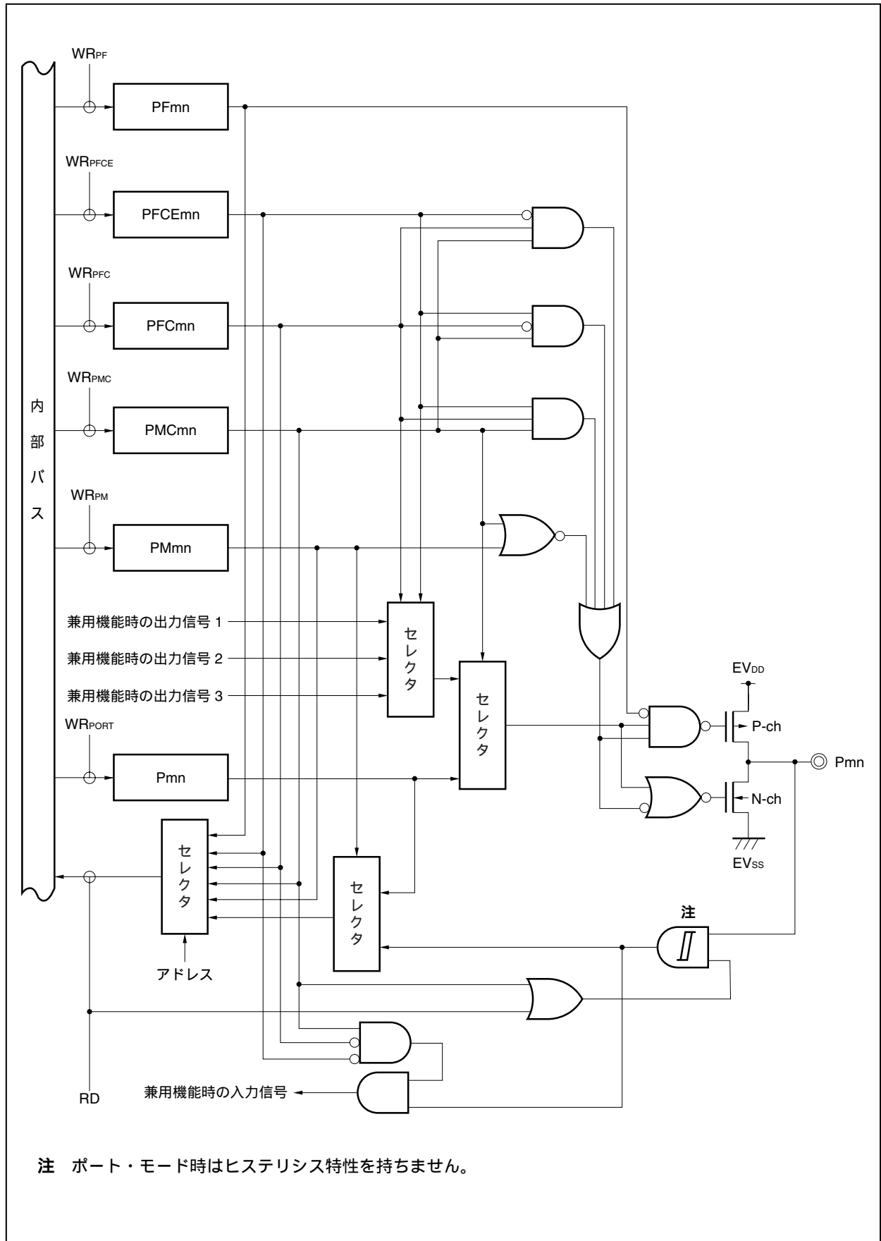
図4 - 26 タイプU - 2のブロック図
