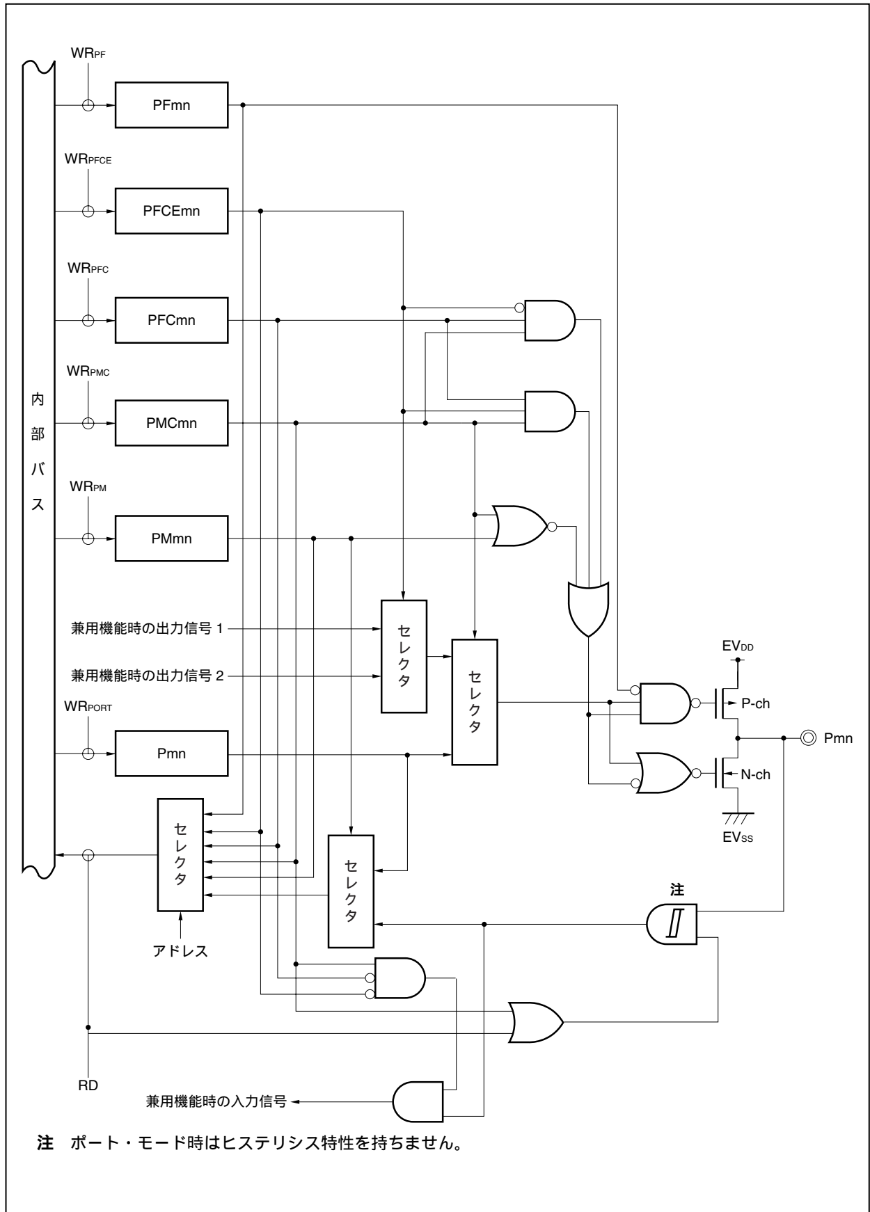
図4 - 28 タイプU - 4のブロック図
