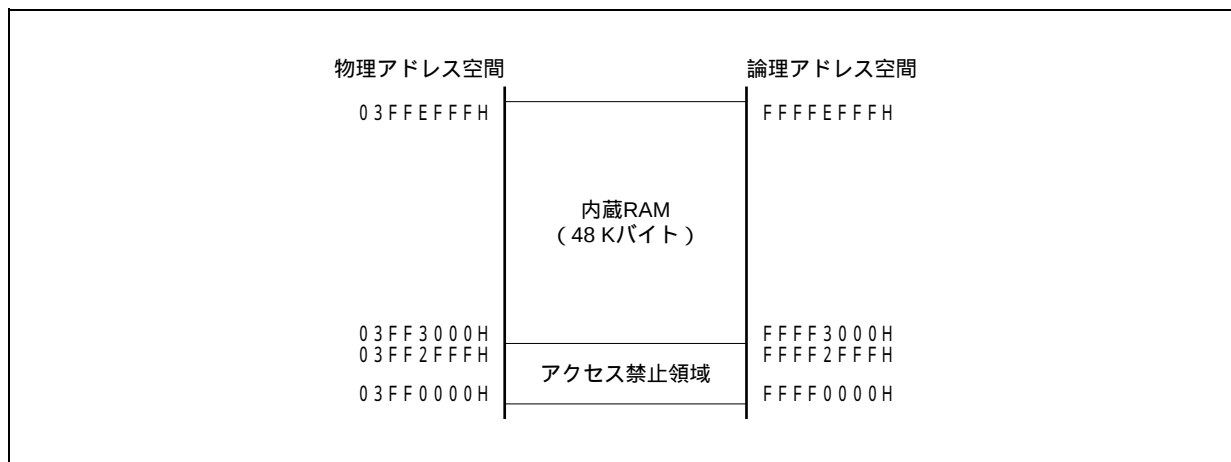
図3 - 9 内蔵RAM領域 (48 Kバイト)
