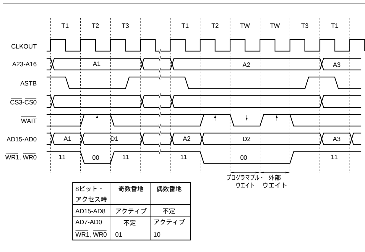
図5-7 マルチプレクス・バス・ライト・タイミング (バス・サイズ: 8ビット)
