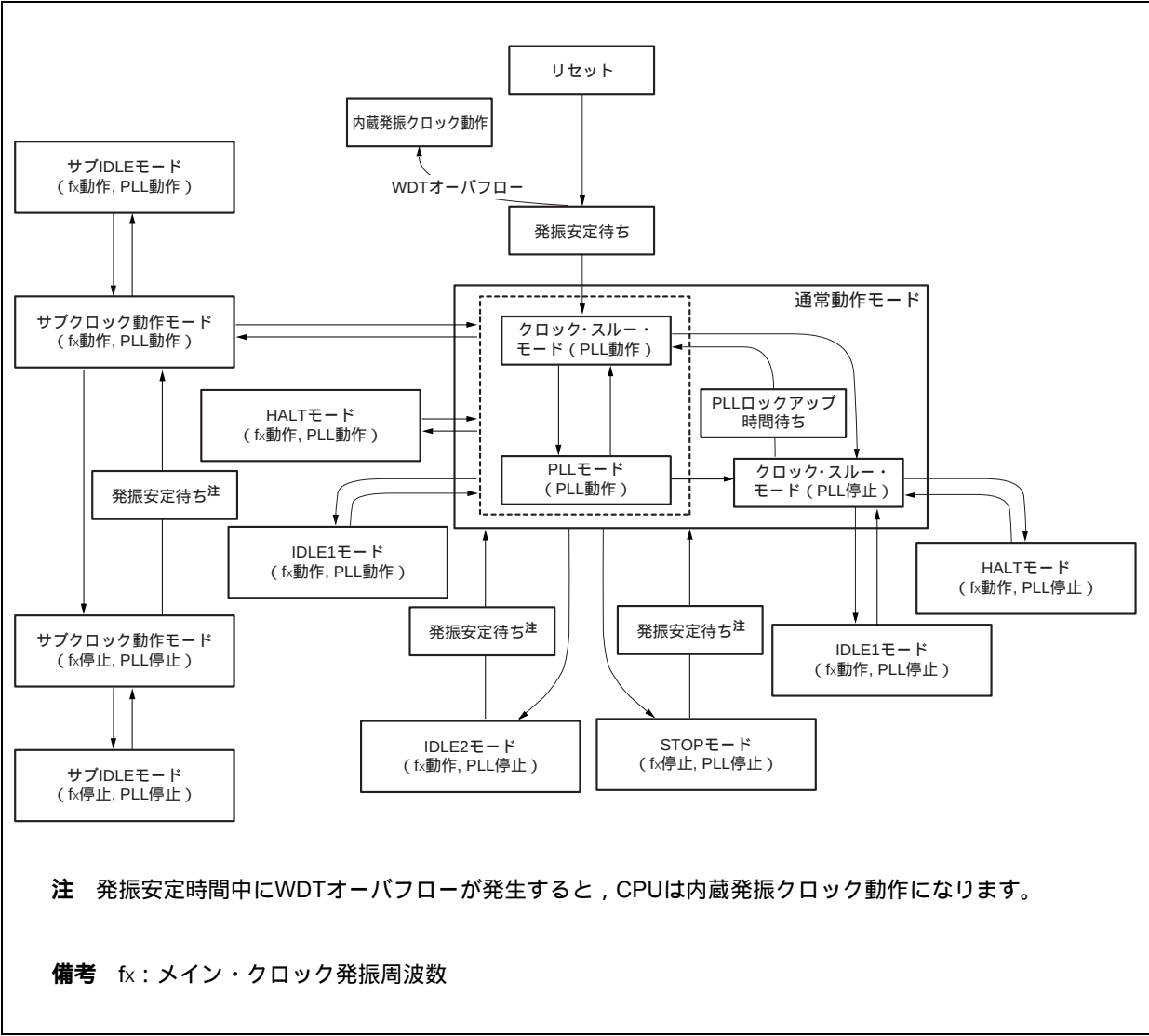
図24 - 1 状態遷移図
