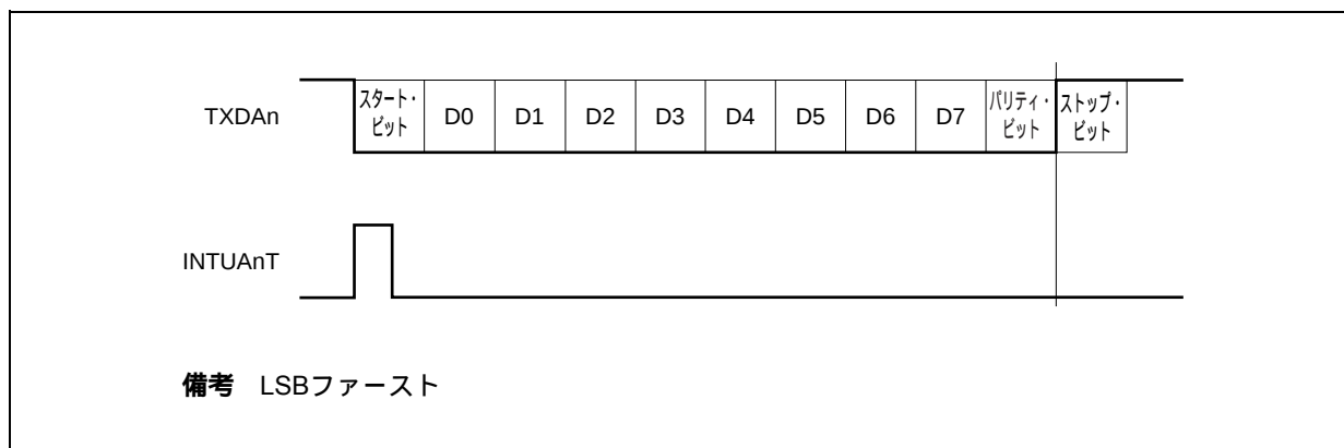
図15 - 10 UART送信
