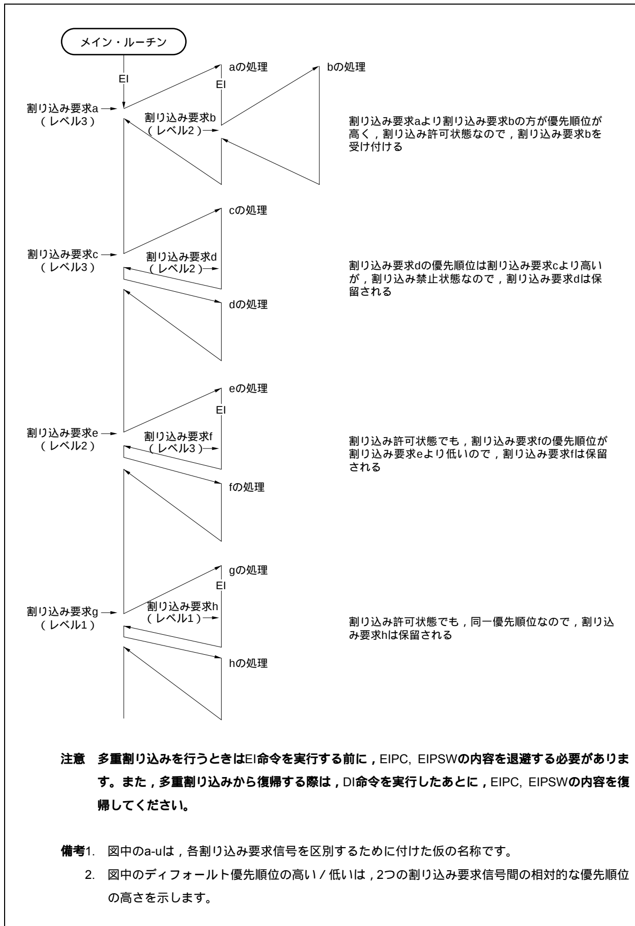
図22 - 7 割り込み処理中にほかの割り込み要求信号が発生した場合の処理例 (1/2)
