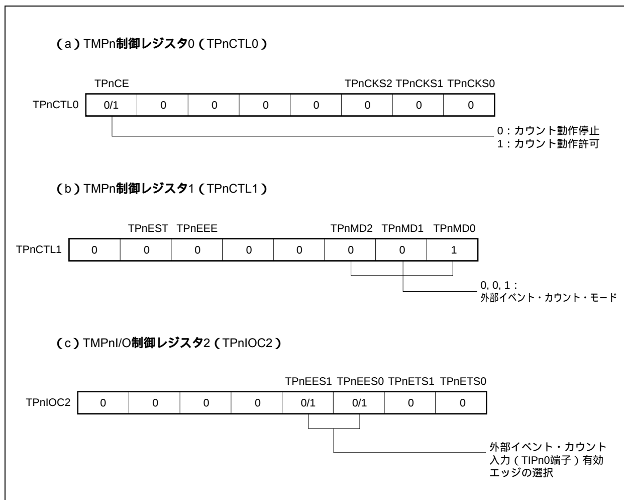
図7 - 15 外部イベント・カウンタ・モード動作時のレジスタ設定内容（1/2）
