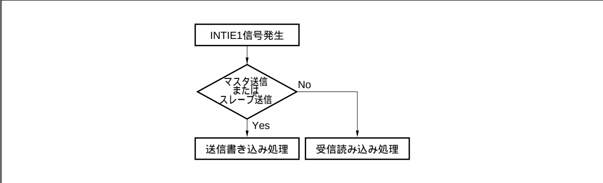
図18 - 24 INTIE1信号の割り込み判定例 (INTIE1, INTIE2信号使用時)
