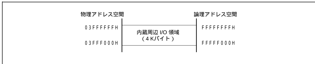
図3 - 10 内蔵周辺I/O領域
