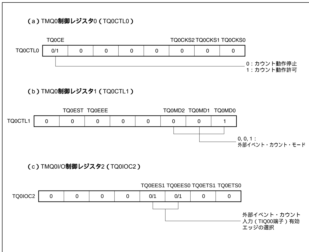
図8 - 15 外部イベント・カウンタ・モード動作時のレジスタ設定内容(1/2)
