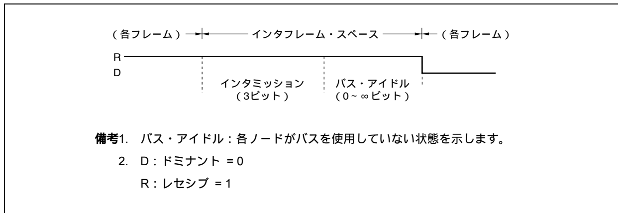
図19 - 13 インタフレーム・スペース（エラー・アクティブ状態のノードの場合）
