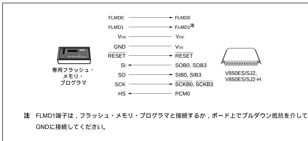
図30 - 5 専用フラッシュ・メモリ・プログラマとの通信 (CSIB0 + HS, CSIB3 + HS)
