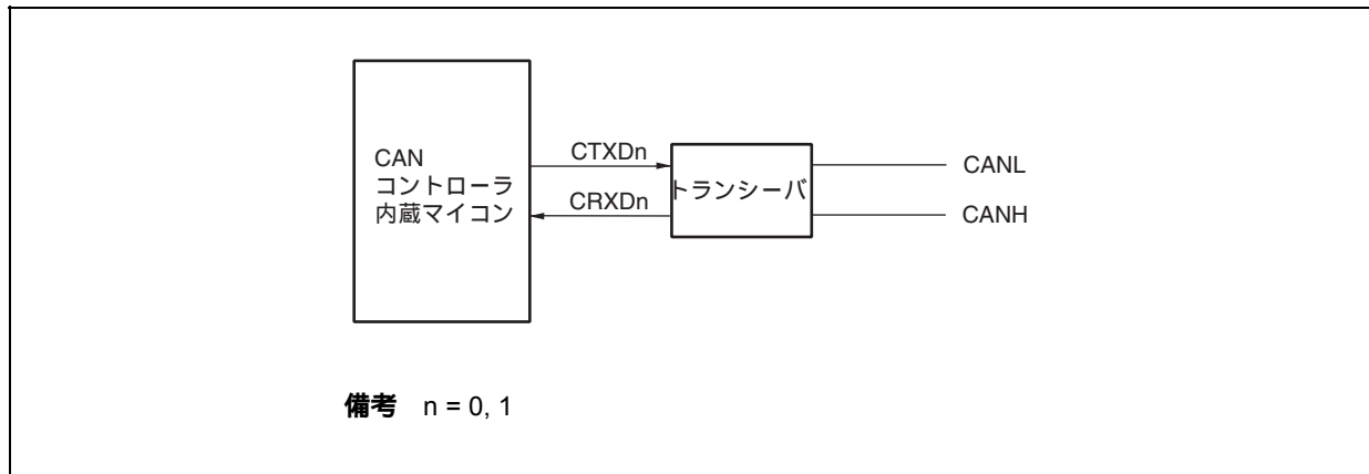
図19 - 22 CANバスへの接続
