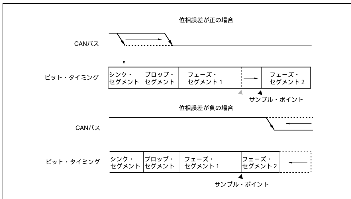
図19 - 21 再同期
