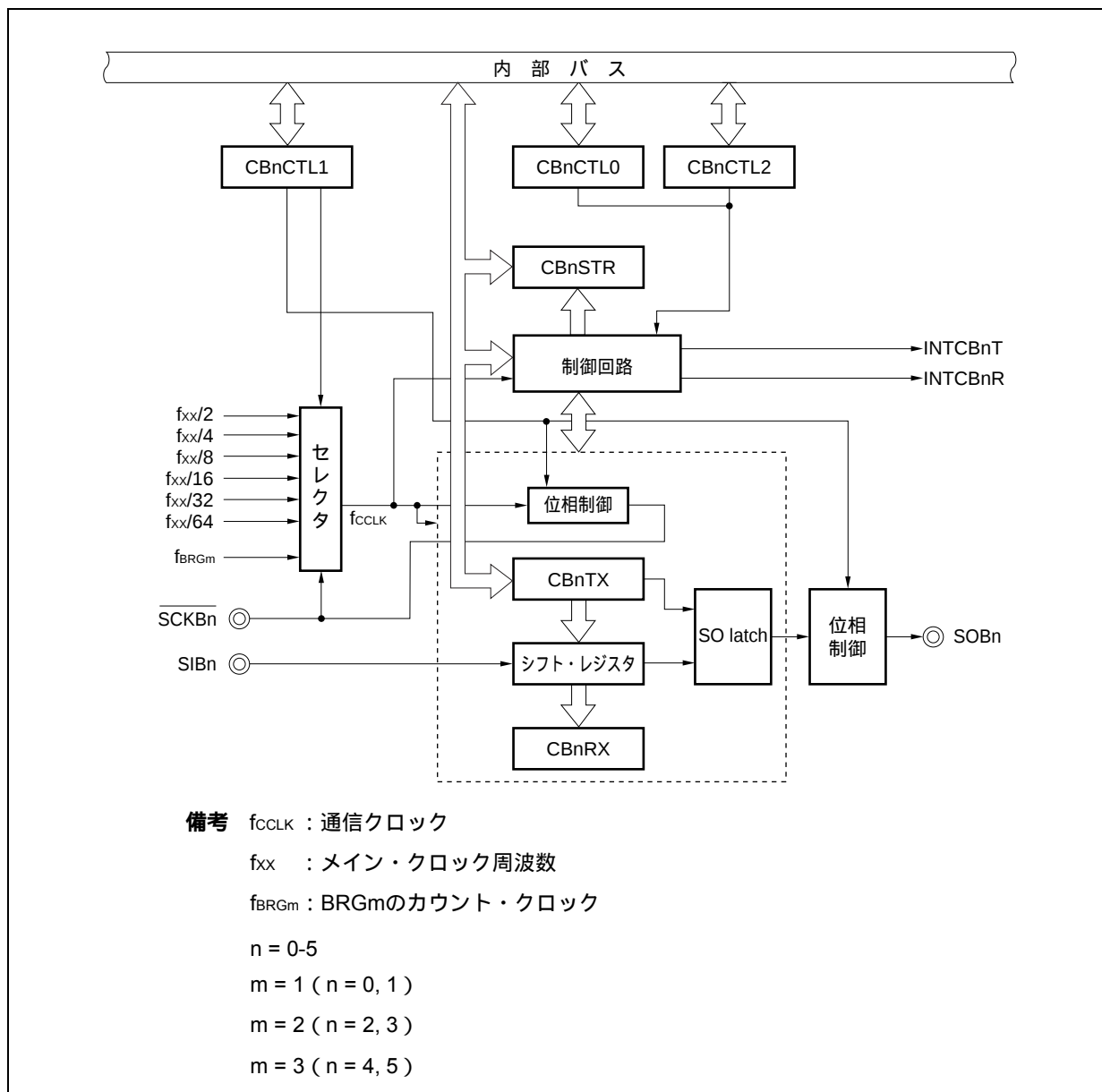
図16 - 3 CSIBnのブロック図
