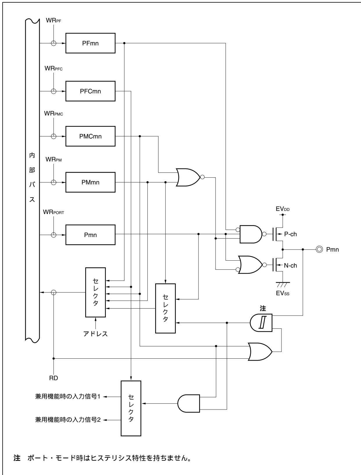
図4 - 16 タイプG - 4のブロック図
