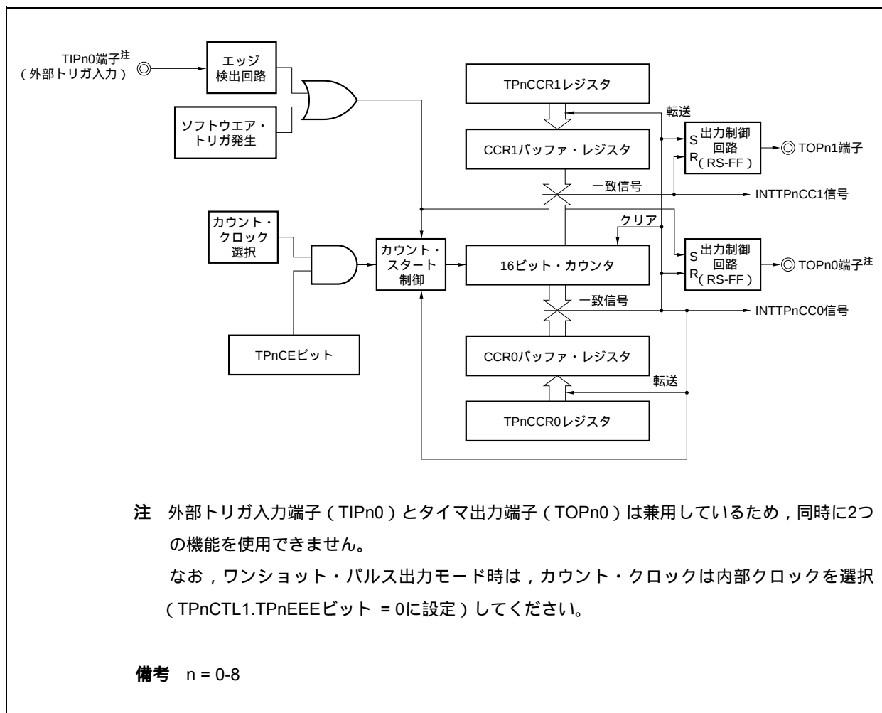
図7-24 ワンショット・パルス出力モードの構成図
