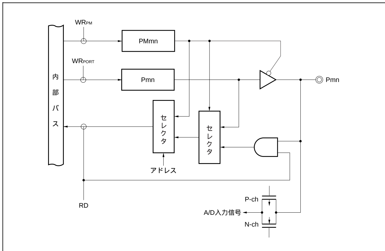
図4 - 4 タイプA - 2のブロック図
