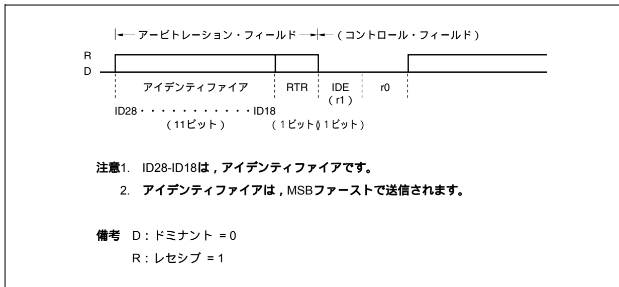
図19 - 6 アービトレーション・フィールド（標準フォーマット・モード時）
