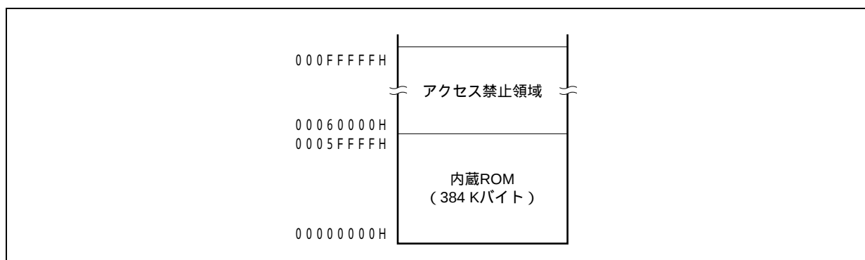
図3 - 4 内蔵ROM領域 (384 Kバイト)
