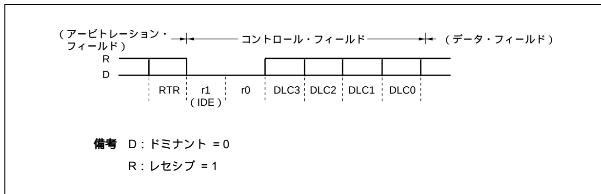
図19 - 8 コントロール・フィールド
