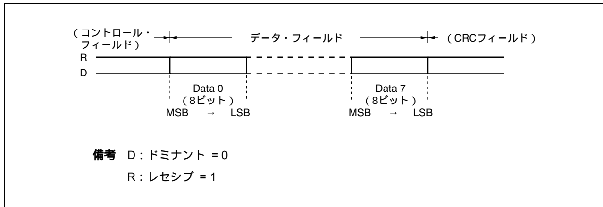
図19 - 9 データ・フィールド
