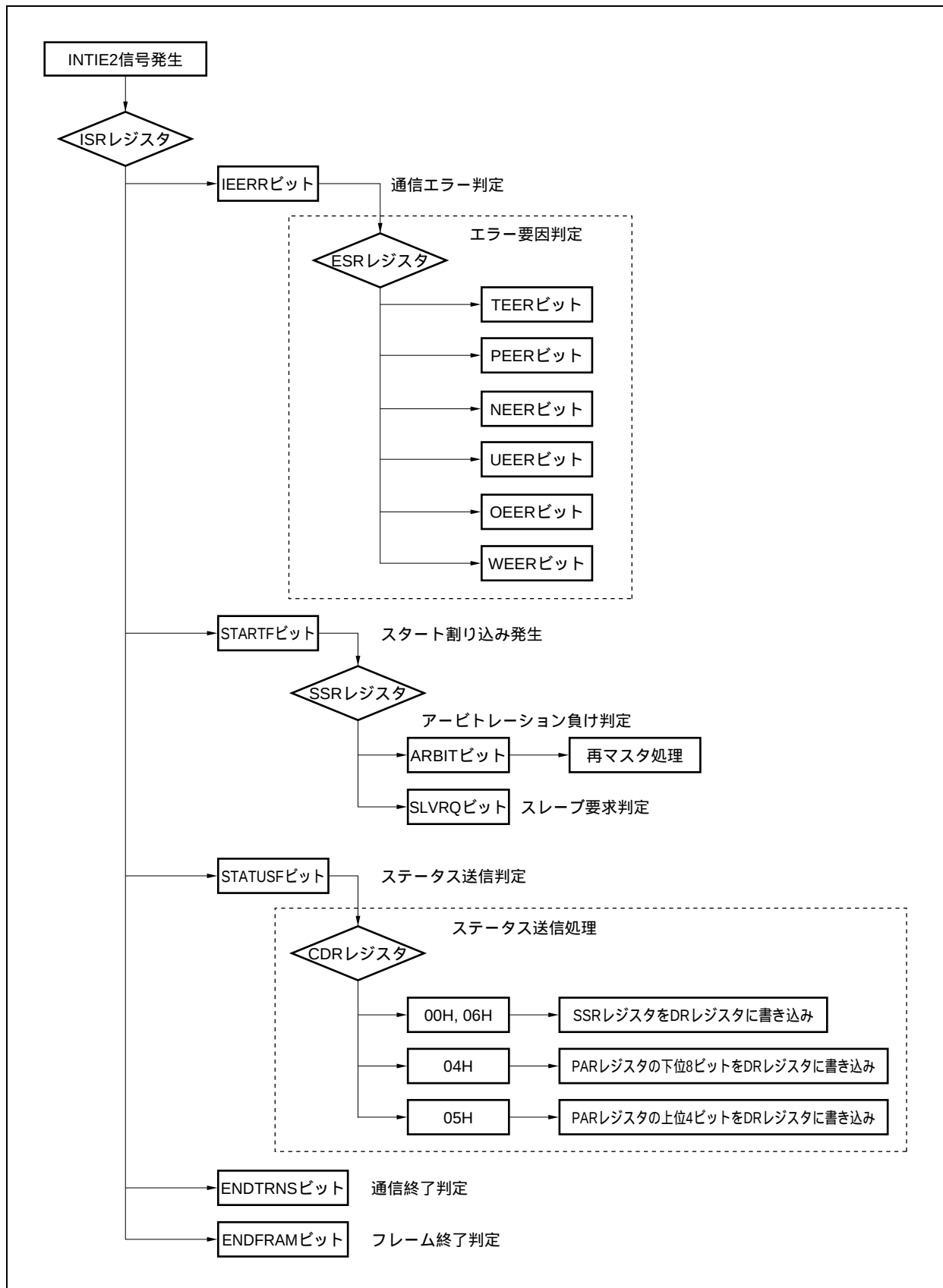
図18 - 25 INTIE2信号の割り込み判定例 (INTIE1, INTIE2信号使用時)
