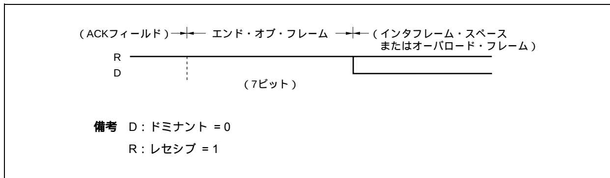
図19 - 12 エンド・オブ・フレーム (EOF)
