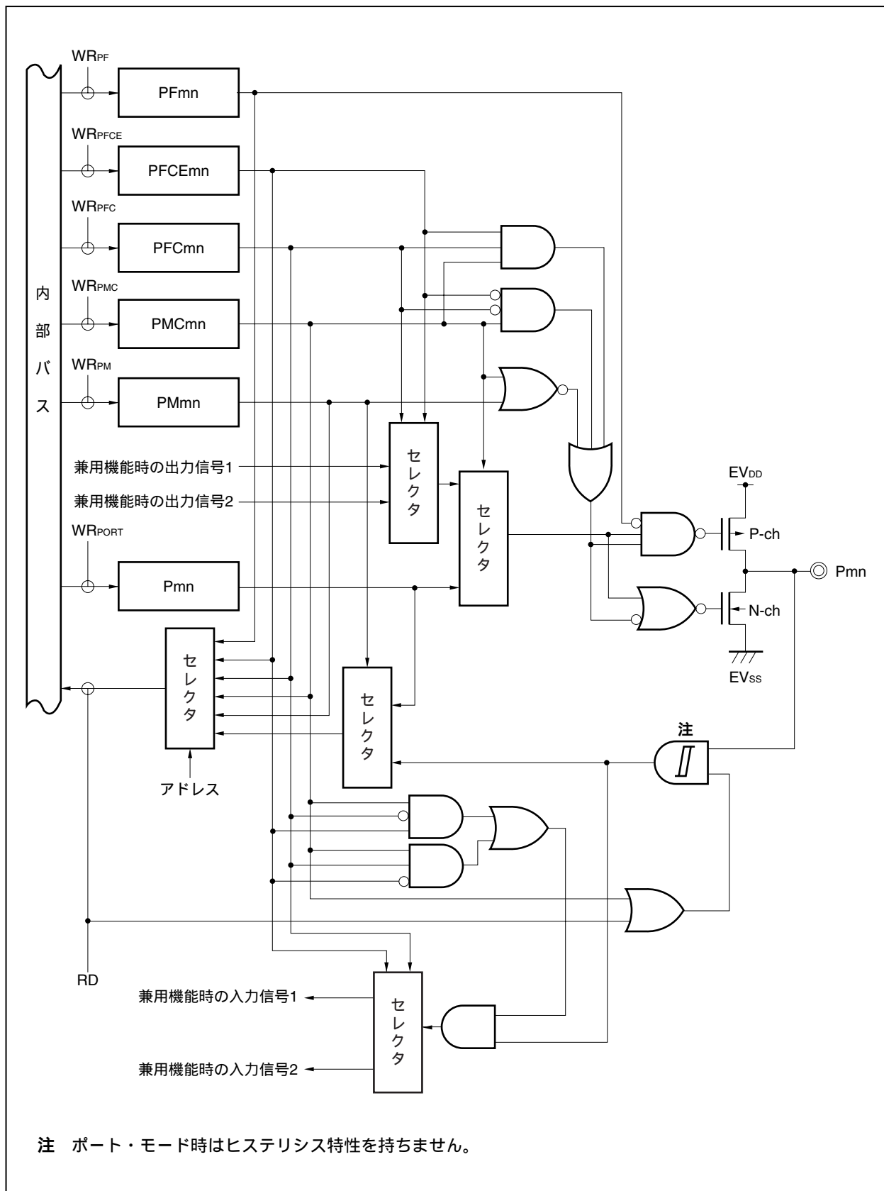
図4 - 38 タイプU - 14のブロック図
