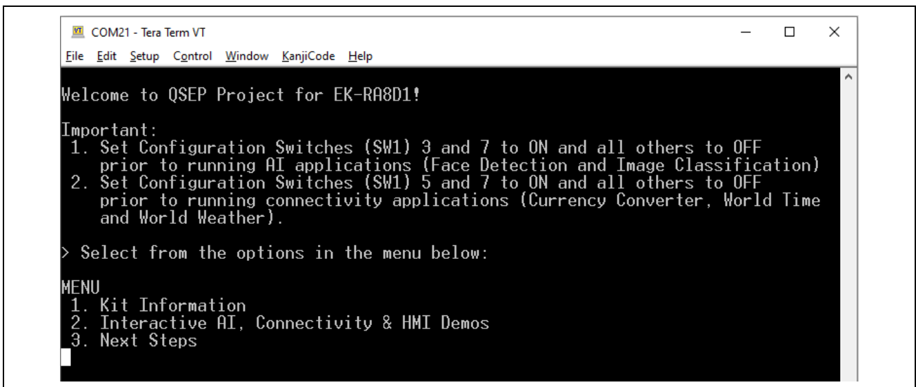
図 25. Welcome and Main メニュー
