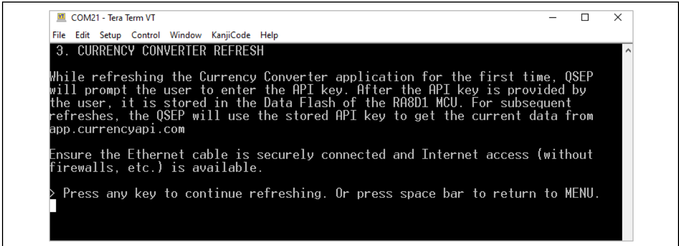
図 29. Currency Converter のリフレッシュ
