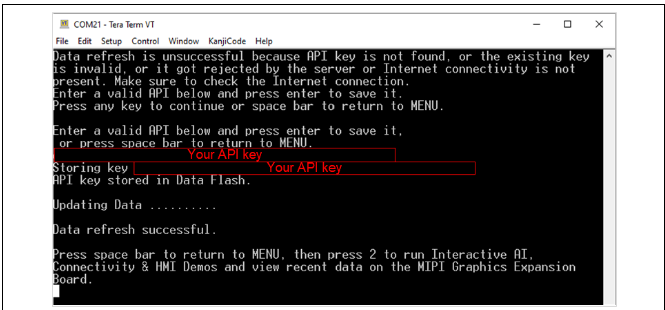
図 30. Currency API キーの初回入力
