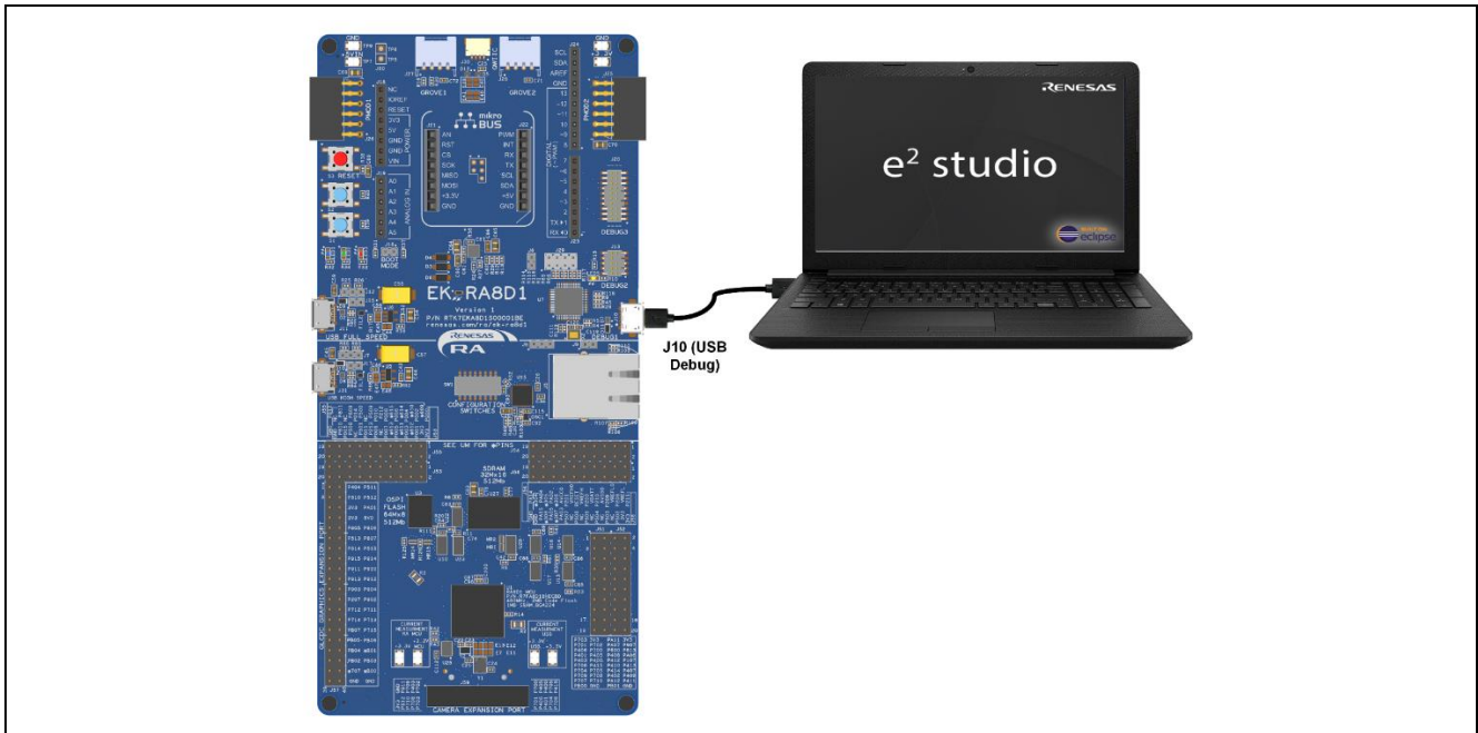
図 50. USB デバッグポートを使用した EK-RA8D1 ボードとホスト PC の接続
