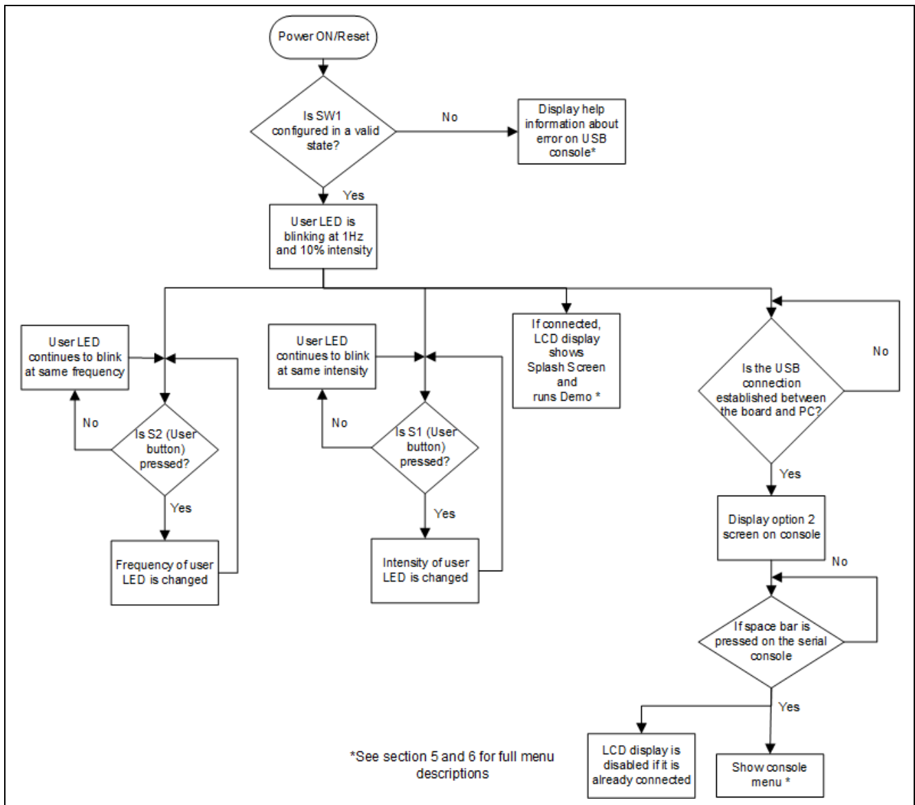
図 6. クイック スタート サンプル プロジェクト フロー
