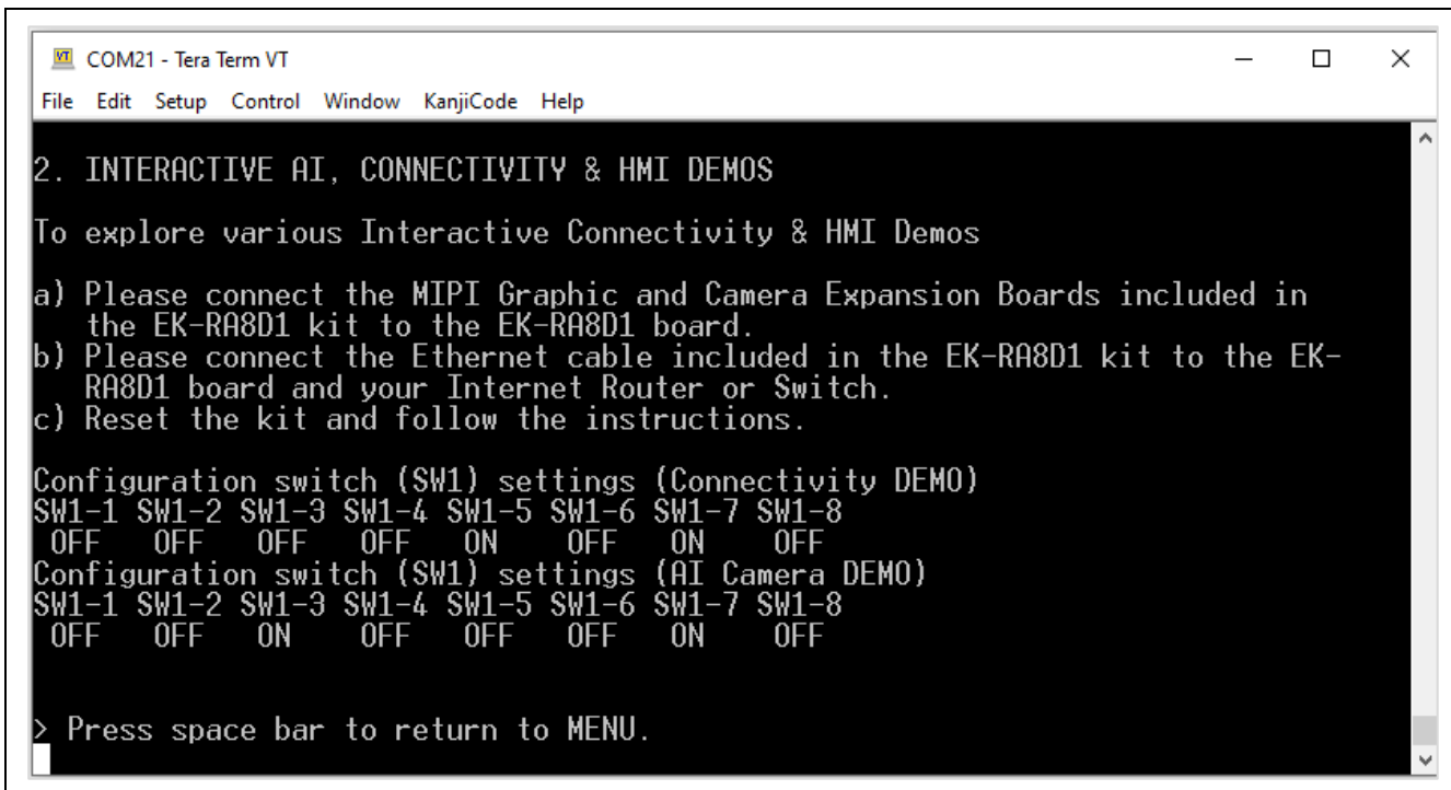
図 12. 失敗した構成
