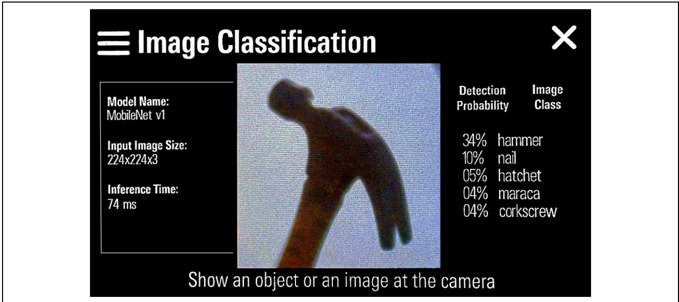
図 24. Image Classification の例
