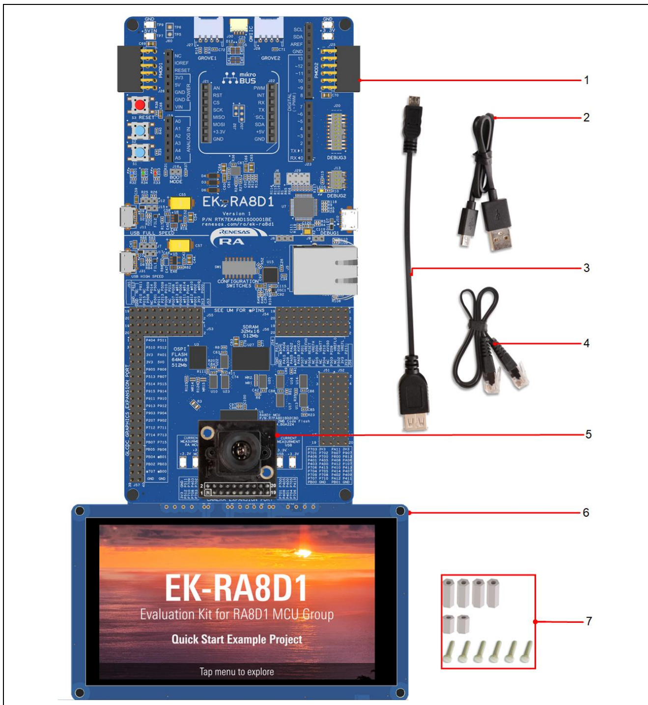
図 1. EK-RA8D1 評価キット内容
