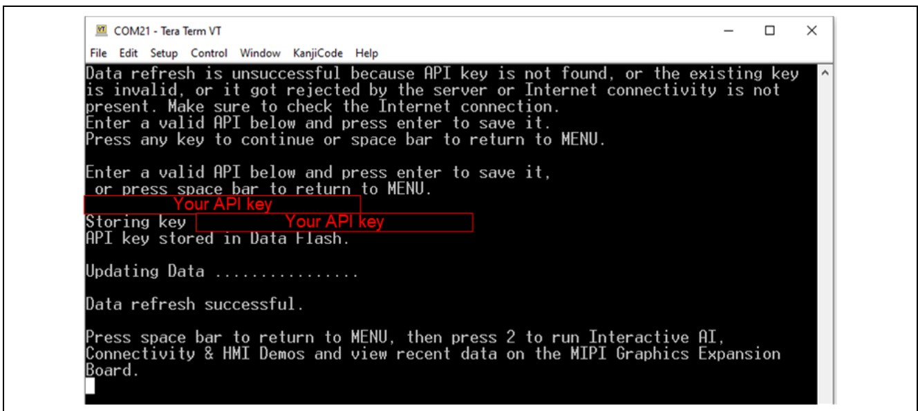
図 34. World Weather API キーの初回入力
