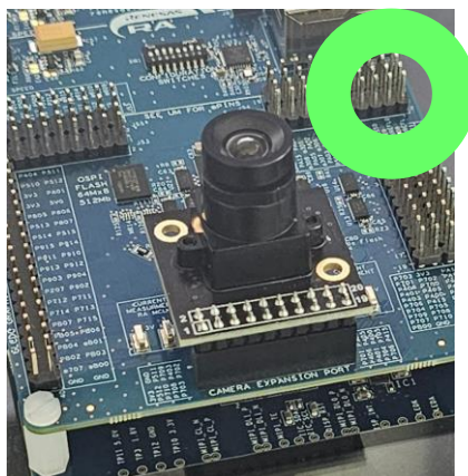
図 3. カメラ拡張ボードの正しい接続
