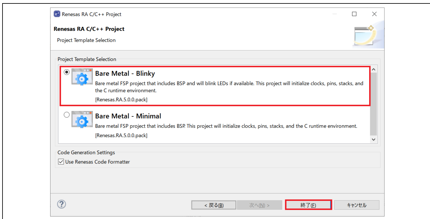
図 3-22 ライブラリ用プロジェクトテンプレートの選択
