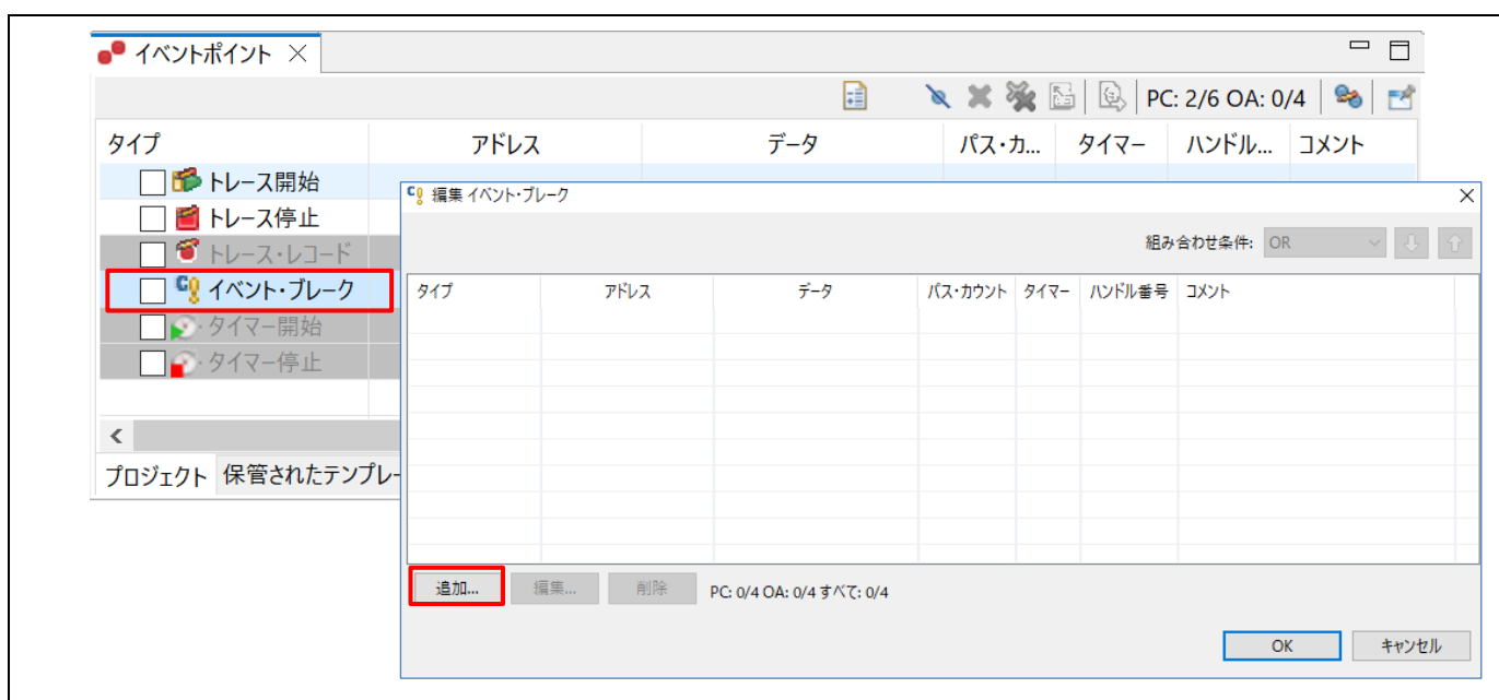
図 5-27 デバッガ - [イベントポイント] ビュー(1/2)
