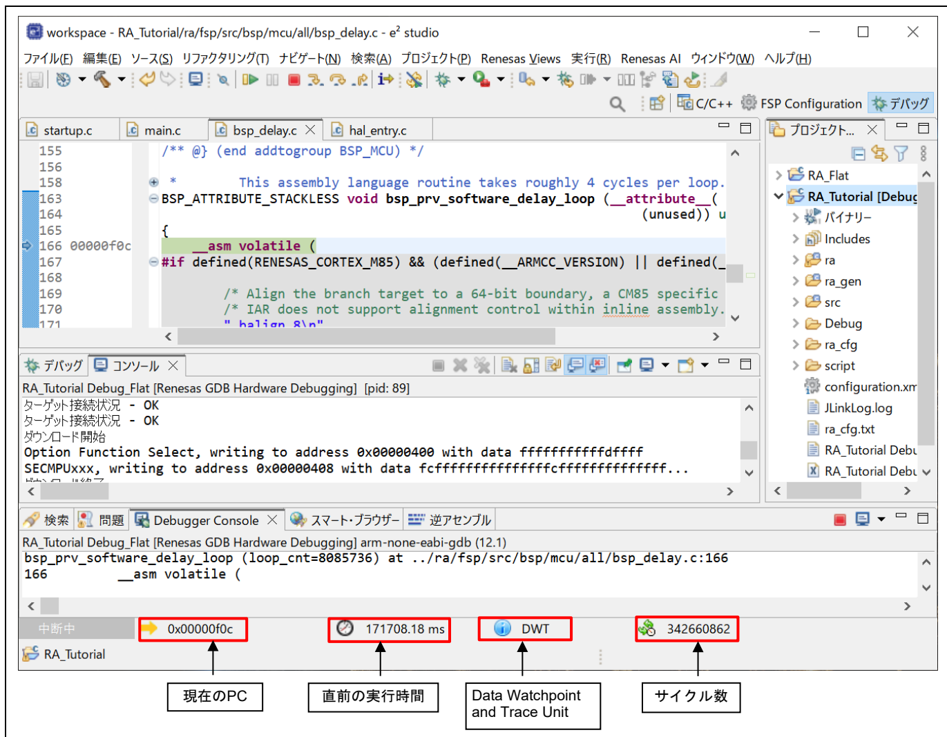
図 5-38 Run Break Timer による直前のプログラム実行のパフォーマンス表示
