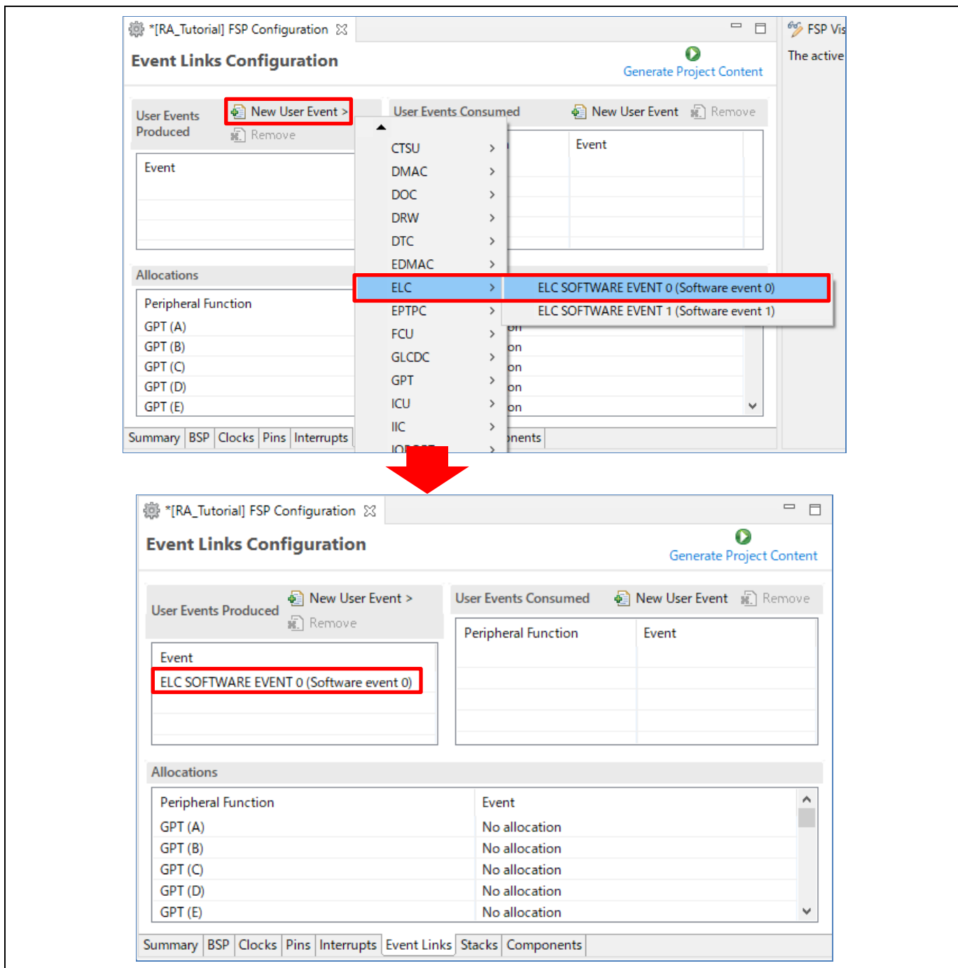
図 3-60 発生させるユーザイベントの設定
