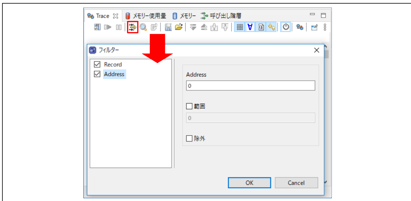
図 5-34 デバッガー トレース結果のフィルタ
