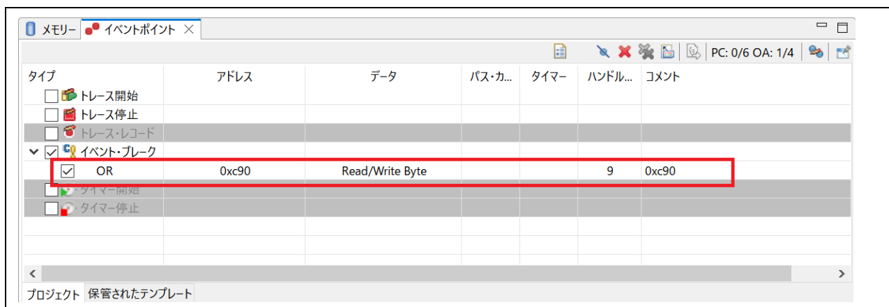
図 5-19 デバッガー - [イベントポイント] ビュー
