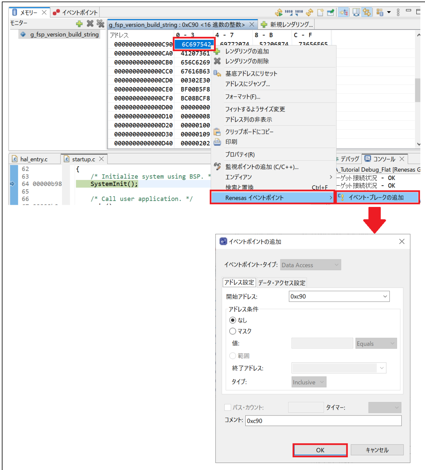
図 5-18 デバッグ - イベントポイントとして設定
