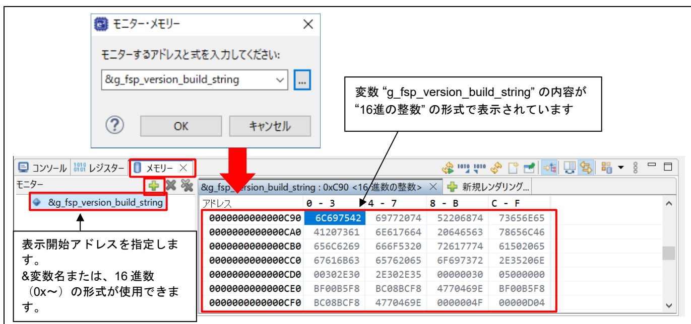
図 5-16 デバッガー [メモリー] ビュー
