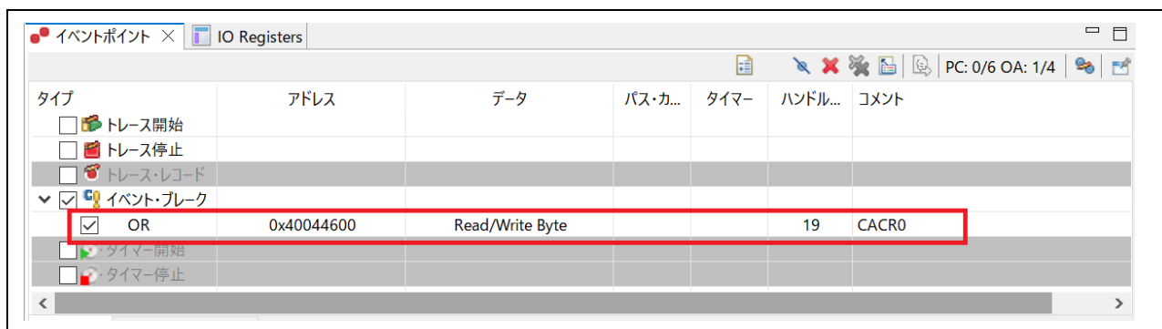
図 5-26 デバッガ - [イベントポイント] ビュー
