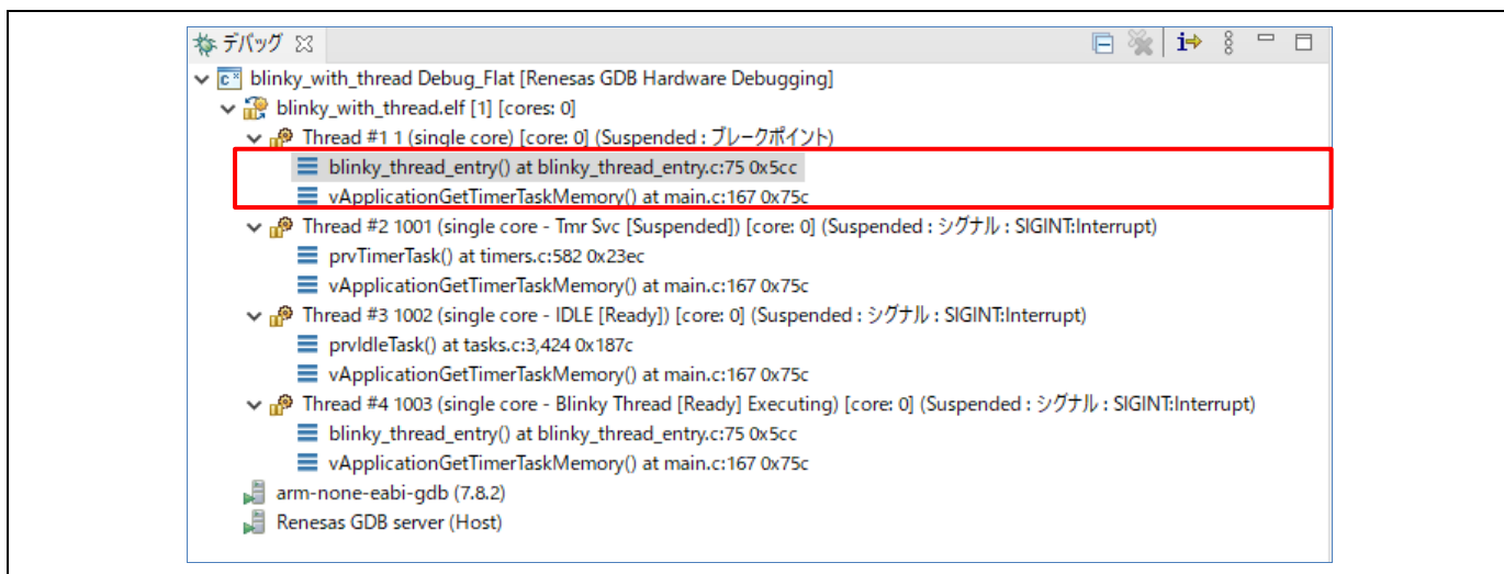
図5-9 デバッガー - [デバッグ] ビュー
