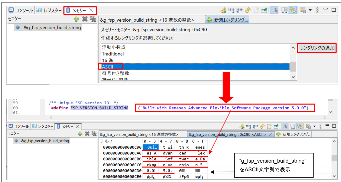
図 5-17 デバッガー - [メモリー] ビューの新規レンダリング（表示方式）
