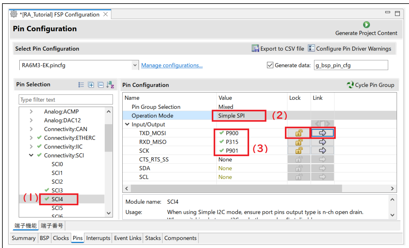
図 3-43 RA プロジェクト構成 – 端子構成の設定 (周辺機能ごとに設定)
