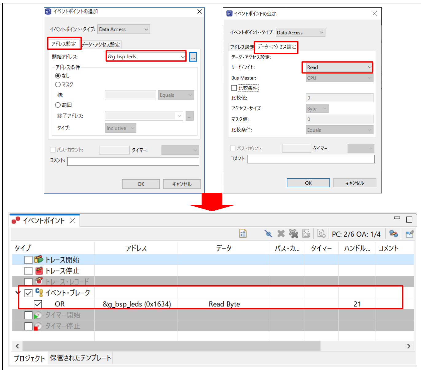
図 5-28 デバッガー [イベントポイント] ビュー(2/2)
