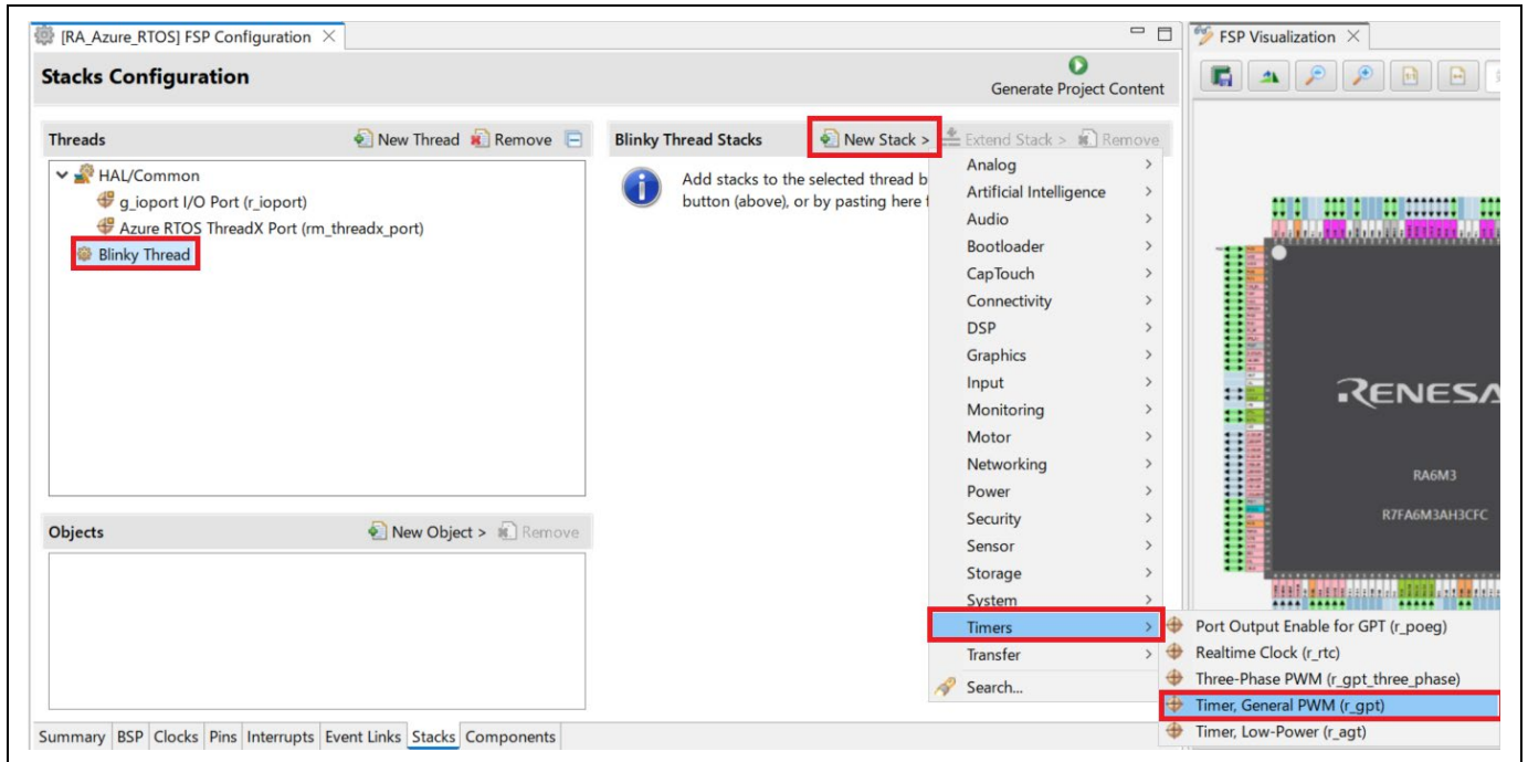
図7-3 Azure RTOSアプリケーションの設定 – GPTモジュールの追加
