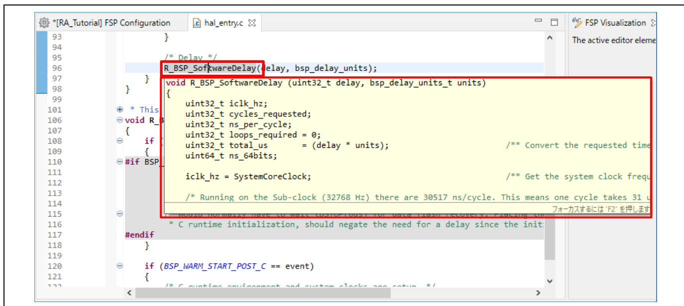
図 3-63 吹き出し機能による情報の表示
