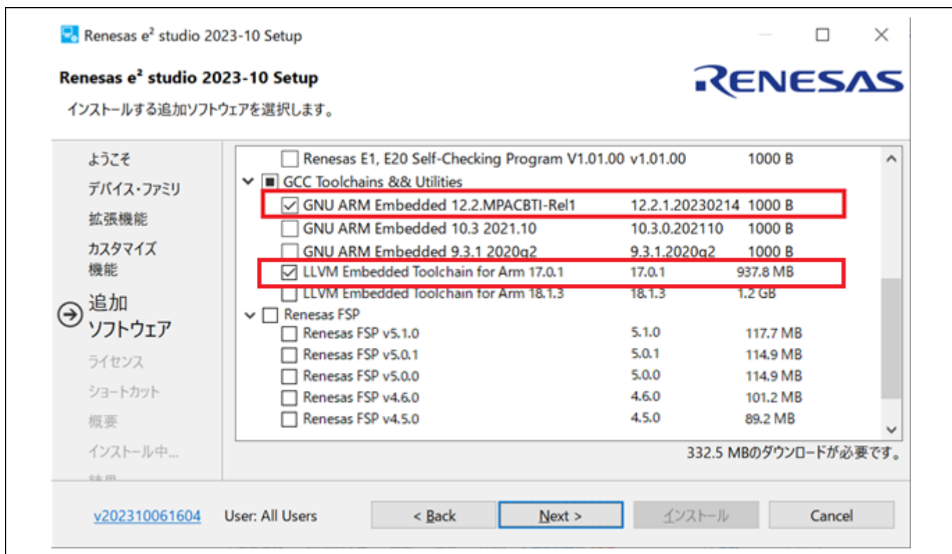
図 2-17 インストール – [追加ソフトウェア] ページ
