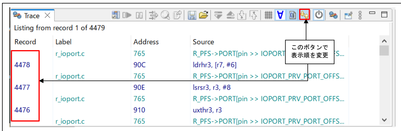
図 5-33 表示順の変更
