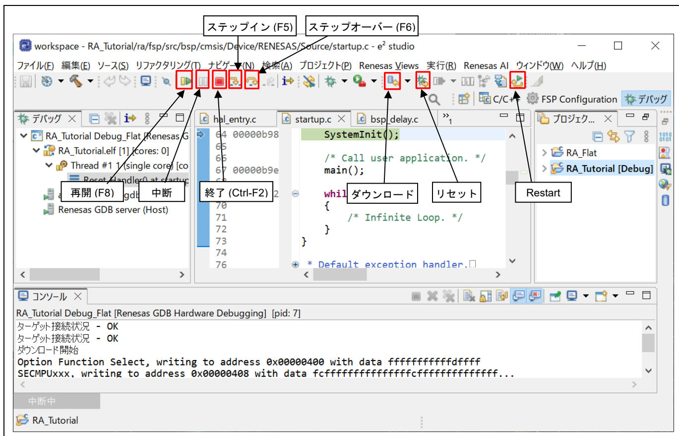
図 5-7 デバッグ - [デバッグ] ビューの便利なツールバー
