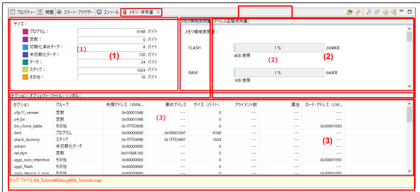
図 5-21 [メモリー使用量] ビューのエリア
