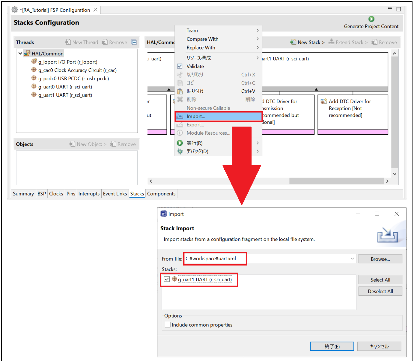
図 3-53 RA スタックのインポート
