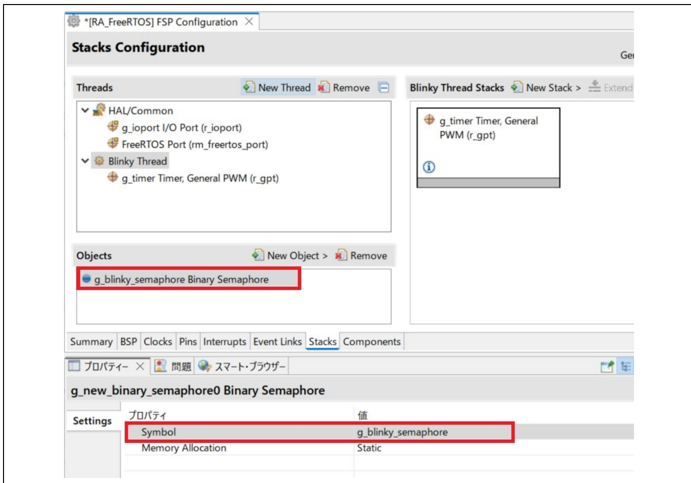
図 6-6 FreeRTOS アプリケーションの設定 – セマフォオブジェクトの設定
