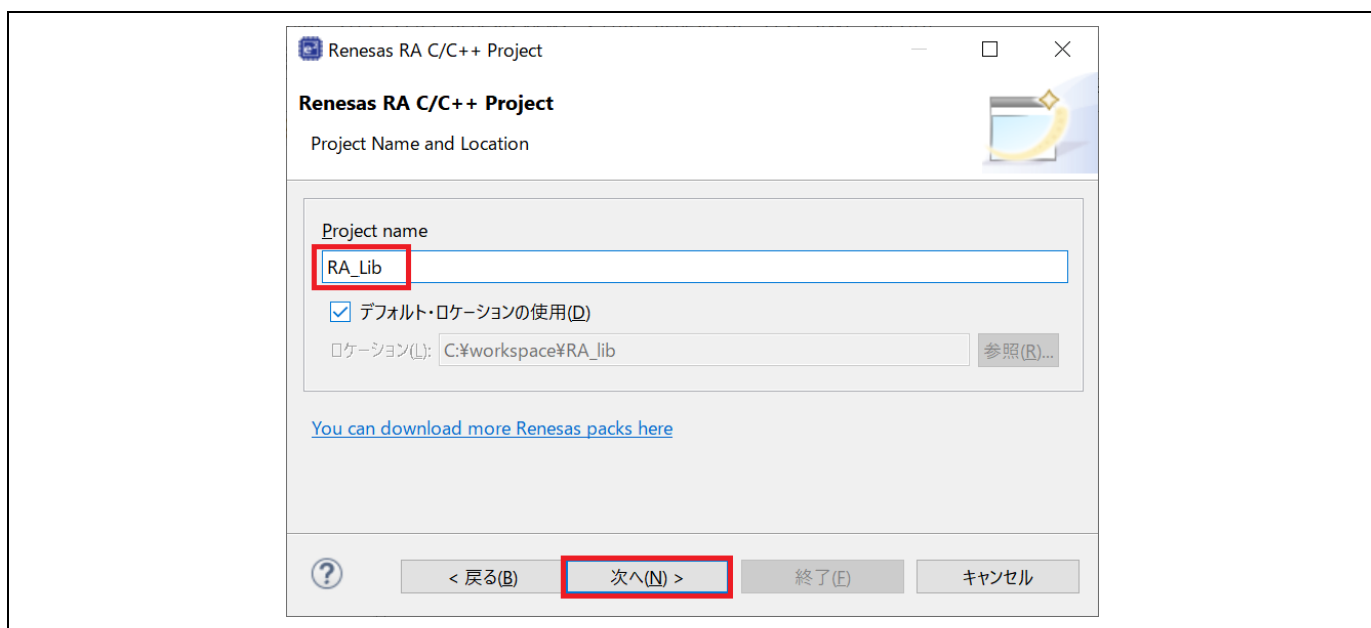
図 3-19 ライブラリプロジェクトの設定
