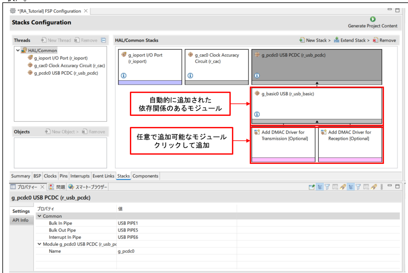
図 3-49 RA プロジェクト構成 – 依存関係のあるモジュール
