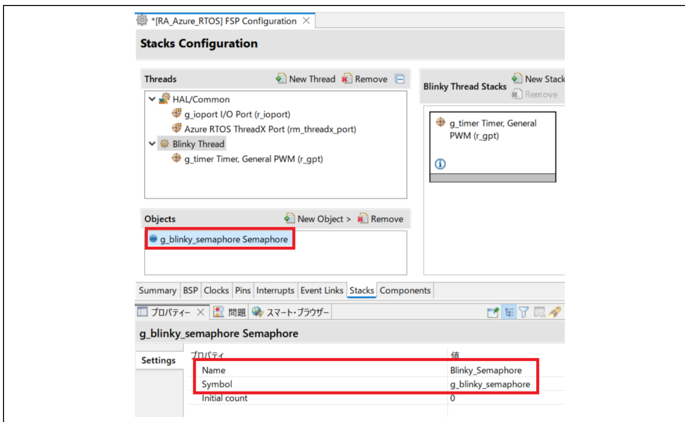
図 7-6 Azure RTOS アプリケーションの設定 – セマフォオブジェクトの設定
