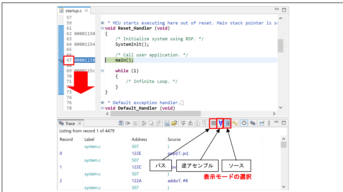
図 5-32 デバッガ - [トレース] ビューの表示モード選択
