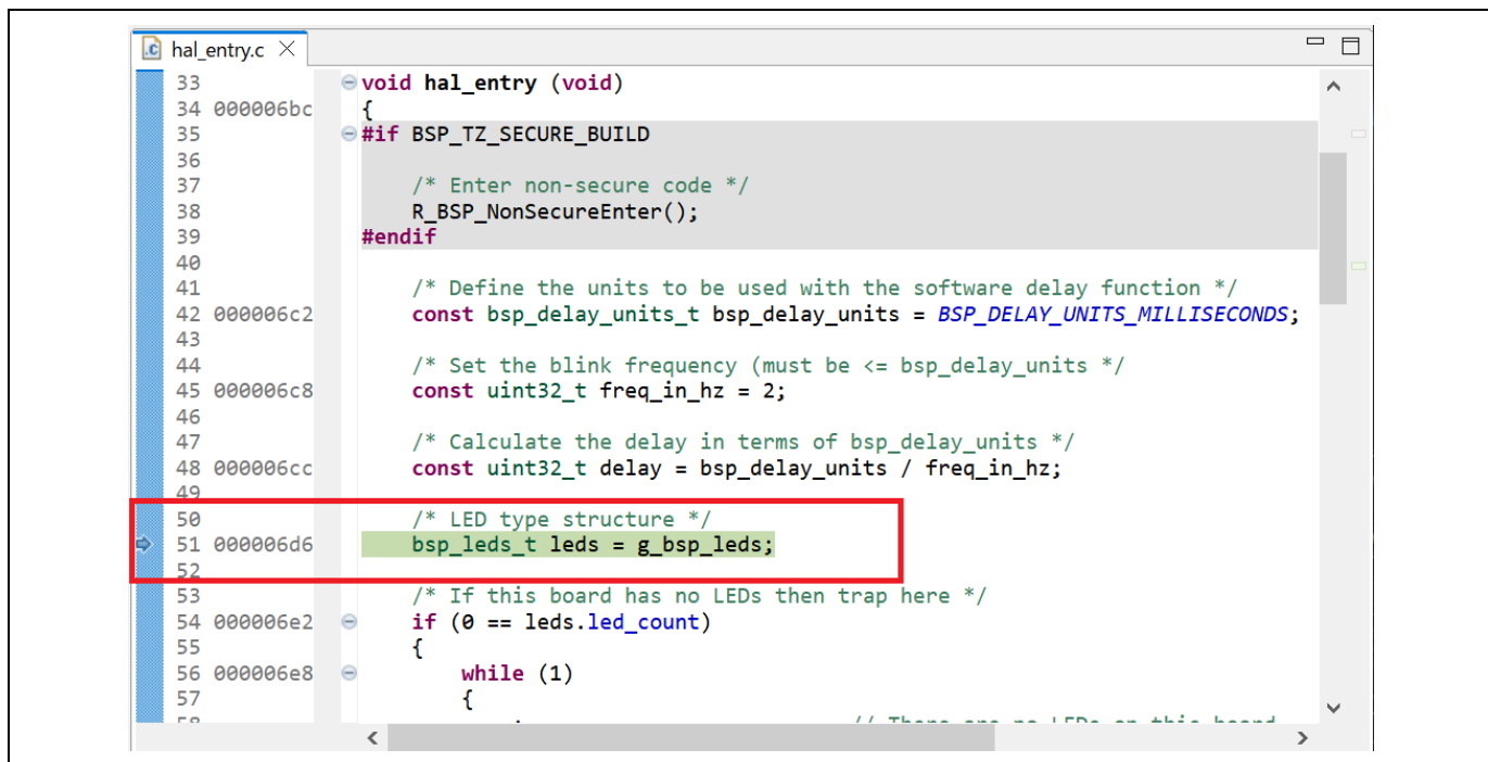
図 5-29 デバッガ – イベントブレークの実行
