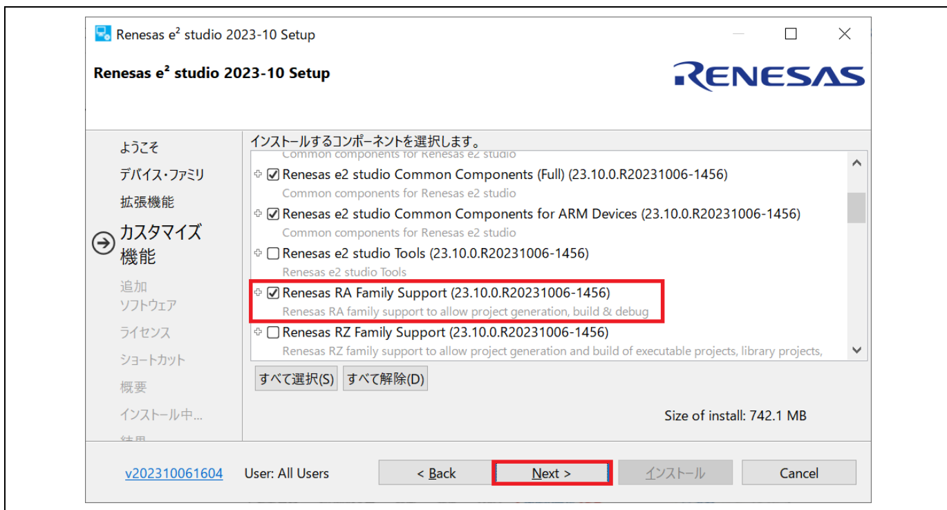
図 2-16 インストール – [カスタマイズ機能] ページ
