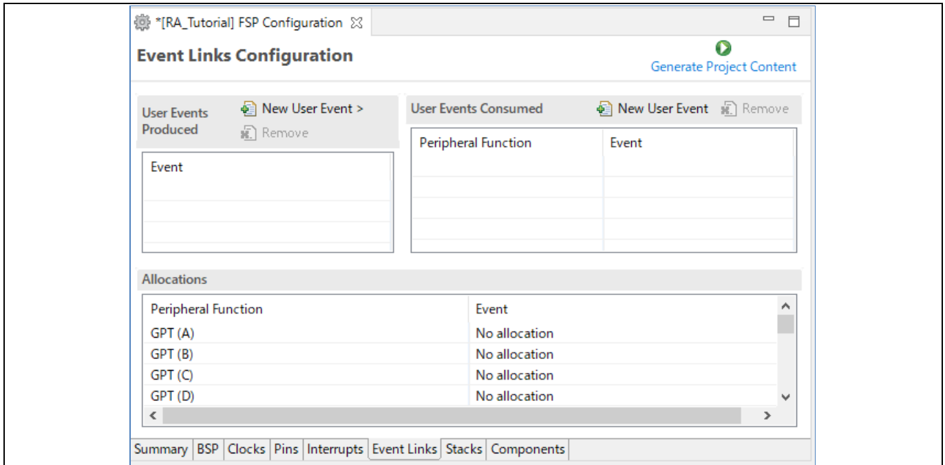
図 3-59 [Event Links Configuration] ページ
