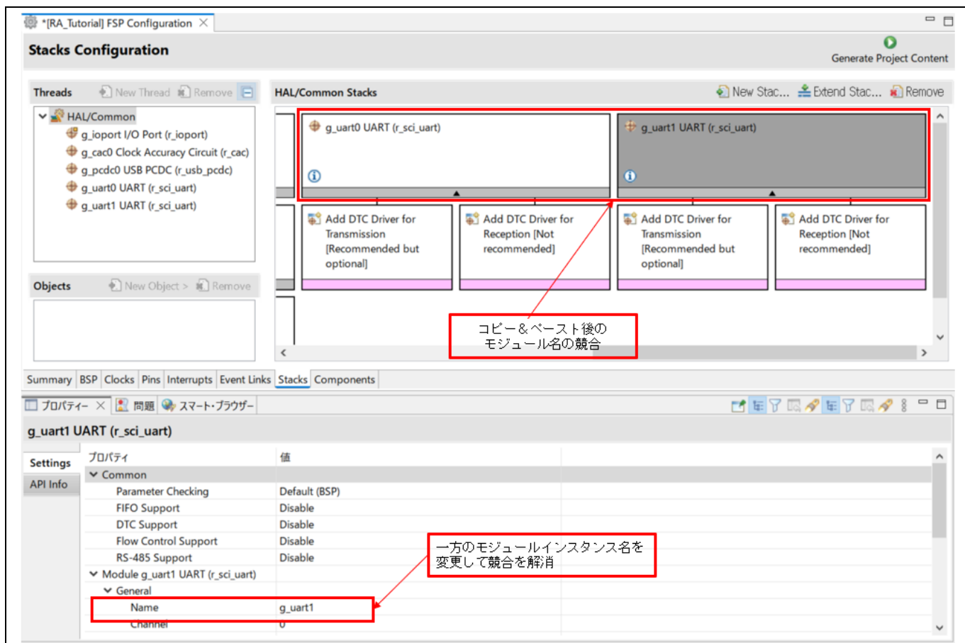
図 3-51 モジュールインスタンス名の競合
