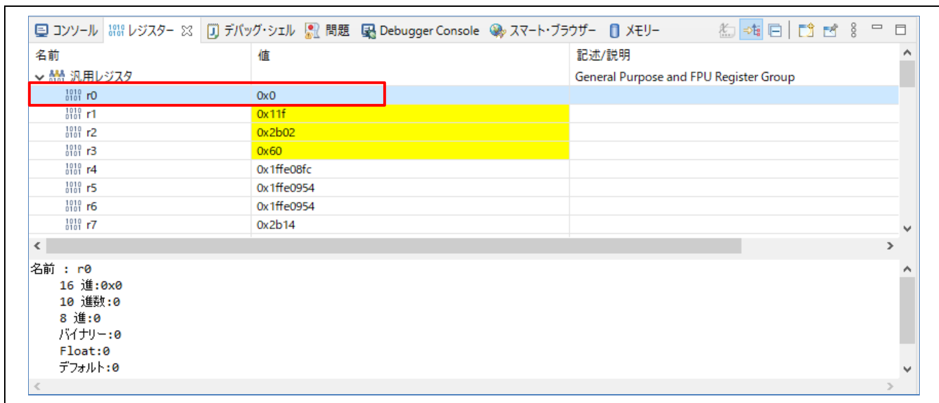
図 5-15 デバッガー [レジスタ] ビュー
