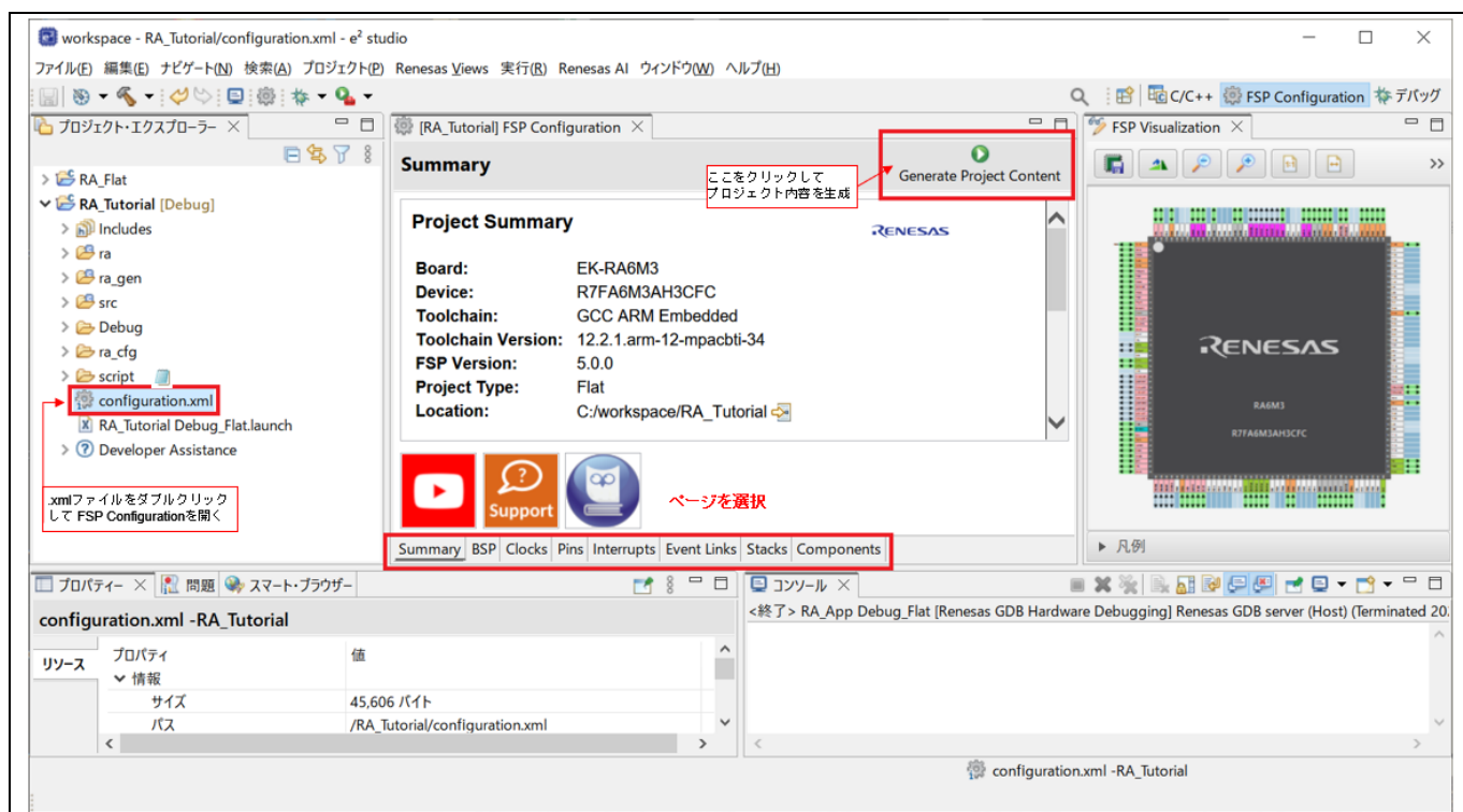
図 3-33 RA プロジェクト構成 – [RA プロジェクトコンフィグレーションエディタ] ビュー
