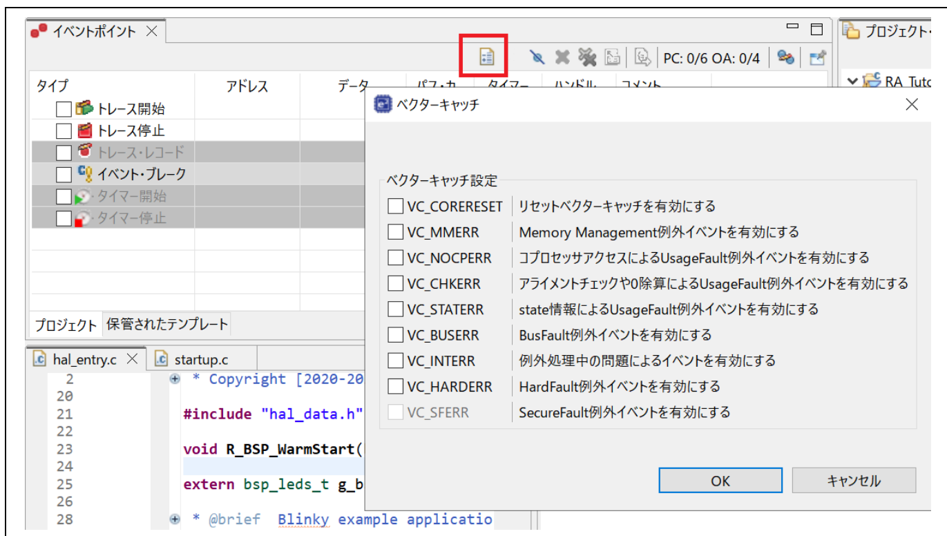
図 5-30 デバッガ – ベクタキャッチによるブレーク
