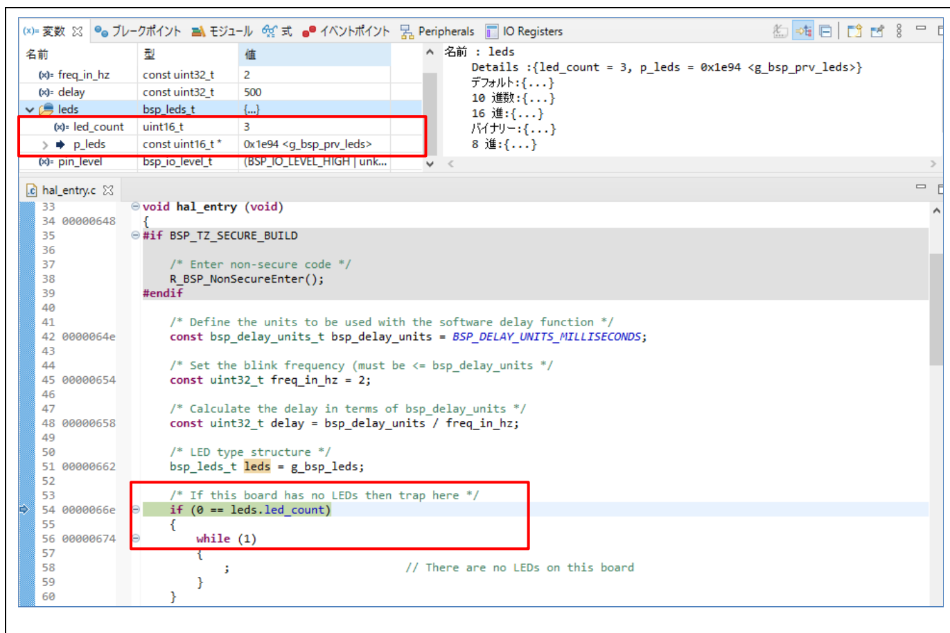
図 5-23 デバッガー - [変数] ビュー
