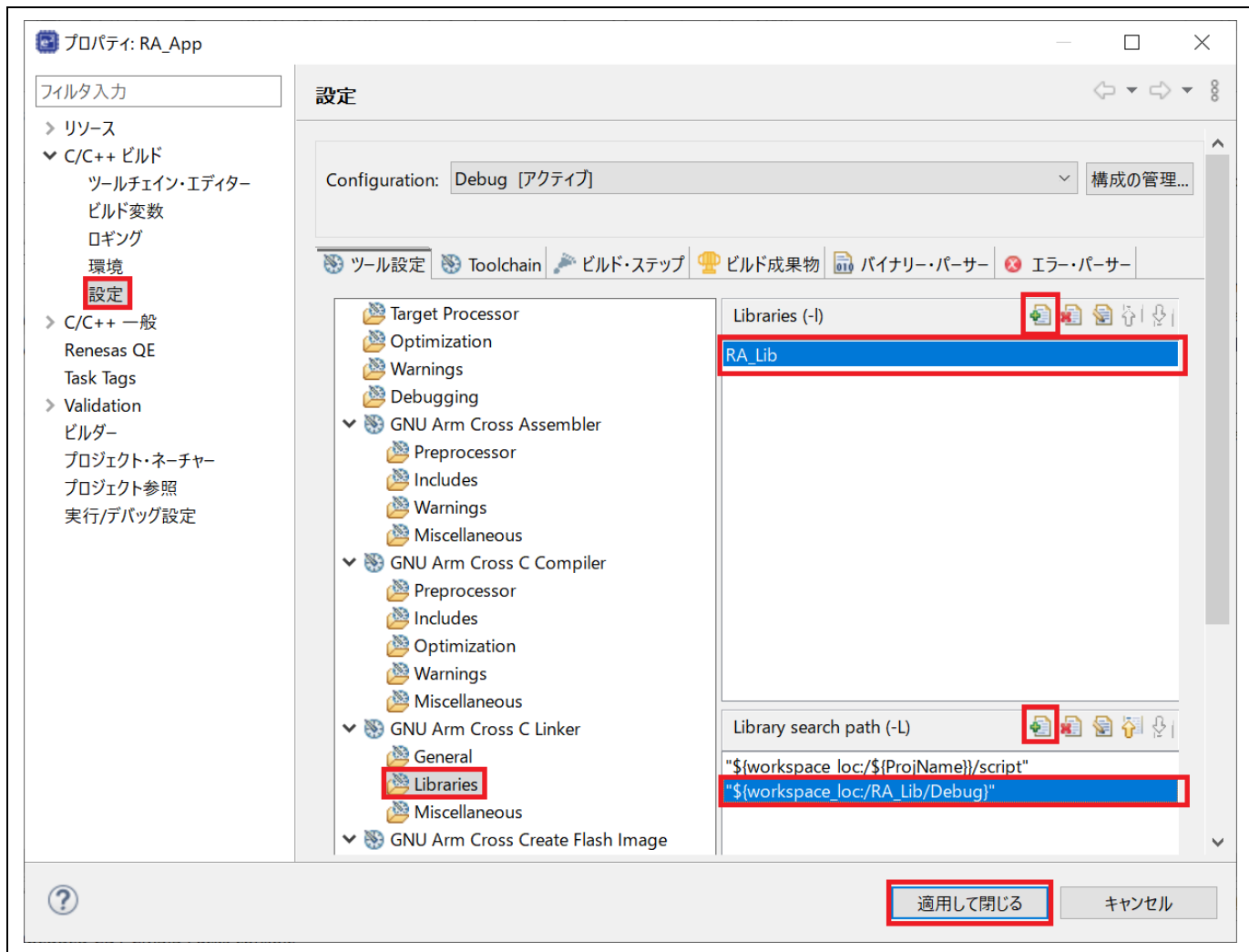
図 3-29 プロジェクトプロパティの設定
