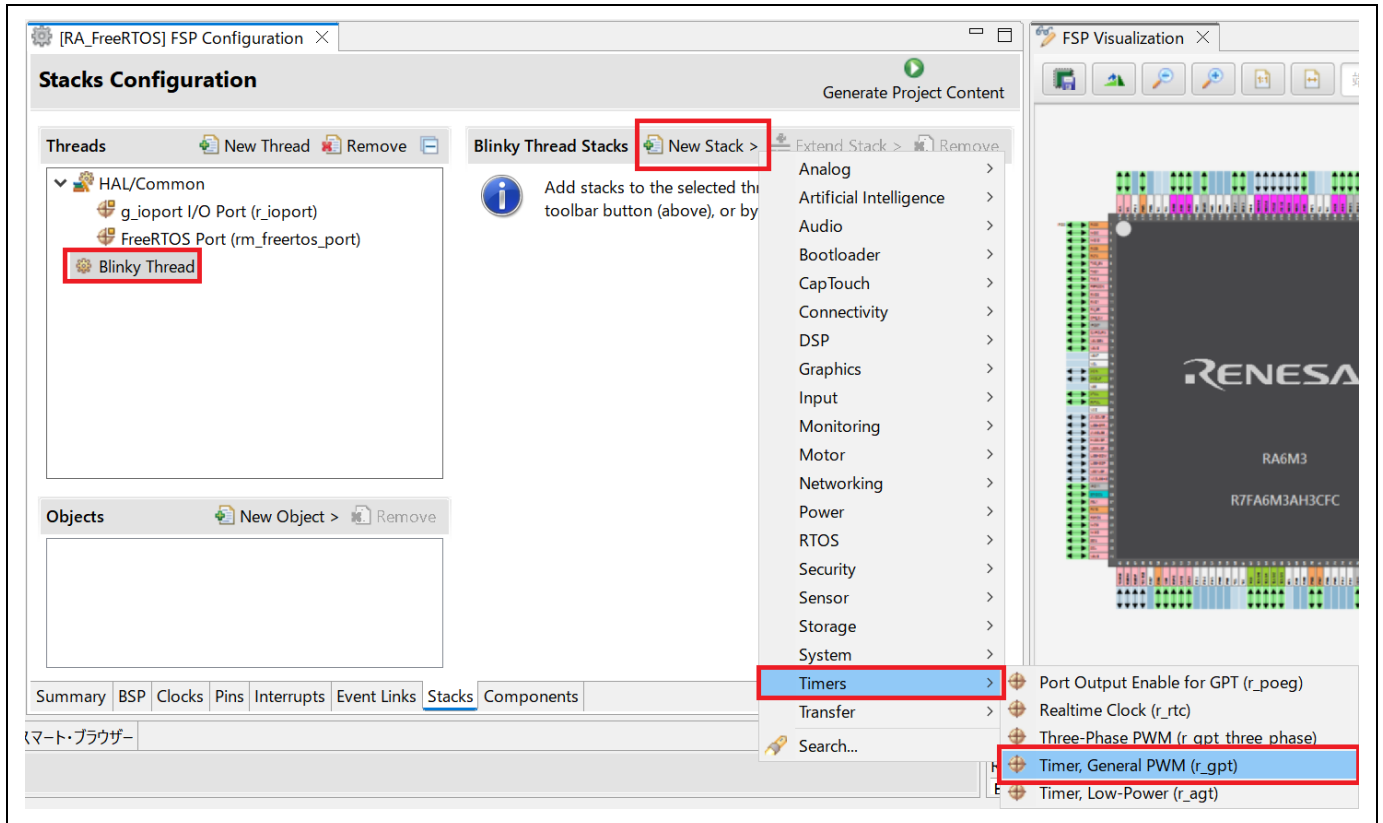
図 6-3 FreeRTOS アプリケーションの設定 – GPT モジュールの追加
