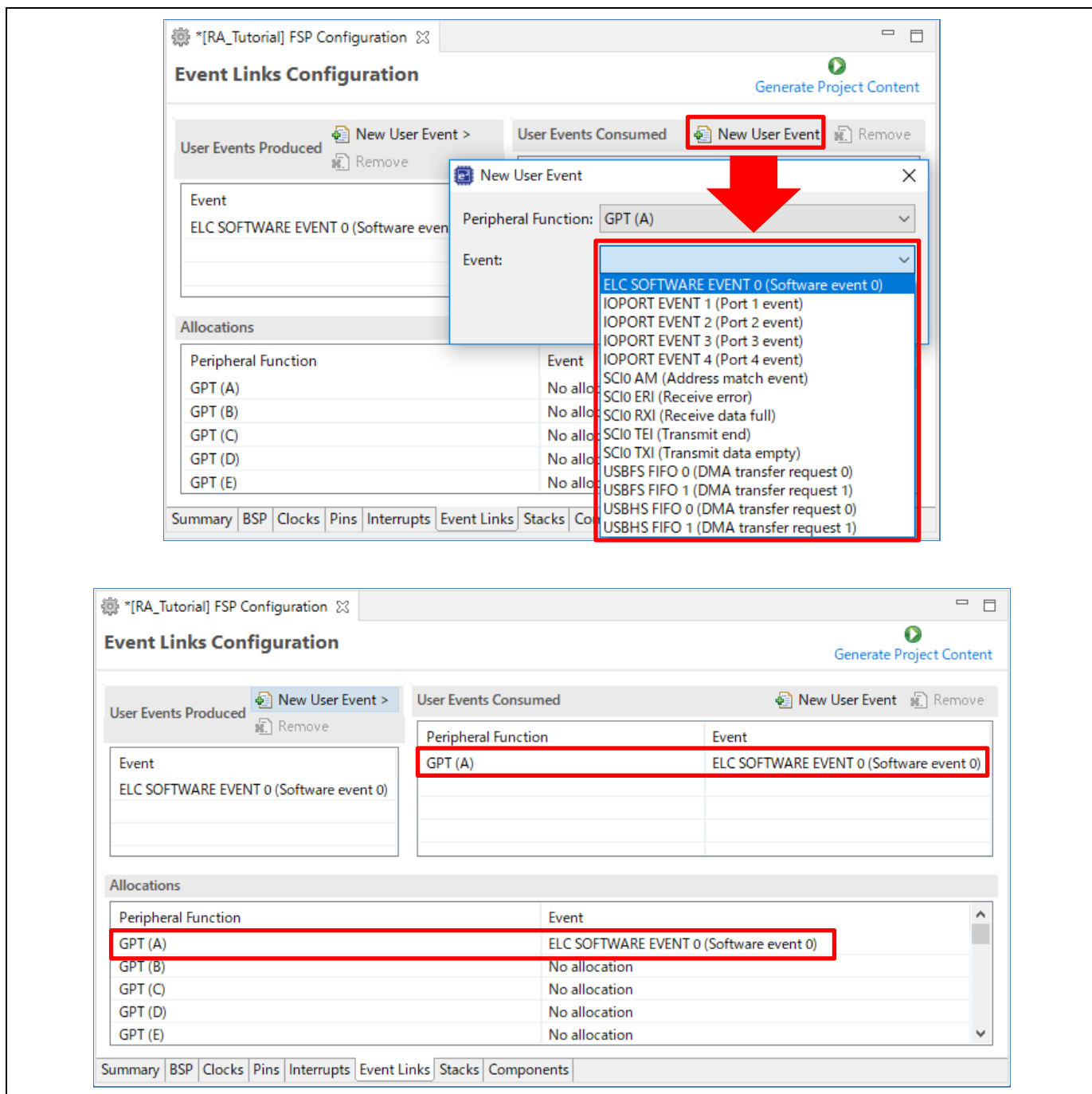
図 3-61 使用するユーザイベントの設定
