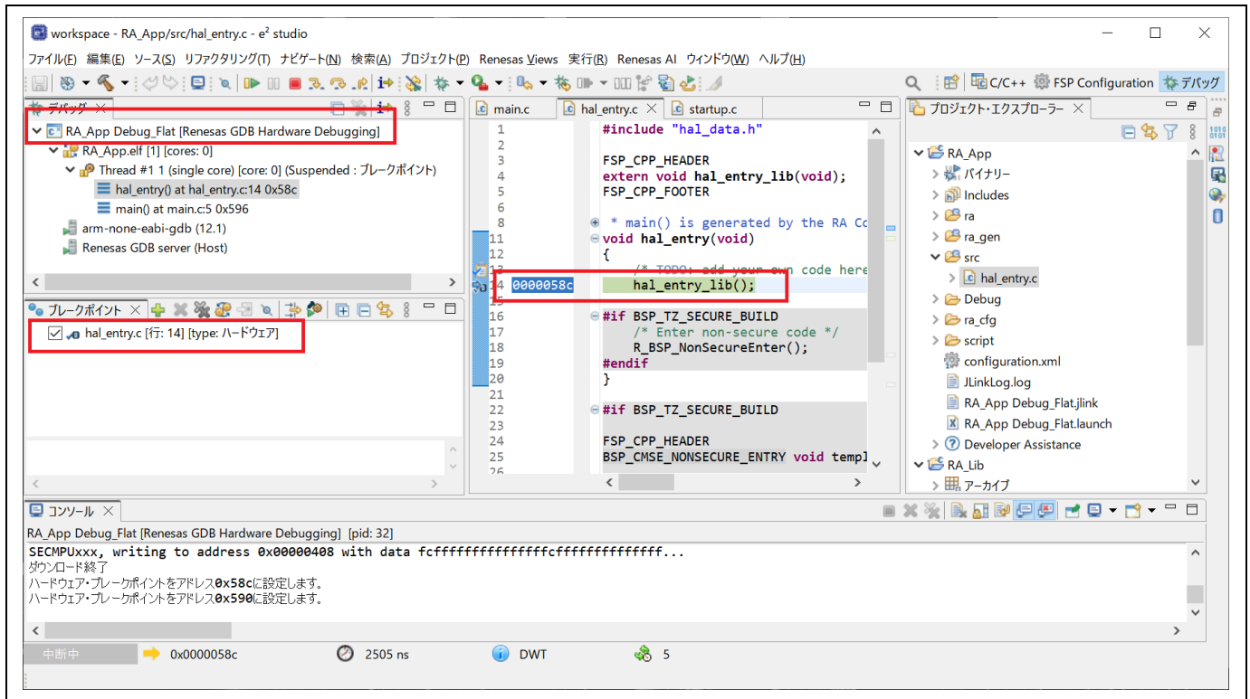
図 3-32 アプリケーションプロジェクトでのライブラリ関数の実行
