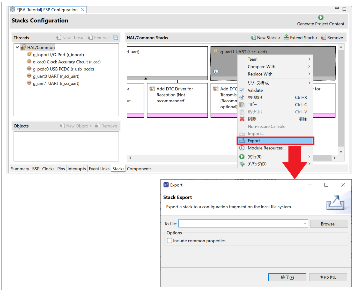
図 3-52 RA スタックのエクスポート
