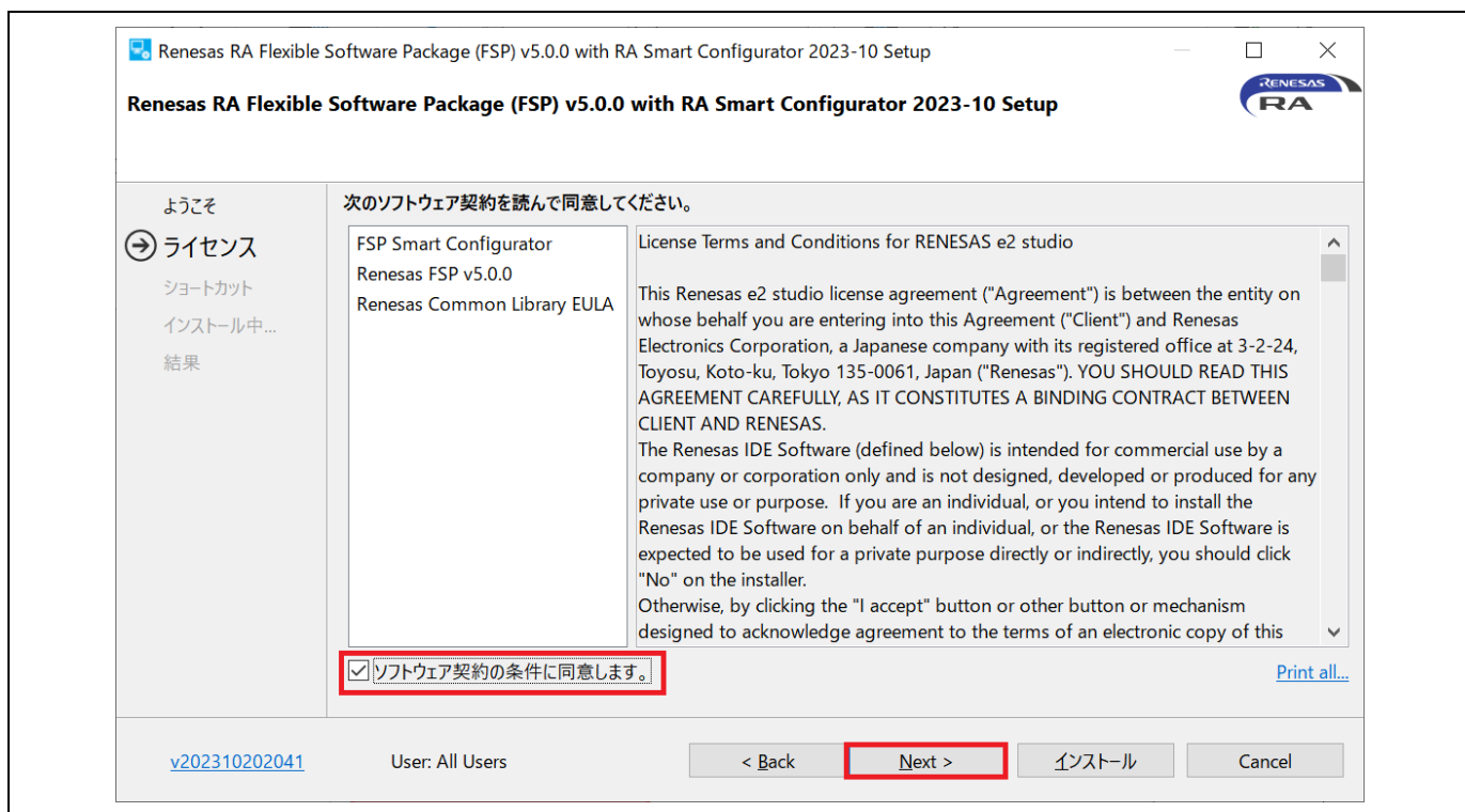
図 2-22 インストール – ソフトウェア契約
