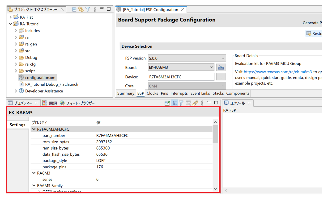
図 3-36 ボードのプロパティ
