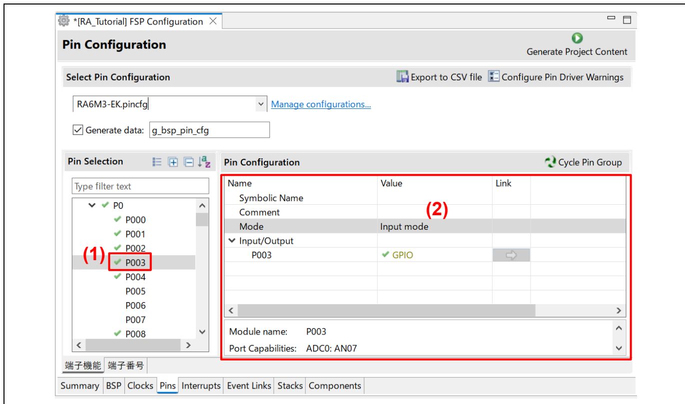
図 3-44 RA プロジェクト構成 – 端子構成の設定（端子ごとに設定）
