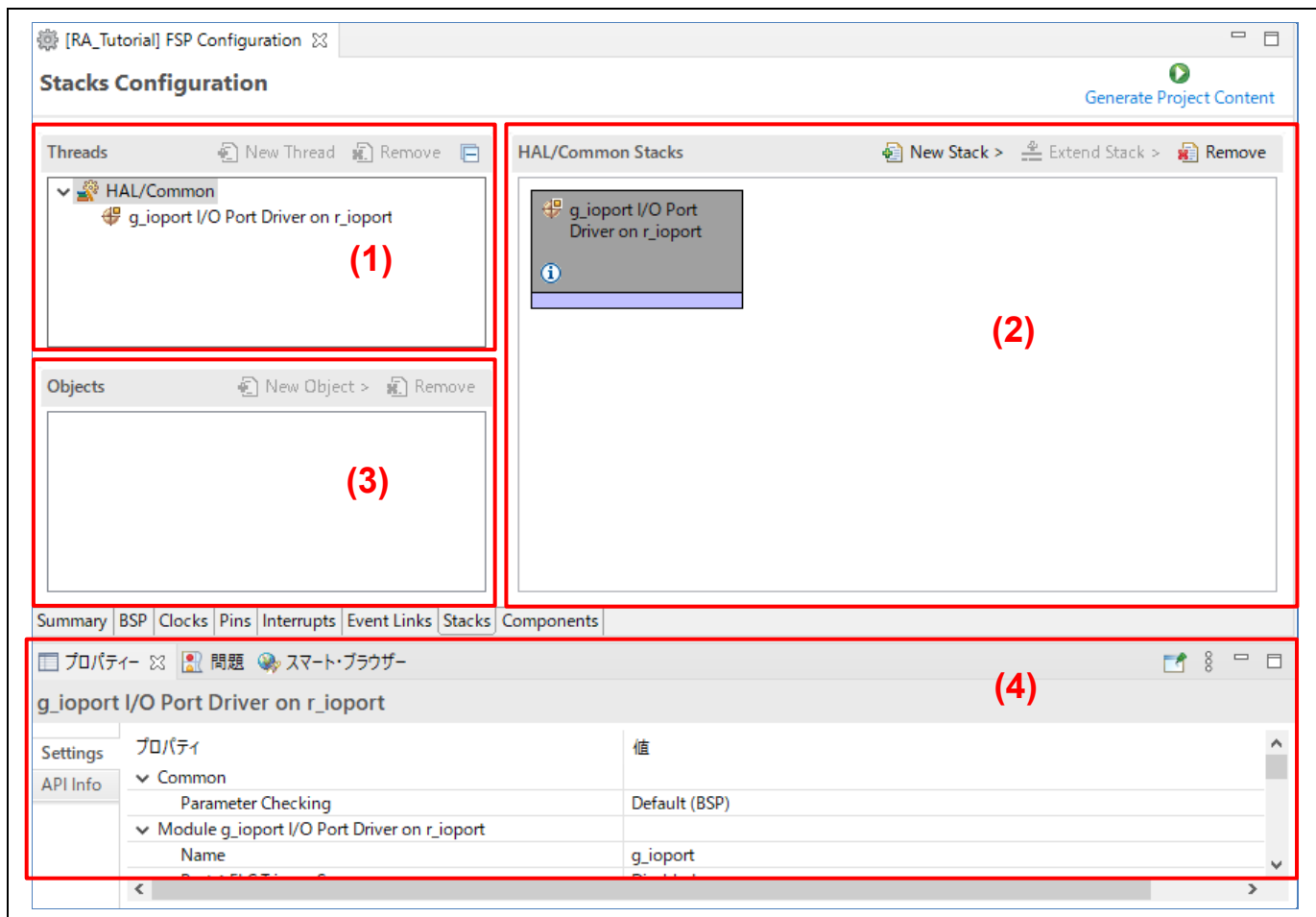
図 3-47 RA プロジェクト構成 – [Stacks Configuration] ページ
