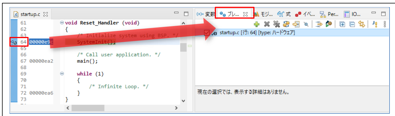
図 5-11 デバッガ [ブレークポイント] ビュー
