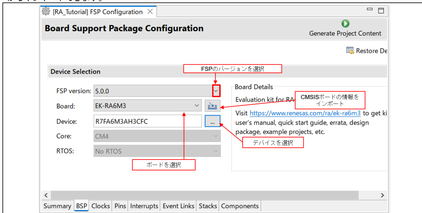
図 3-35 RA プロジェクト構成 – [BSP] ページ
