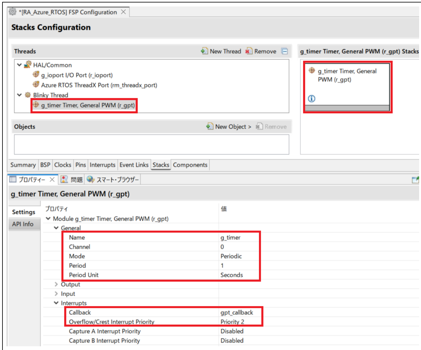
図 7-4 Azure RTOS アプリケーションの設定 - GPT モジュールの設定
