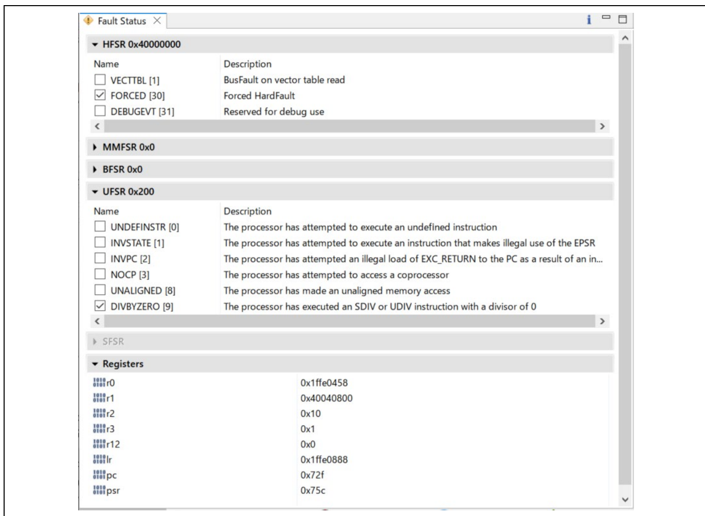
図 5-37 [Fault Status] ビュー — ハードウェアフォルト発生
