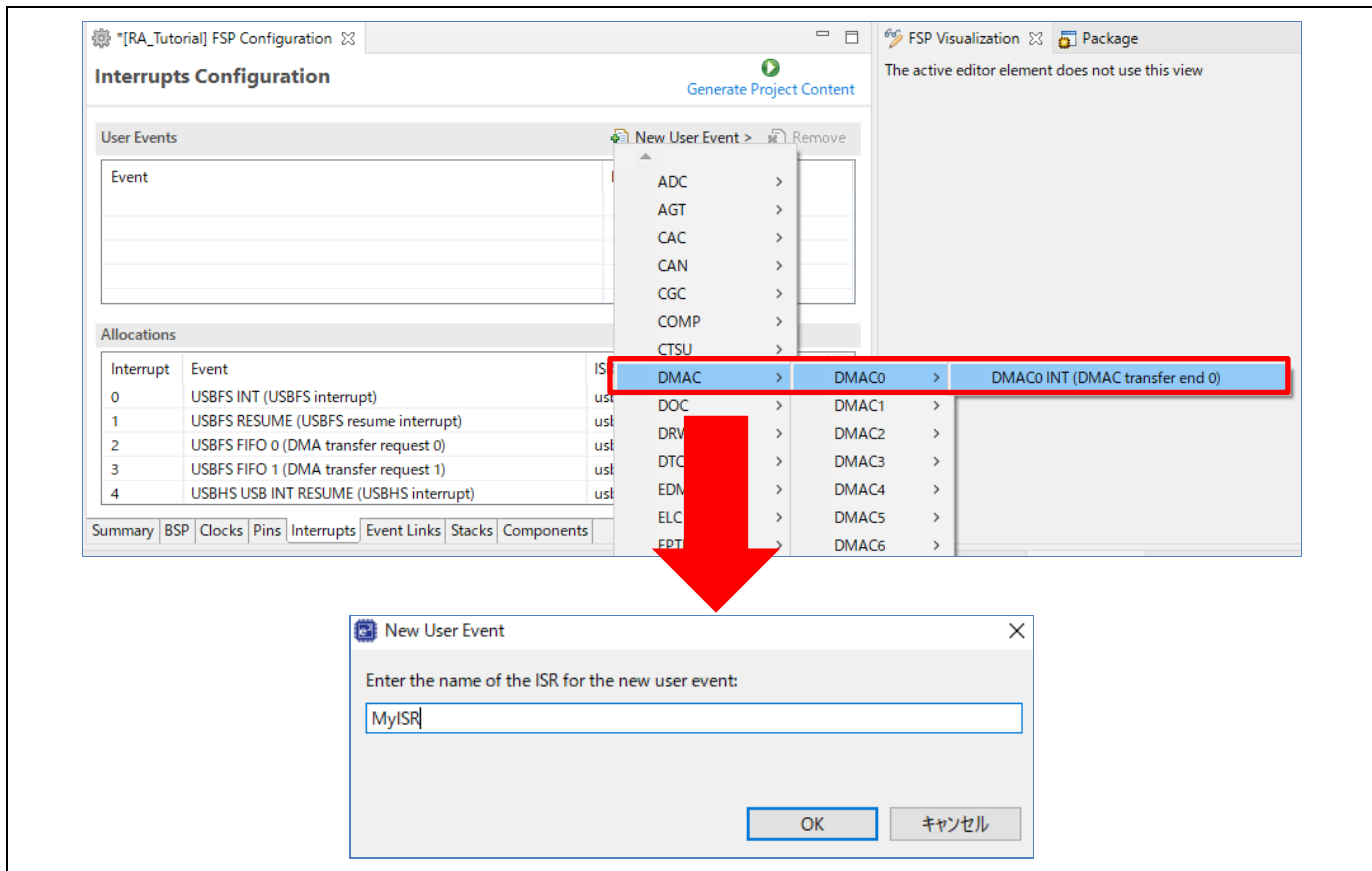
図 3-56 [Interrupts Configuration] ページ – 新規ユーザイベントの追加
