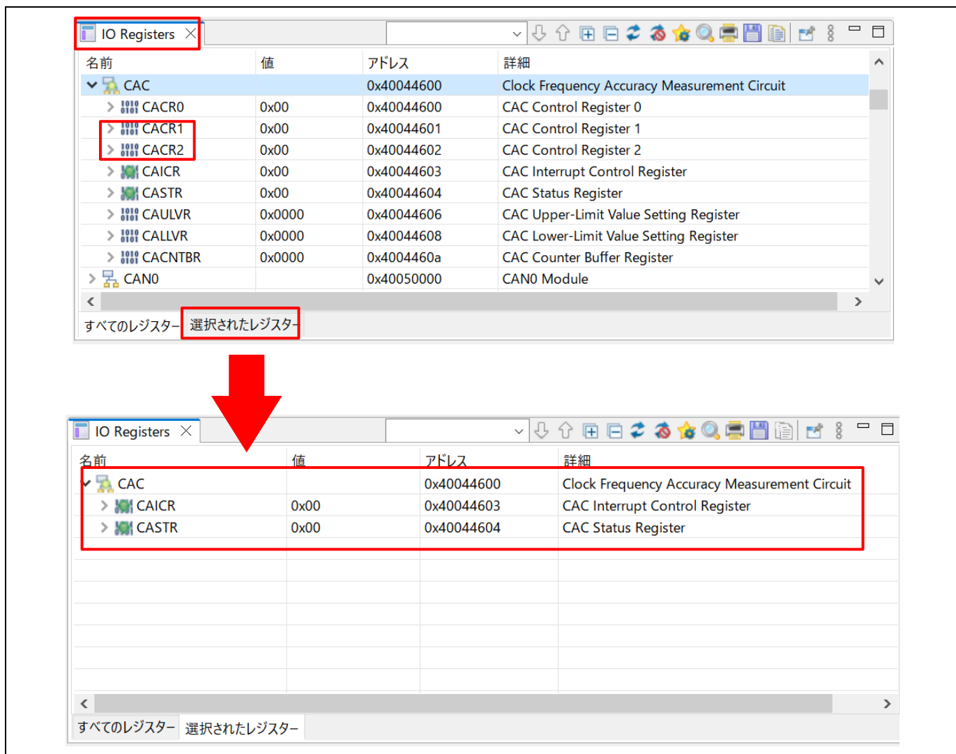
図 5-24 デバッグ - [IO Registers] ビュー
