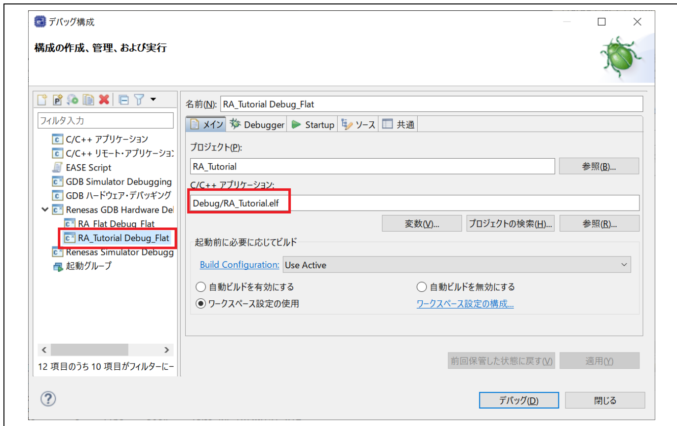
図 5-3 デバッグ – ロードモジュールの選択
