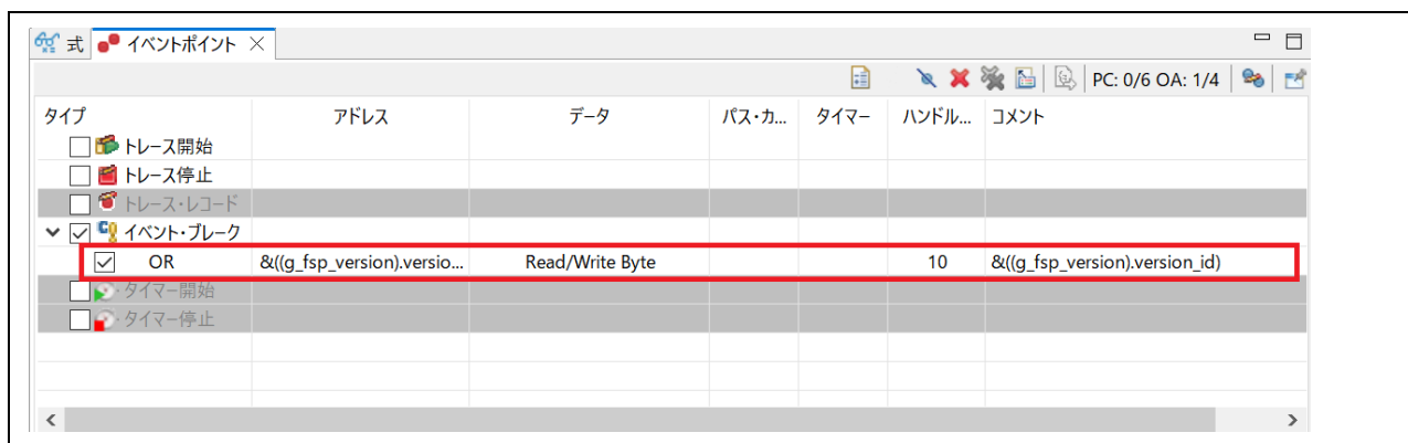
図 5-14 デバッグ – [イベントポイント] ビュー
