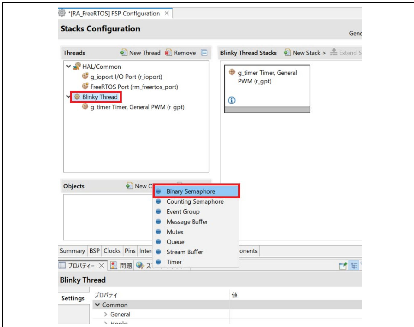
図 6-5 FreeRTOS アプリケーションの設定 – セマフォオブジェクトの追加
