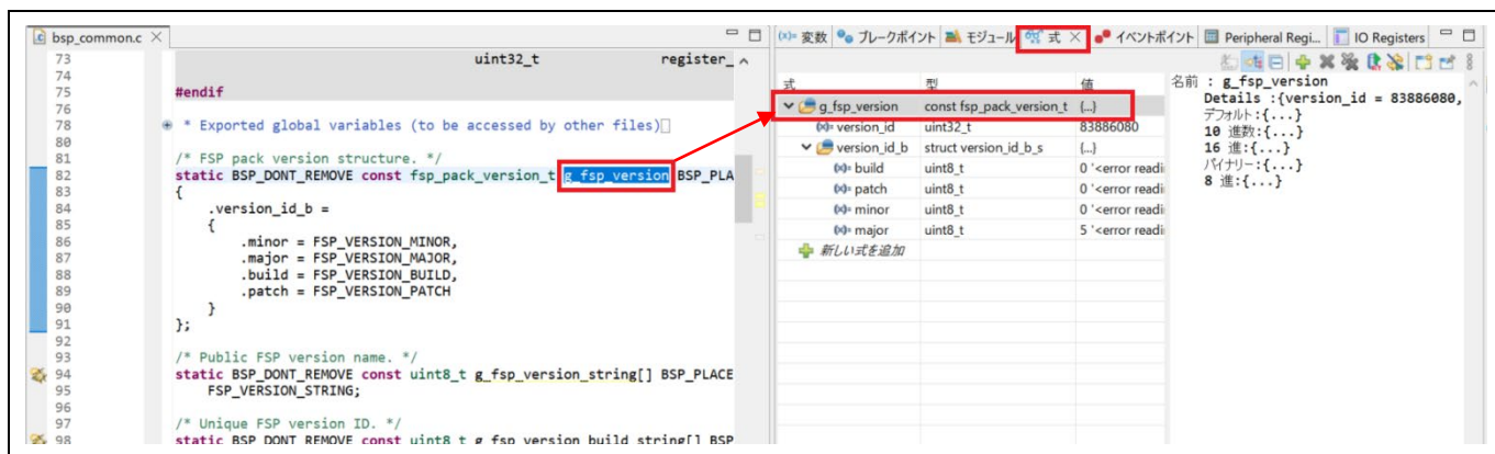
図 5-12 デバッグ - [式] ビュー
