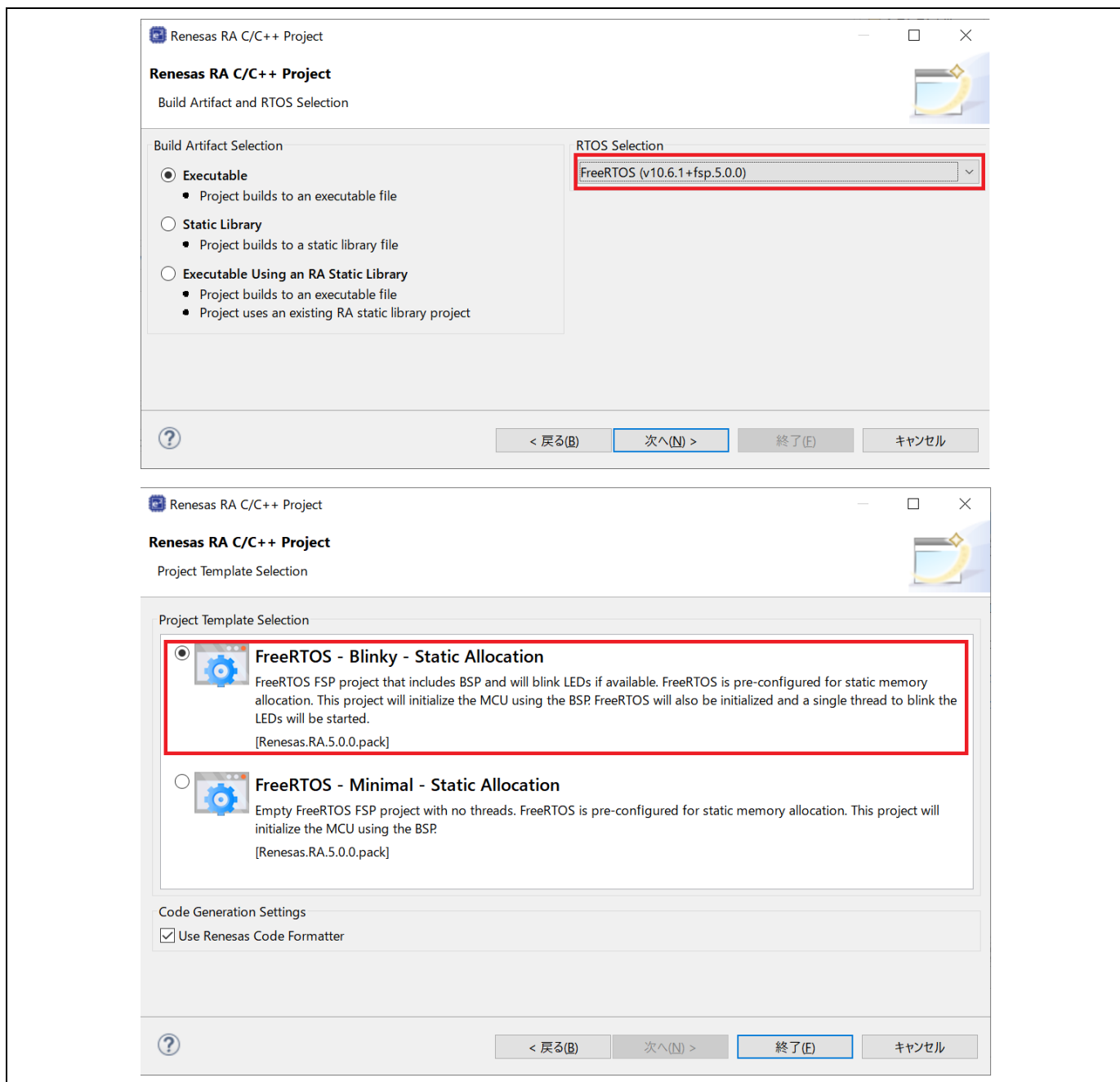
図 6-2 FreeRTOS アプリケーションの設定 – 新規プロジェクトの作成
