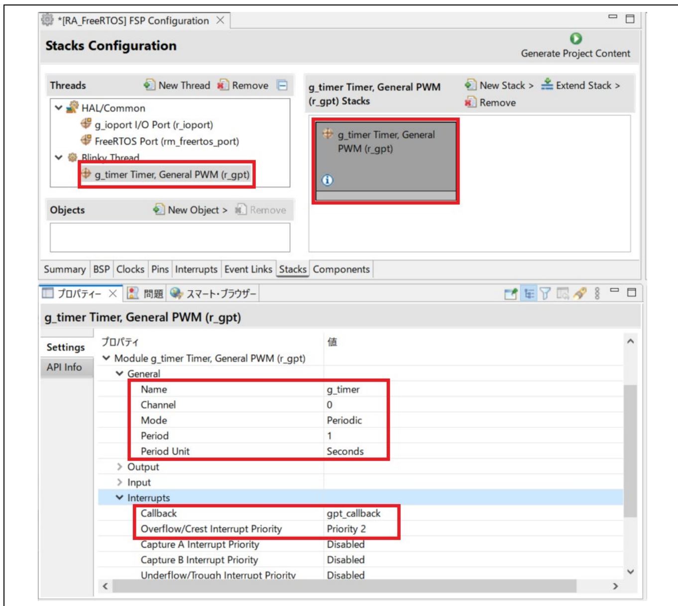
図 6-4 FreeRTOS アプリケーションの設定 – GPT モジュールの設定
