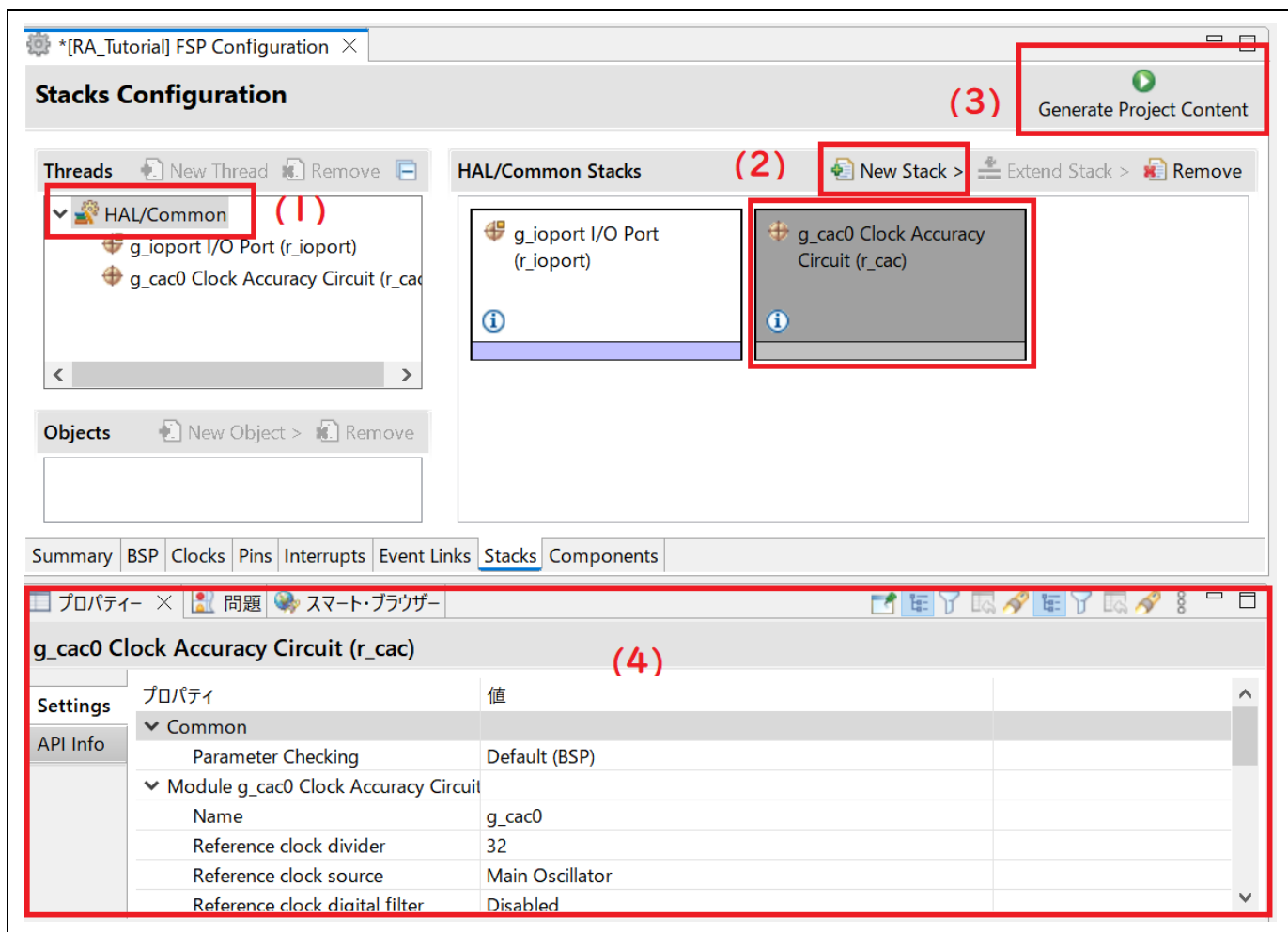
図 3-48 RA プロジェクト構成 - スレッドにモジュールを追加
