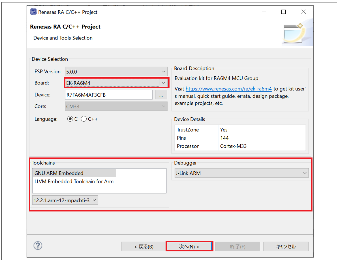
図 3-9 プロジェクトの作成 - デバイスの選択
