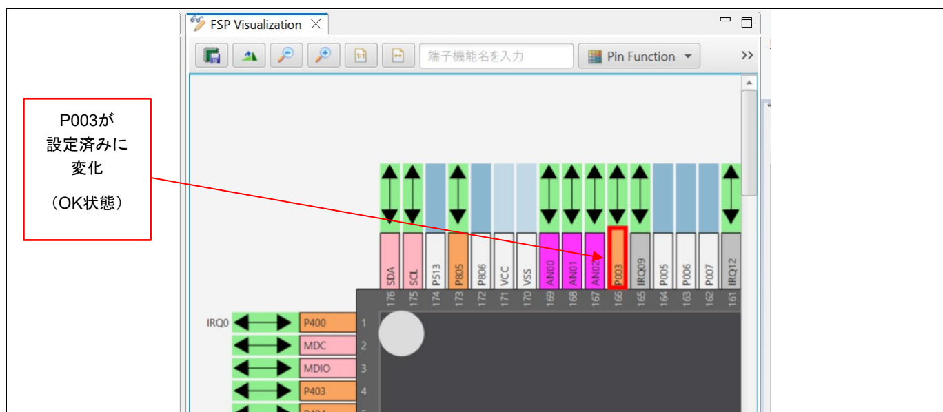
図 3-45 RA プロジェクト構成 – [Visualization] ビュー（接続状態）
