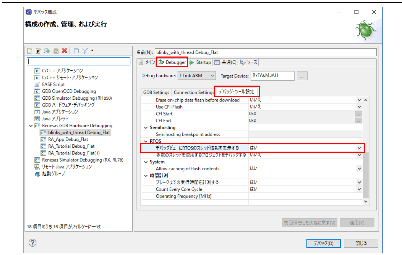
図5-10 デバッガー - デバッグ・ツール設定
