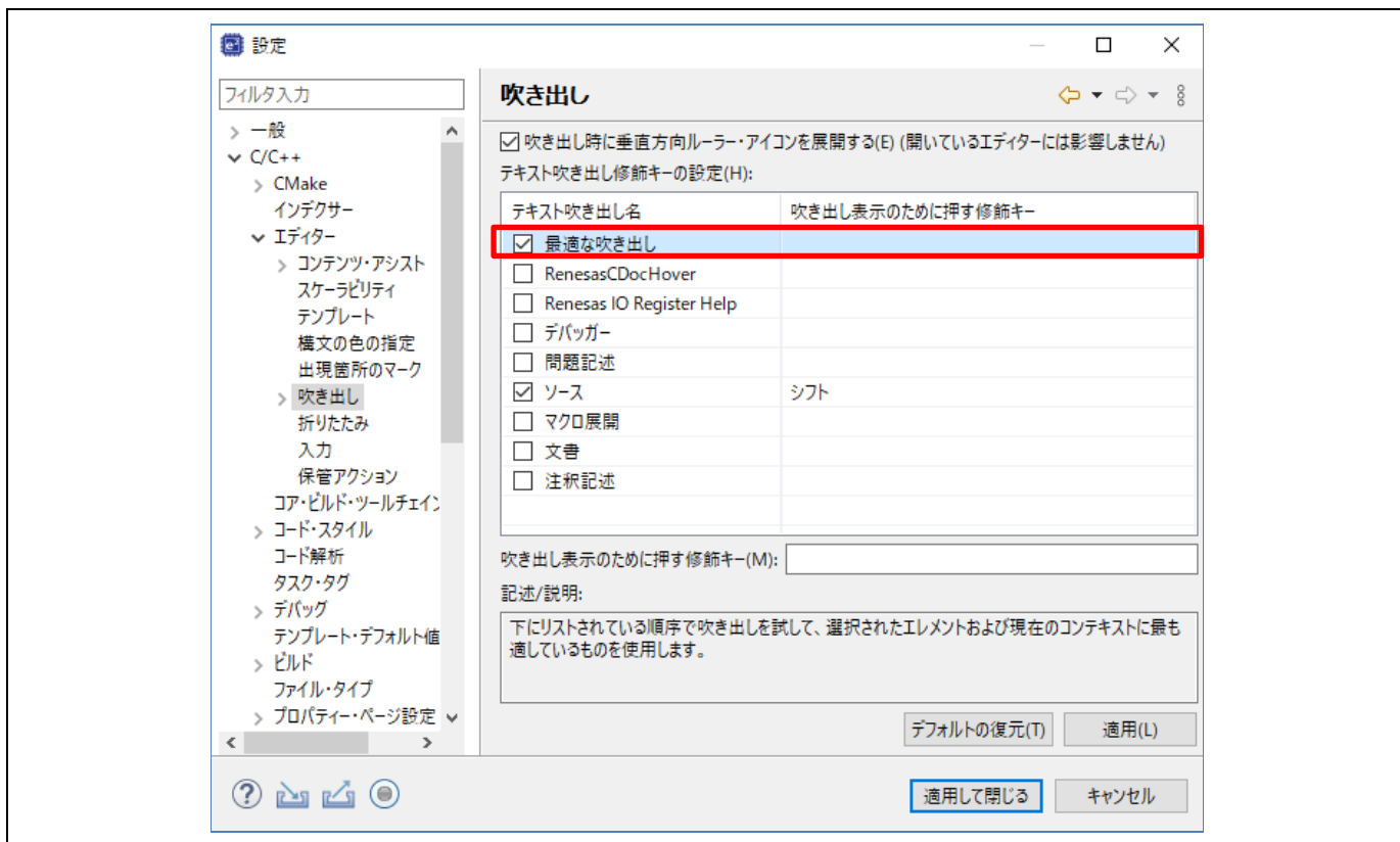
図 3-62 吹き出しの設定
