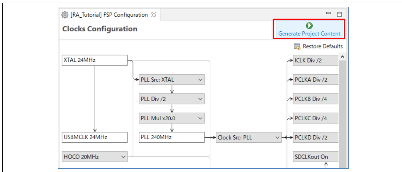
図 3-39 プロジェクト内容の生成
