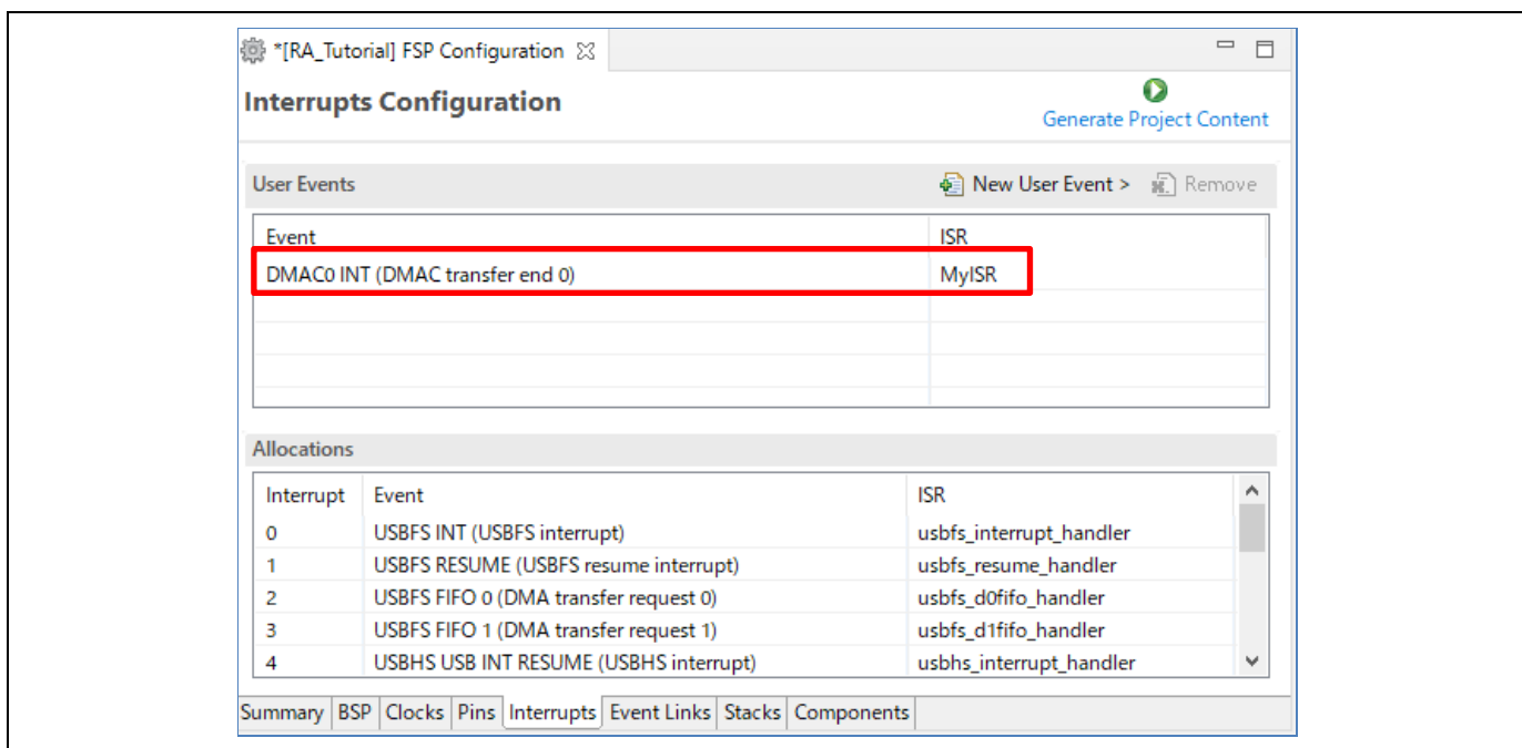
図 3-57 [Interrupts Configuration] ページ – ソースコードの生成
