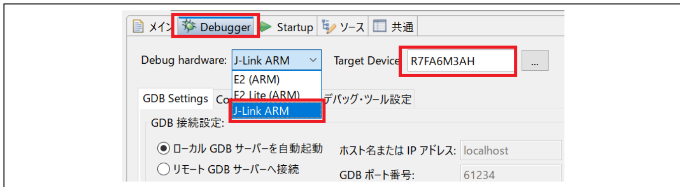
図 5-4 デバッグ – 接続設定の変更
