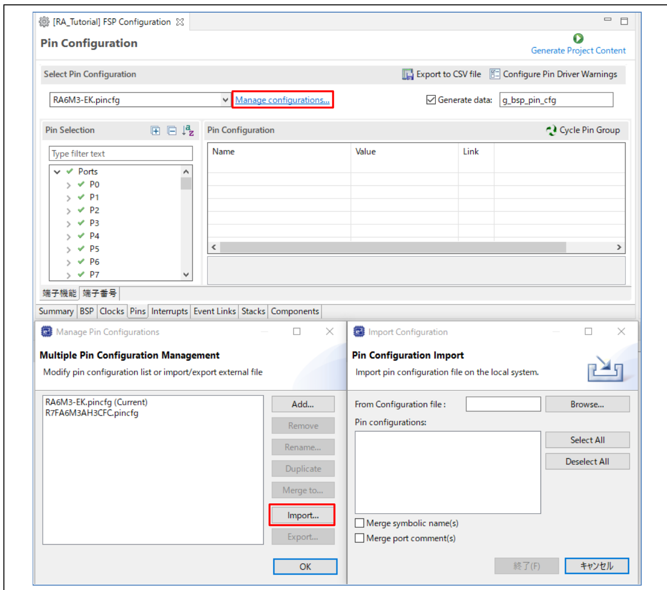
図 3-46 既存の端子構成を現在のプロジェクトにインポート
