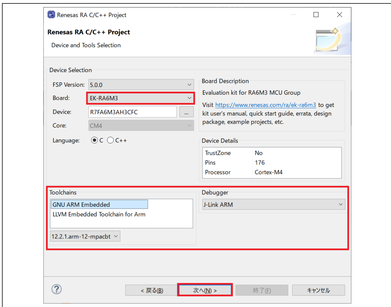
図 3-4 プロジェクトの作成 – デバイスの選択
