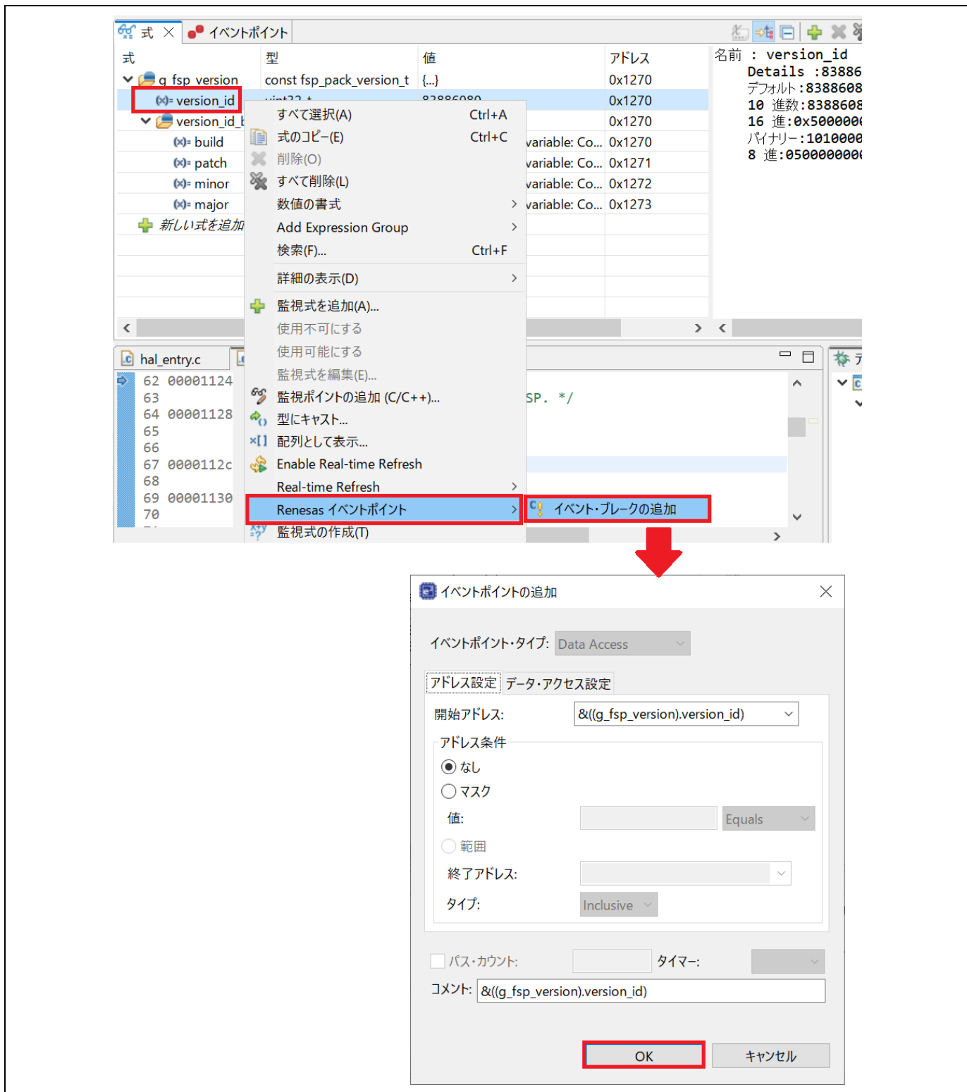
図 5-13 デバッガー イベントポイントとして設定
