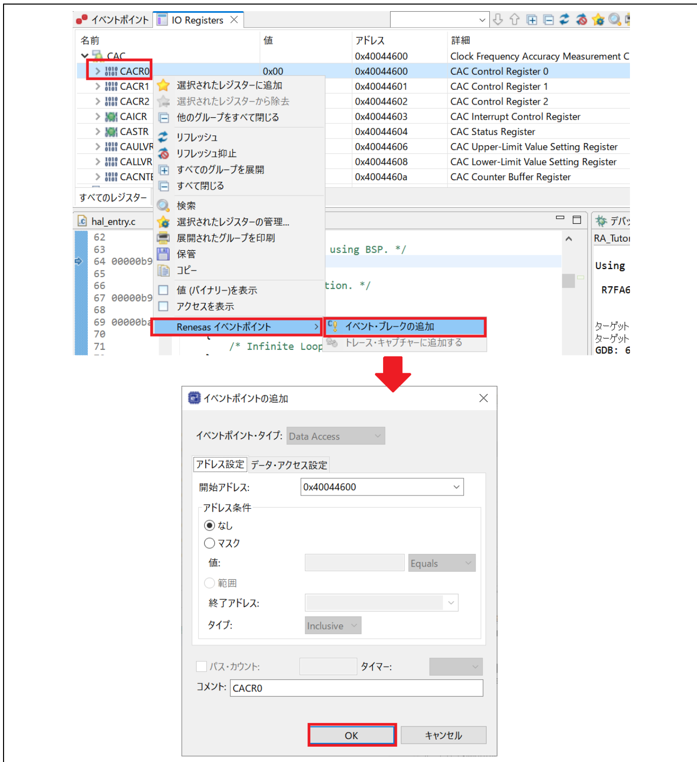
図 5-25 デバッガー イベントポイントとして設定
