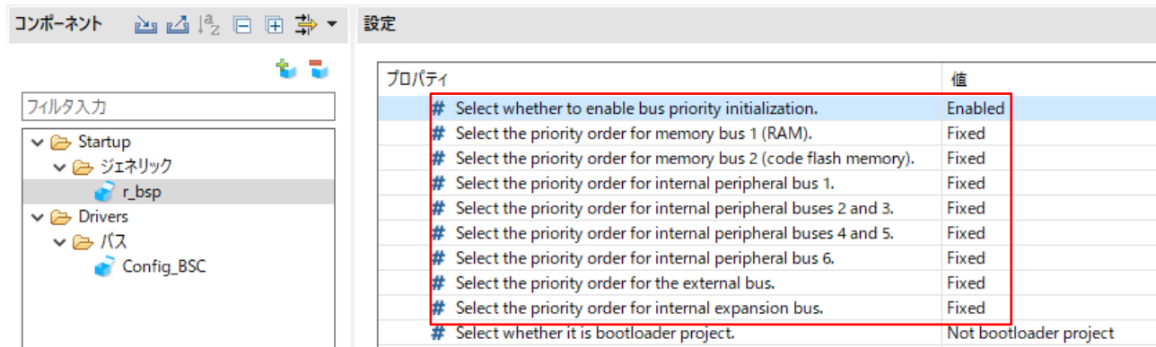
図 5-6 BSP のバス優先度設定
