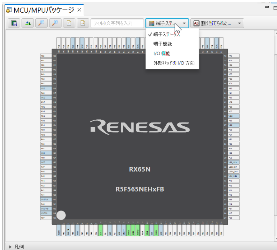
図 2-2 MCU パッケージビューの入出力表示
