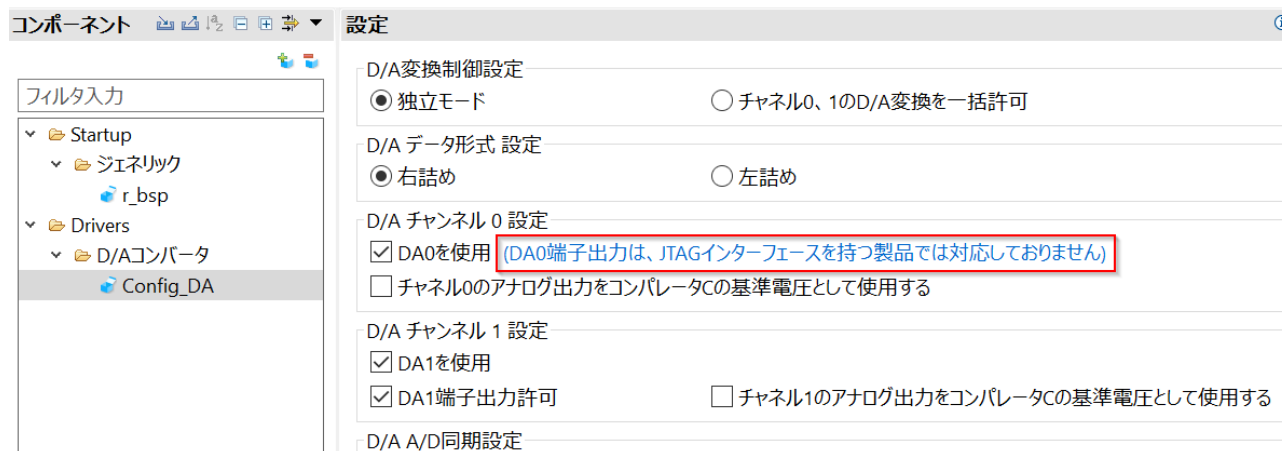
図 3-1 D/A コンバータの設定
