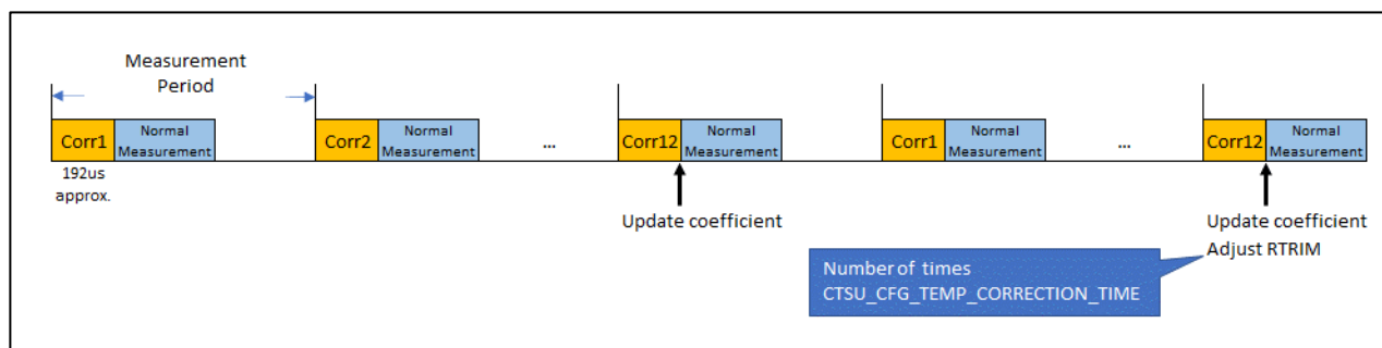
図 12 温度補正計測タイミングチャート
