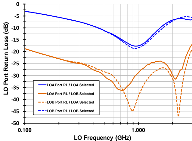
LO Port Return Loss
