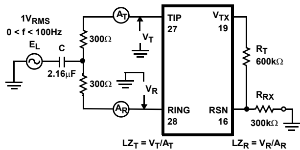
FIGURE 2. LONGITUDINAL IMPEDANCE
