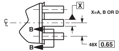
VIEW Y
