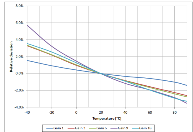
Figure 2.4 ALS vs. Temperature at 1000 lux
