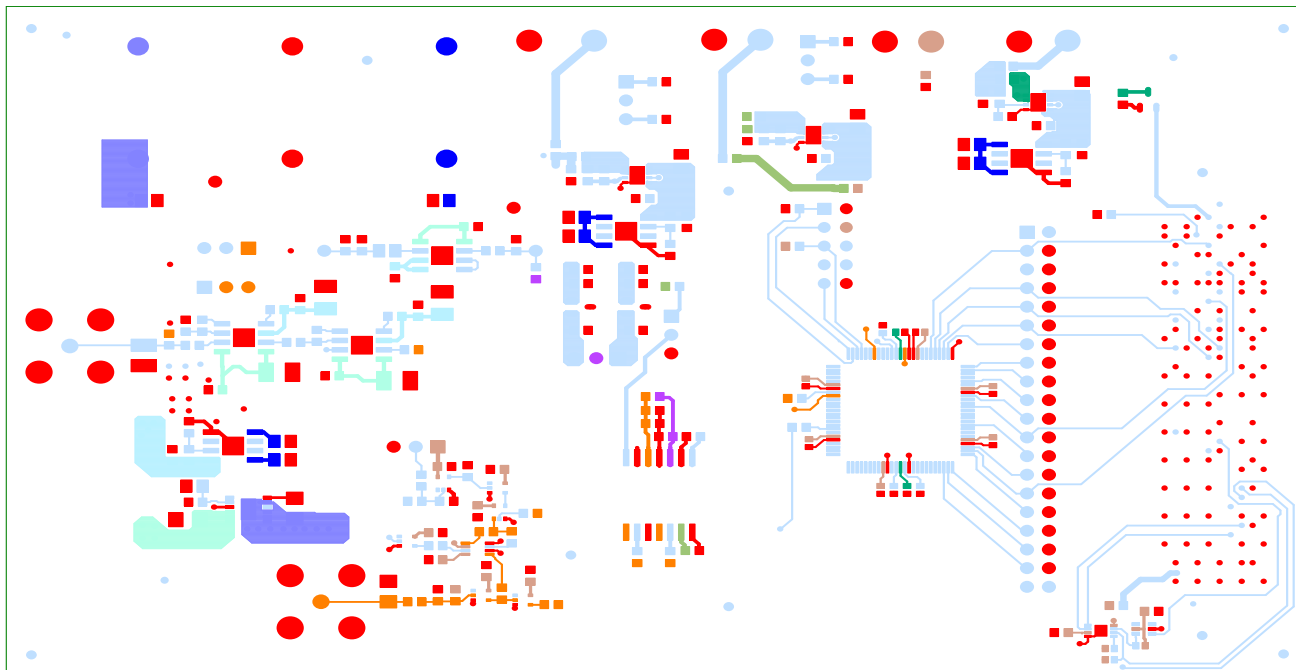
Figure 22. Top Layer
