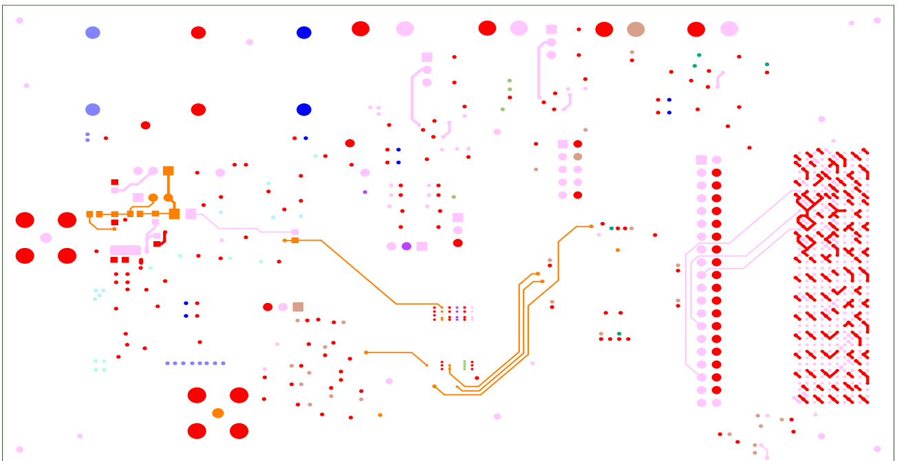
Figure 29. Bottom Layer
