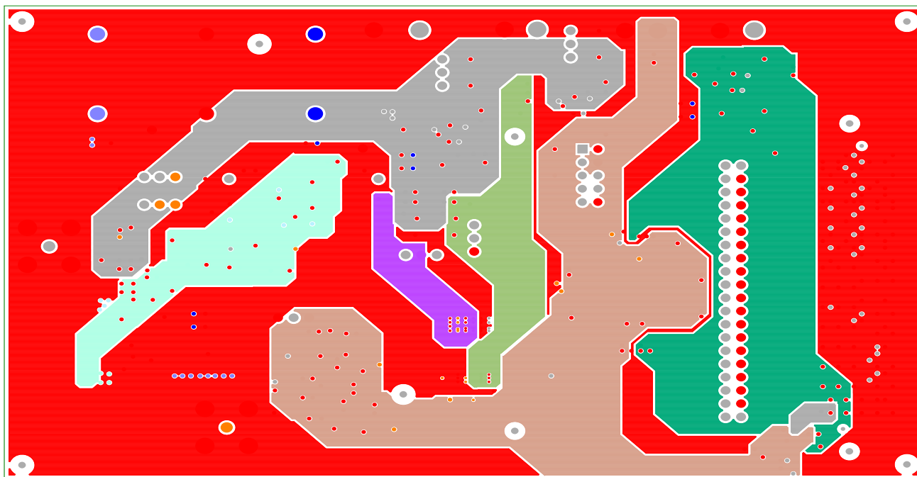
Figure 24. Layer 3
