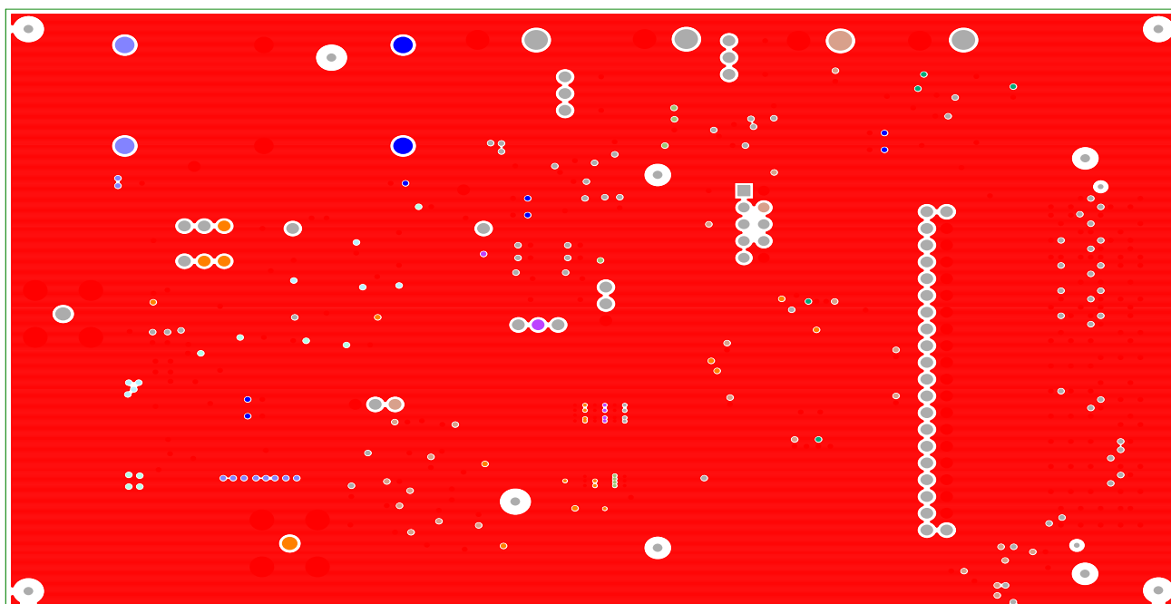
Figure 25. Layer 4
