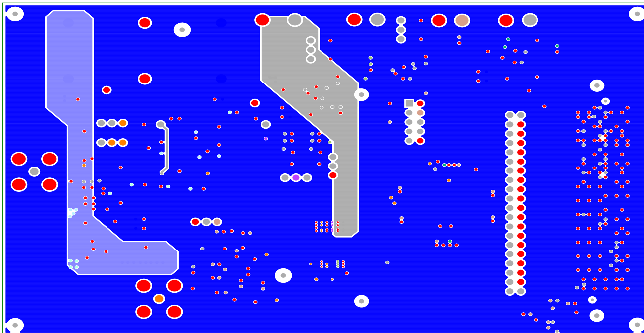
Figure 26. Layer 5
