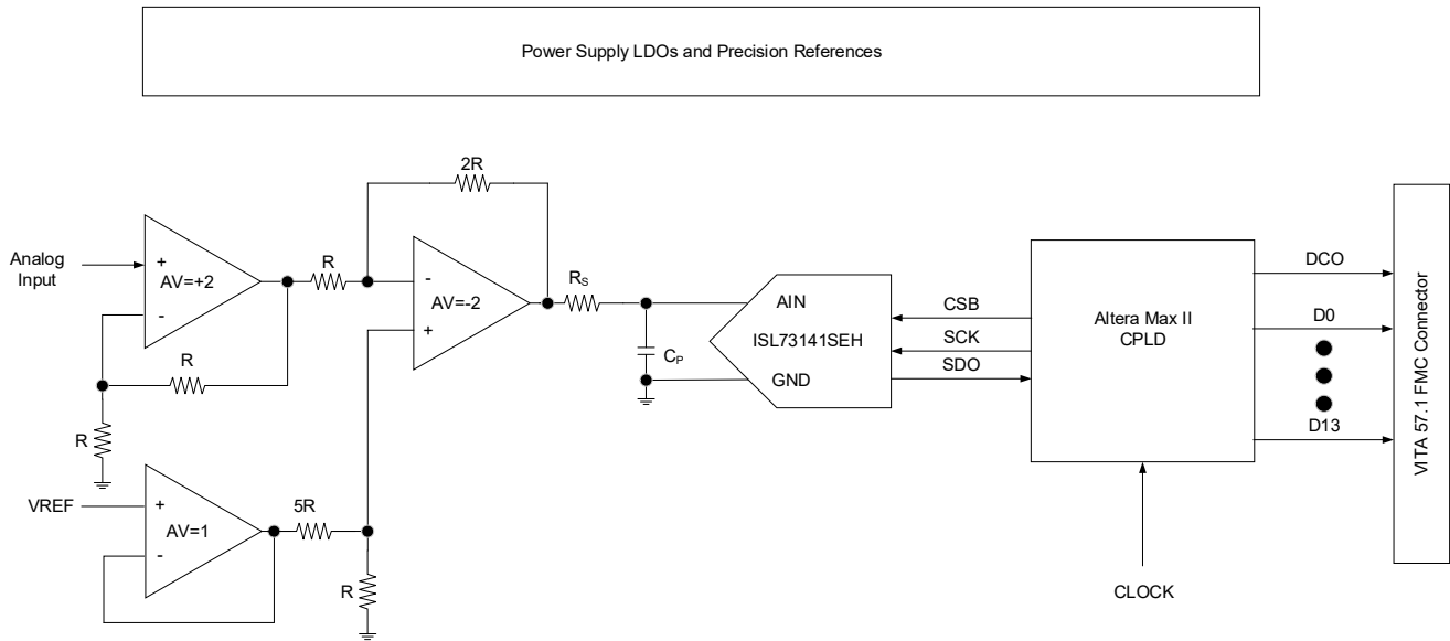
Figure 1. ISL73141SEHF7EV1Z and ISL73141SEHFNEV1Z Block Diagram
