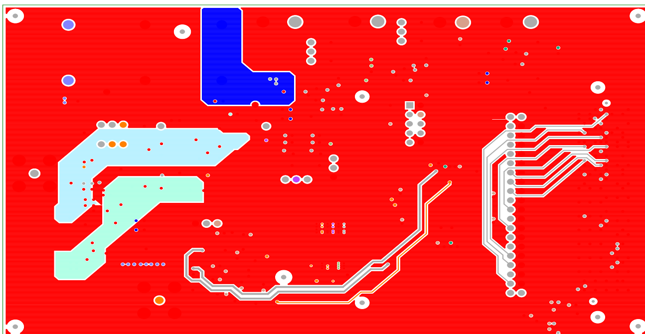
Figure 27. Layer 6
