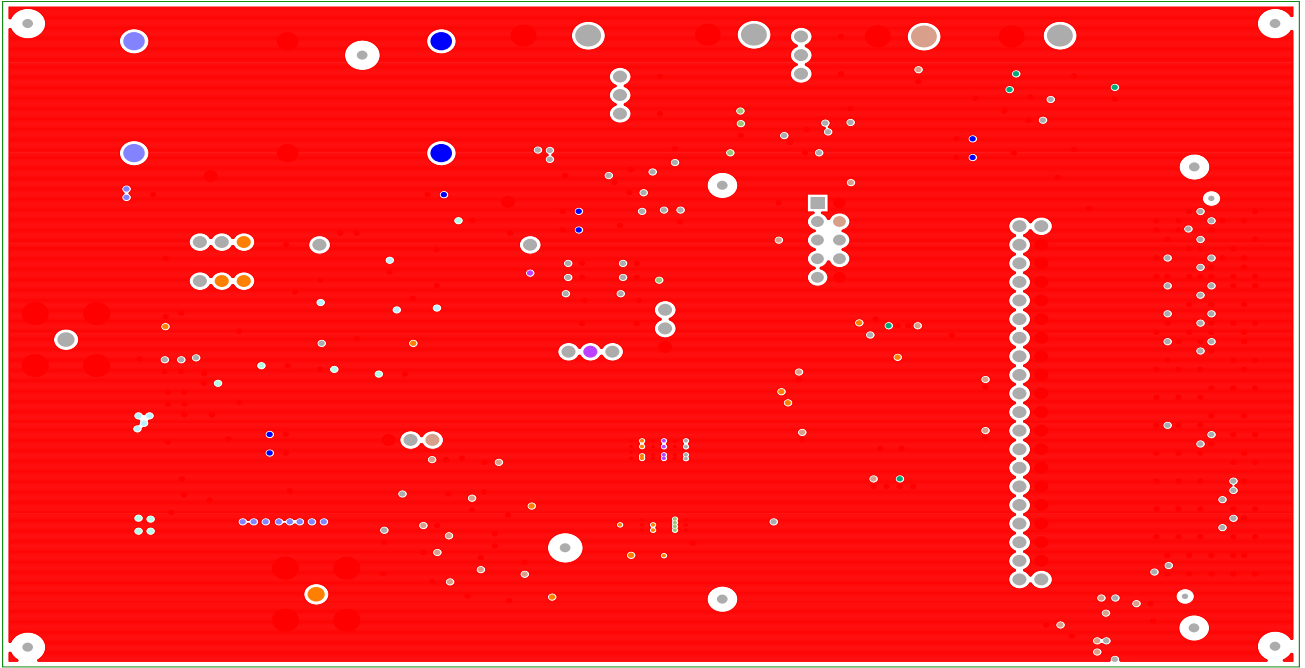
Figure 28. Layer 7
