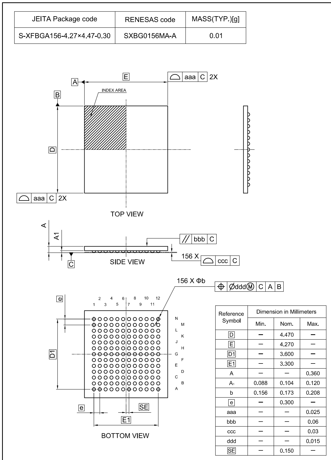
図 A.3 156ピンWLBGA (SXBG0156MA-A)
